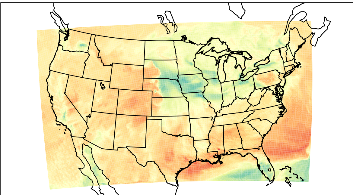
WRF (2023-03-05_20:00:00)
