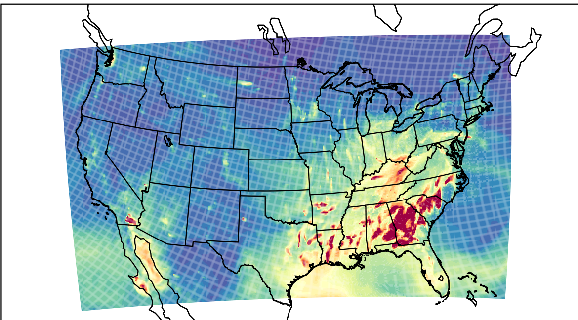
WRF 2023-03-07_04:00:00
