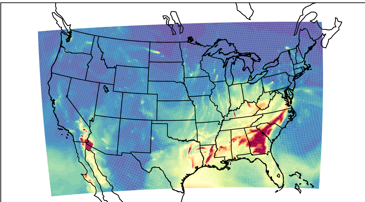
WRF 2023-03-07_08:00:00
