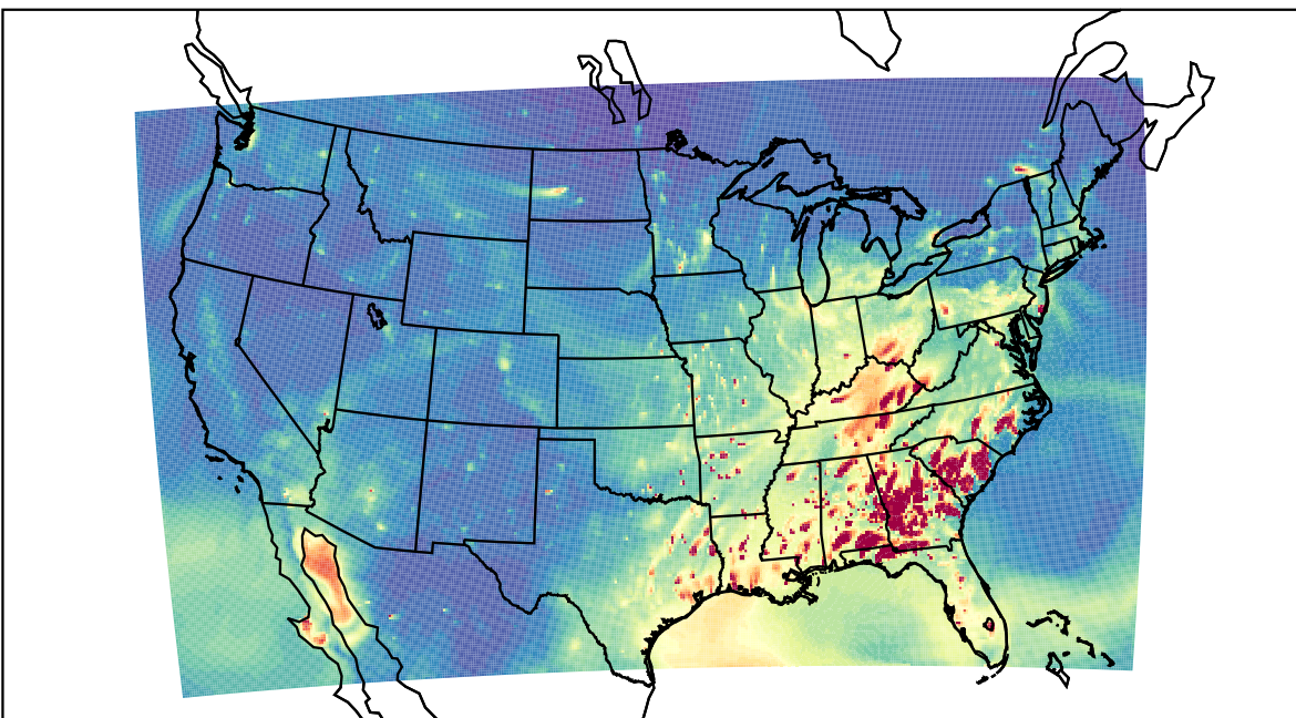
WRF 2023-03-07_01:00:00
