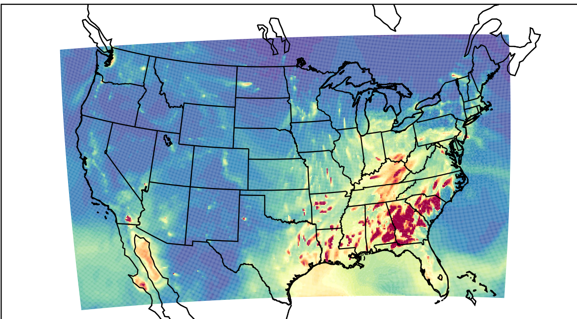
WRF 2023-03-07_03:00:00
