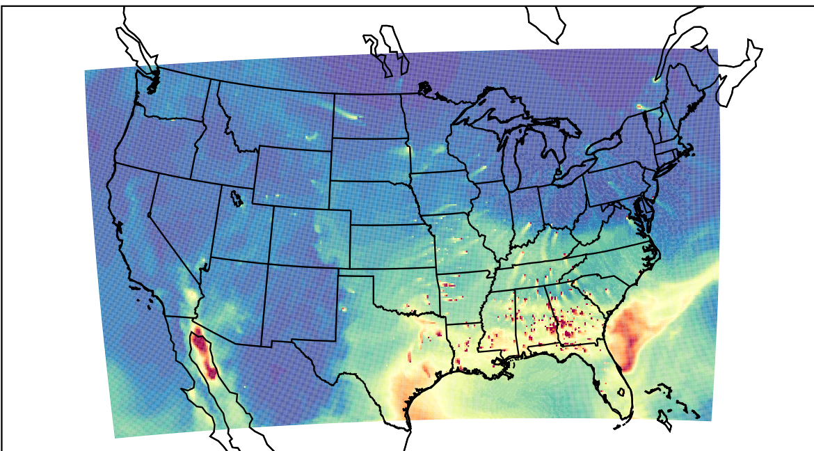
WRF 2023-03-07_20:00:00
