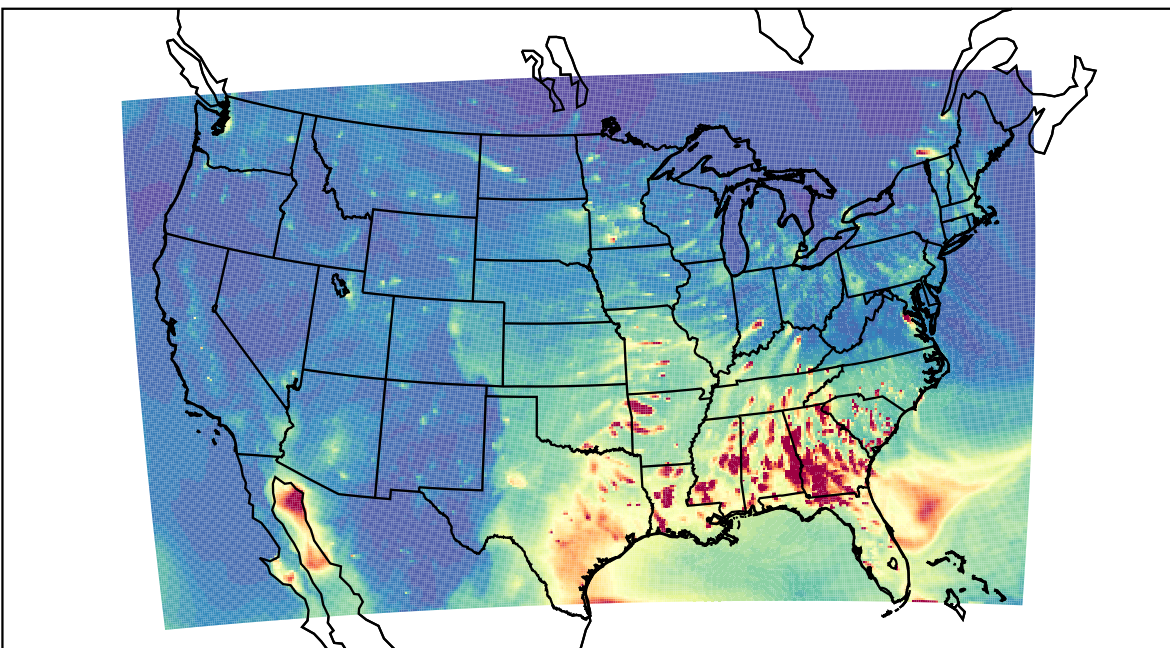
WRF 2023-03-08_01:00:00
