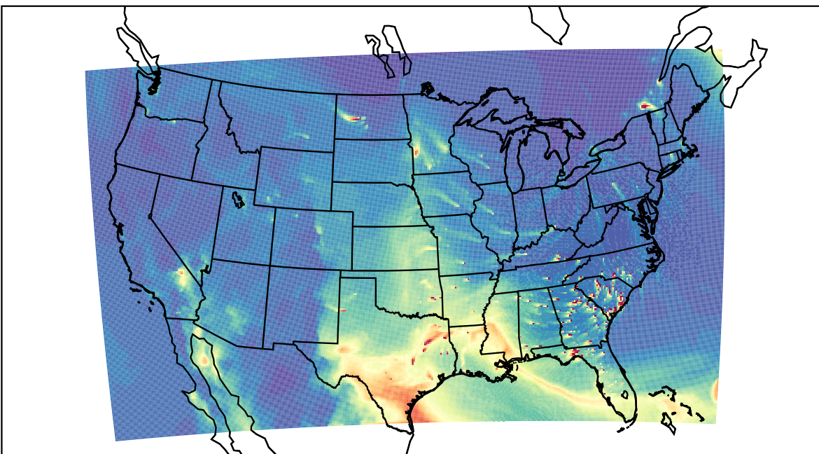
WRF 2023-03-08_19:00:00
