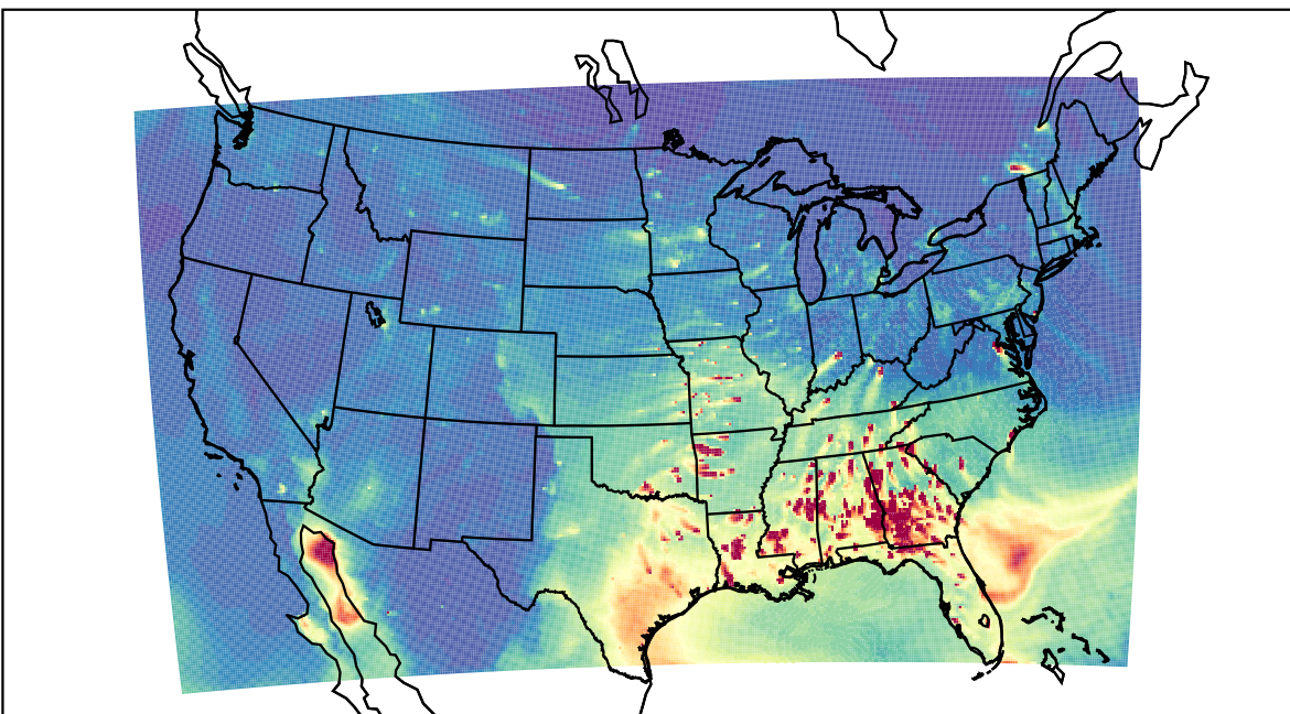
WRF 2023-03-08_00:00:00
