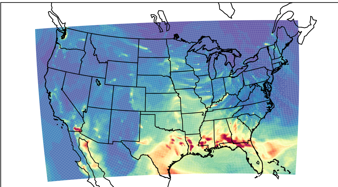
WRF 2023-03-08_06:00:00
