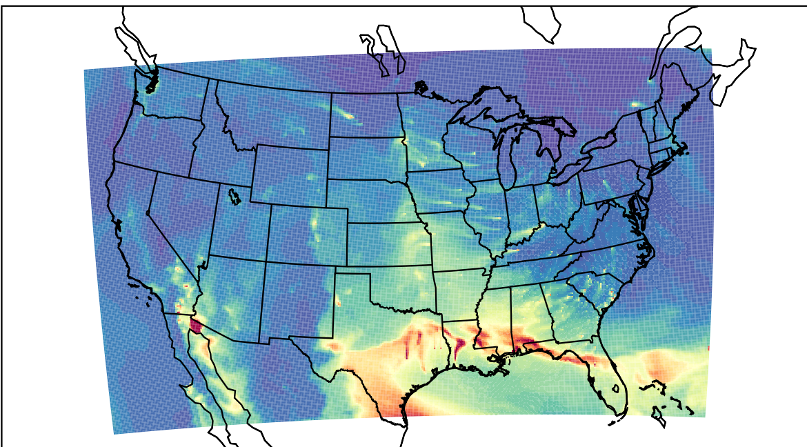
WRF 2023-03-08_10:00:00
