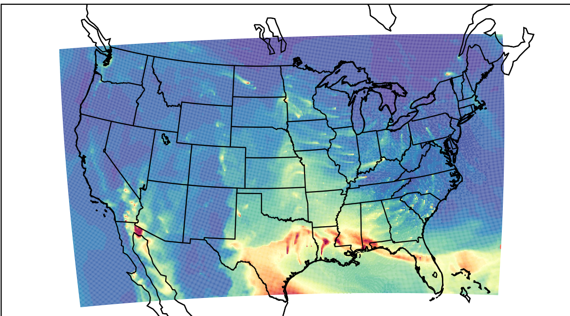
WRF 2023-03-08_11:00:00
