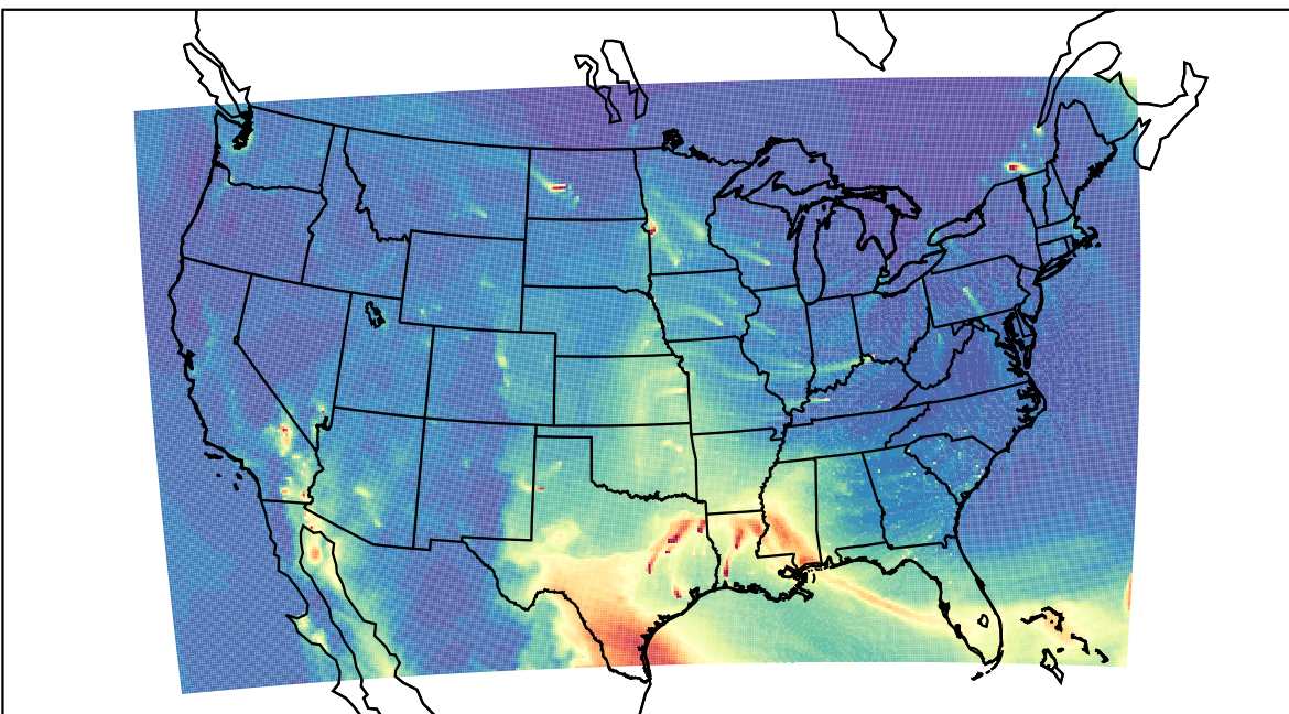
WRF 2023-03-08_16:00:00
