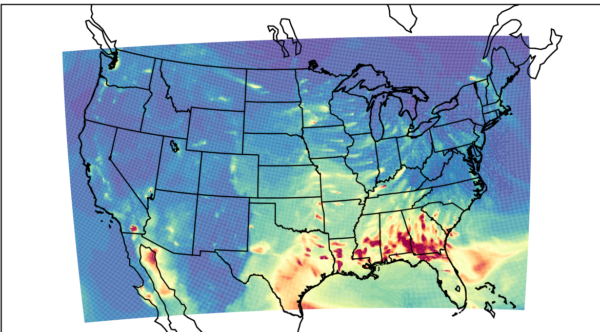
WRF 2023-03-08_04:00:00
