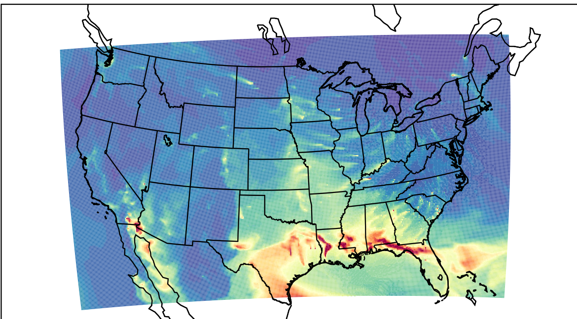
WRF 2023-03-08_08:00:00
