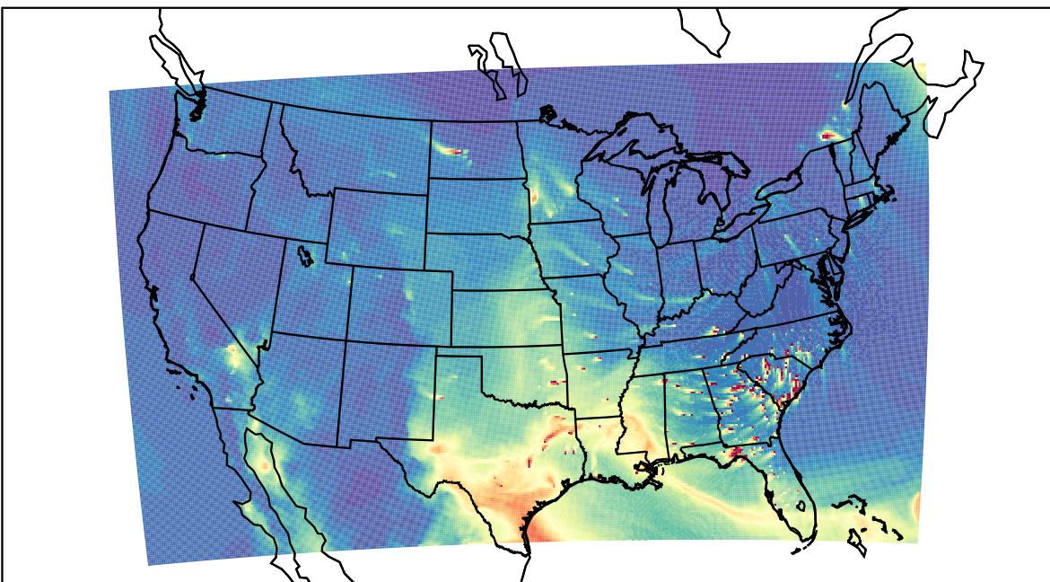
WRF 2023-03-08_20:00:00
