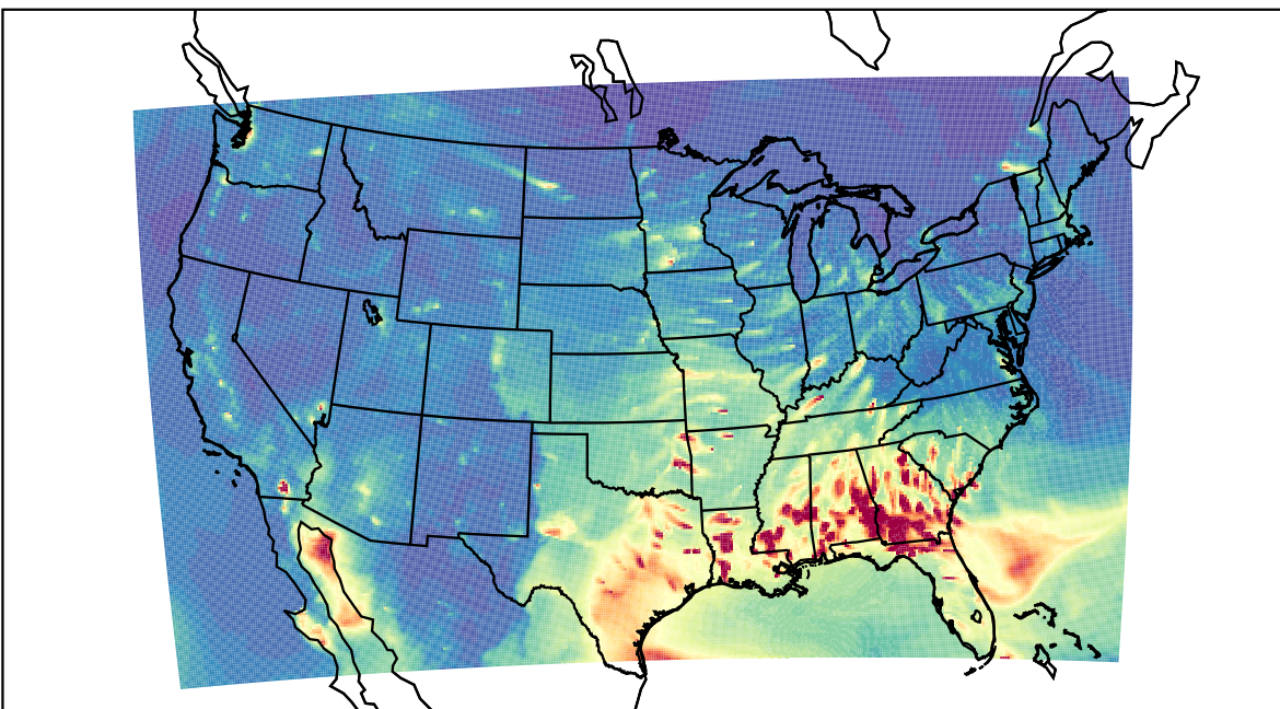
WRF 2023-03-08_03:00:00
