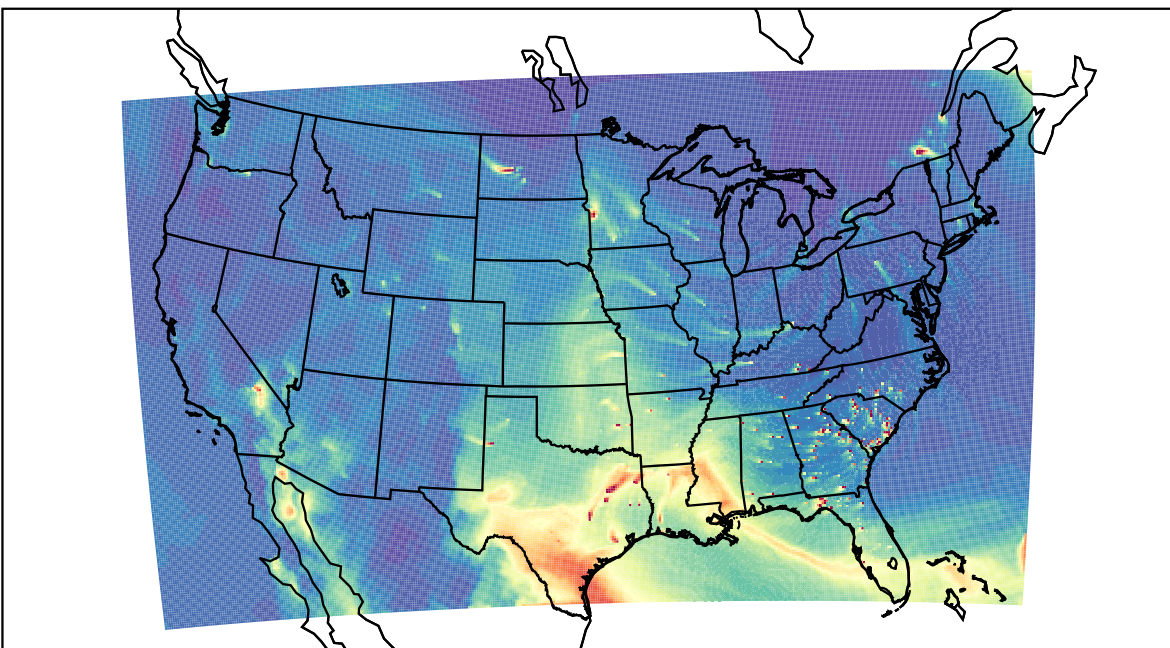
WRF 2023-03-08_18:00:00
