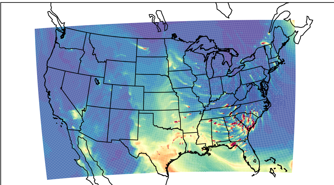
WRF 2023-03-08_22:00:00
