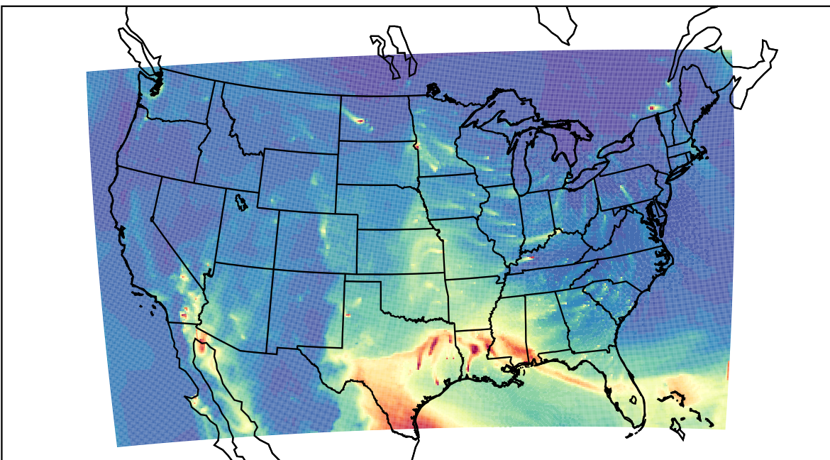
WRF 2023-03-08_13:00:00
