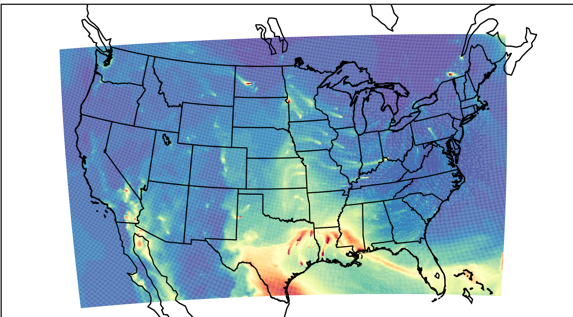
WRF 2023-03-08_15:00:00
