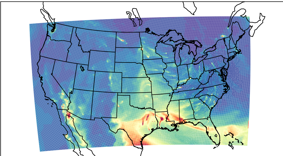
WRF 2023-03-08_12:00:00
