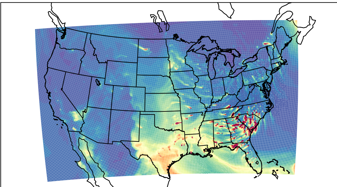
WRF 2023-03-08_23:00:00
