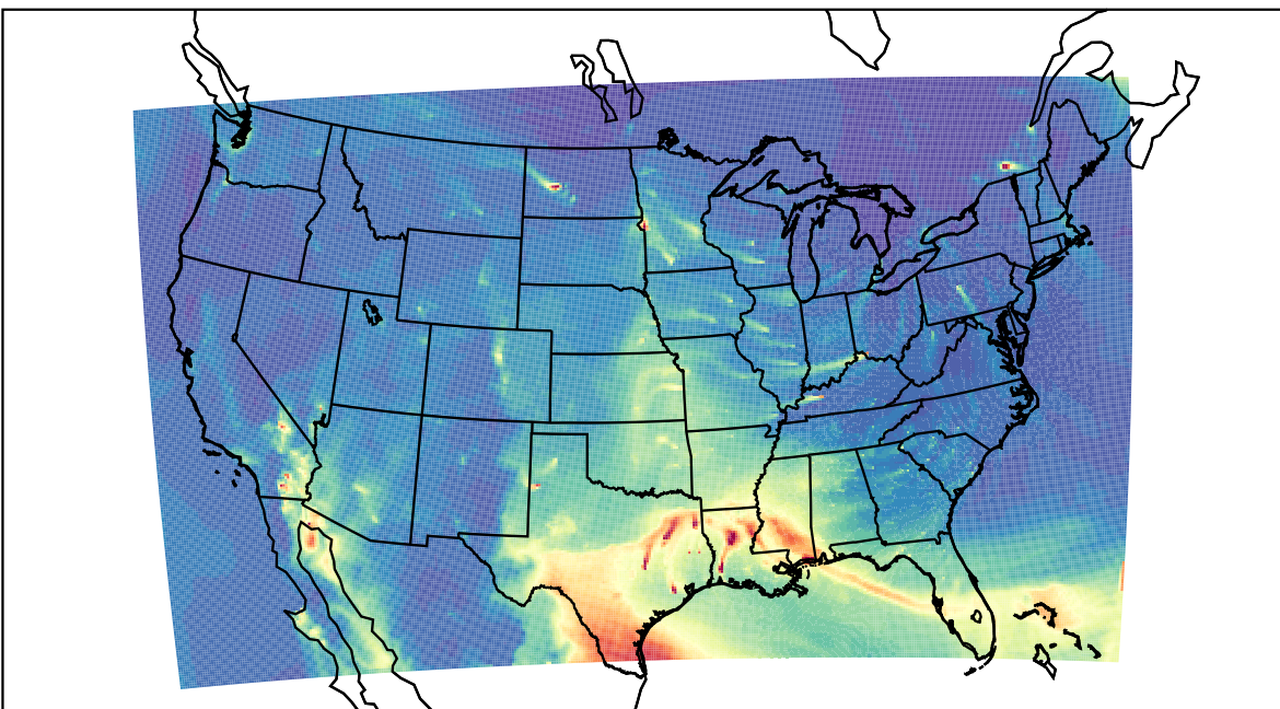
WRF 2023-03-08_14:00:00
