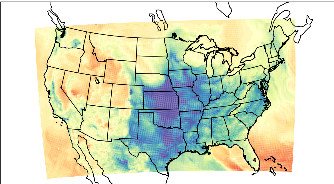
WRF (2023-03-09_06:00:00)
