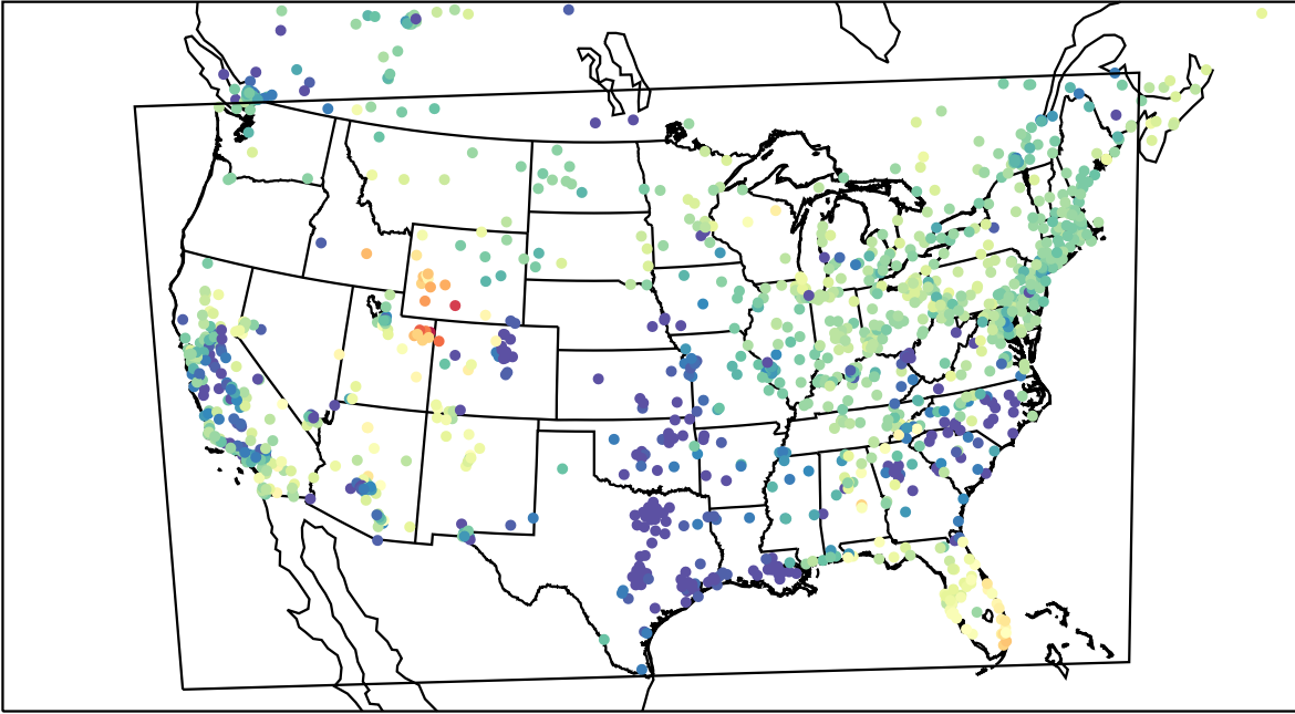
AirNOW (2023-03-09_03:00:00)
