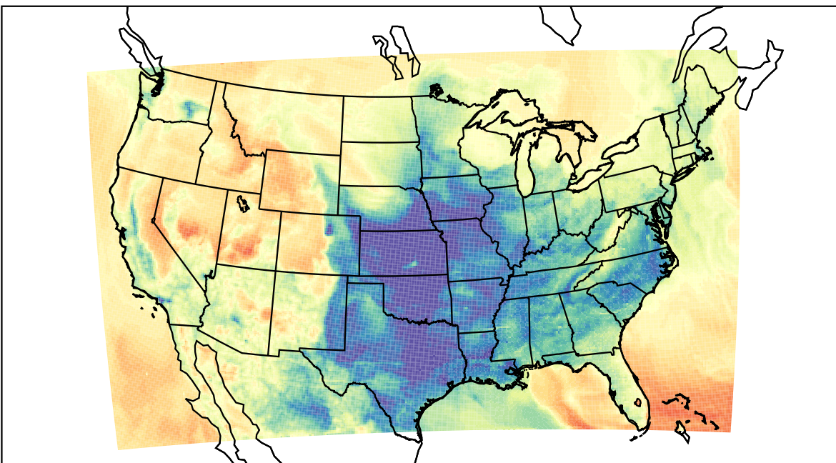
WRF (2023-03-09_09:00:00)
