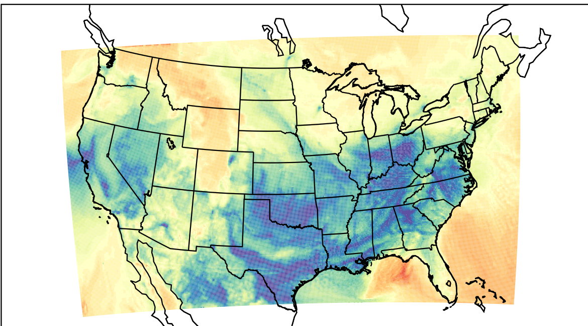
WRF (2023-03-10_14:00:00)
