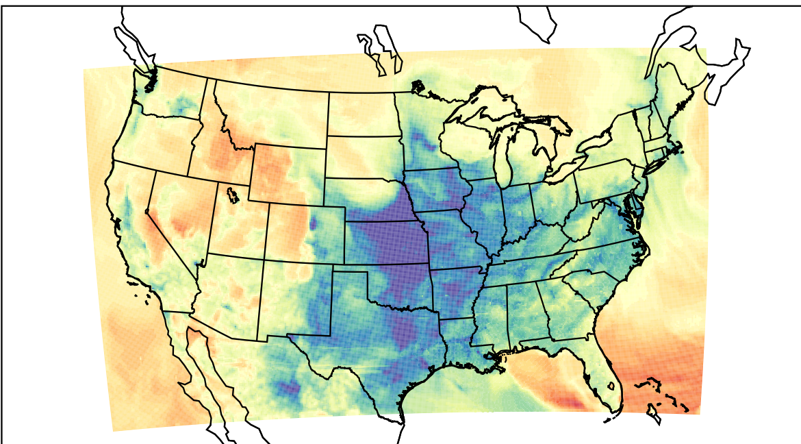
WRF (2023-03-09_04:00:00)
