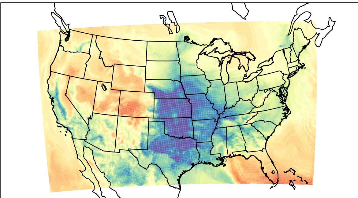
WRF (2023-03-09_16:00:00)
