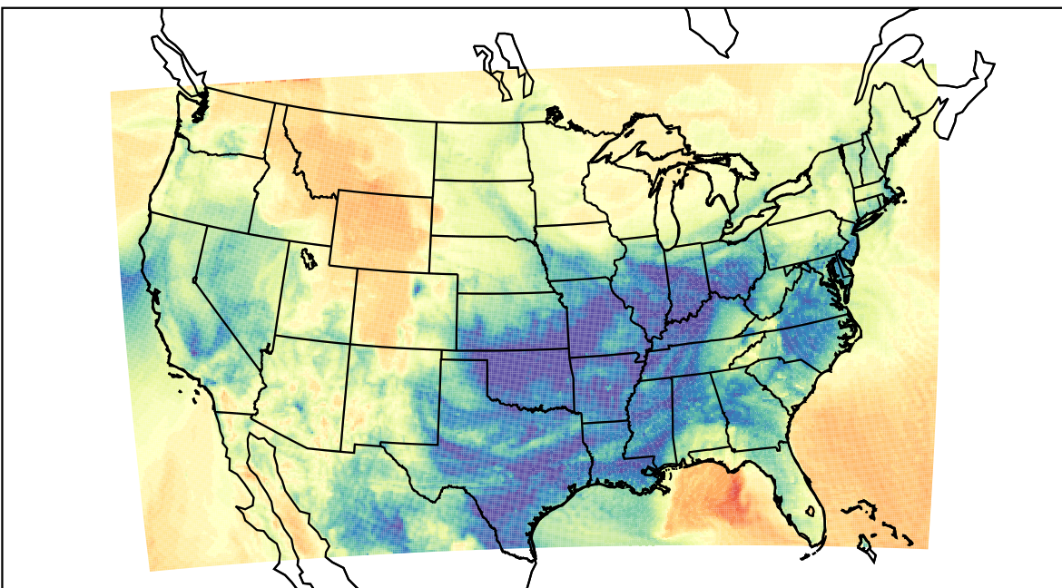
WRF (2023-03-10_10:00:00)
