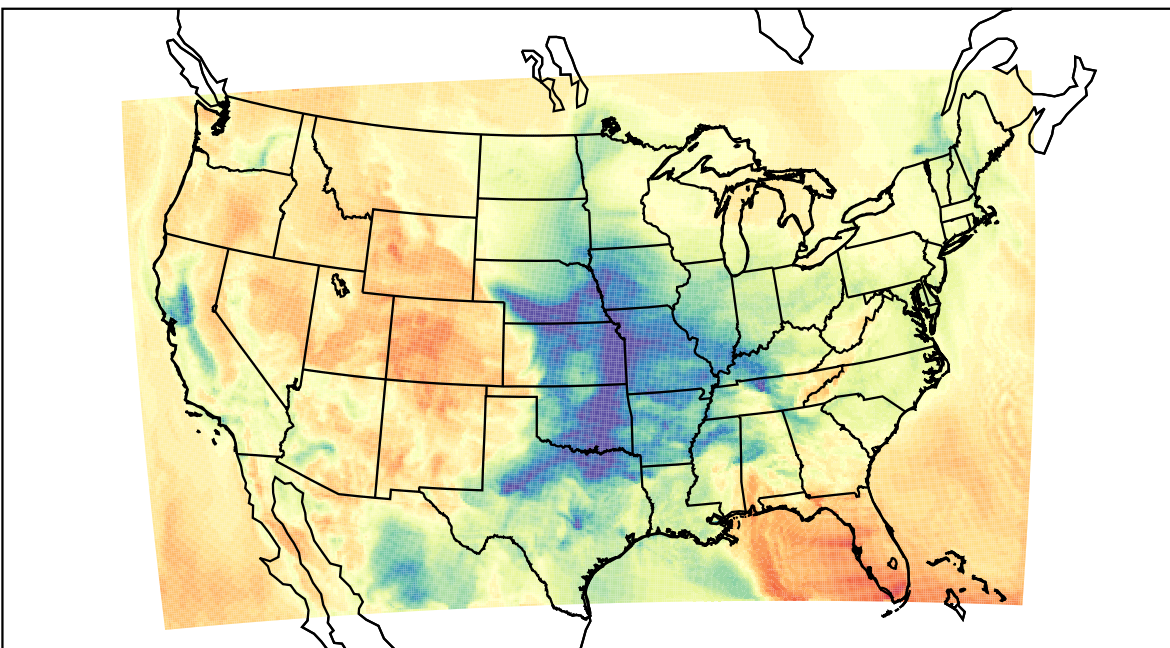
WRF (2023-03-09_18:00:00)
