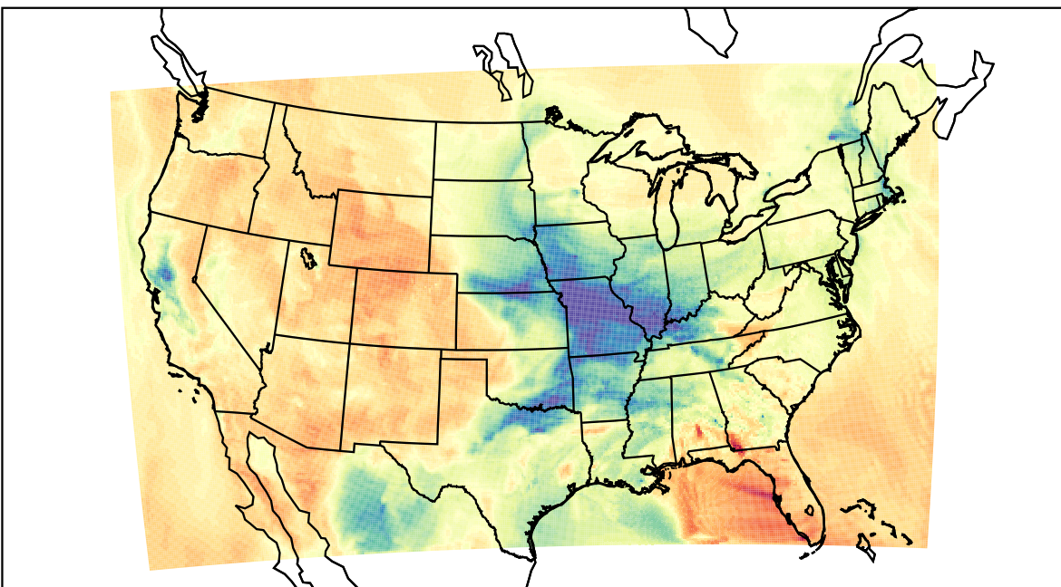
WRF (2023-03-09_22:00:00)
