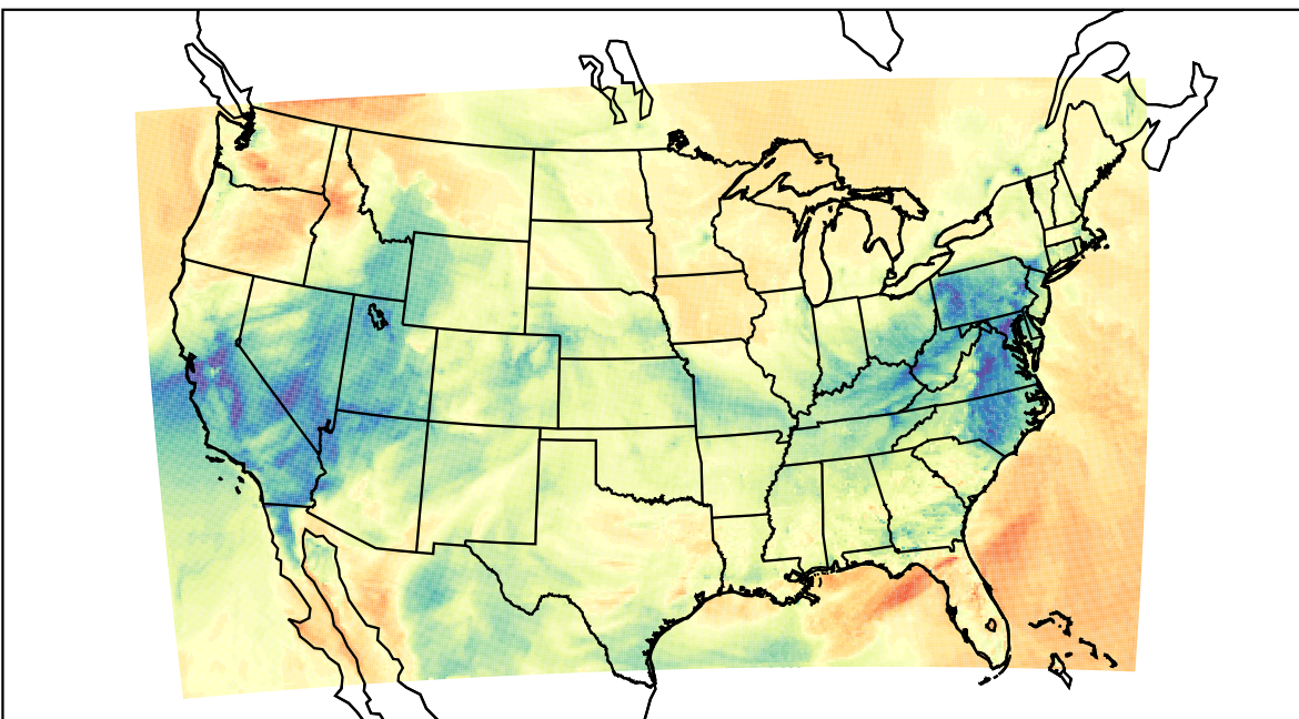
WRF (2023-03-10_23:00:00)
