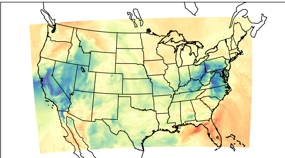
WRF (2023-03-10_20:00:00)
