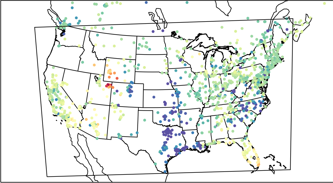
AirNOW (2023-03-09_01:00:00)
