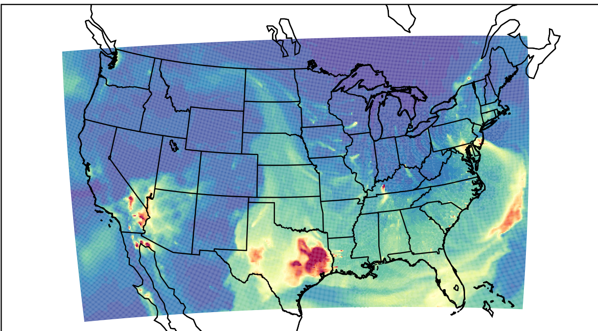
WRF 2023-03-11_10:00:00
