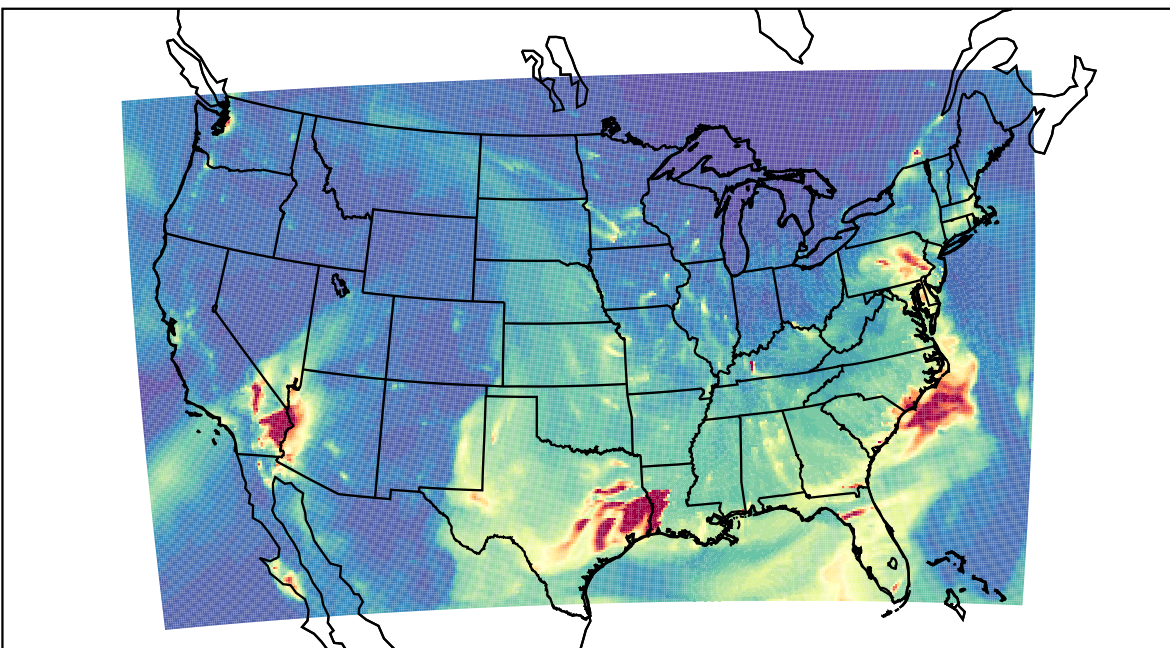
WRF 2023-03-11_04:00:00
