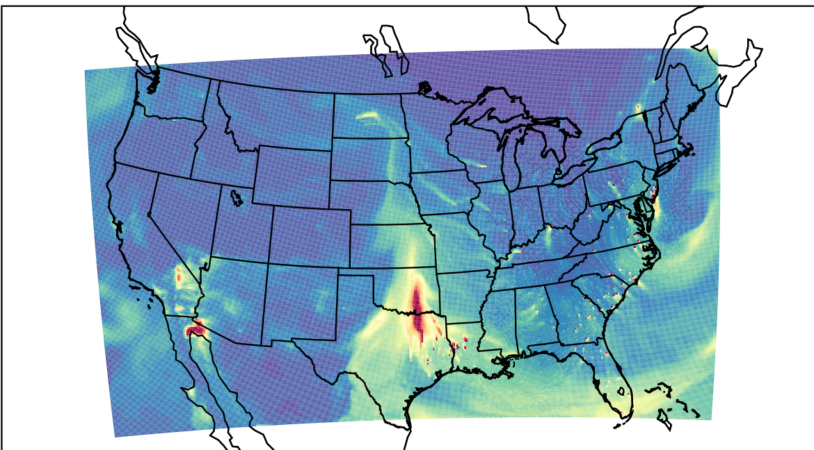
WRF 2023-03-11_19:00:00
