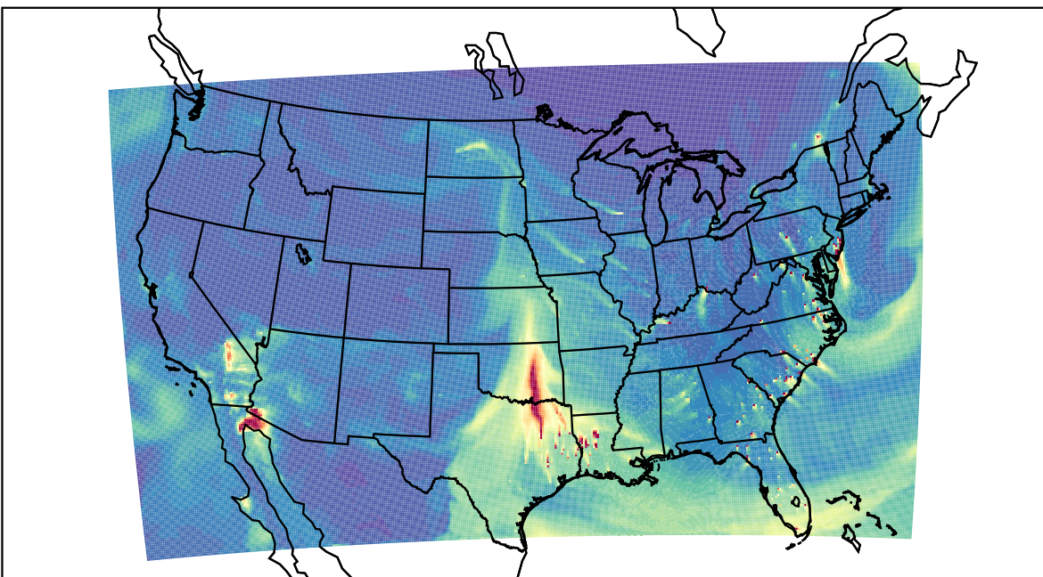
WRF 2023-03-11_20:00:00
