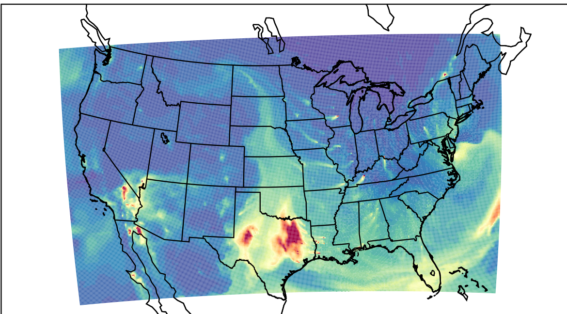
WRF 2023-03-11_14:00:00
