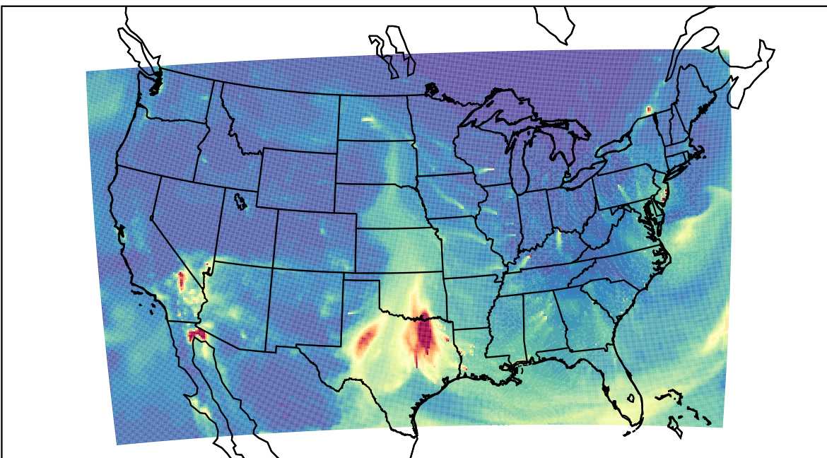
WRF 2023-03-11_16:00:00
