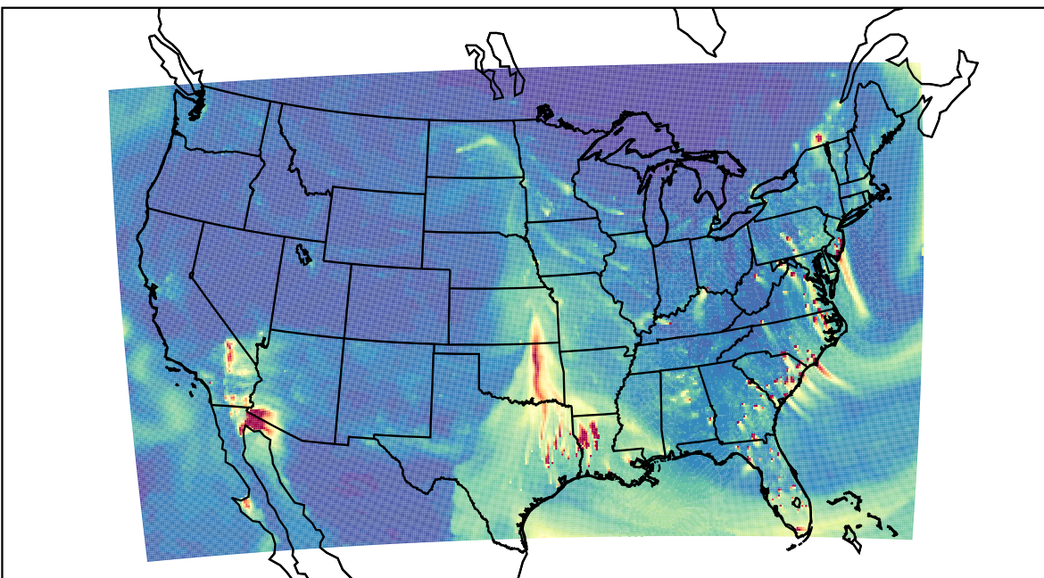
WRF 2023-03-11_23:00:00
