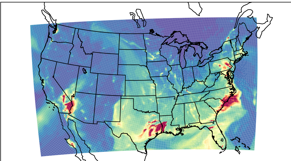
WRF 2023-03-11_03:00:00
