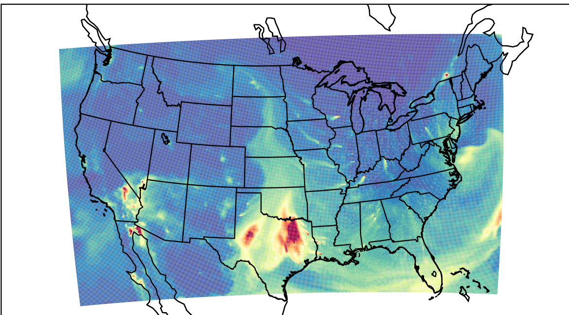
WRF 2023-03-11_15:00:00
