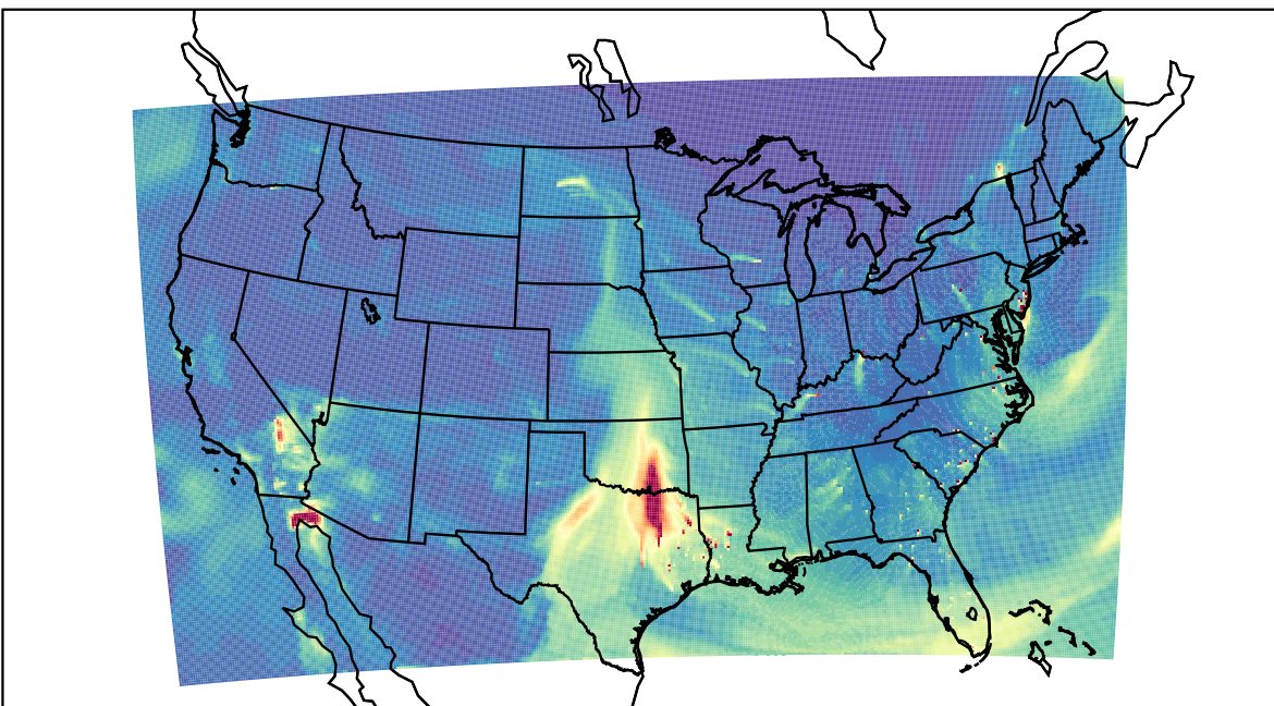
WRF 2023-03-11_18:00:00
