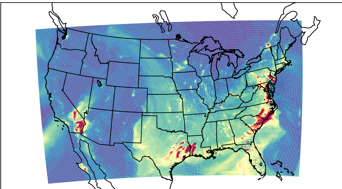
WRF 2023-03-11_01:00:00
