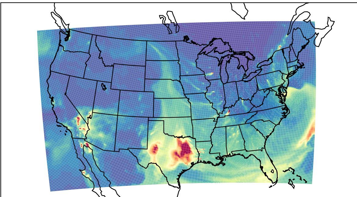
WRF 2023-03-11_13:00:00
