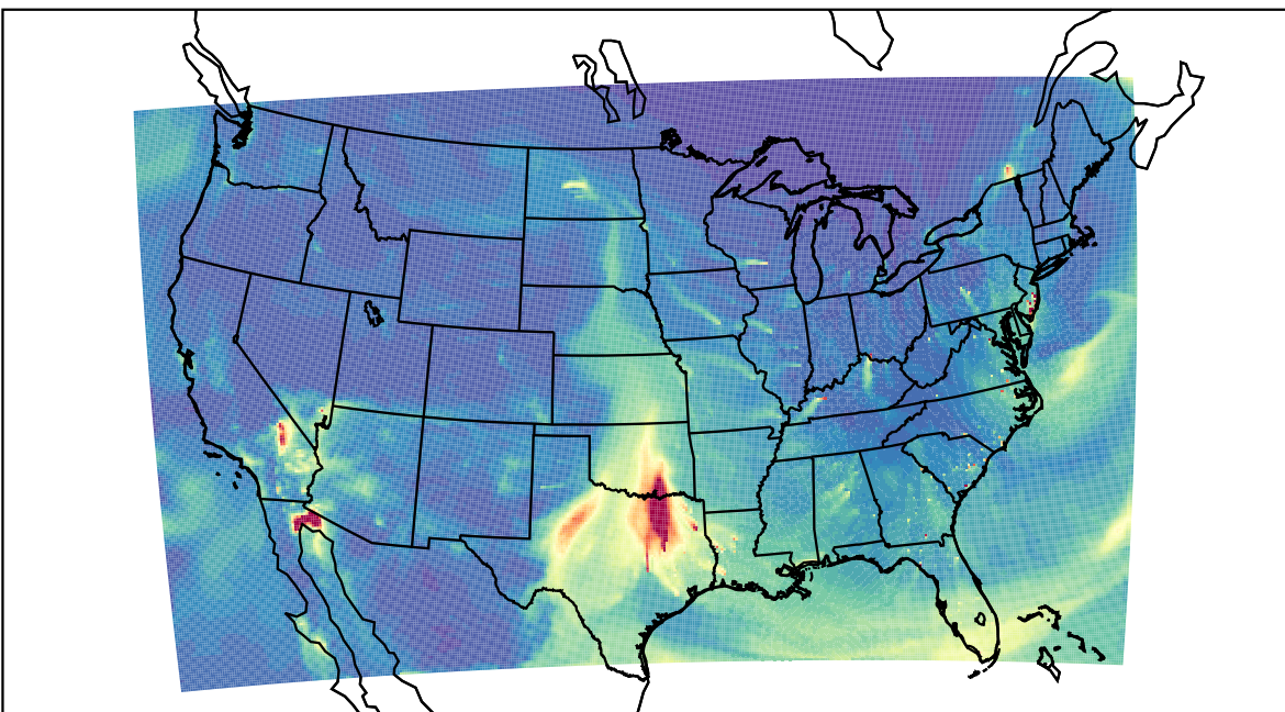
WRF 2023-03-11_17:00:00
