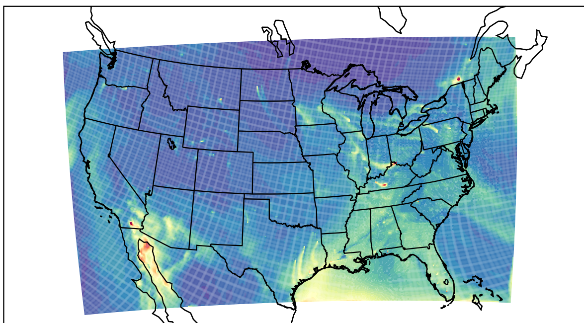
WRF 2023-03-12_19:00:00
