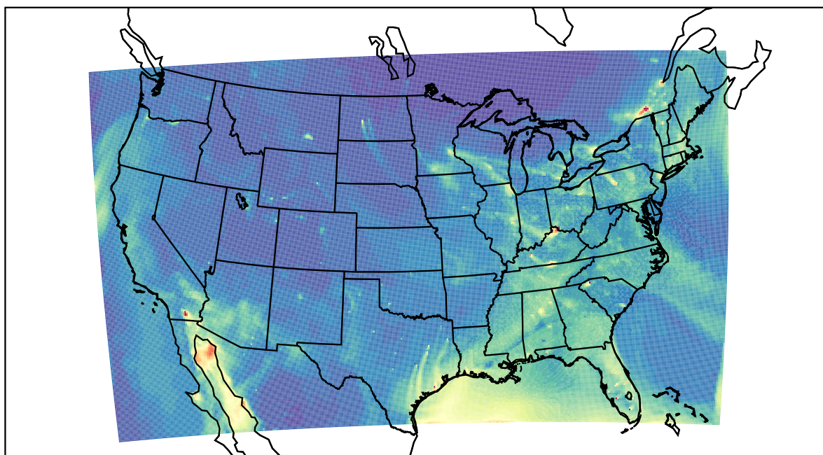
WRF 2023-03-12_22:00:00
