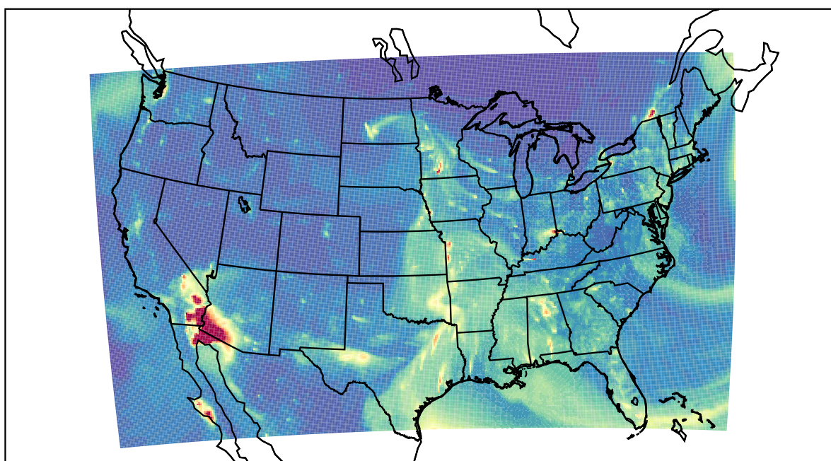
WRF 2023-03-12_03:00:00
