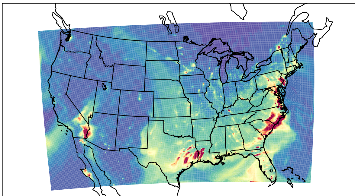
WRF 2023-03-11_01:00:00
