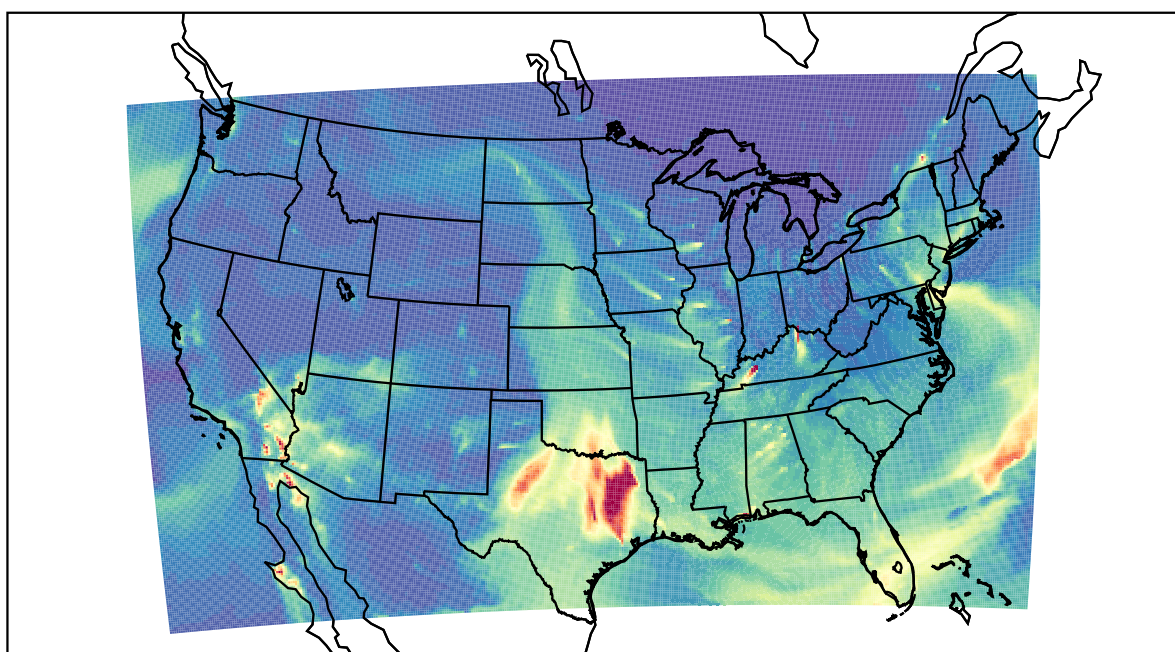
WRF 2023-03-11_13:00:00
