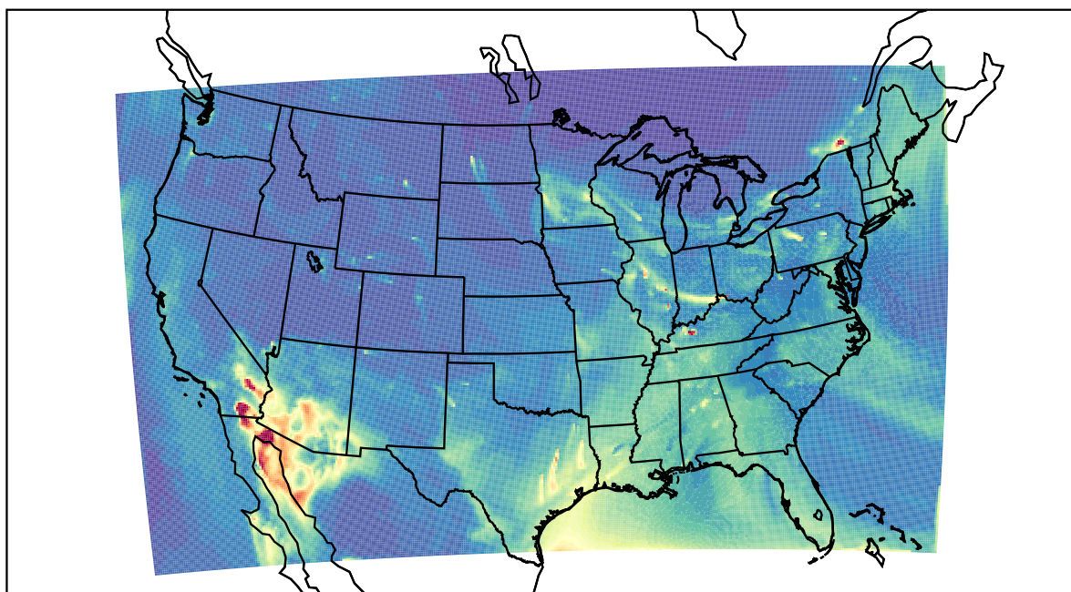
WRF 2023-03-12_16:00:00
