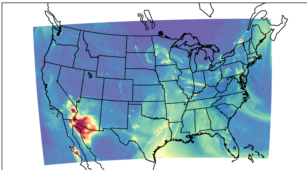
WRF 2023-03-12_11:00:00
