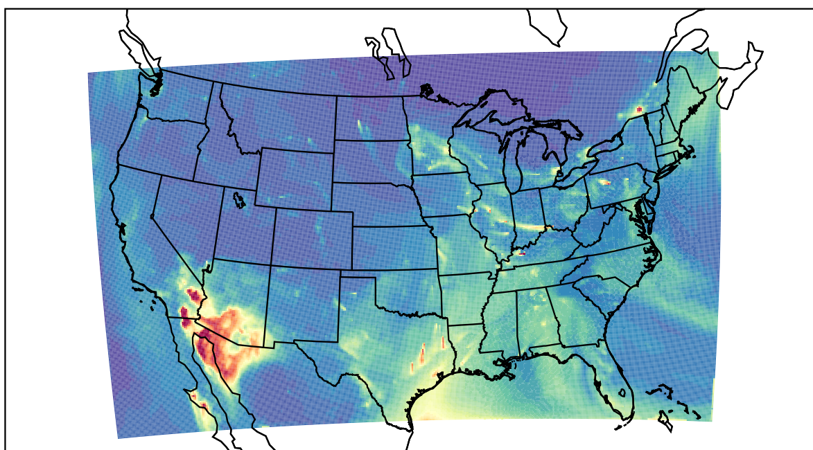
WRF 2023-03-12_14:00:00
