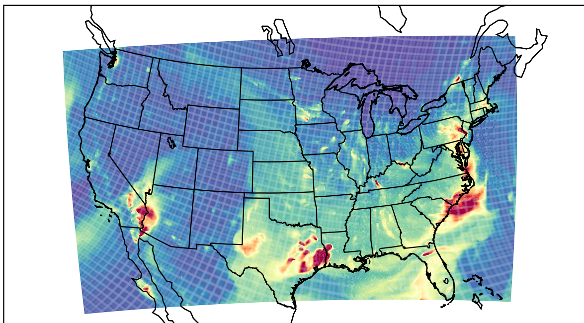
WRF 2023-03-11_04:00:00
