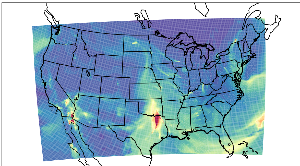
WRF 2023-03-11_17:00:00
