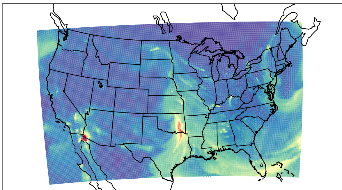
WRF 2023-03-11_20:00:00
