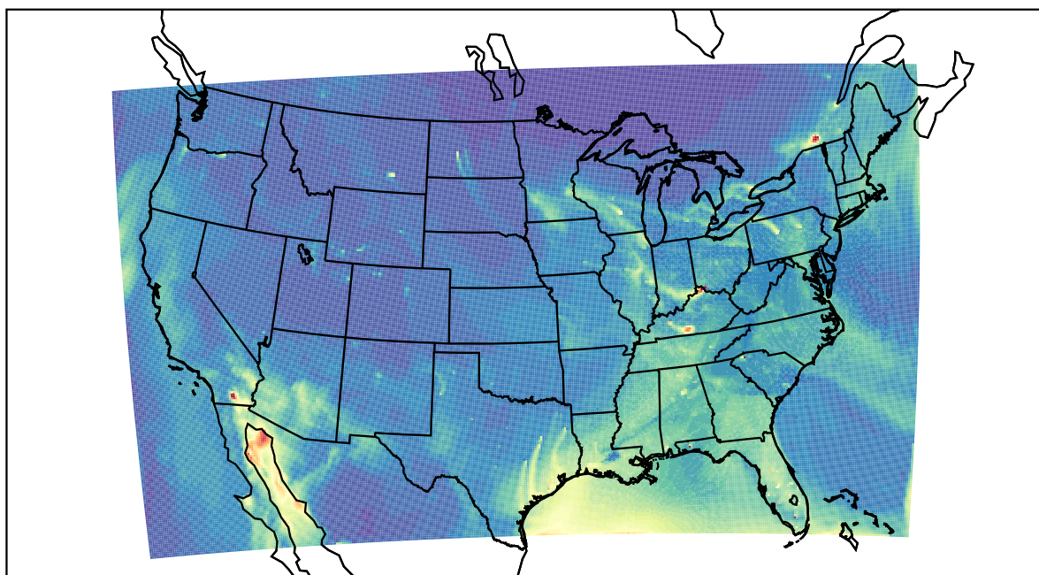
WRF 2023-03-12_20:00:00
