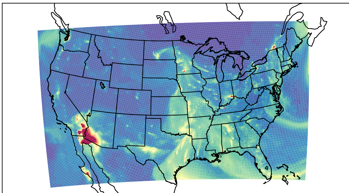
WRF 2023-03-12_04:00:00
