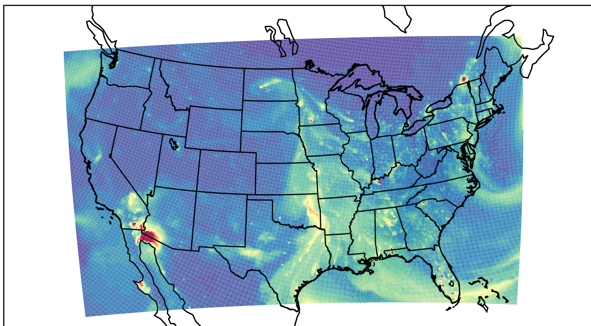
WRF 2023-03-12_00:00:00
