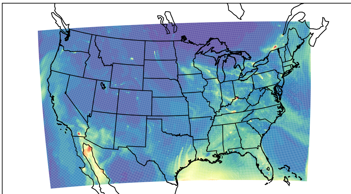
WRF 2023-03-12_21:00:00
