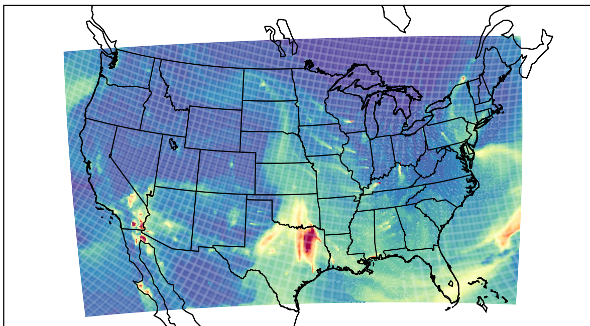
WRF 2023-03-11_15:00:00
