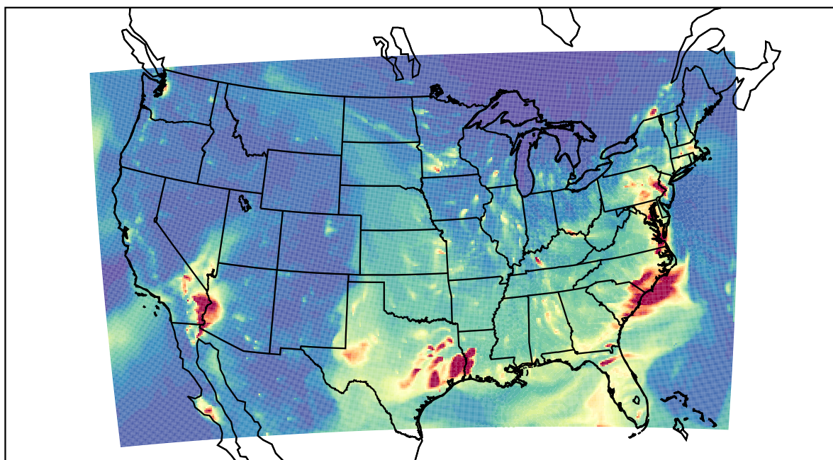
WRF 2023-03-11_03:00:00
