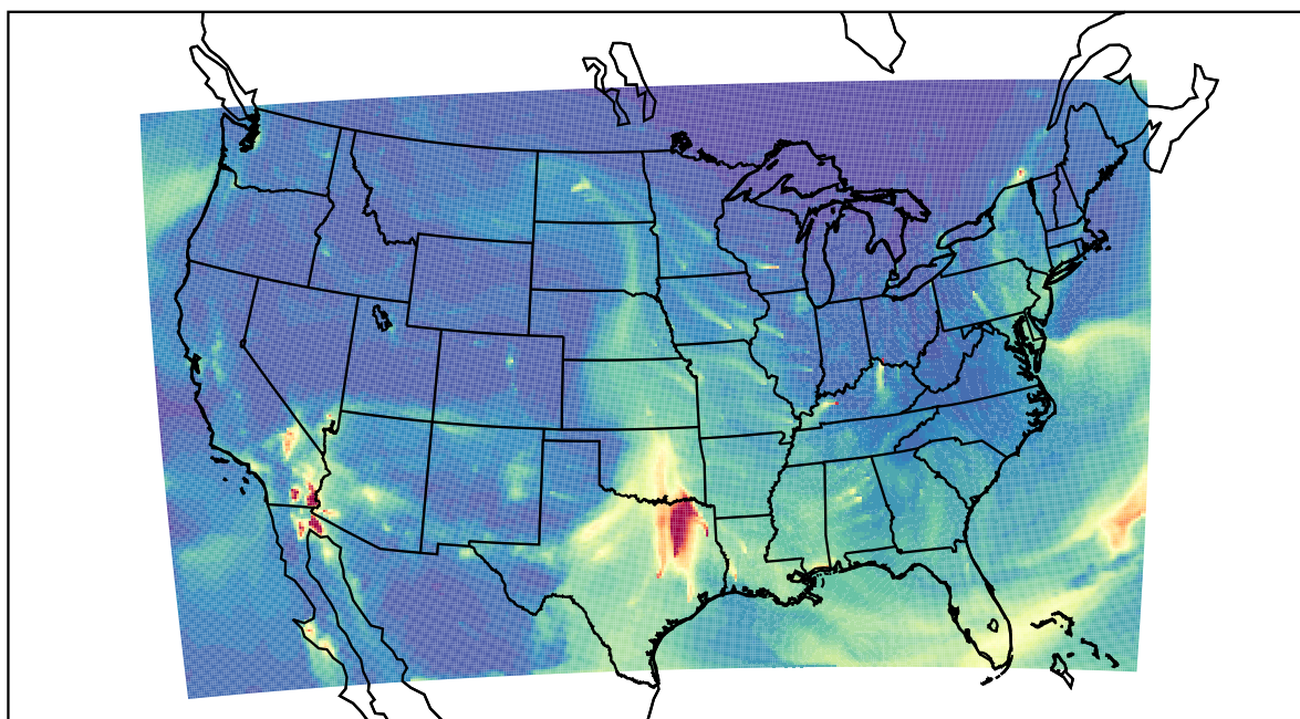
WRF 2023-03-11_16:00:00
