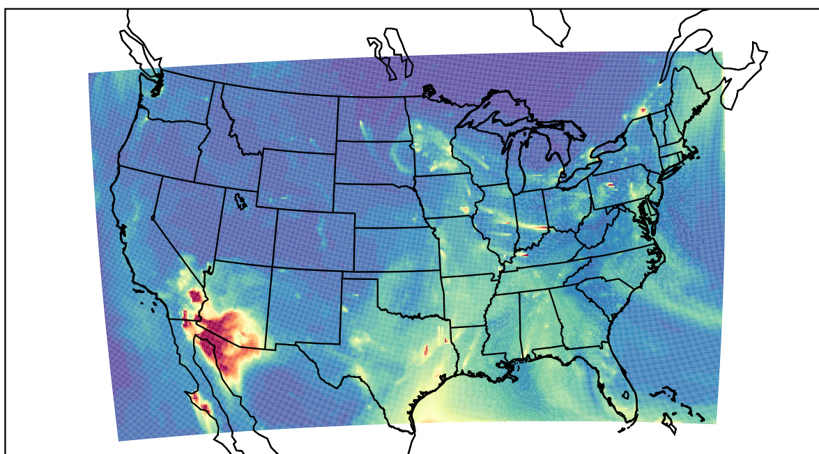
WRF 2023-03-12_12:00:00
