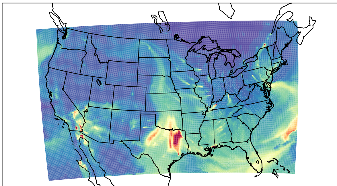
WRF 2023-03-11_14:00:00
