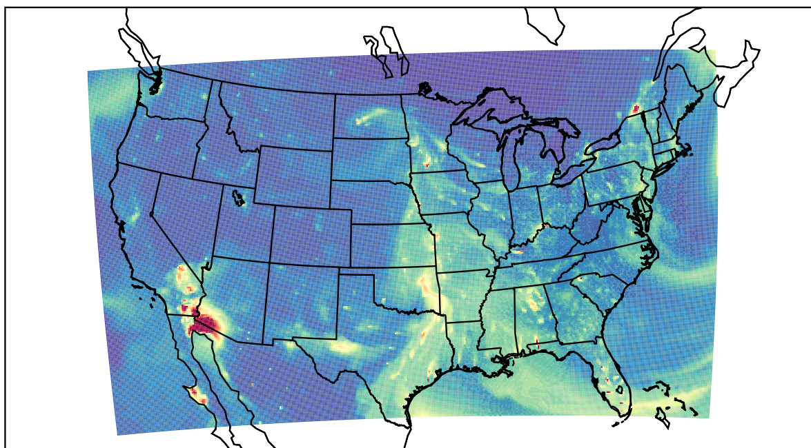
WRF 2023-03-12_01:00:00
