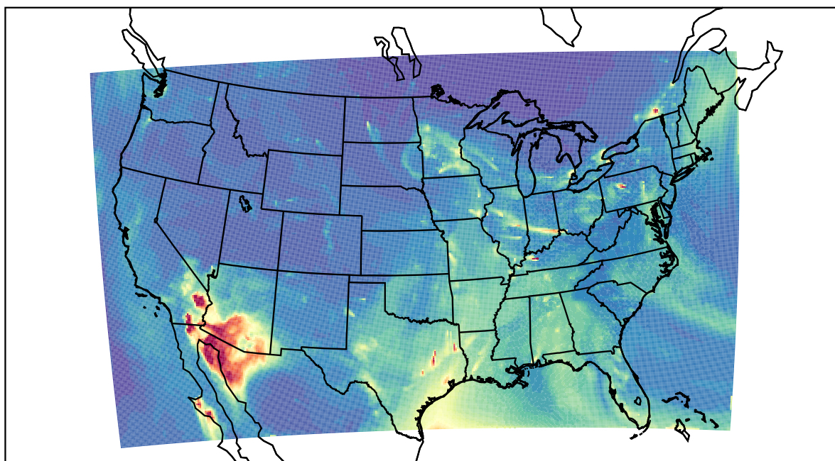
WRF 2023-03-12_13:00:00
