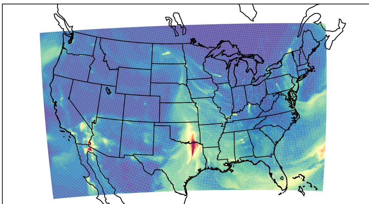
WRF 2023-03-11_18:00:00
