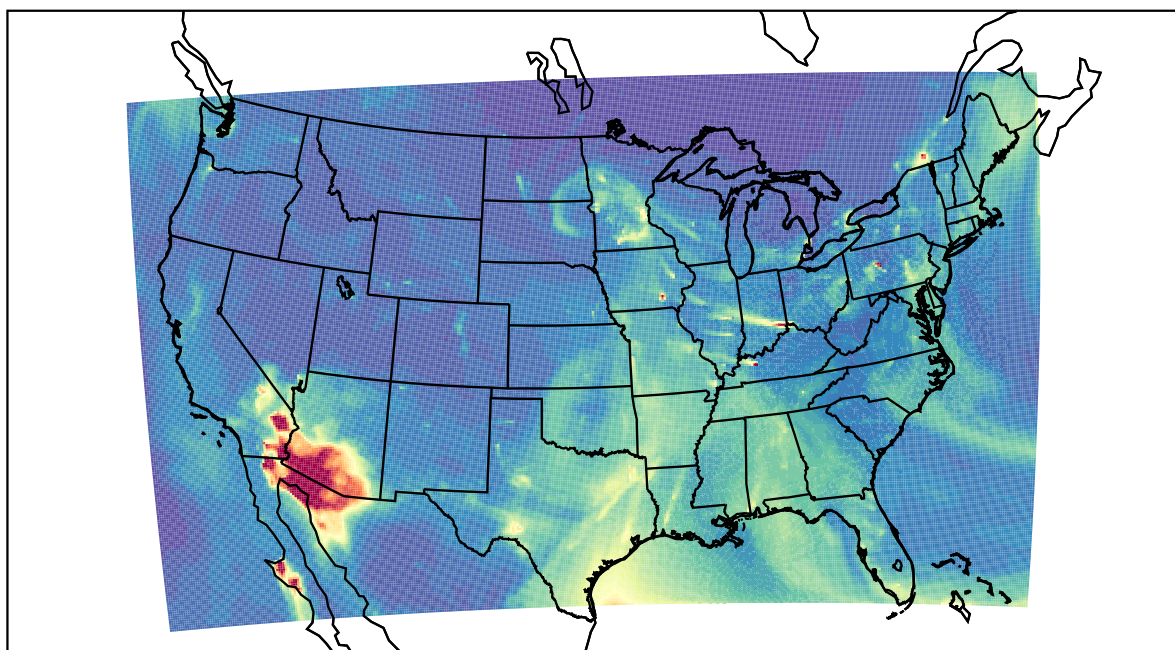
WRF 2023-03-12_10:00:00
