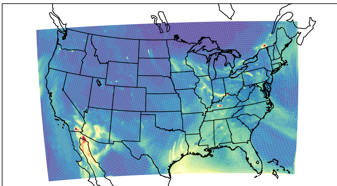
WRF 2023-03-12_18:00:00
