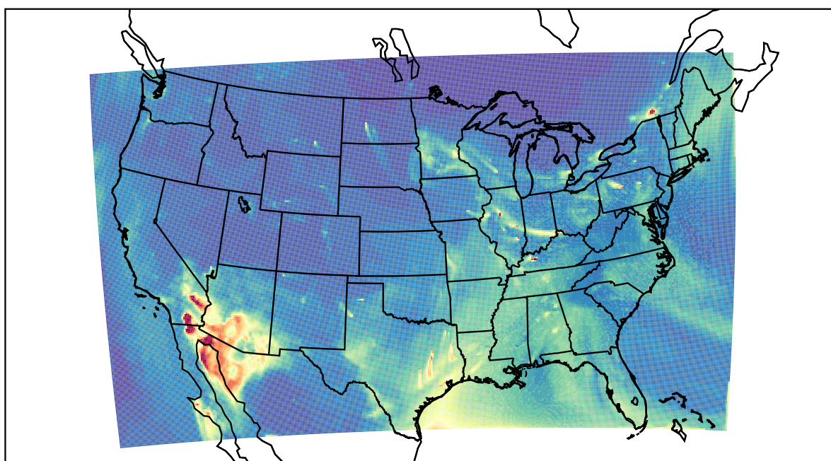
WRF 2023-03-12_15:00:00
