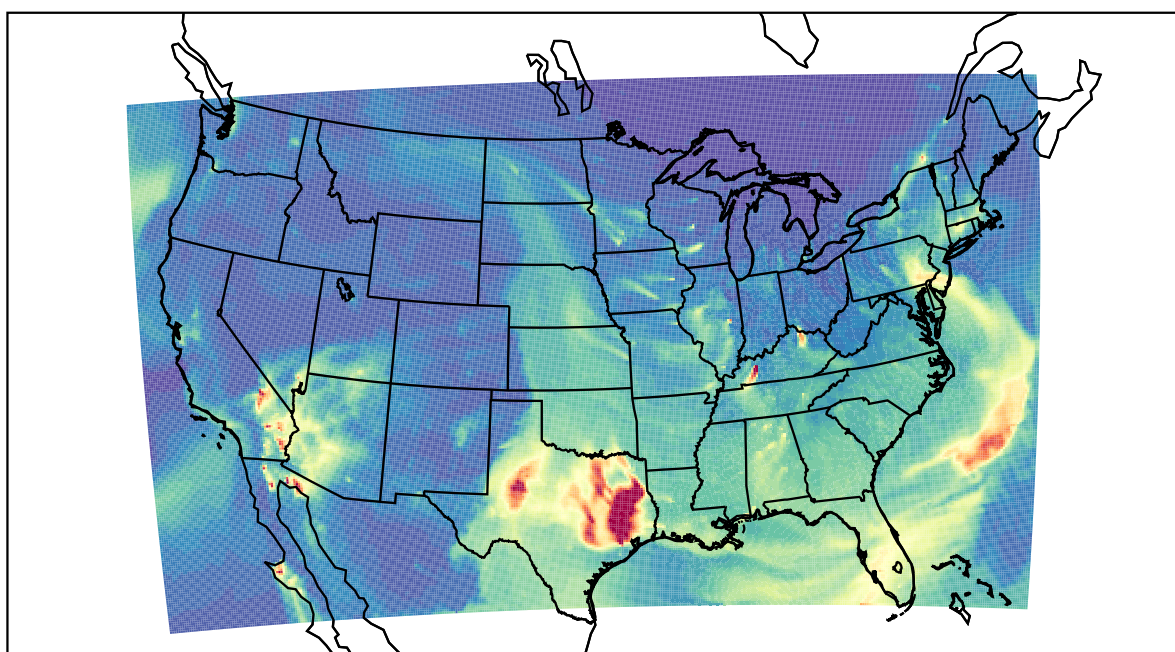
WRF 2023-03-11_10:00:00
