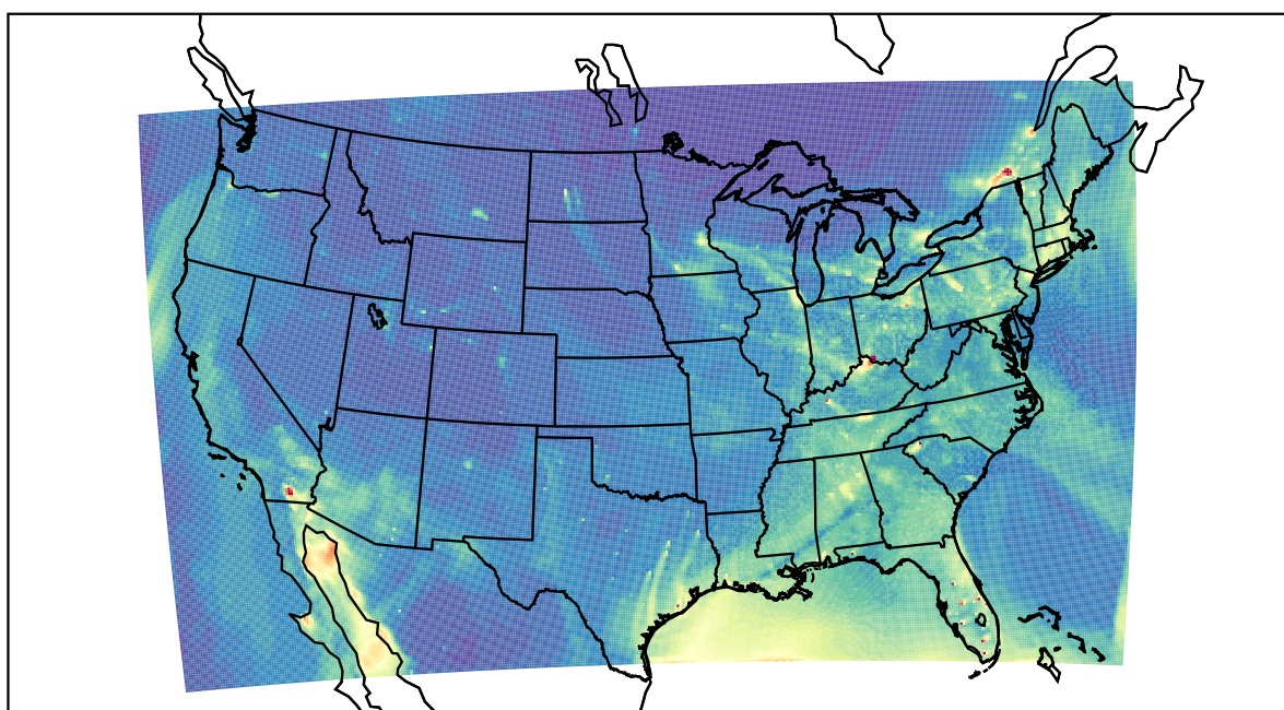
WRF 2023-03-12_23:00:00
