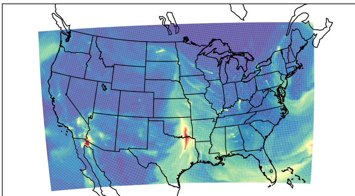
WRF 2023-03-11_19:00:00
