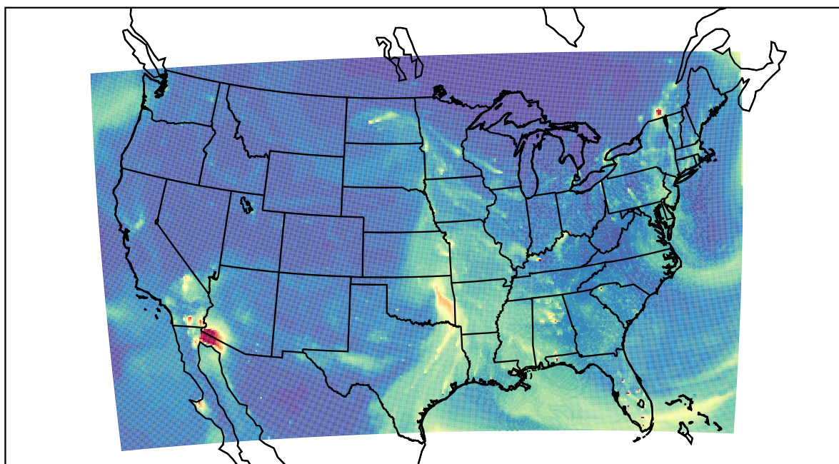
WRF 2023-03-11_23:00:00
