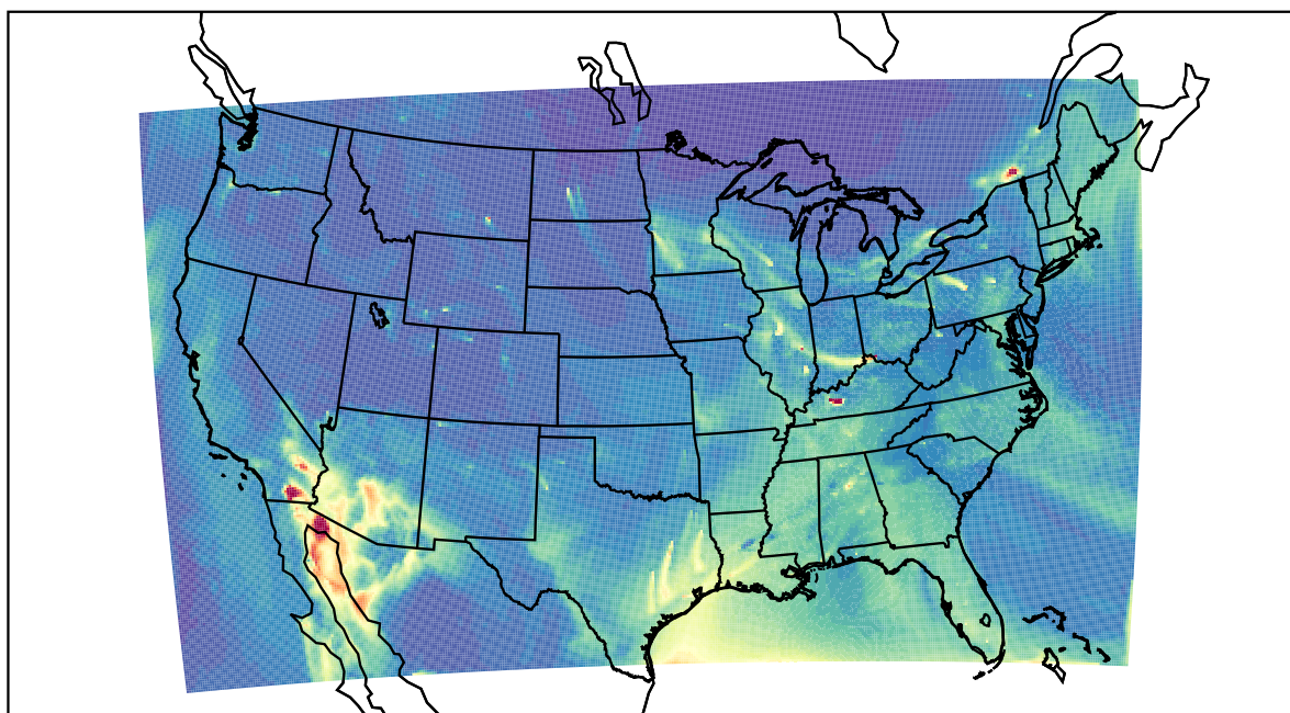
WRF 2023-03-12_17:00:00
