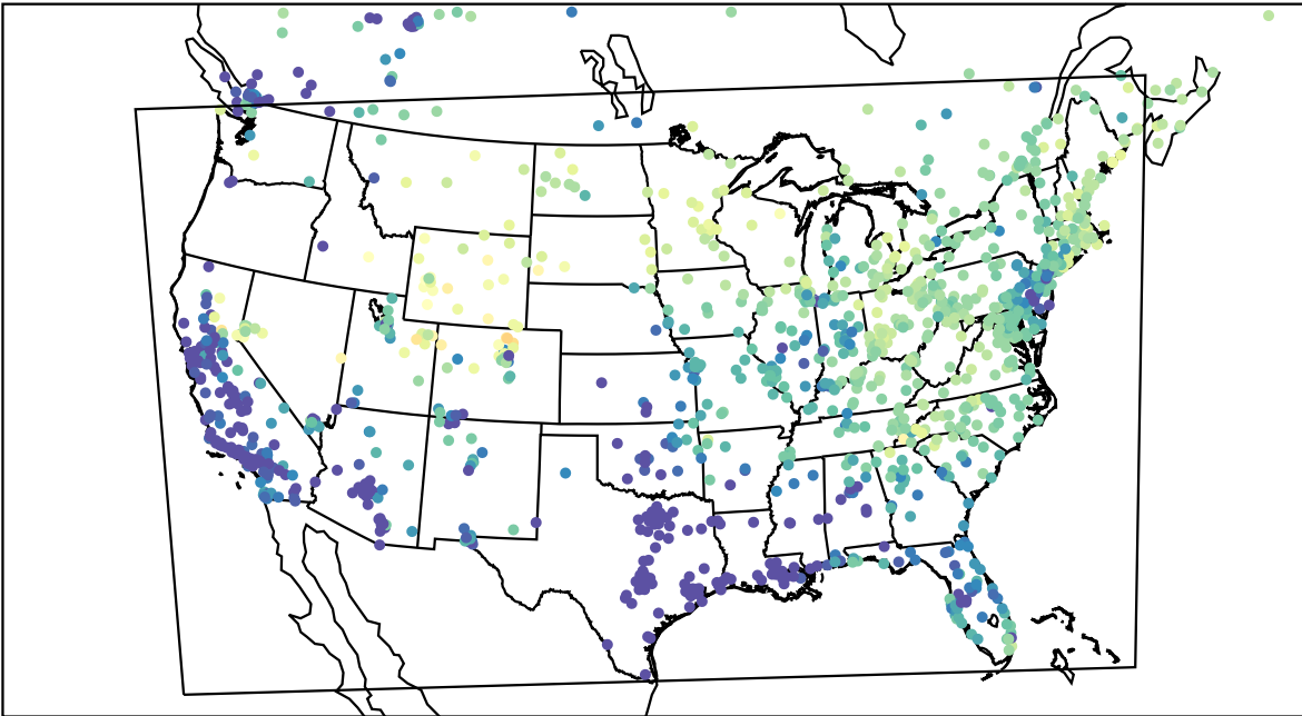
AirNOW (2023-03-11_13:00:00)
