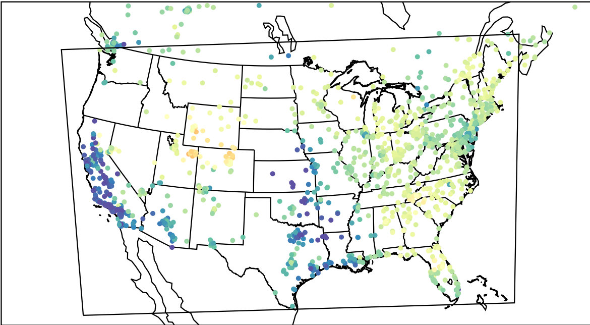
AirNOW (2023-03-11_18:00:00)
