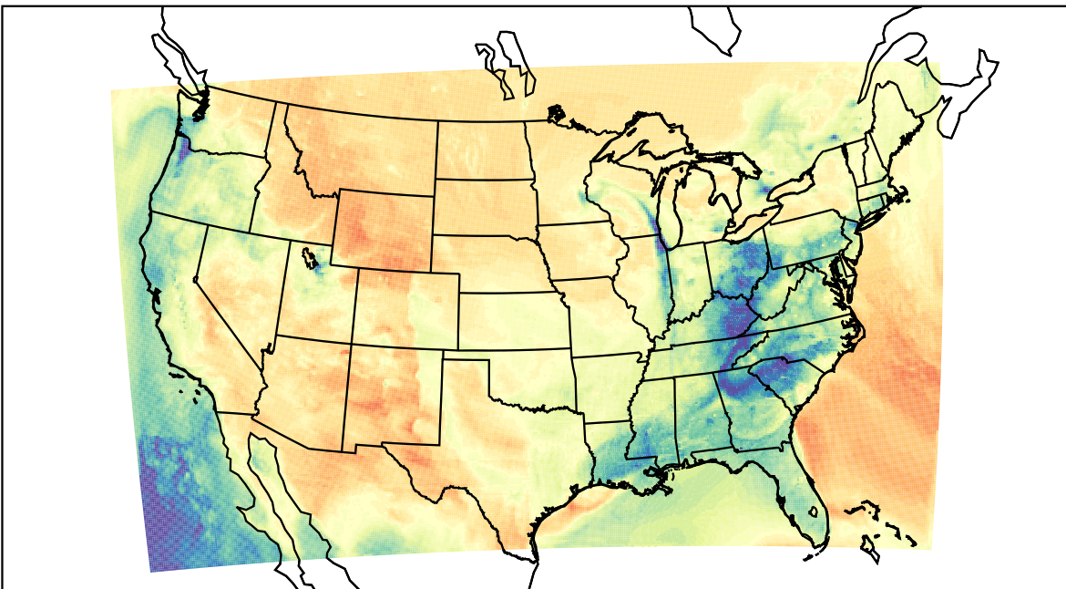
WRF (2023-03-12_23:00:00)
