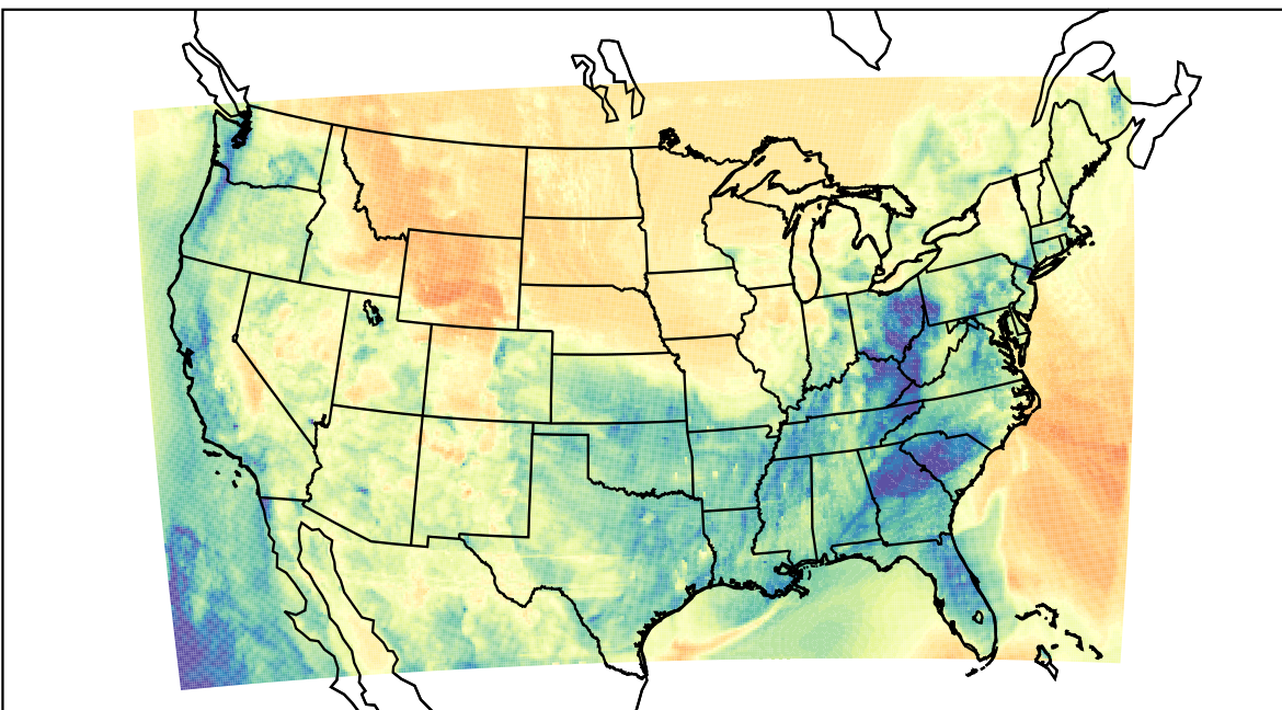
WRF (2023-03-13_04:00:00)
