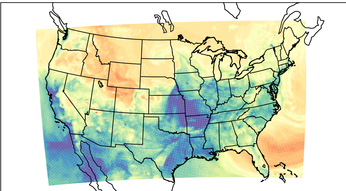
WRF (2023-03-12_04:00:00)
