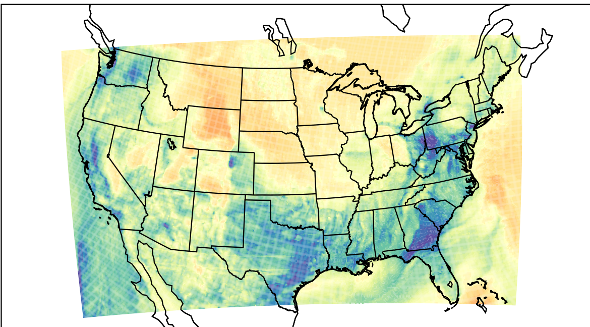
WRF (2023-03-13_13:00:00)
