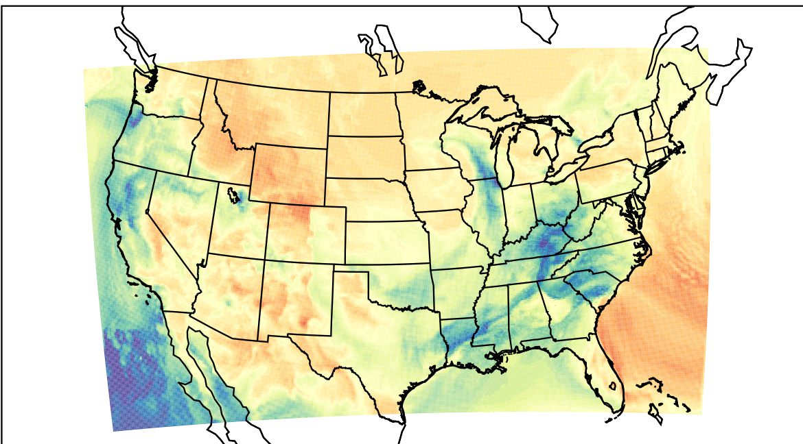
WRF (2023-03-12_19:00:00)
