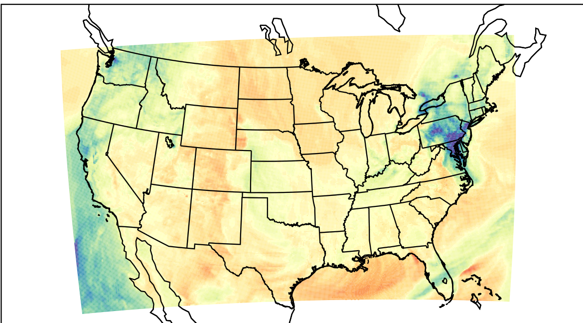
WRF (2023-03-13_22:00:00)
