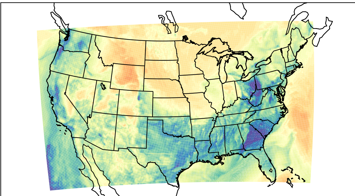
WRF (2023-03-13_10:00:00)
