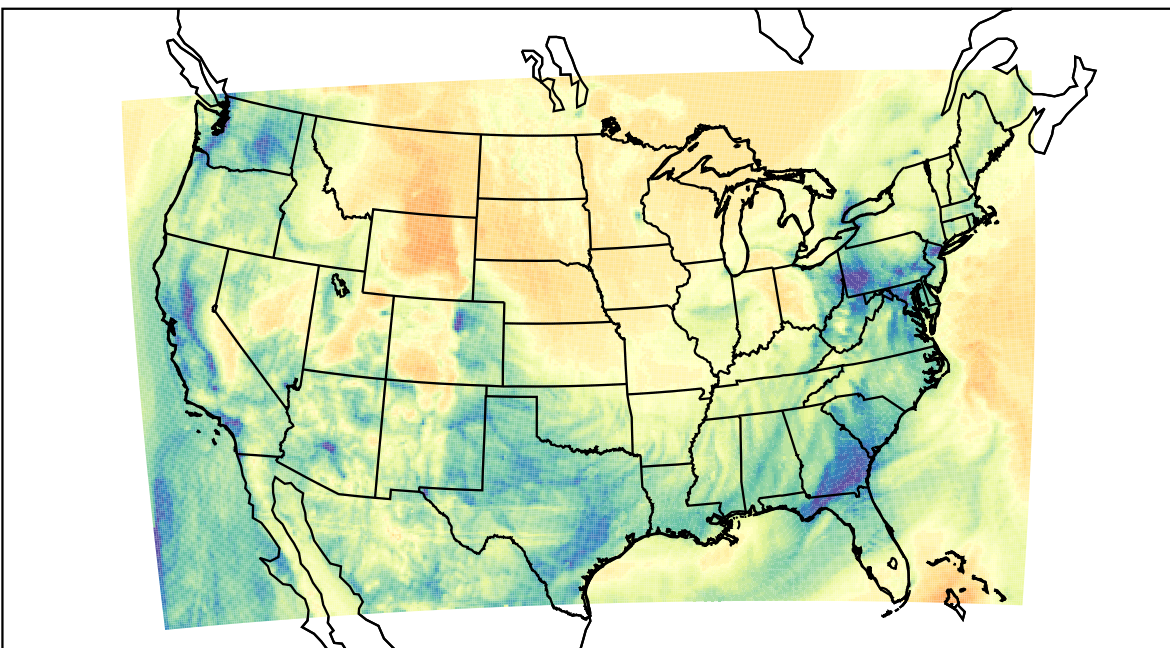
WRF (2023-03-13_14:00:00)
