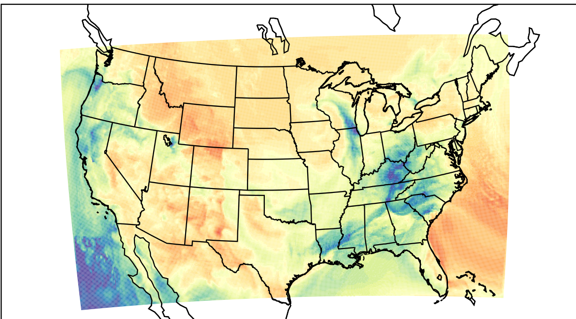
WRF (2023-03-12_20:00:00)
