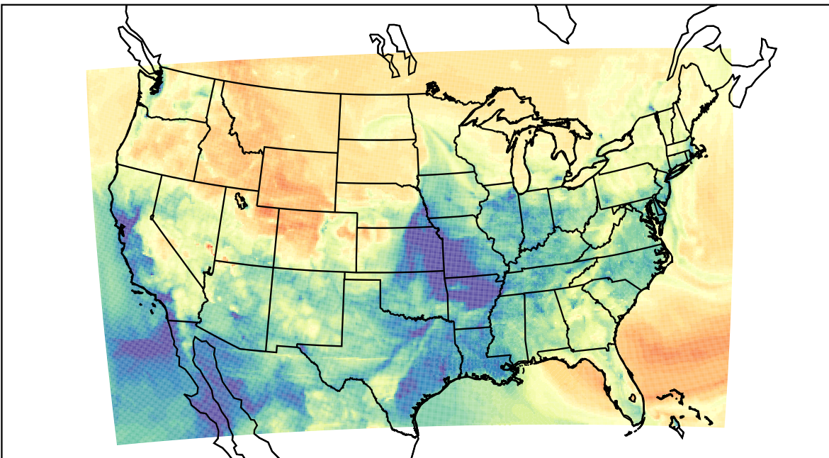
WRF (2023-03-12_03:00:00)
