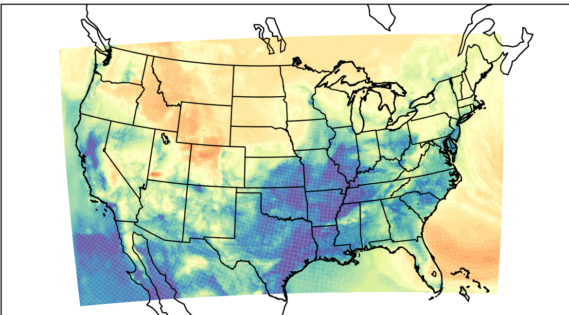
WRF (2023-03-12_11:00:00)
