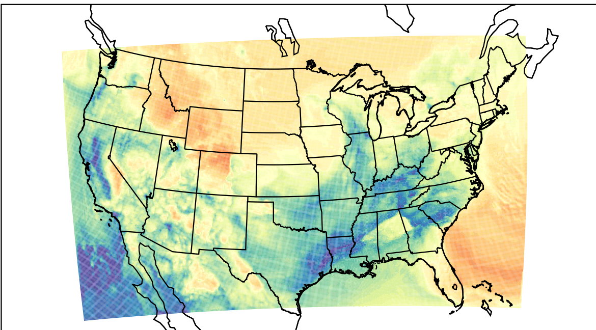
WRF (2023-03-12_16:00:00)
