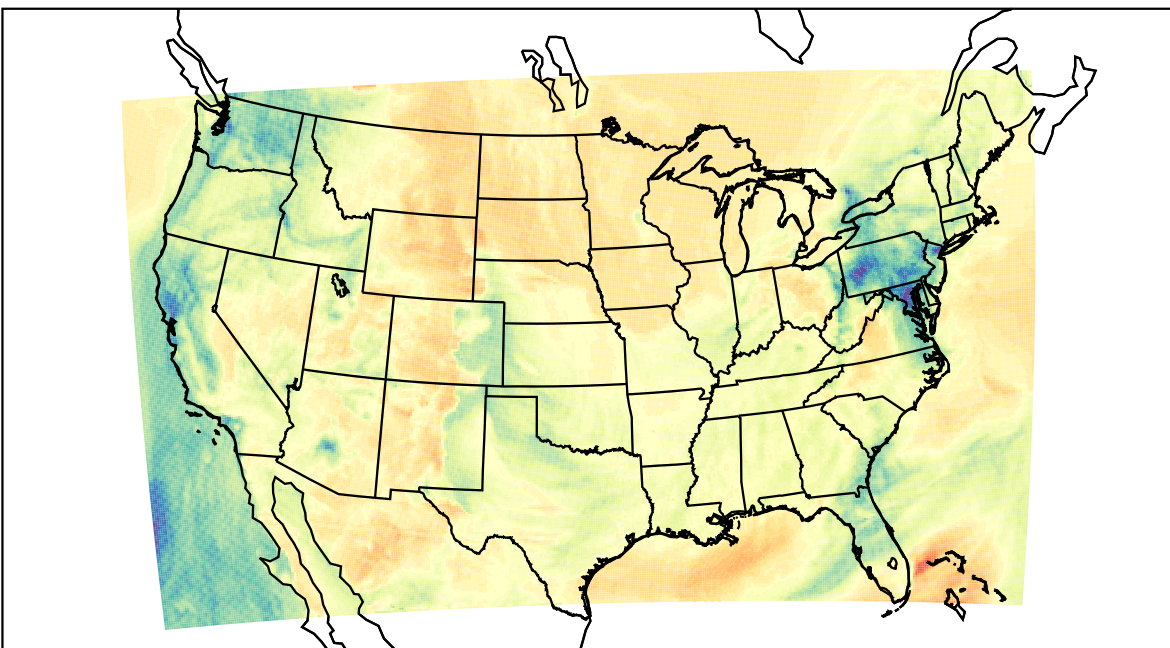
WRF (2023-03-13_18:00:00)
