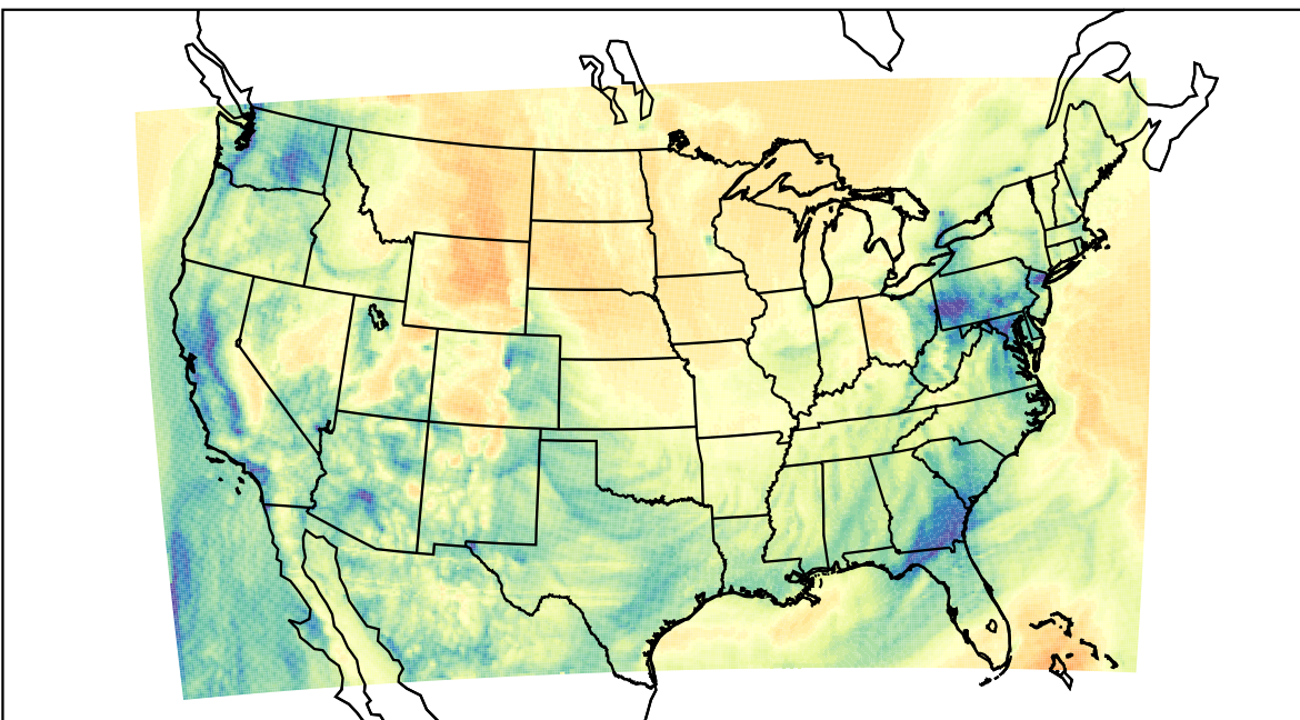
WRF (2023-03-13_15:00:00)
