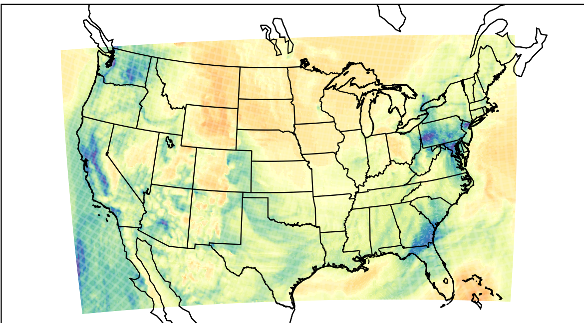
WRF (2023-03-13_16:00:00)
