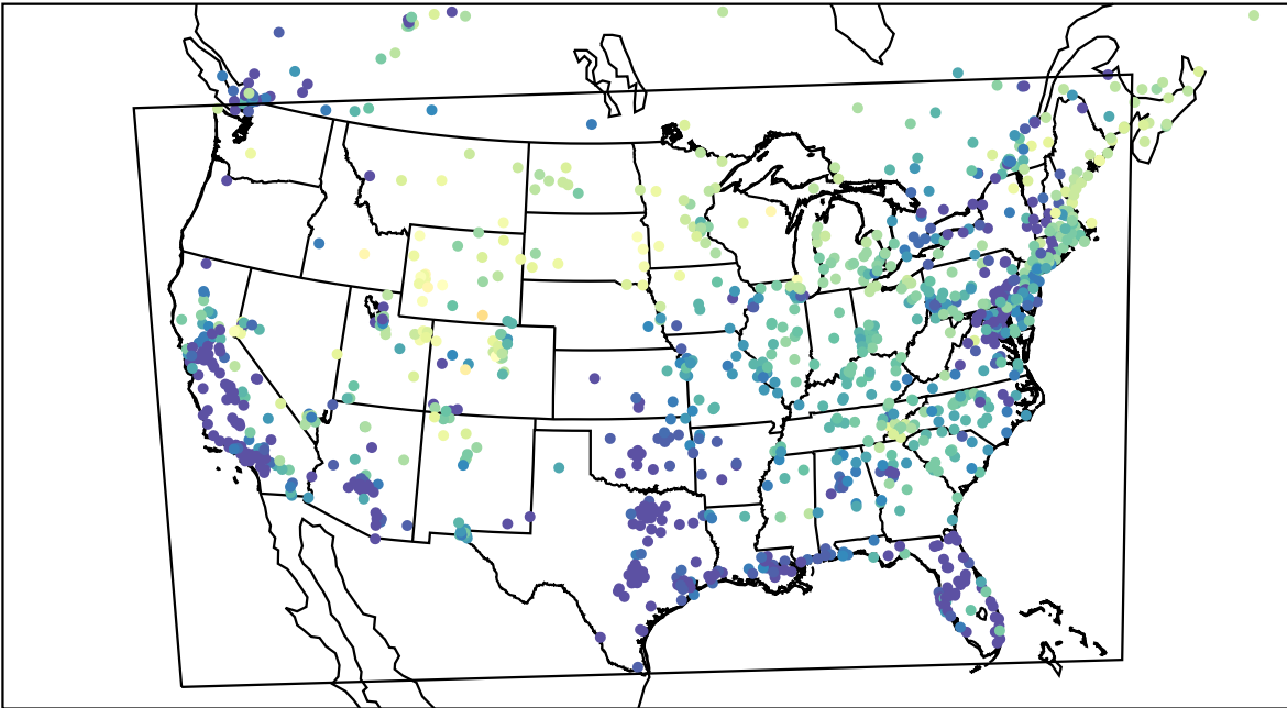
AirNOW (2023-03-12_10:00:00)
