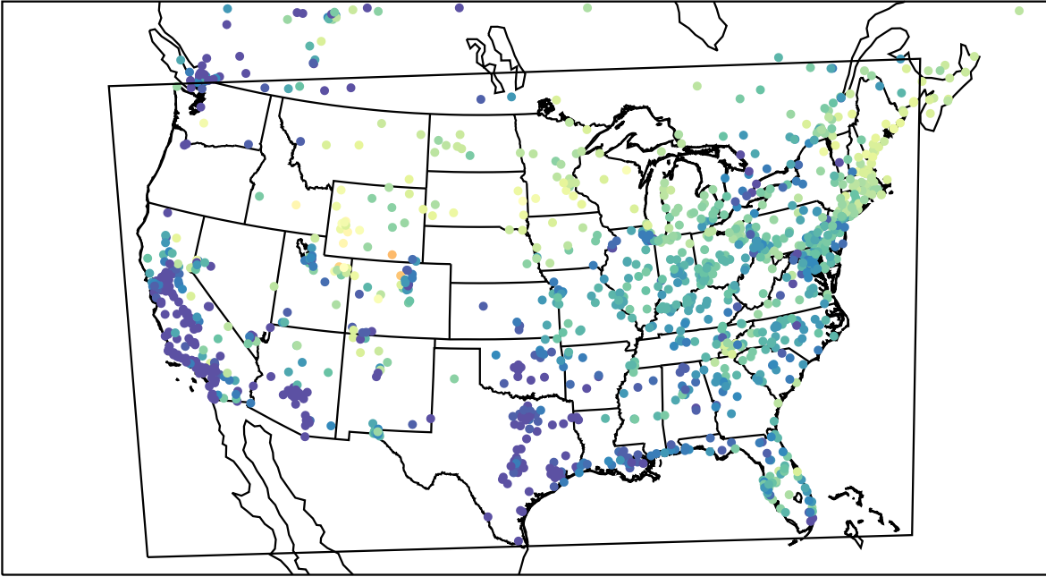
AirNOW (2023-03-12_13:00:00)
