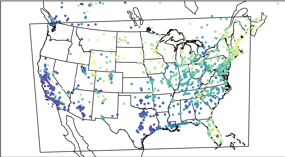
AirNOW (2023-03-12_14:00:00)
