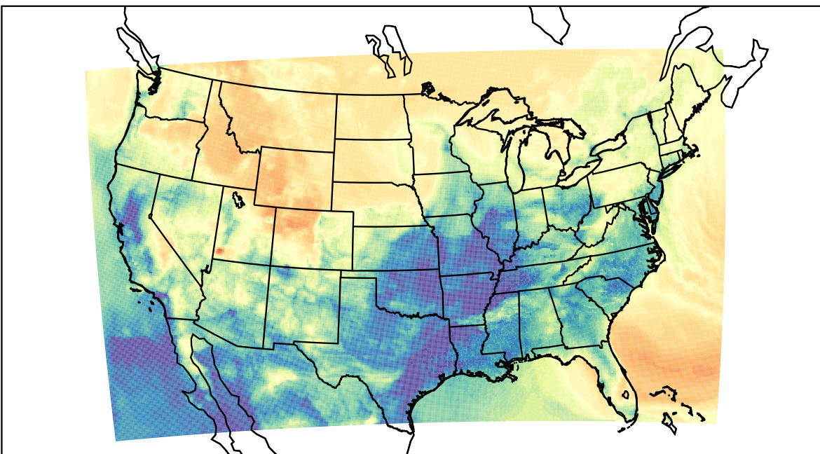
WRF (2023-03-12_10:00:00)
