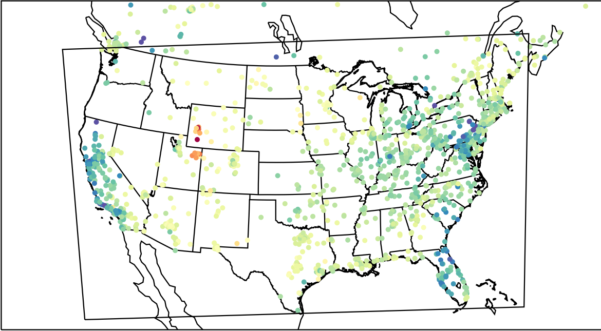
AirNOW (2023-03-13_20:00:00)
