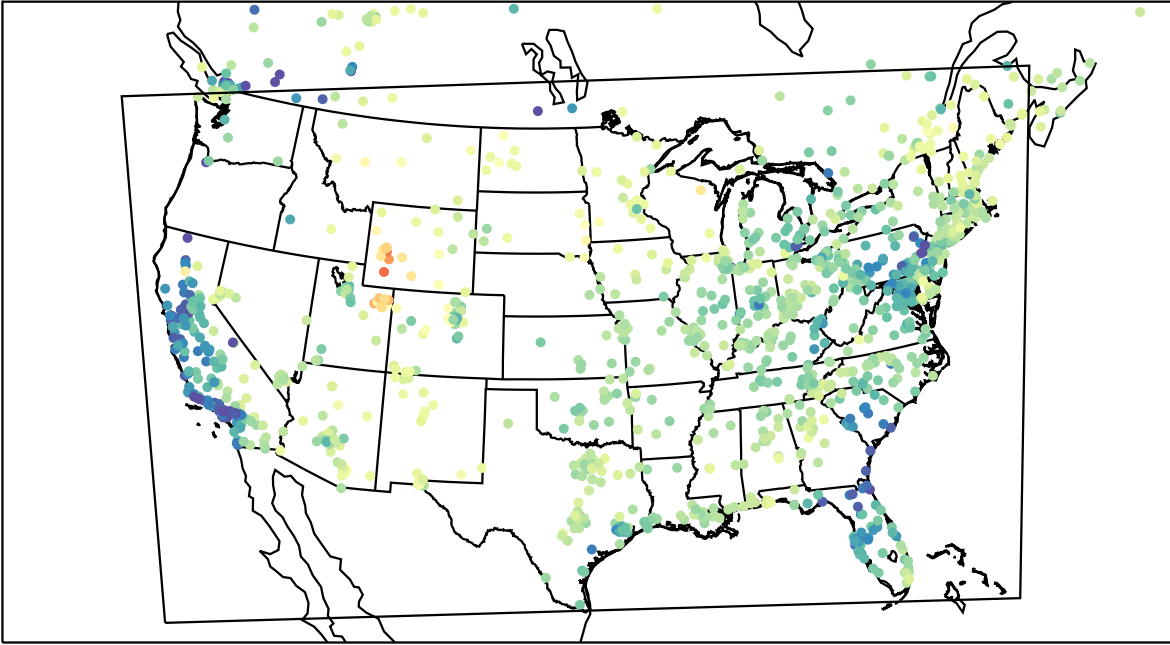
AirNOW (2023-03-13_18:00:00)
