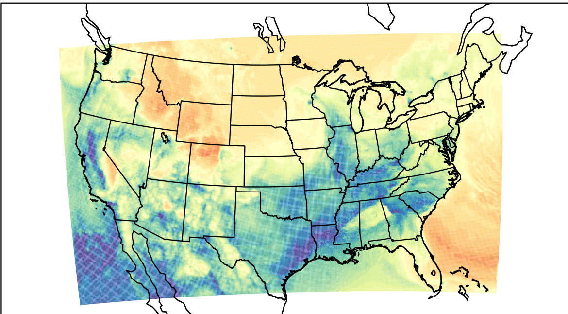
WRF (2023-03-12_15:00:00)
