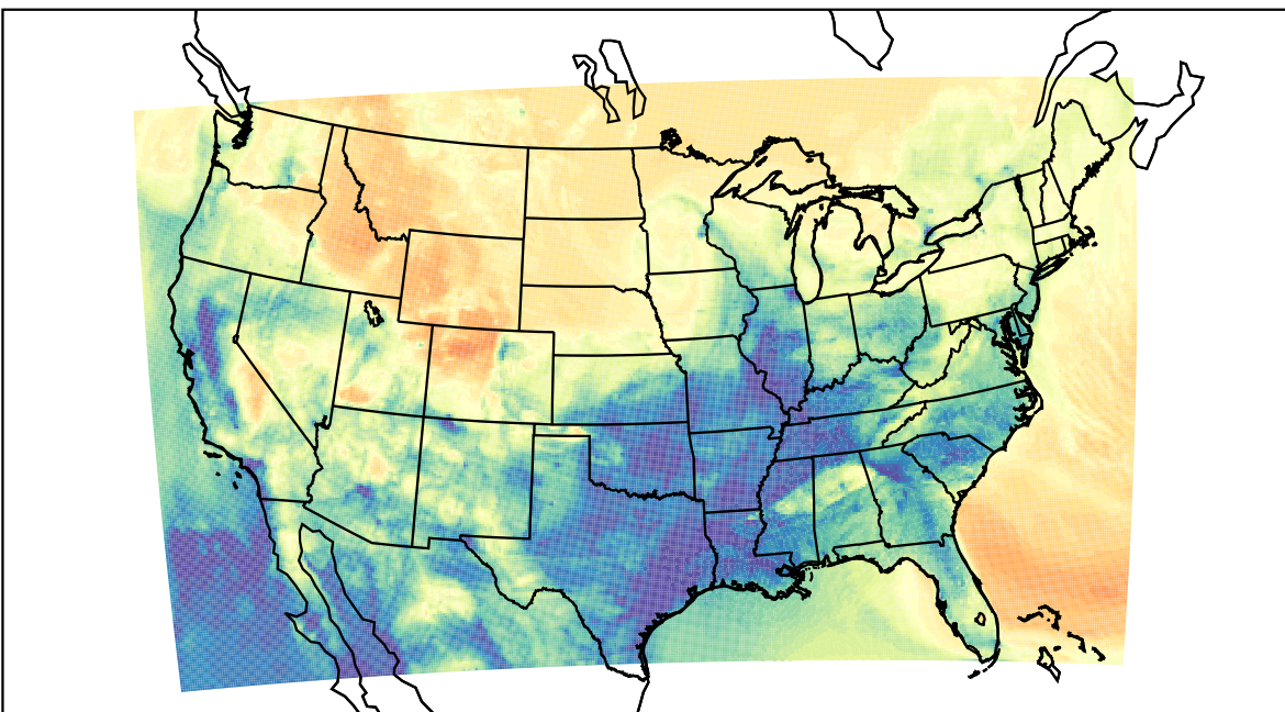
WRF (2023-03-12_13:00:00)
