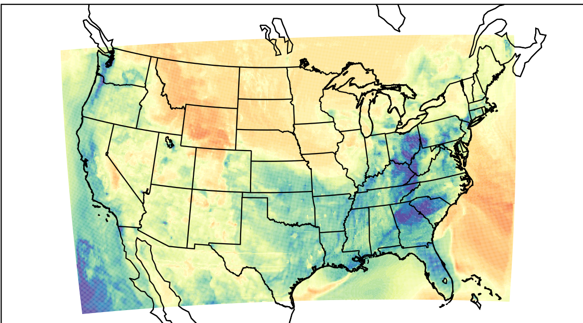
WRF (2023-03-13_03:00:00)
