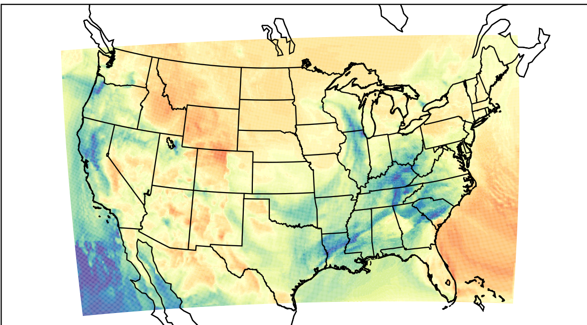
WRF (2023-03-12_18:00:00)
