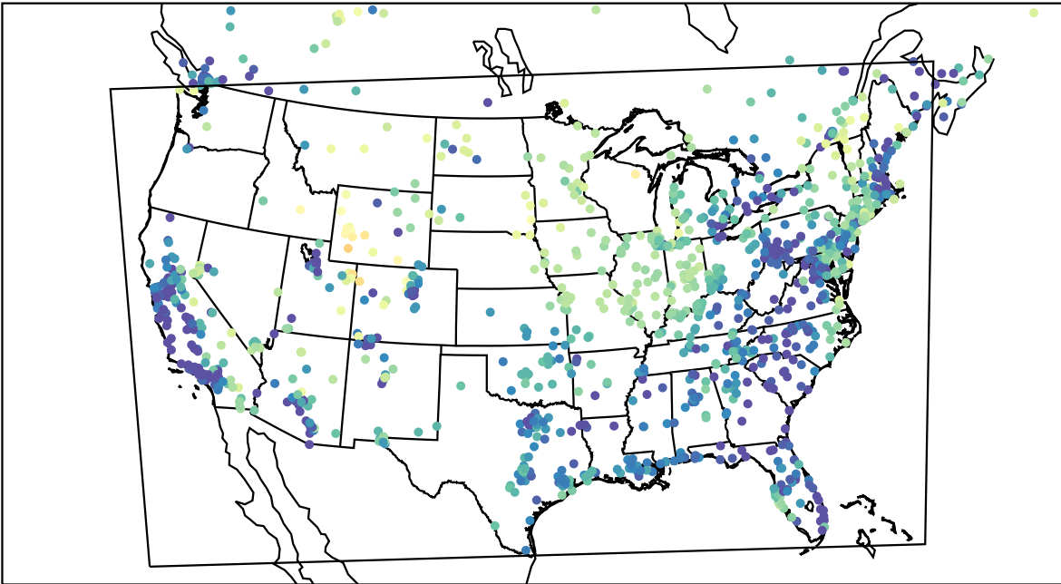
AirNOW (2023-03-13_10:00:00)
