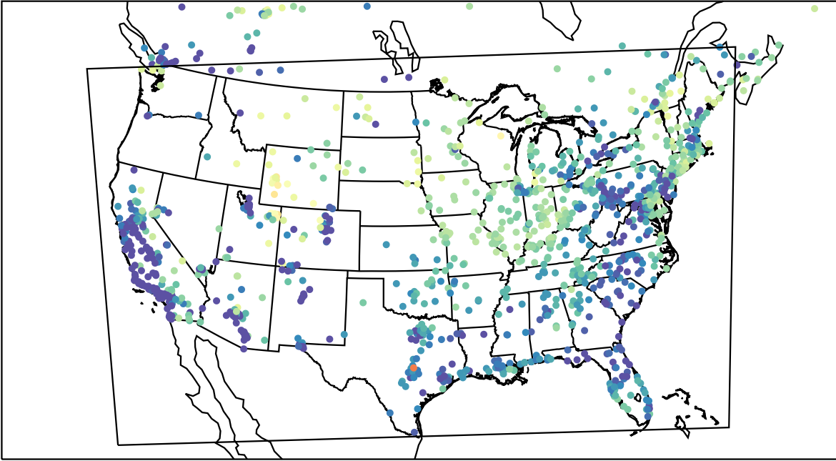
AirNOW (2023-03-13_13:00:00)
