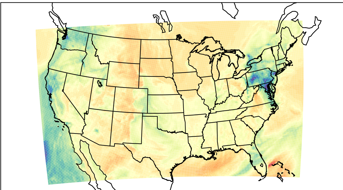
WRF (2023-03-13_19:00:00)
