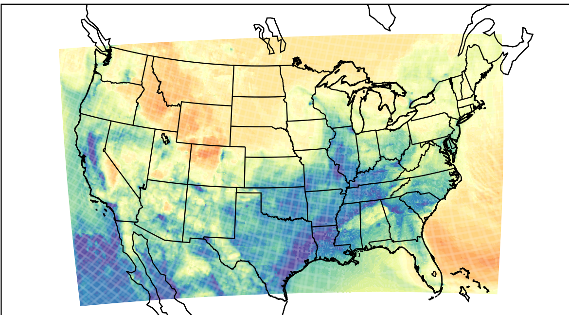
WRF (2023-03-12_14:00:00)
