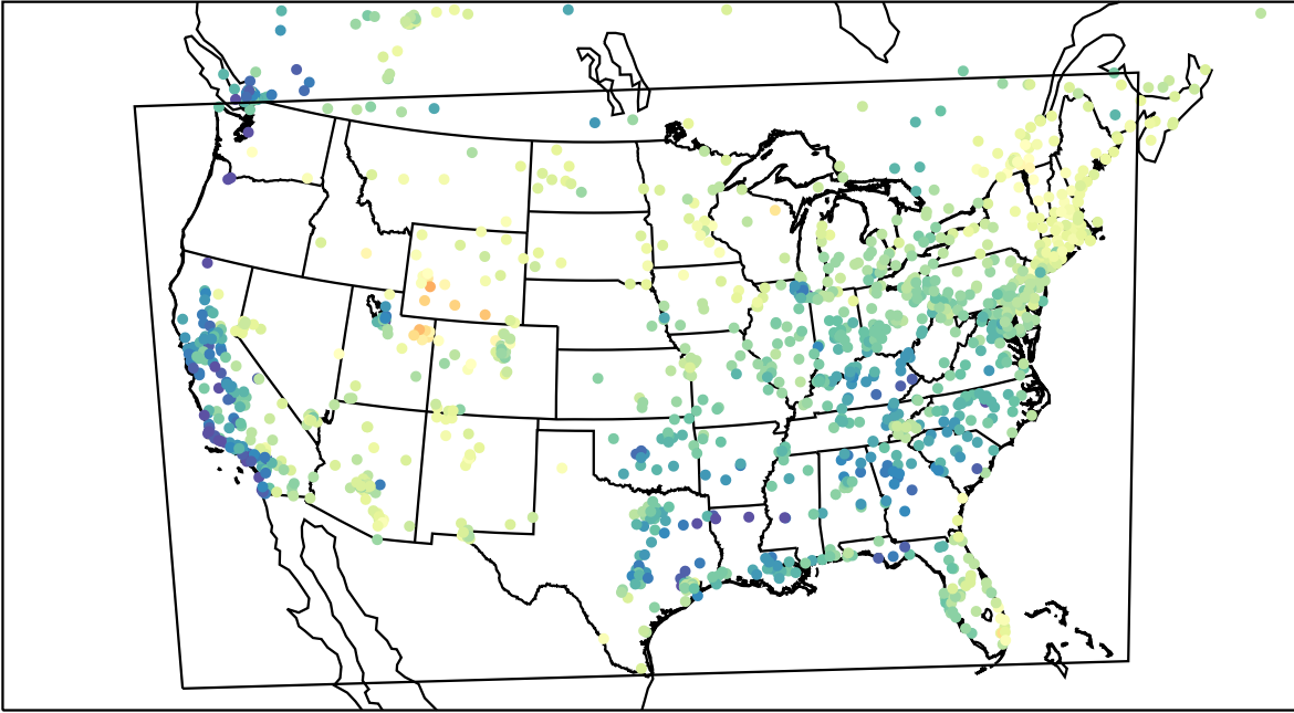
AirNOW (2023-03-12_18:00:00)
