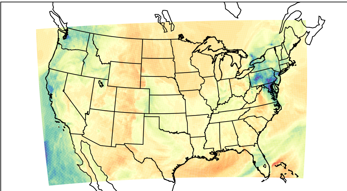
WRF (2023-03-13_20:00:00)
