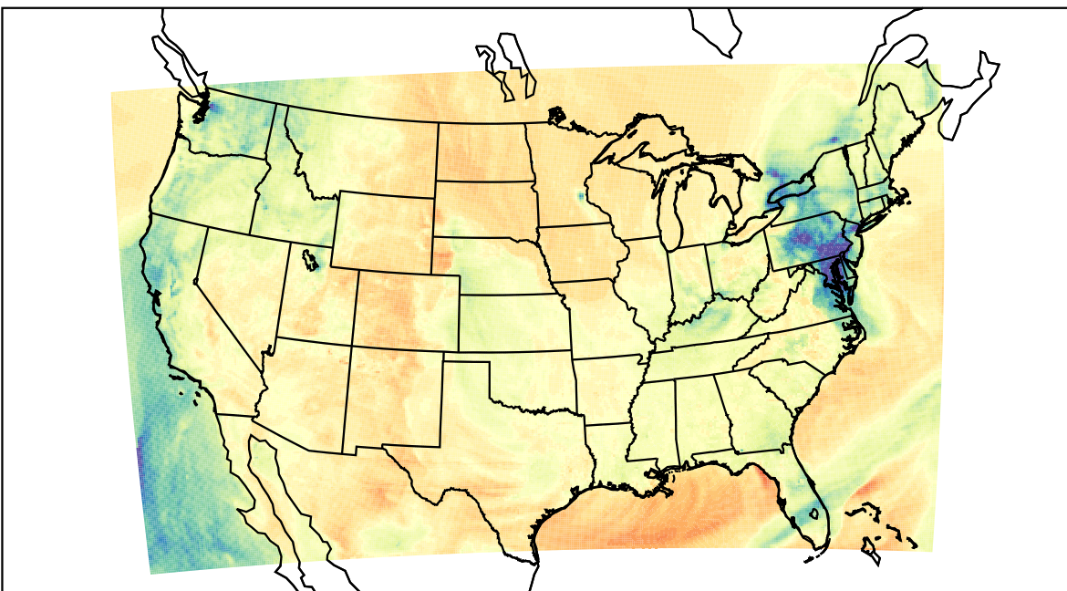
WRF (2023-03-13_23:00:00)
