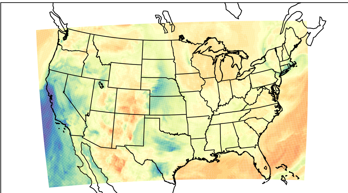
WRF (2023-03-14_18:00:00)
