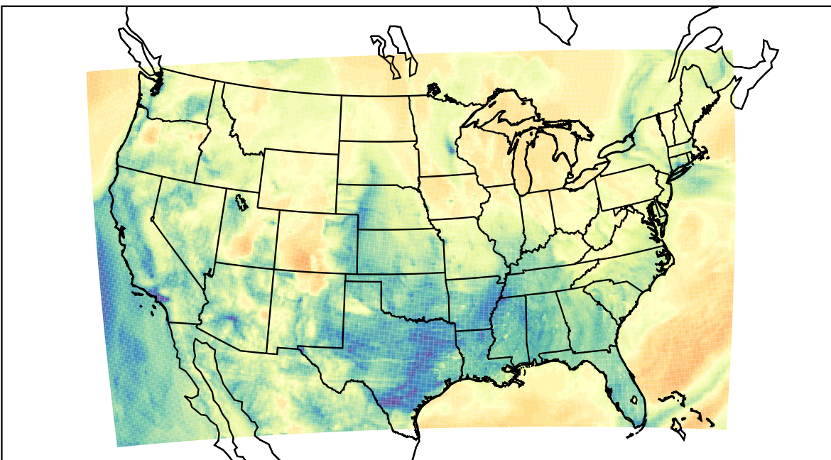
WRF (2023-03-14_13:00:00)
