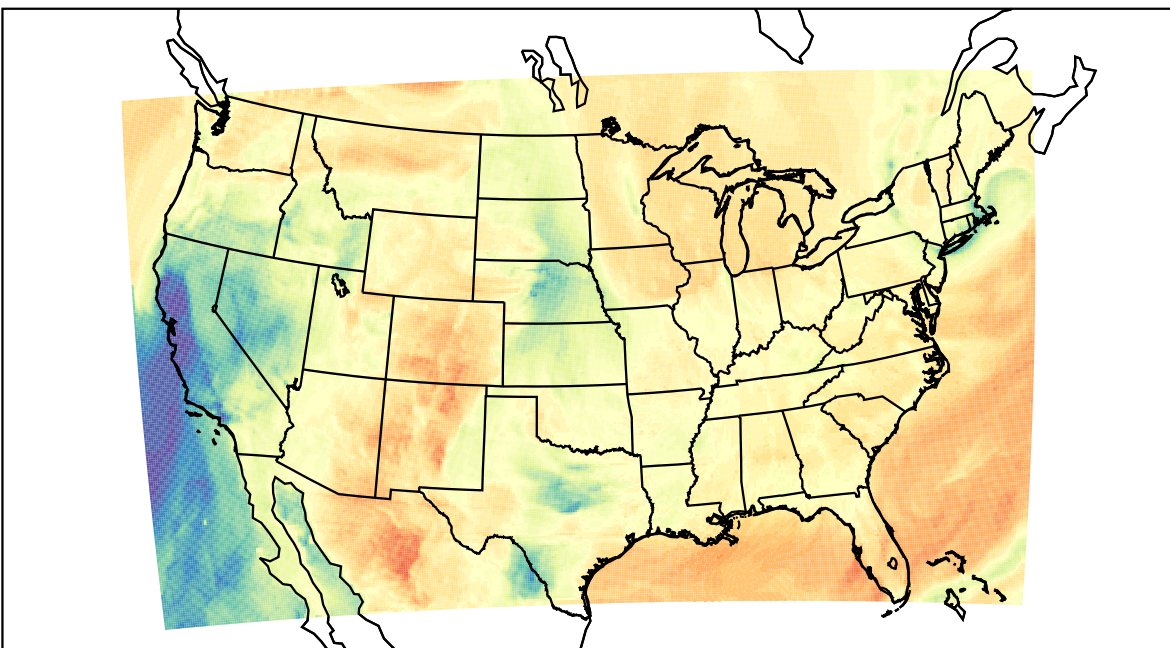
WRF (2023-03-14_20:00:00)
