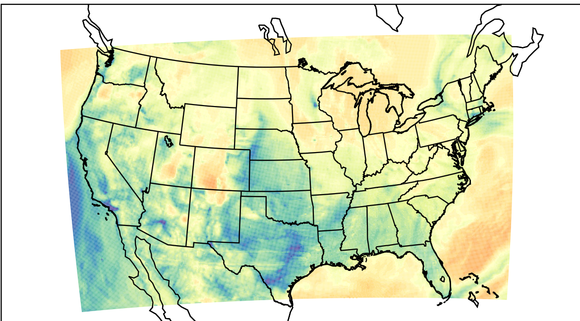
WRF (2023-03-14_14:00:00)
