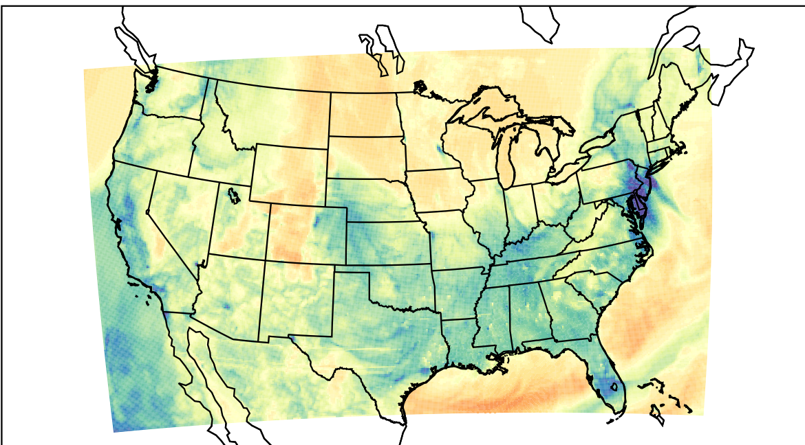
WRF (2023-03-14_04:00:00)
