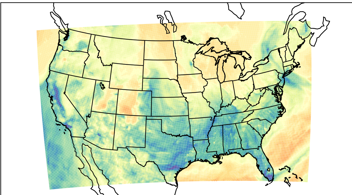
WRF (2023-03-14_10:00:00)
