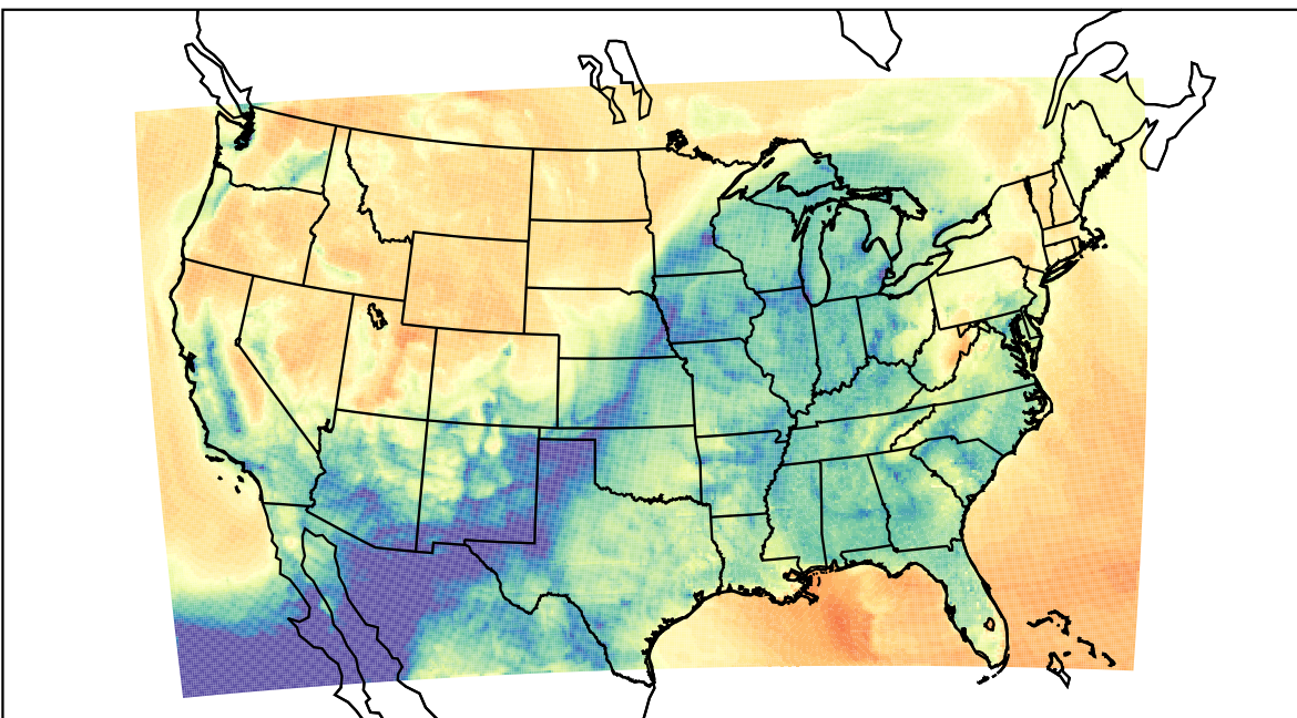
WRF (2023-03-16_13:00:00)
