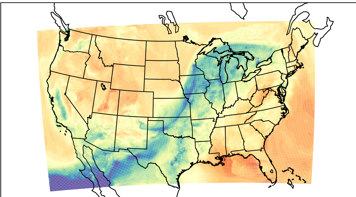
WRF (2023-03-16_18:00:00)
