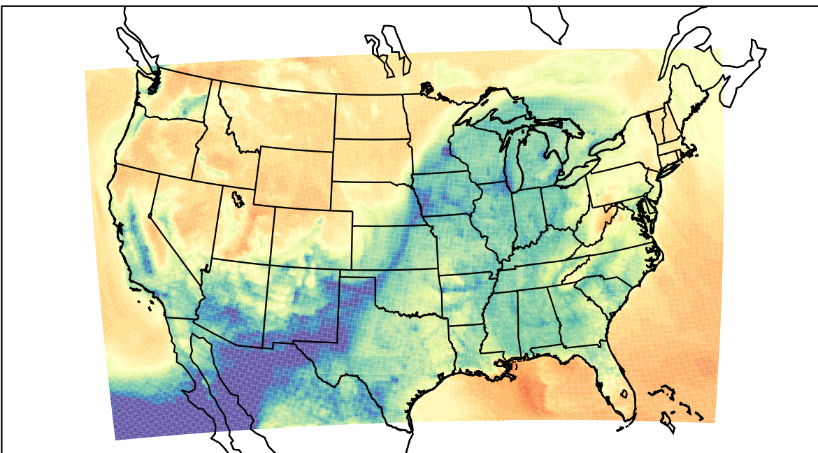
WRF (2023-03-16_14:00:00)
