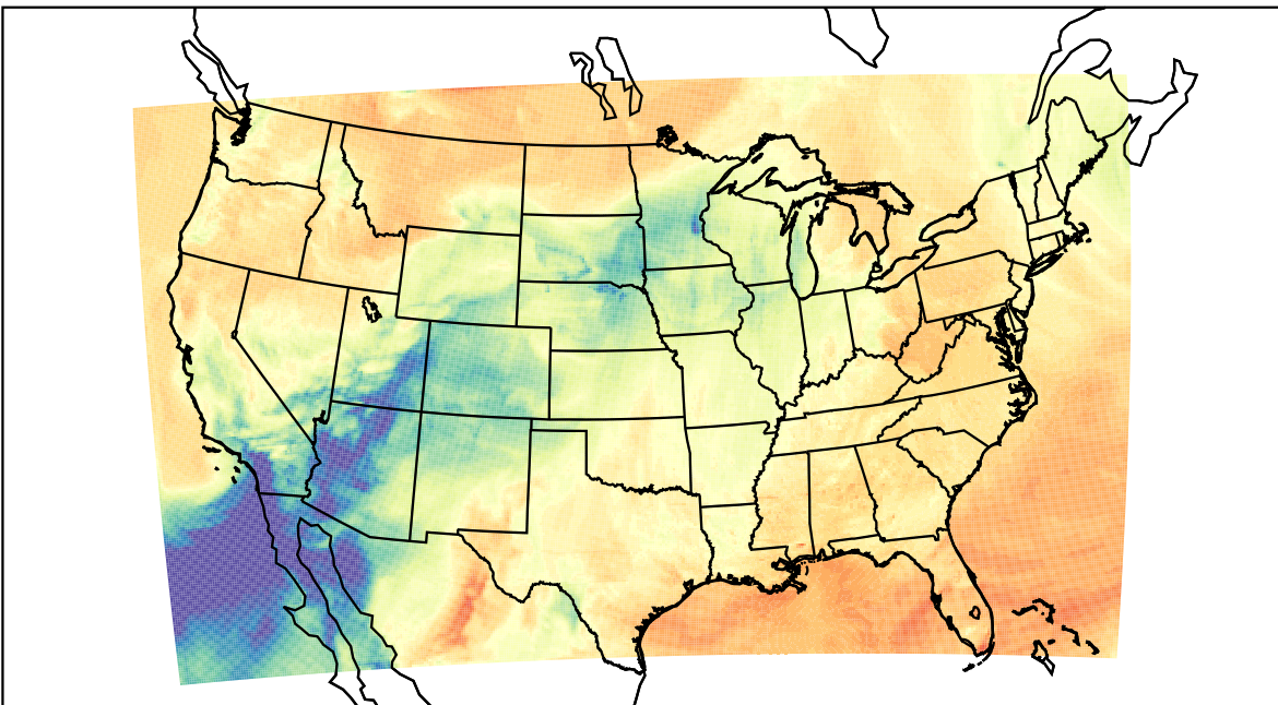
WRF (2023-03-15_20:00:00)
