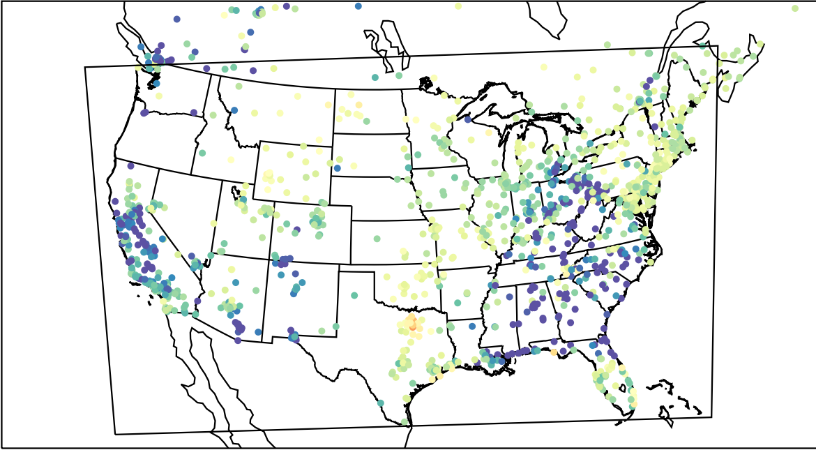
AirNOW (2023-03-16_04:00:00)
