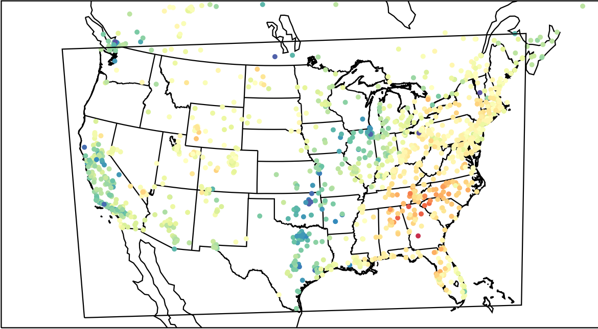
AirNOW (2023-03-16_20:00:00)
