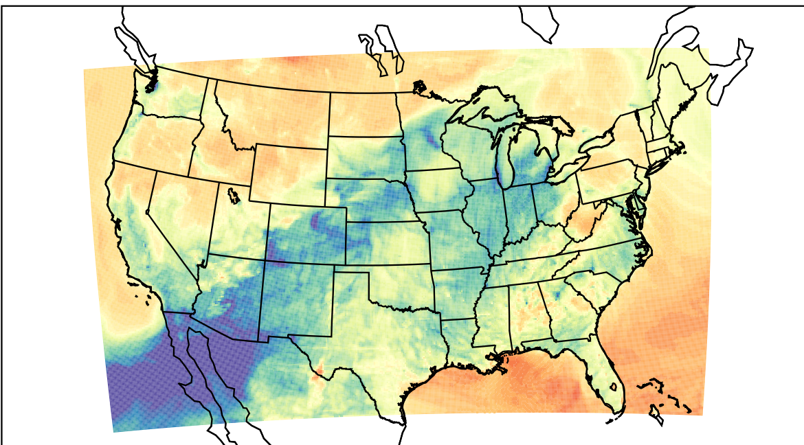
WRF (2023-03-16_03:00:00)
