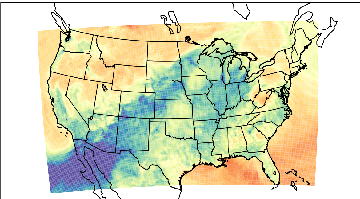
WRF (2023-03-16_04:00:00)
