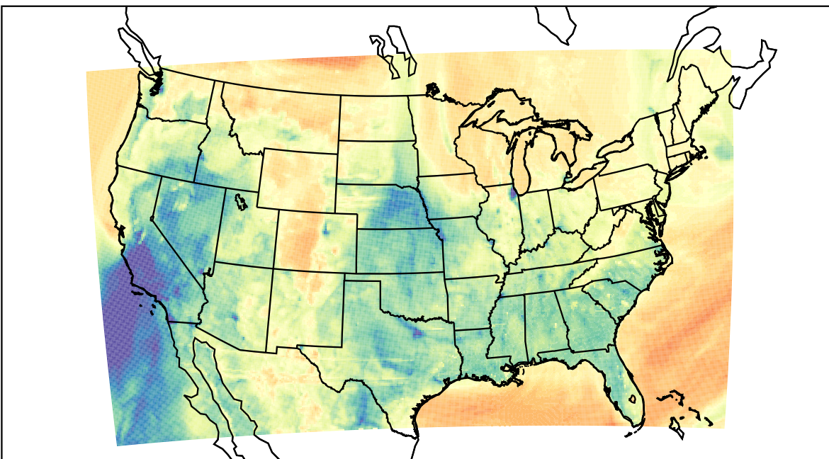
WRF (2023-03-15_03:00:00)
