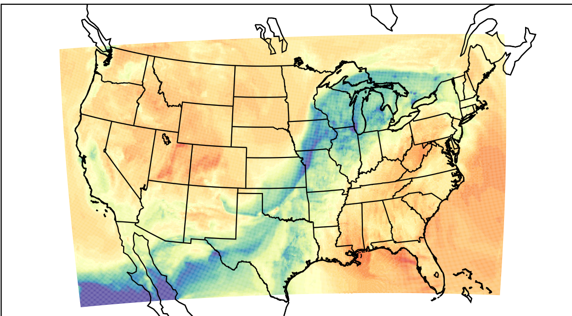
WRF (2023-03-16_20:00:00)
