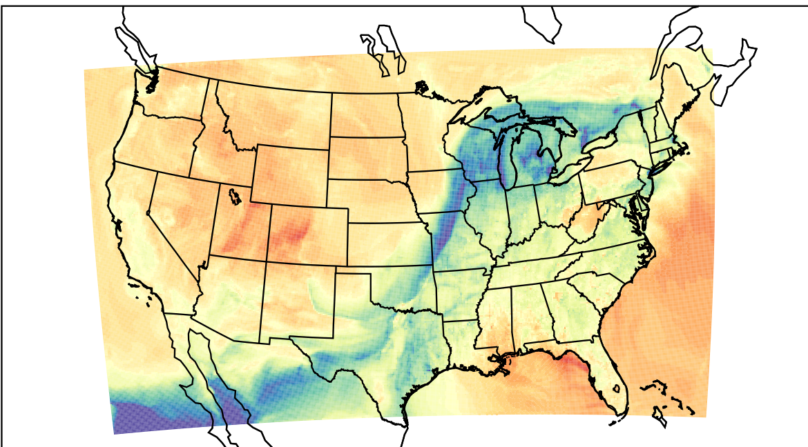
WRF (2023-03-16_23:00:00)
