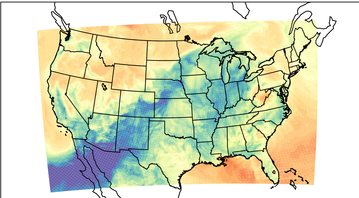
WRF (2023-03-16_06:00:00)
