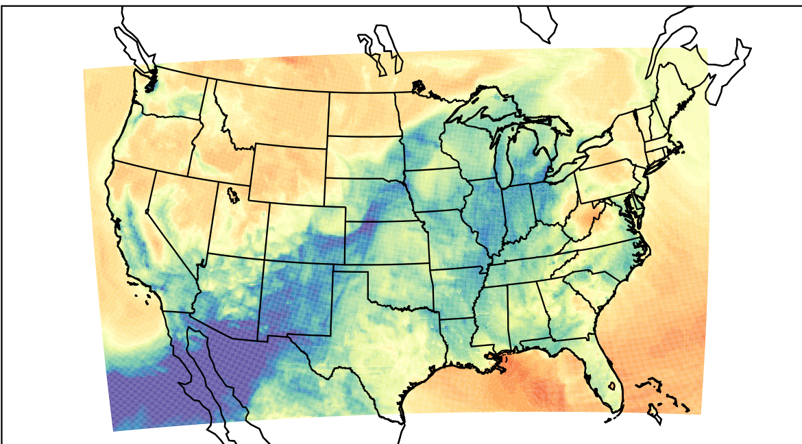
WRF (2023-03-16_07:00:00)
