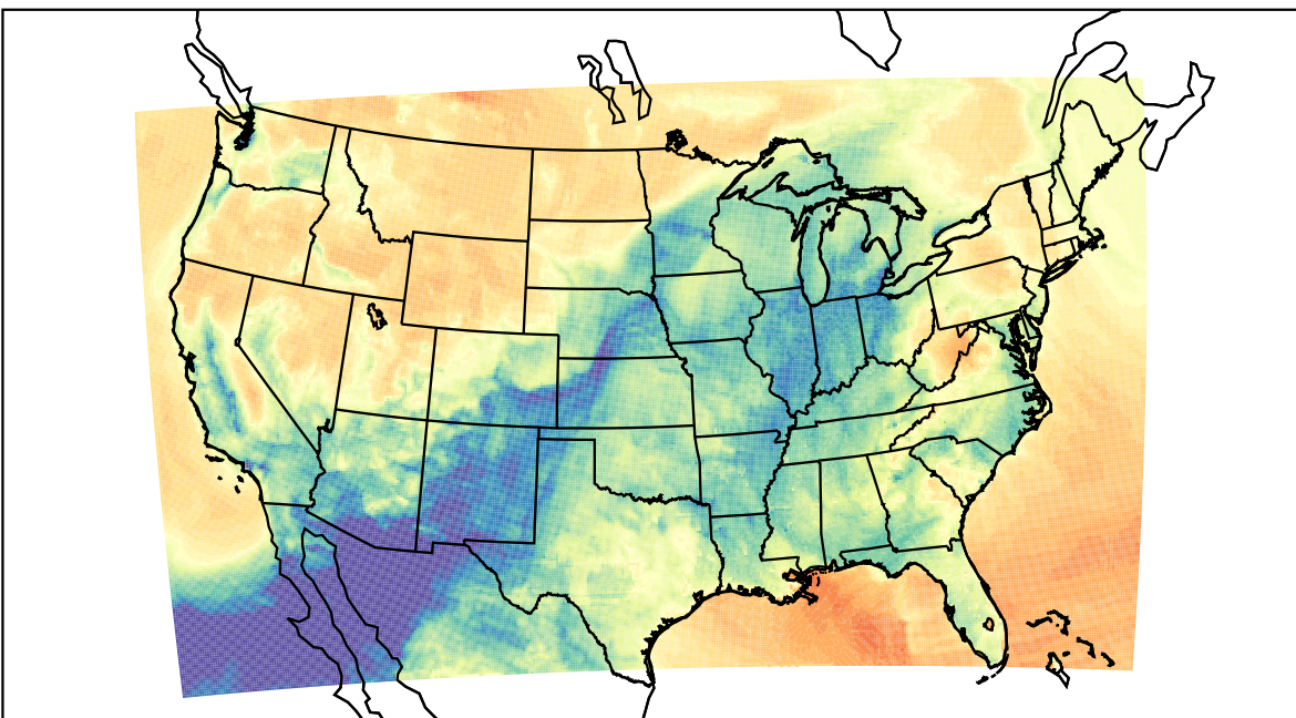
WRF (2023-03-16_08:00:00)
