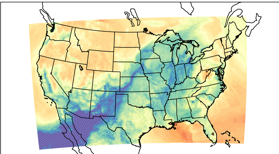
WRF (2023-03-16_10:00:00)
