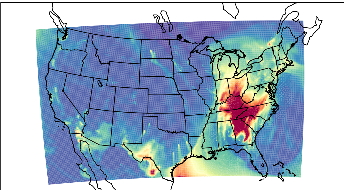
WRF 2023-03-17_08:00:00
