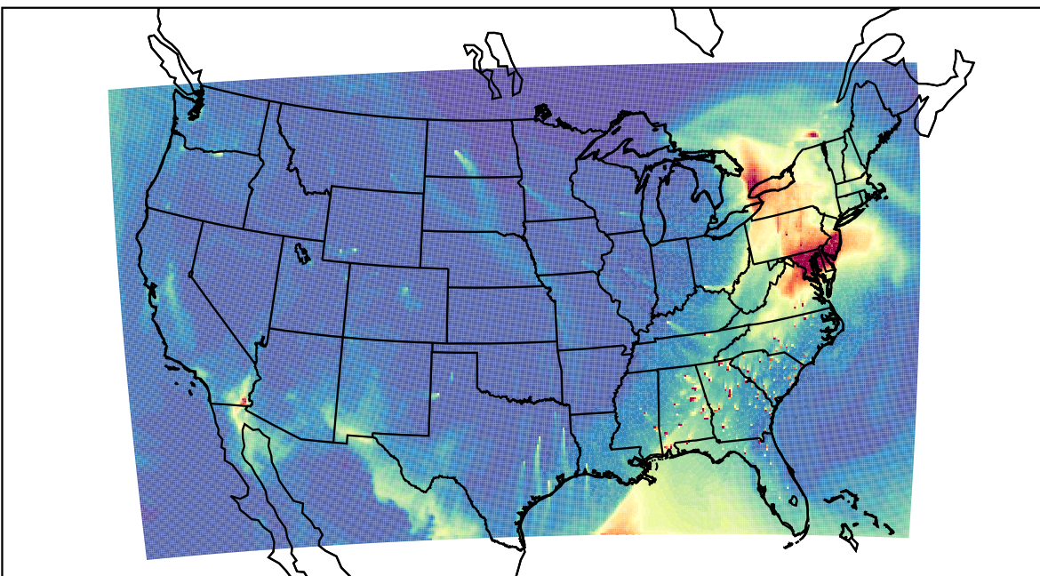
WRF 2023-03-17_18:00:00
