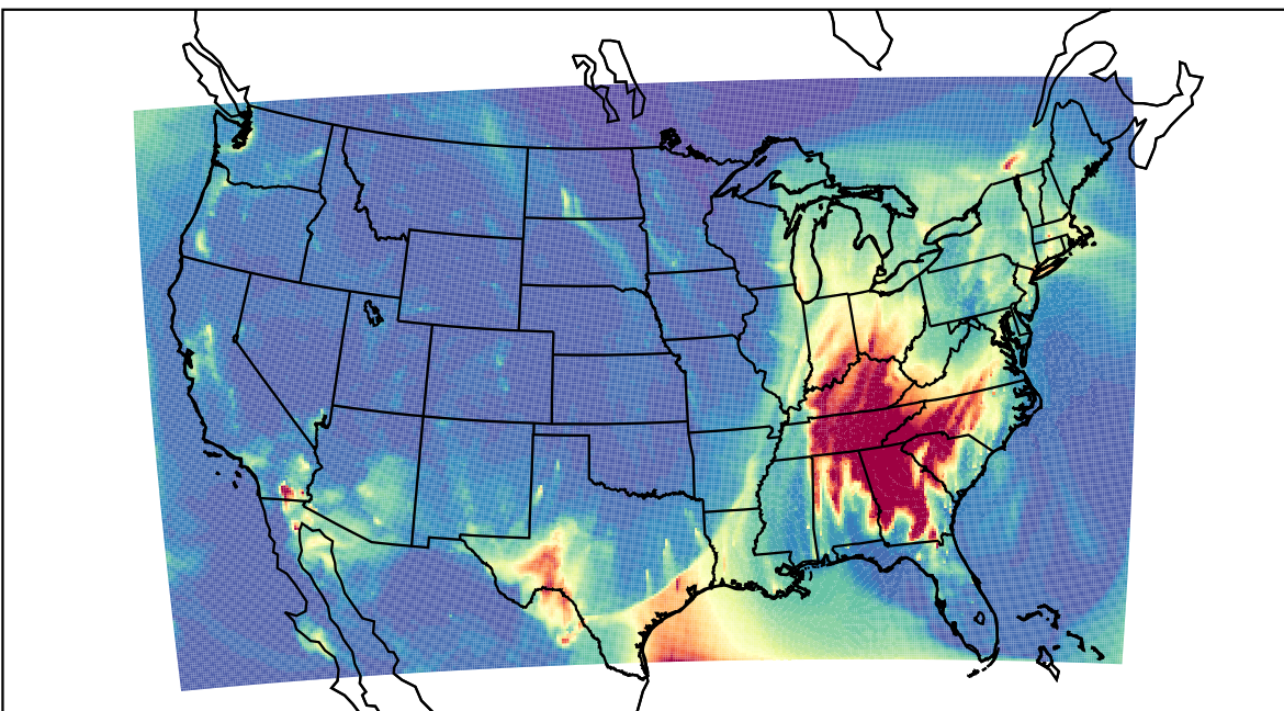
WRF 2023-03-17_06:00:00
