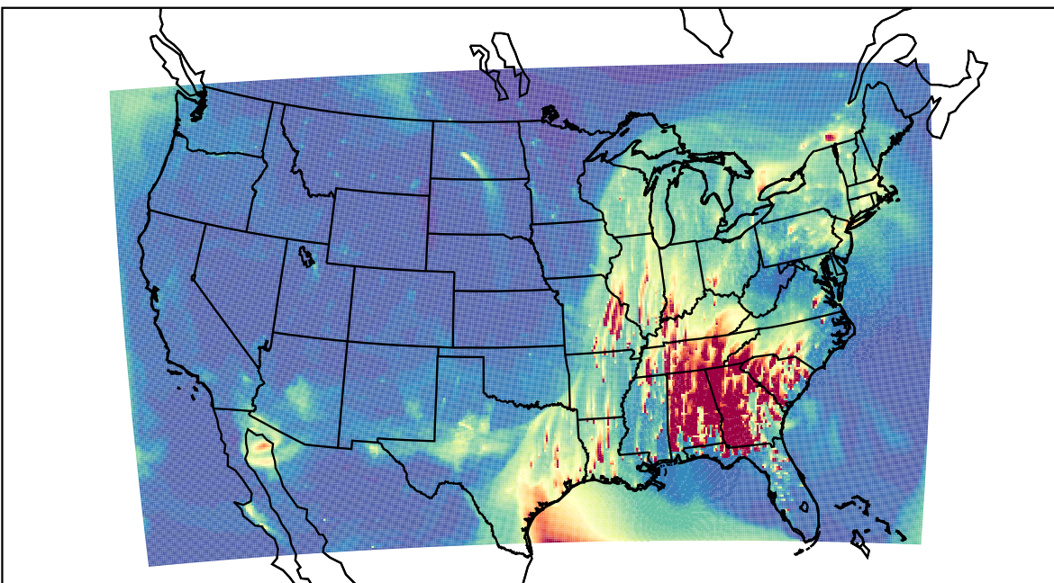
WRF 2023-03-17_00:00:00
