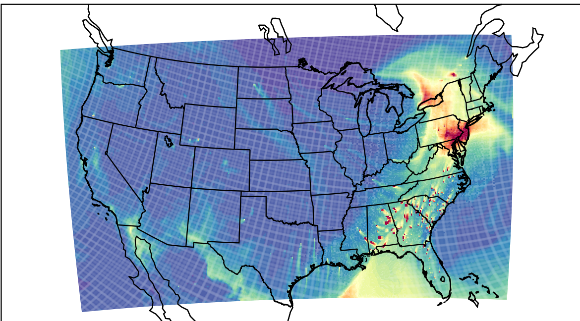
WRF 2023-03-17_20:00:00
