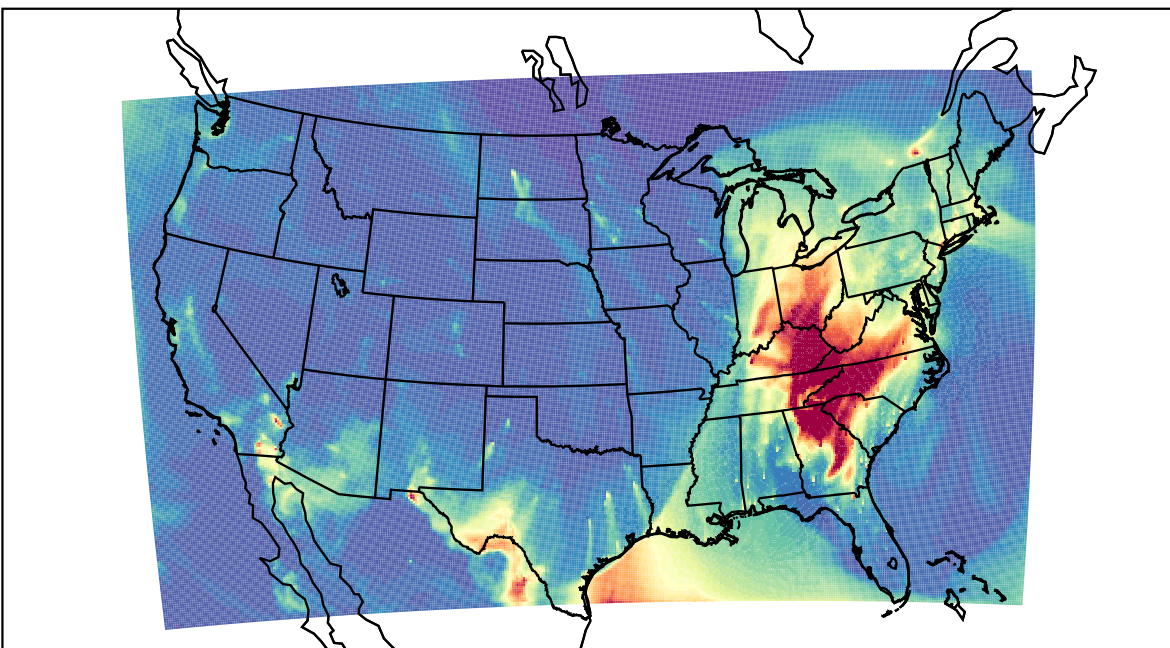
WRF 2023-03-17_09:00:00
