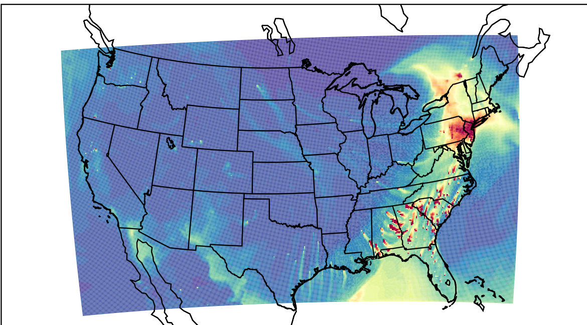
WRF 2023-03-17_22:00:00
