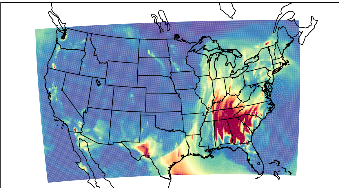
WRF 2023-03-17_04:00:00
