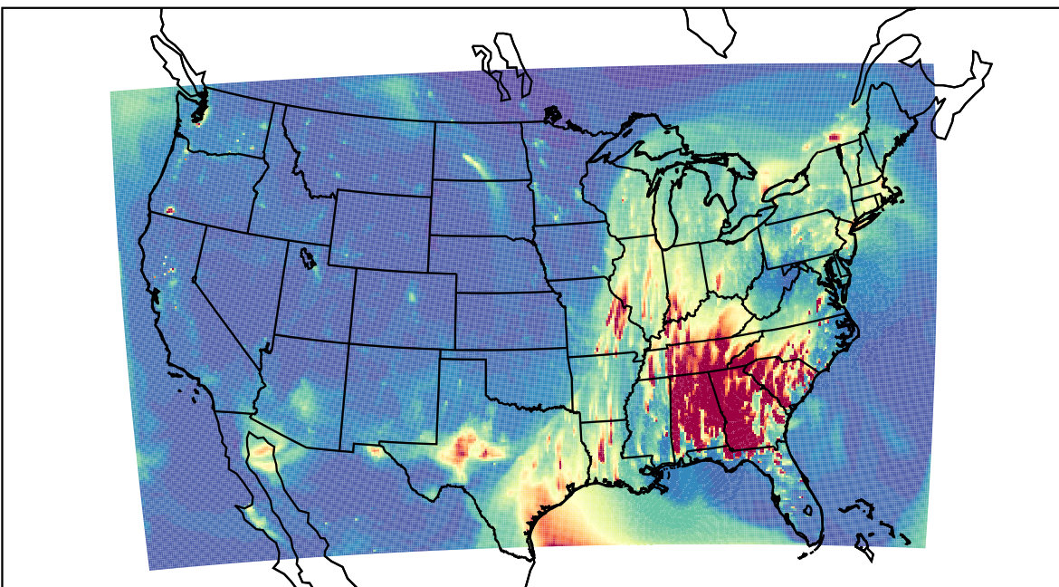
WRF 2023-03-17_01:00:00
