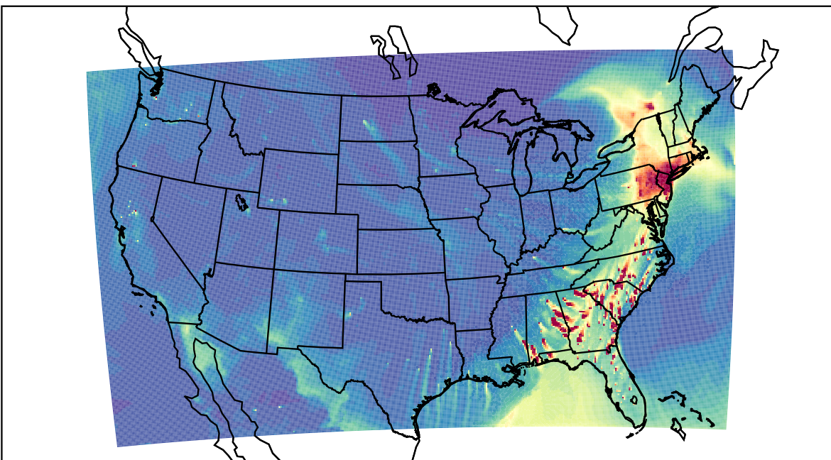
WRF 2023-03-17_23:00:00
