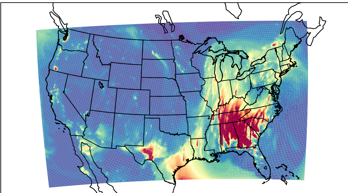
WRF 2023-03-17_03:00:00
