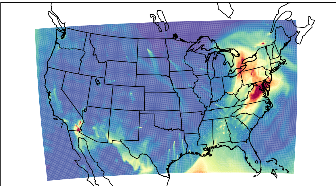
WRF 2023-03-17_16:00:00
