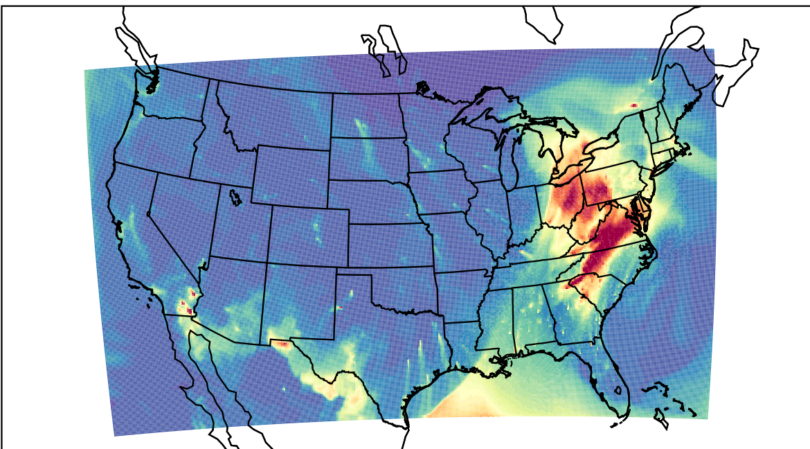
WRF 2023-03-17_13:00:00
