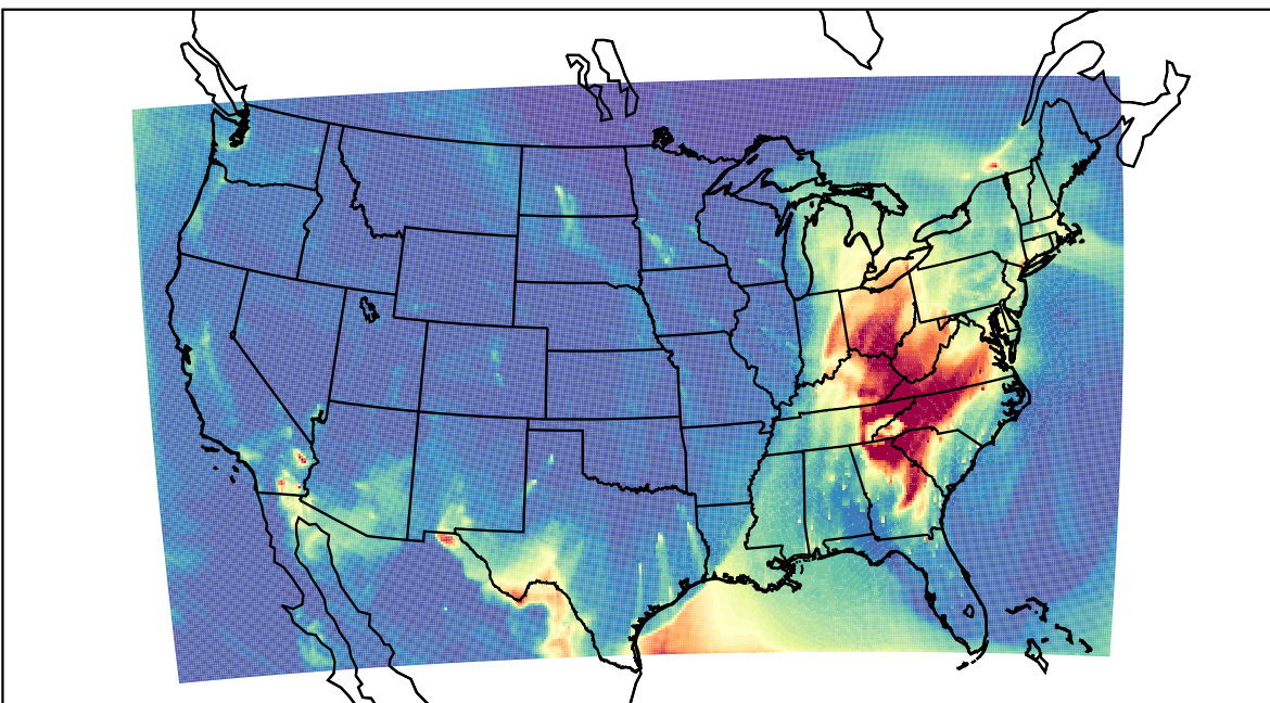
WRF 2023-03-17_10:00:00
