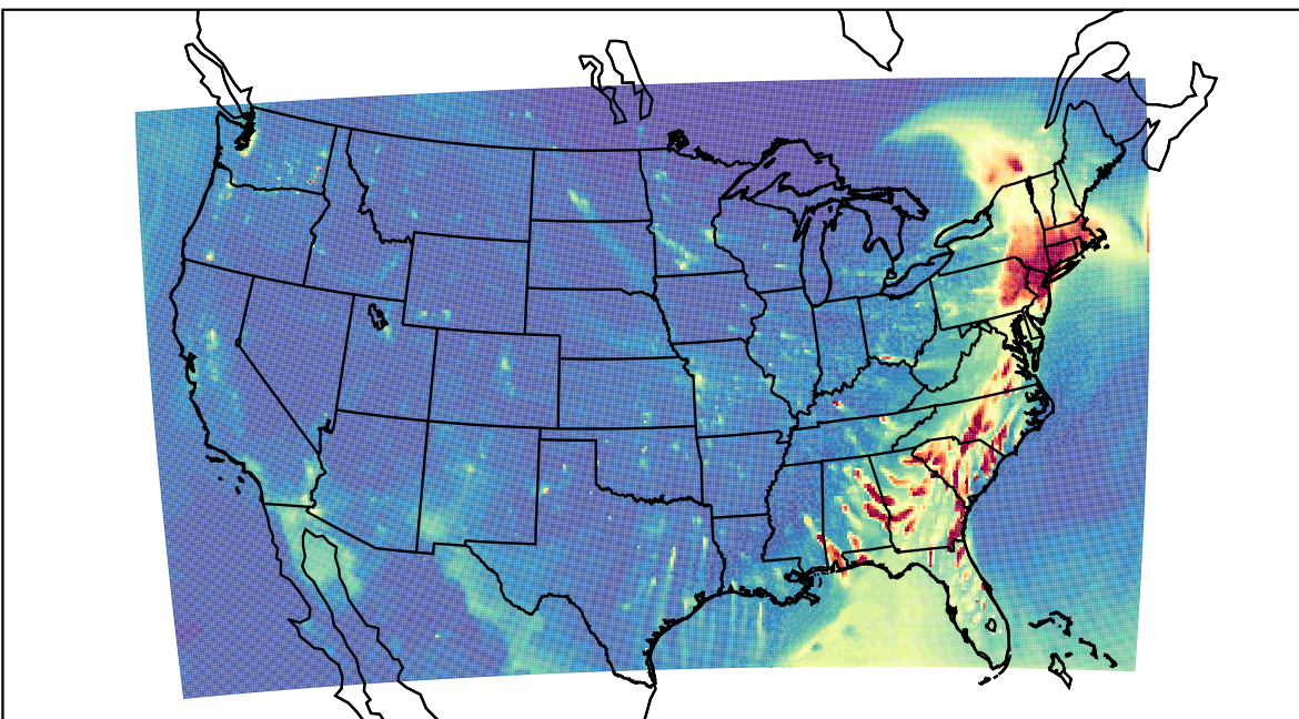
WRF 2023-03-18_01:00:00
