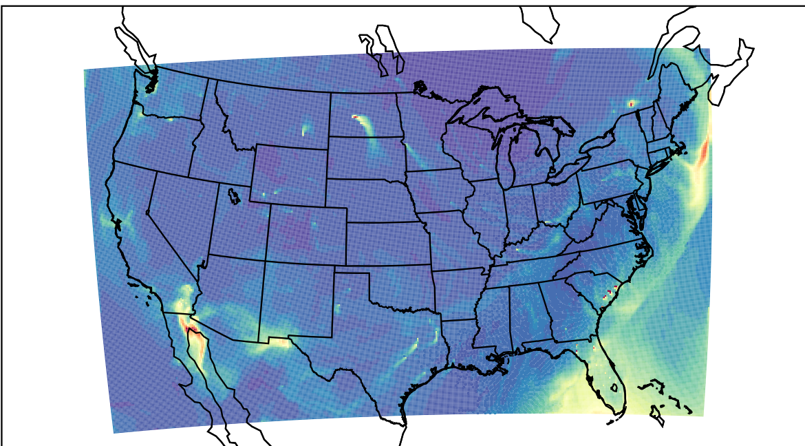
WRF 2023-03-18_18:00:00
