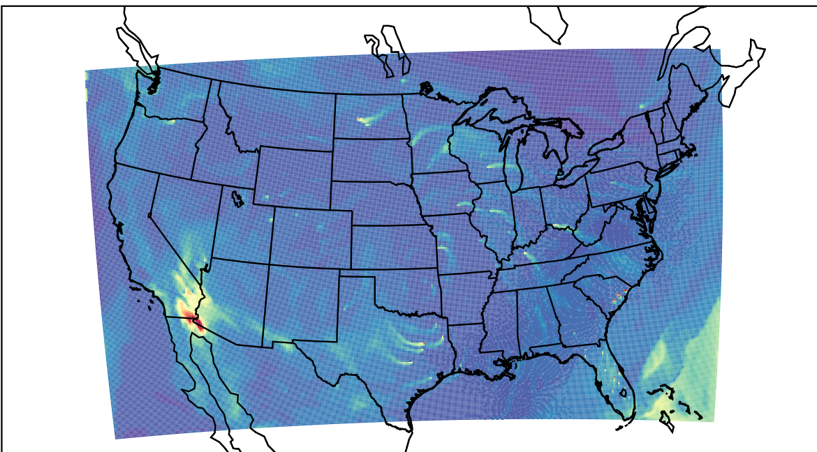
WRF 2023-03-19_18:00:00
