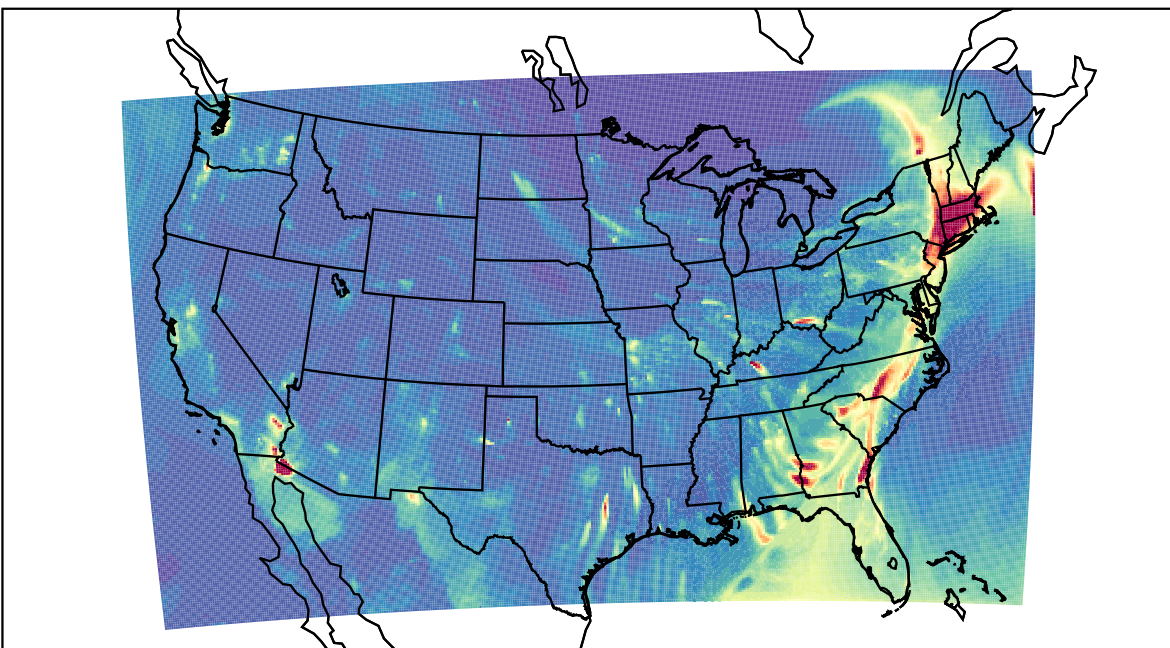
WRF 2023-03-18_04:00:00
