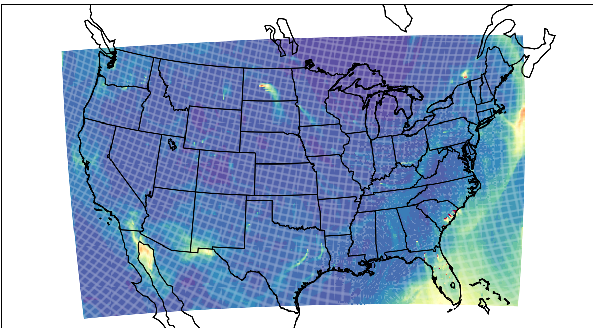
WRF 2023-03-18_20:00:00
