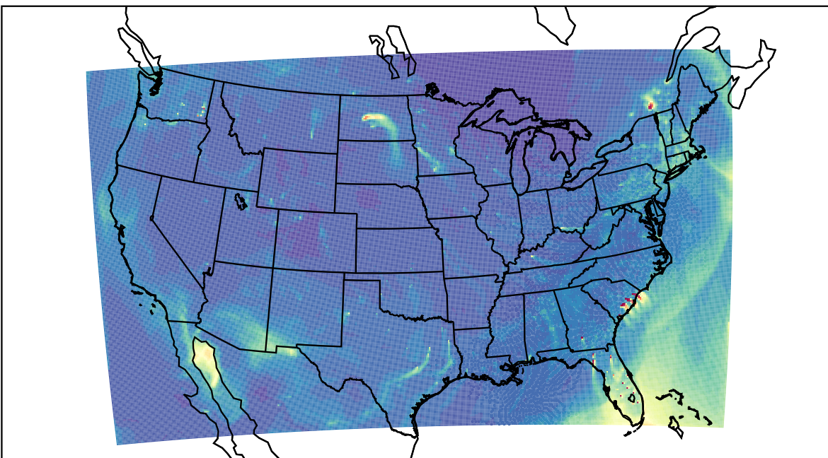
WRF 2023-03-18_23:00:00
