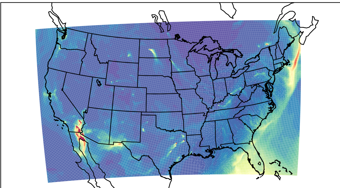
WRF 2023-03-18_16:00:00
