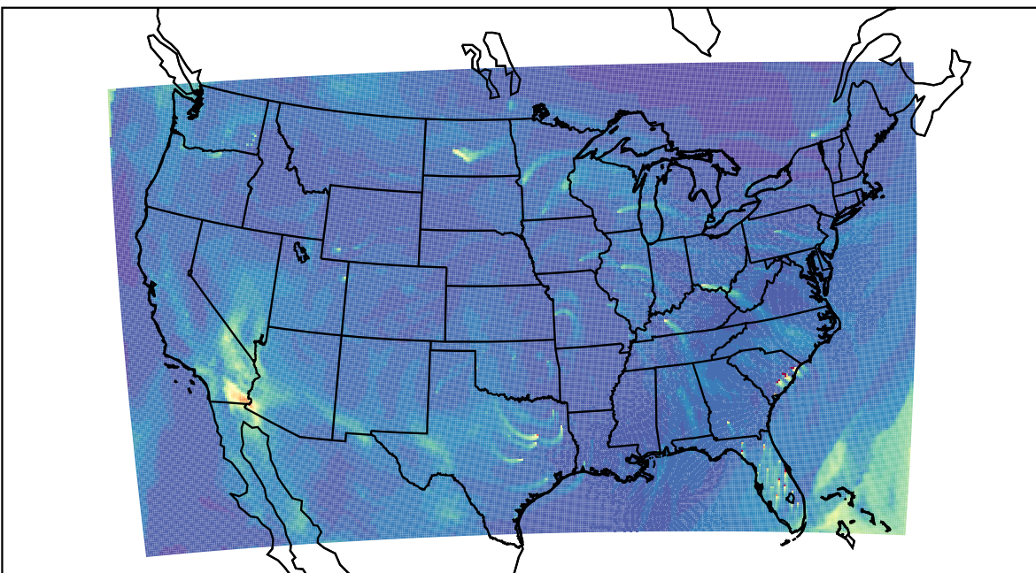
WRF 2023-03-19_20:00:00
