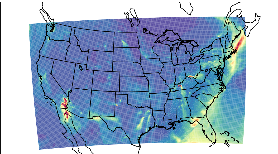
WRF 2023-03-18_11:00:00
