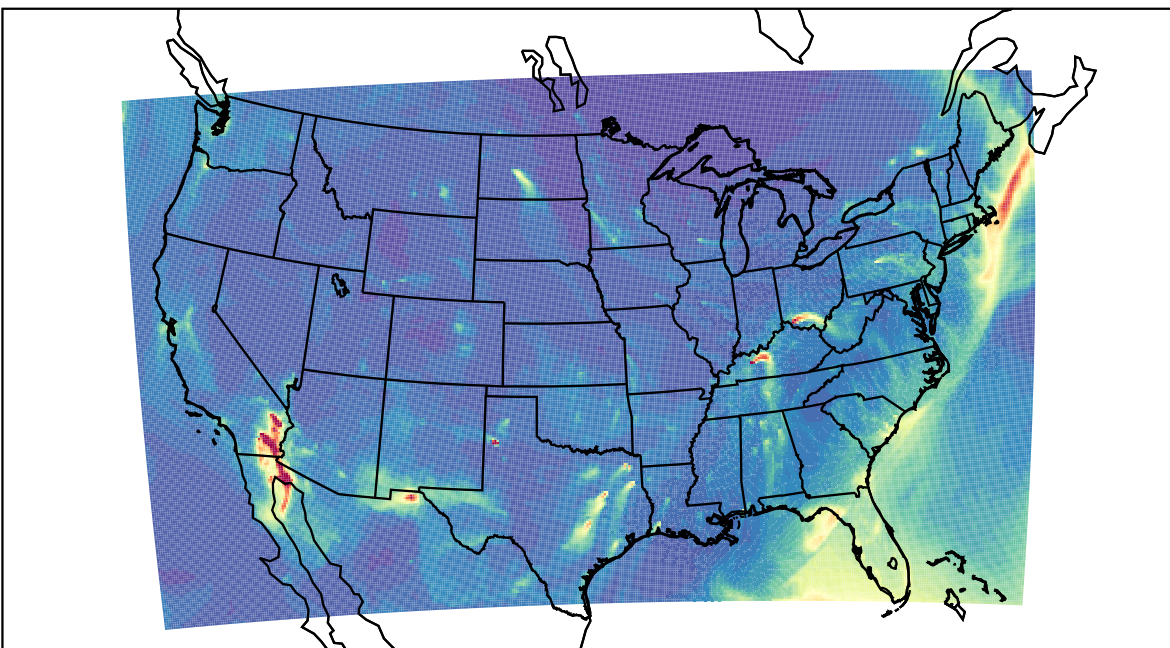
WRF 2023-03-18_13:00:00
