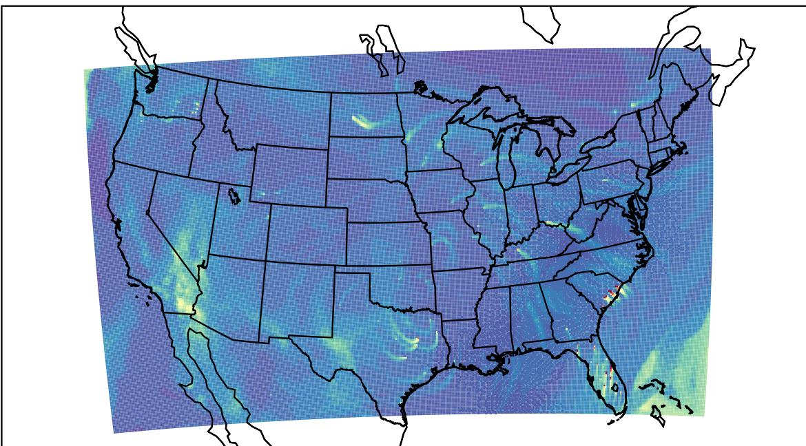
WRF 2023-03-19_22:00:00
