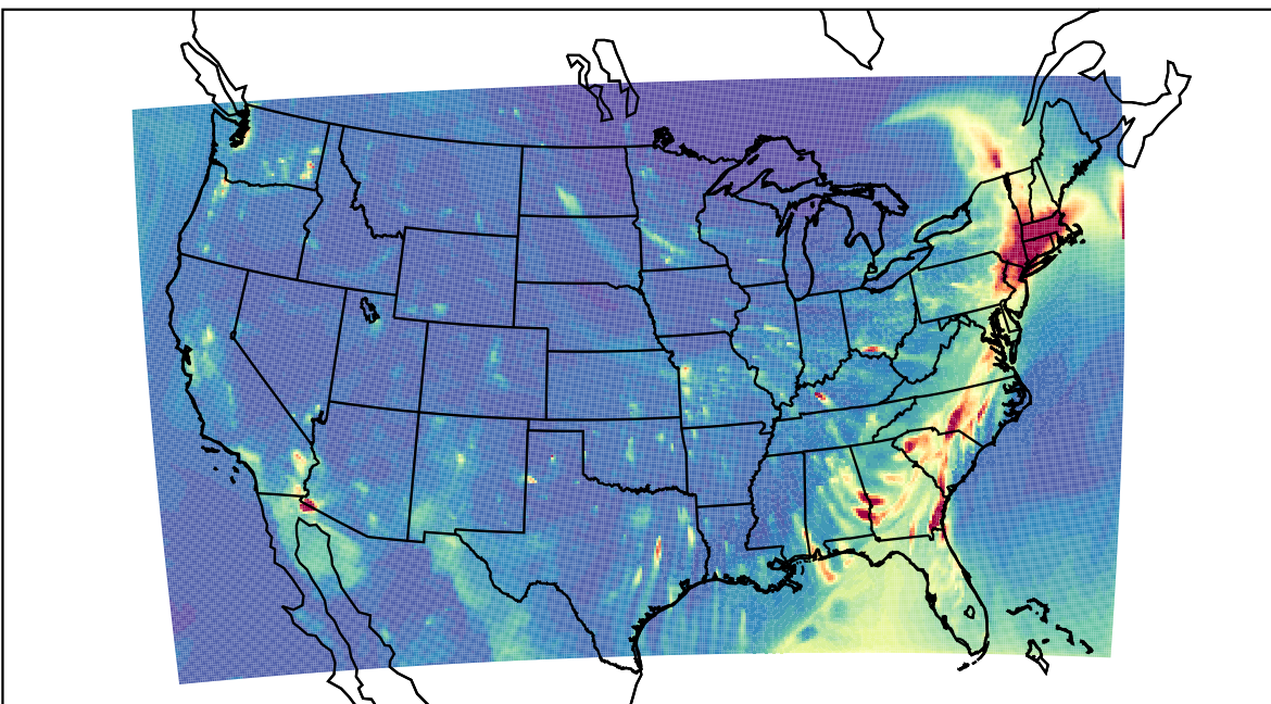
WRF 2023-03-18_03:00:00
