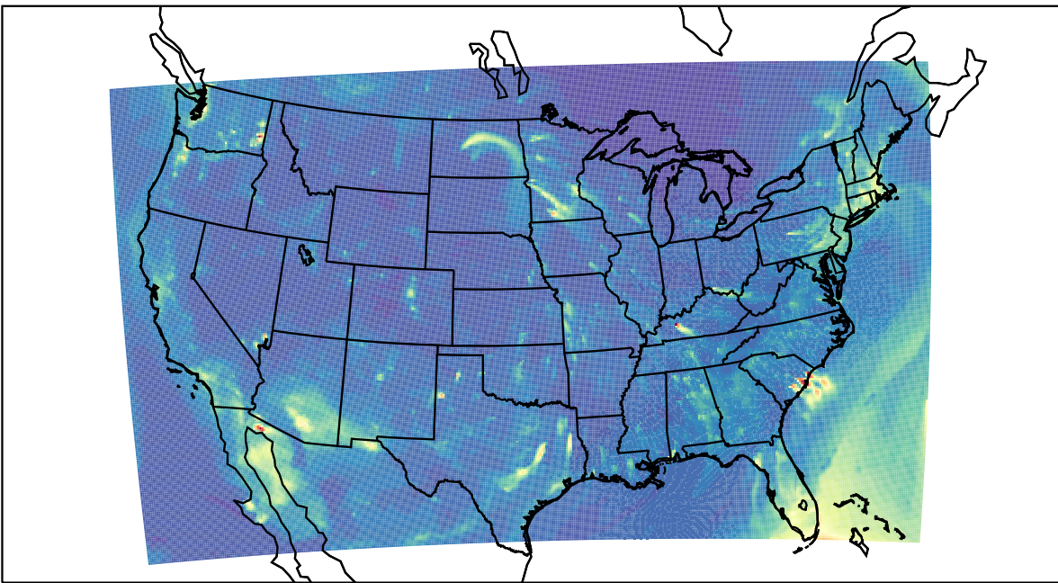
WRF 2023-03-19_03:00:00
