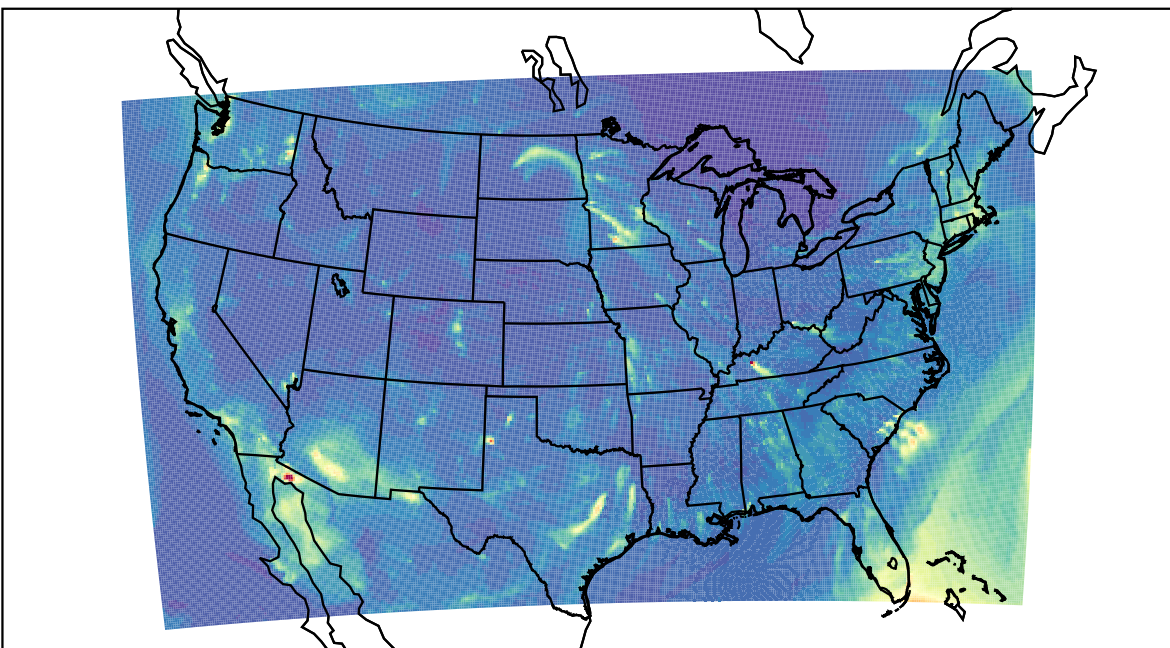
WRF 2023-03-19_04:00:00
