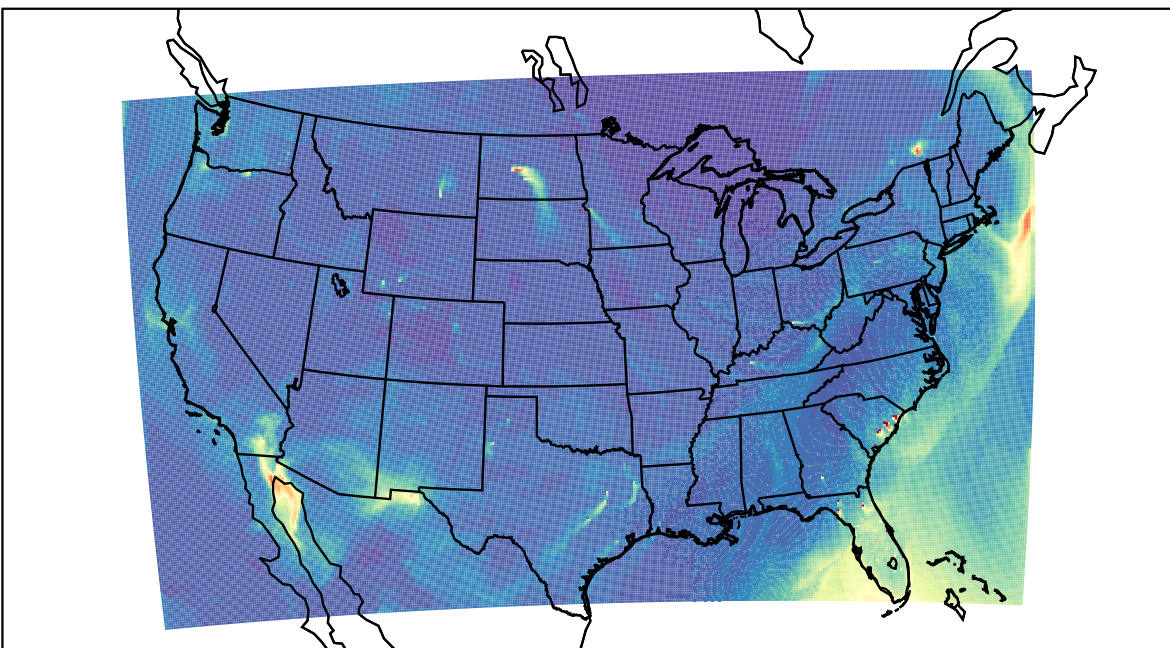
WRF 2023-03-18_19:00:00
