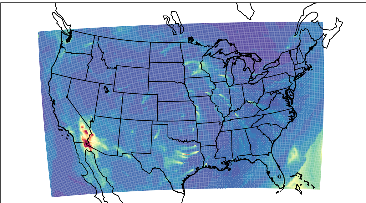
WRF 2023-03-19_14:00:00
