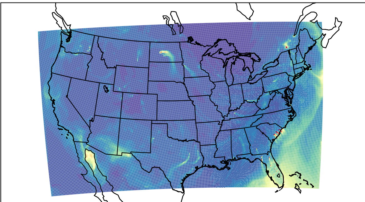
WRF 2023-03-18_22:00:00
