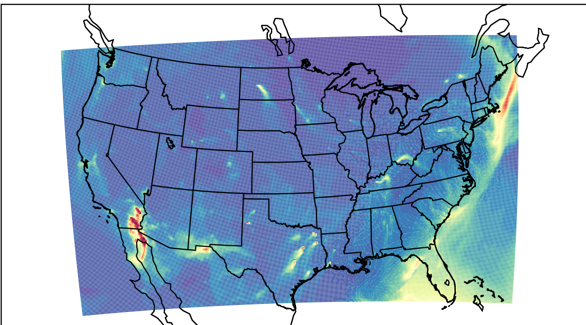
WRF 2023-03-18_14:00:00
