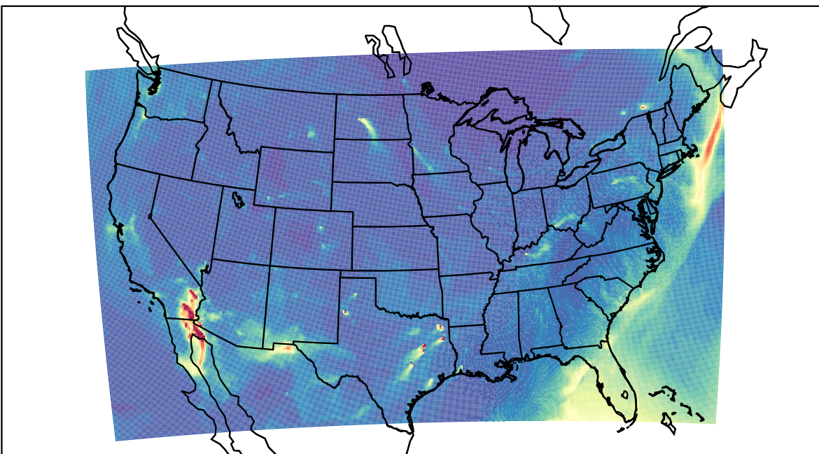
WRF 2023-03-18_15:00:00
