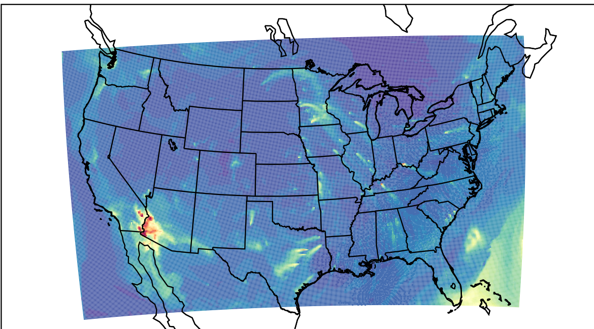
WRF 2023-03-19_10:00:00
