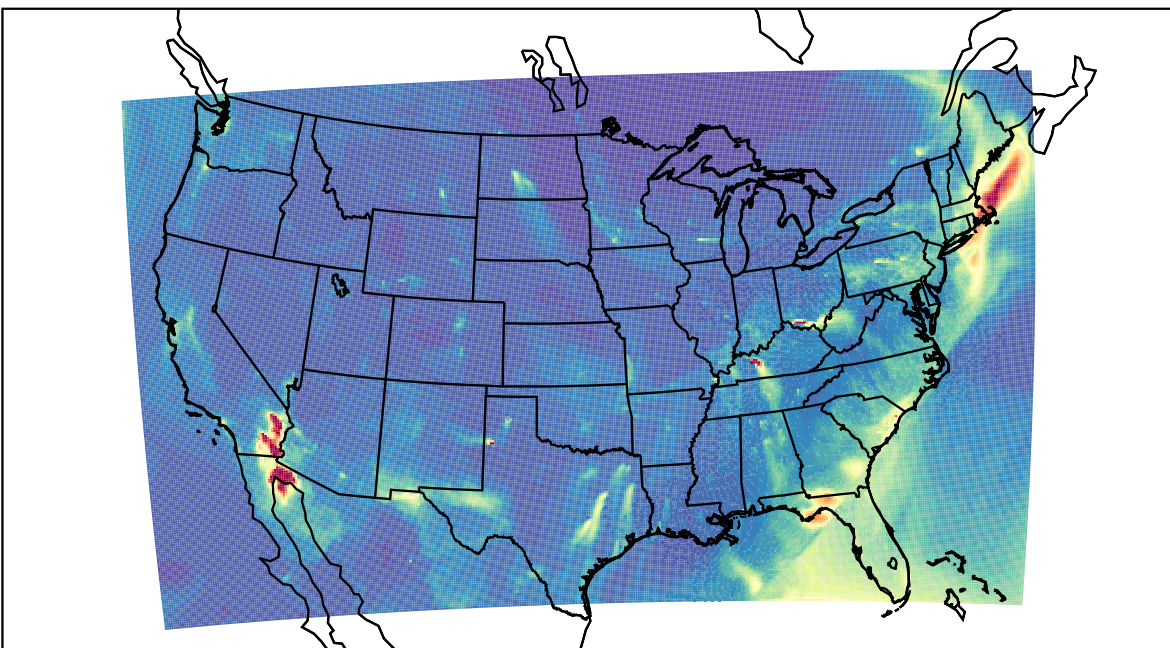
WRF 2023-03-18_10:00:00
