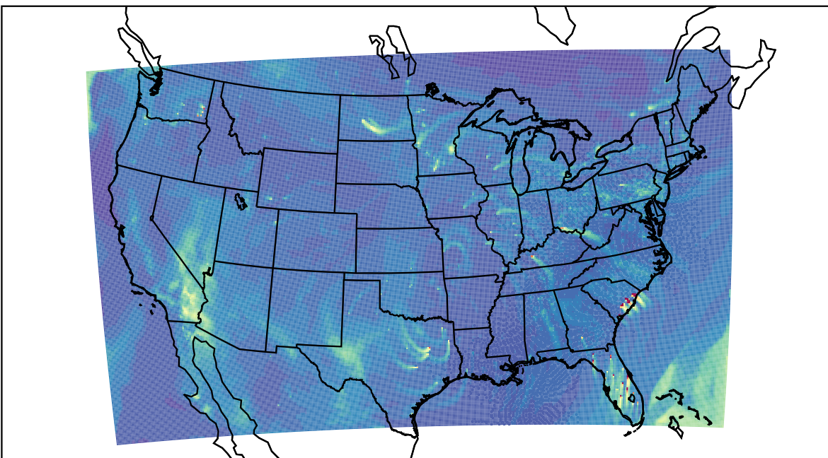
WRF 2023-03-19_23:00:00
