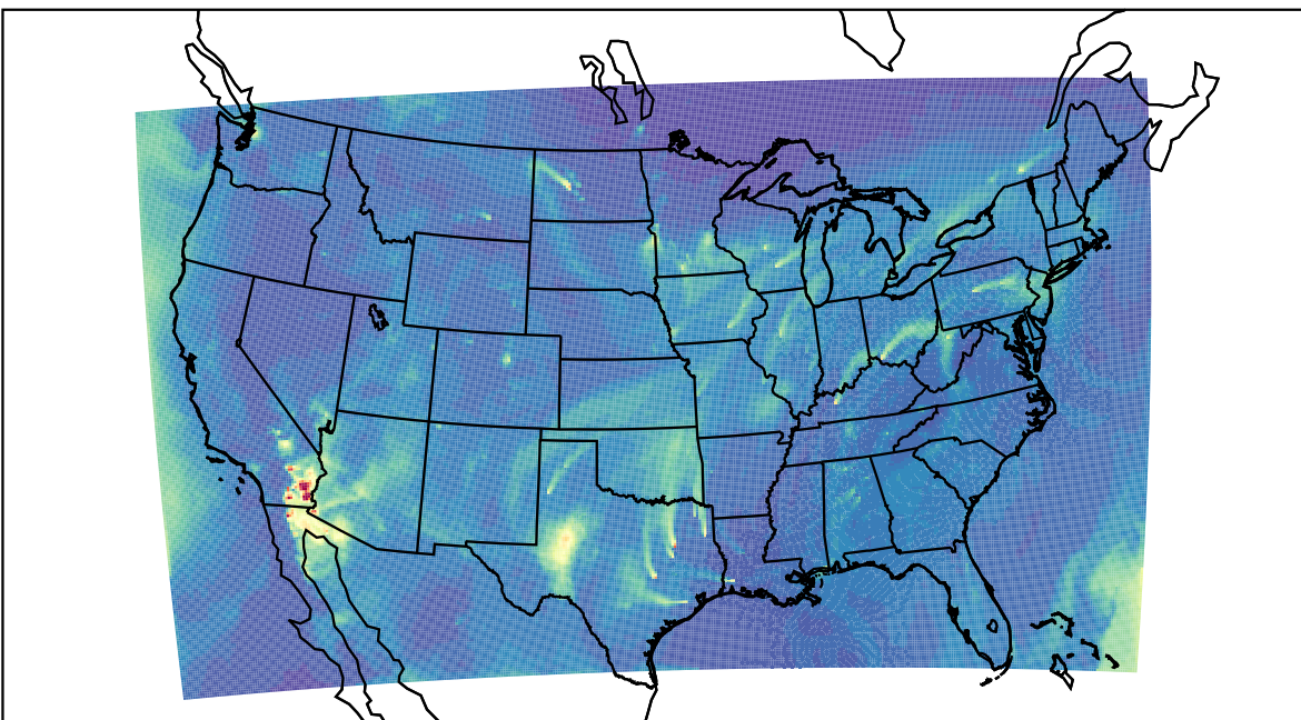
WRF 2023-03-20_16:00:00
