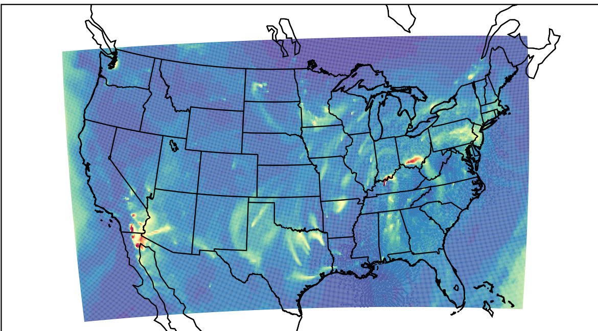
WRF 2023-03-20_11:00:00
