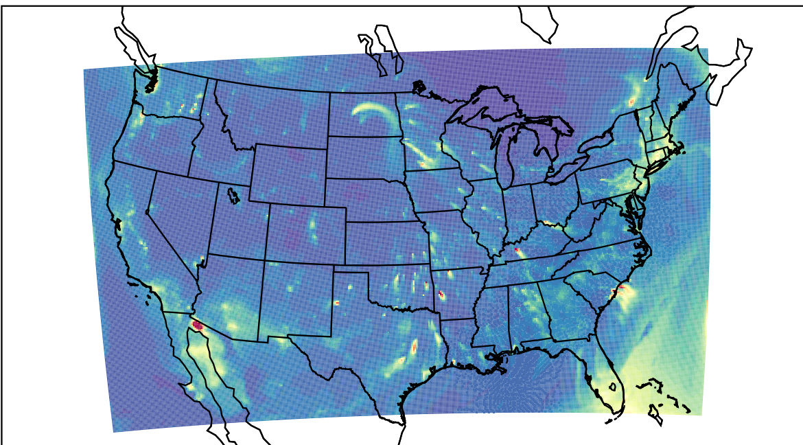
WRF 2023-03-19_03:00:00
