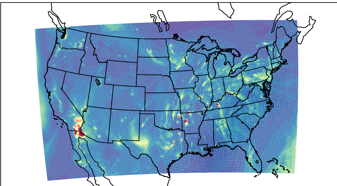
WRF 2023-03-20_03:00:00
