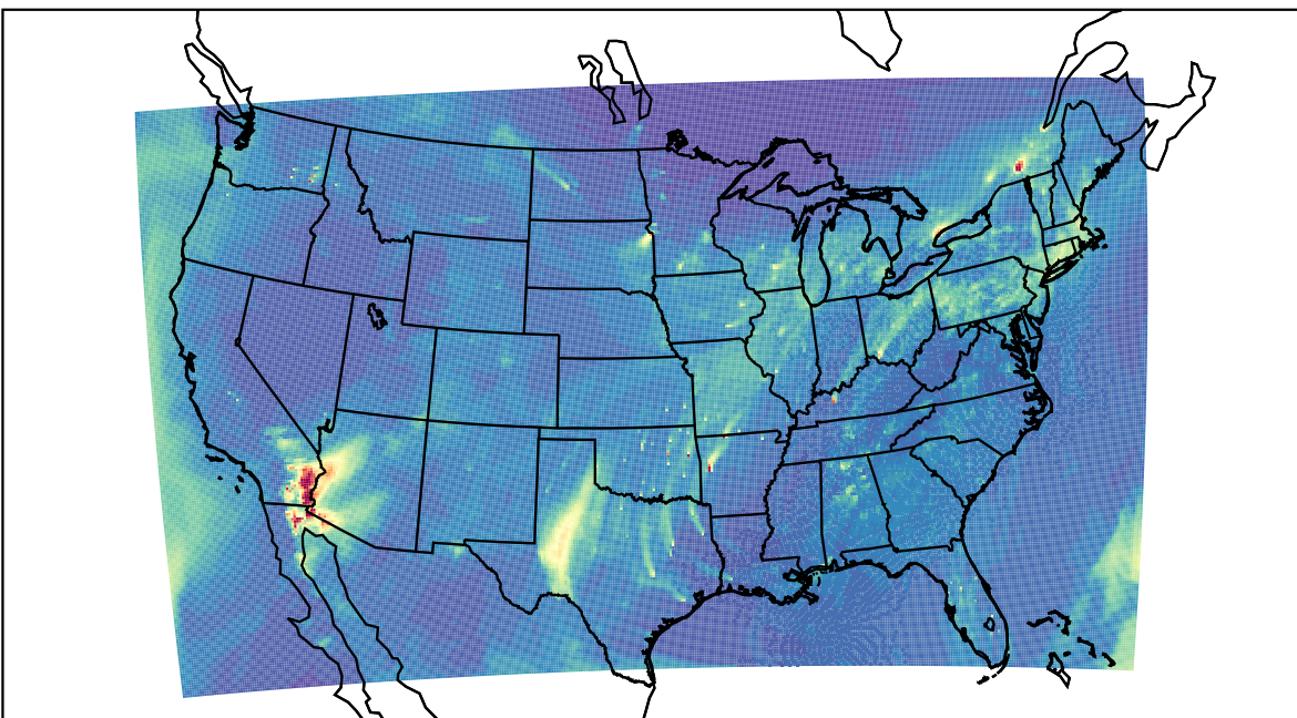
WRF 2023-03-20_23:00:00
