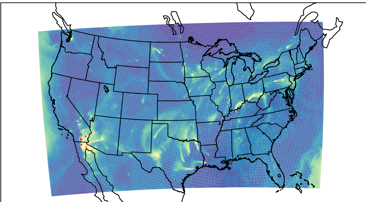
WRF 2023-03-20_14:00:00
