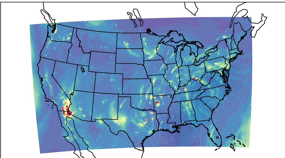
WRF 2023-03-20_04:00:00
