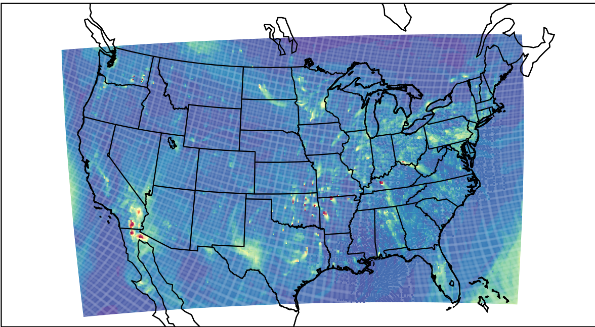
WRF 2023-03-20_01:00:00
