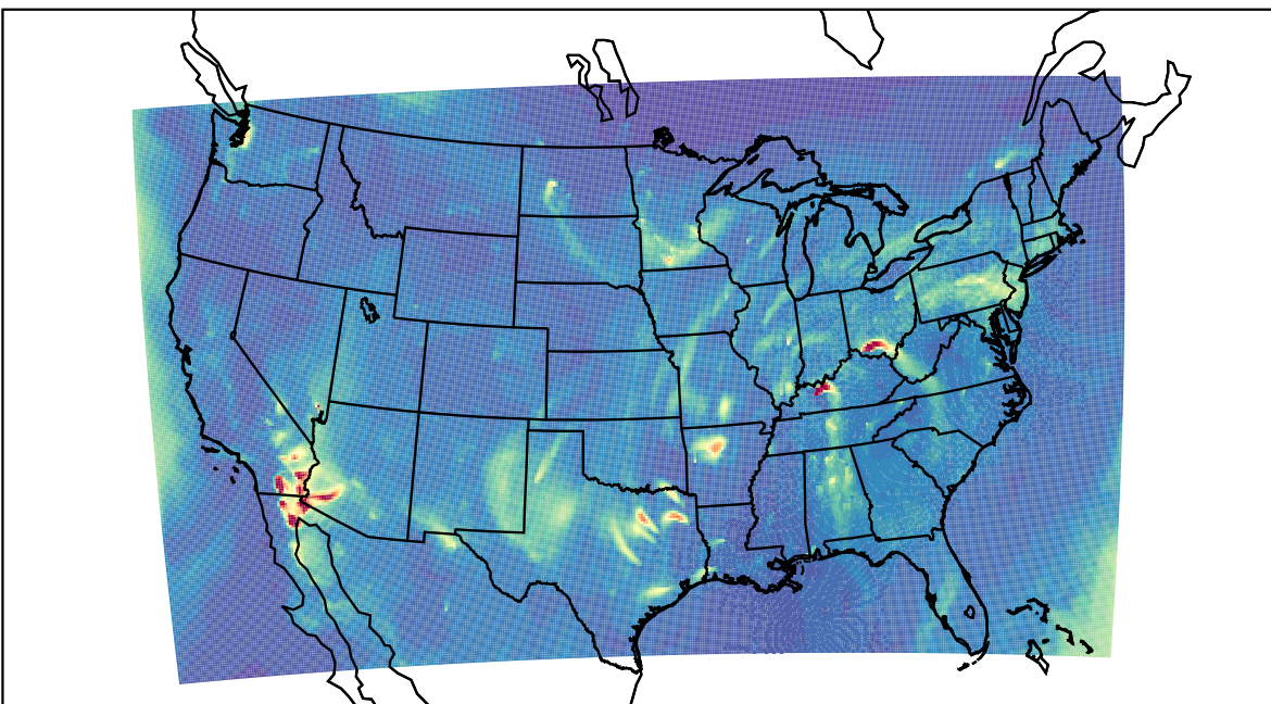
WRF 2023-03-20_08:00:00
