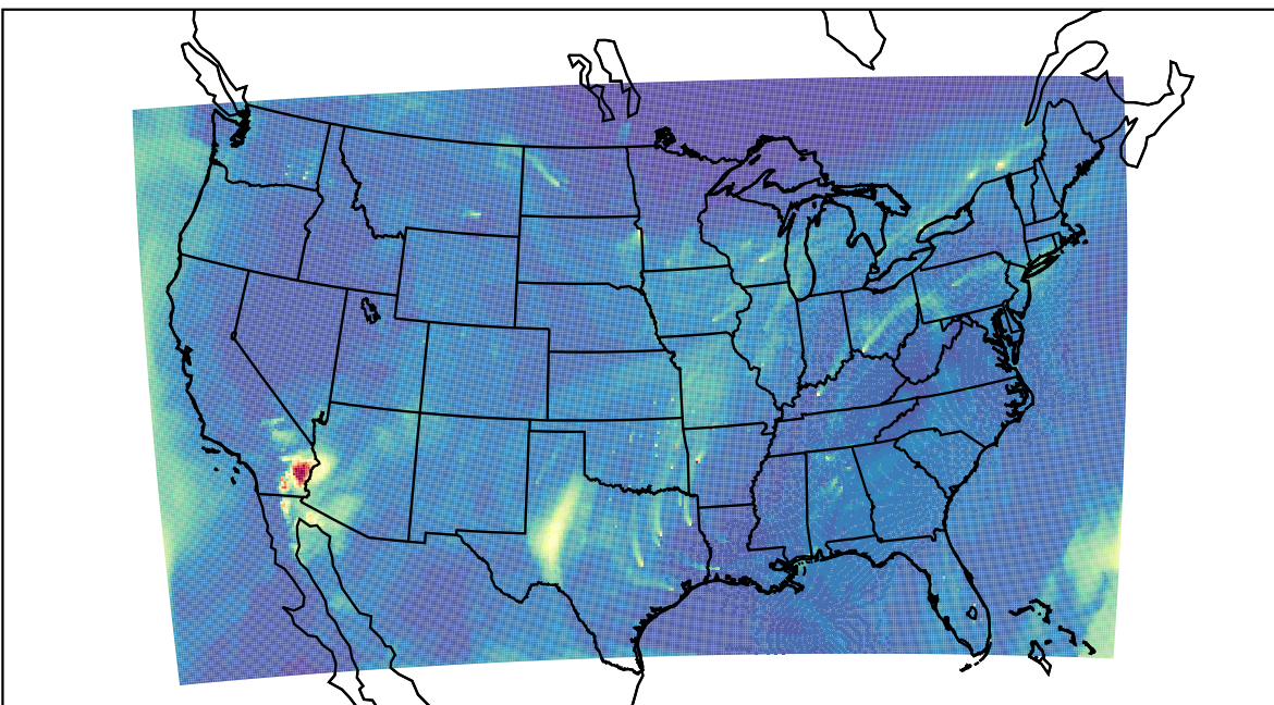
WRF 2023-03-20_20:00:00
