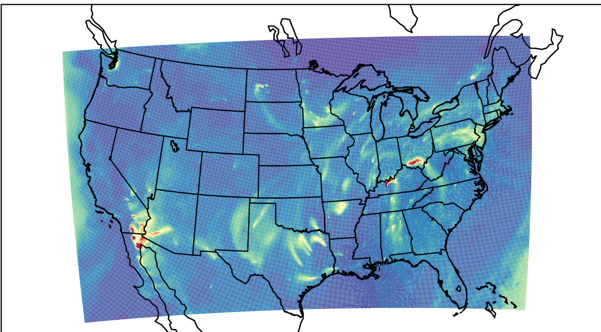
WRF 2023-03-20_10:00:00
