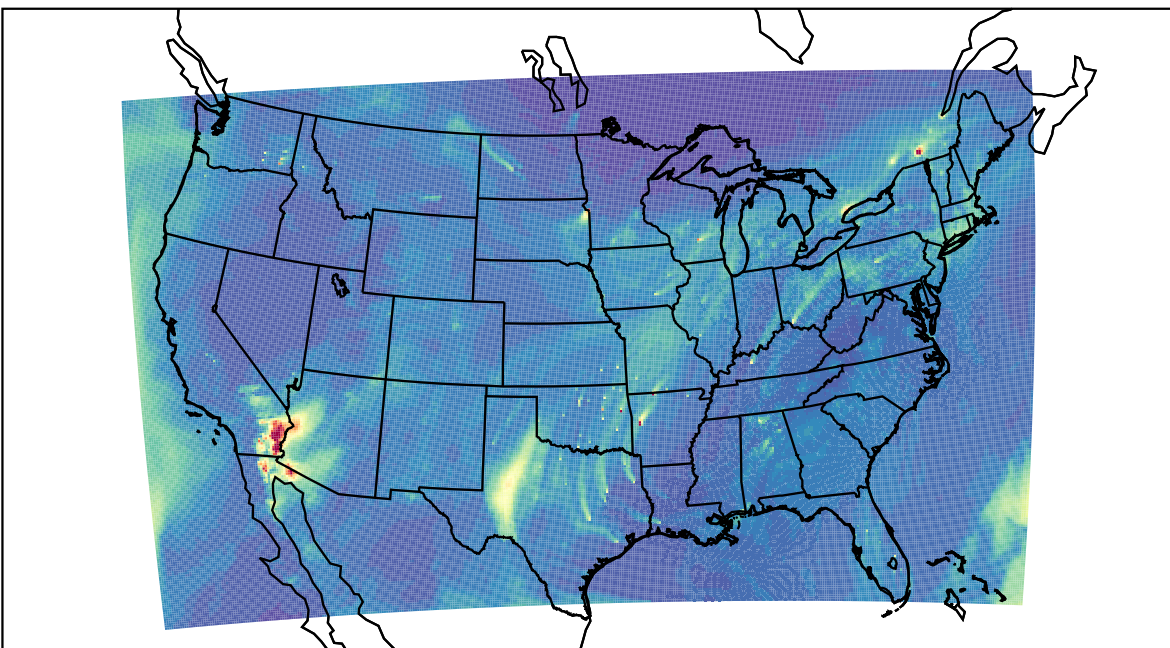
WRF 2023-03-20_22:00:00
