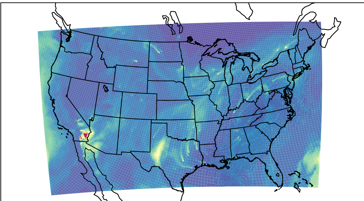
WRF 2023-03-20_19:00:00
