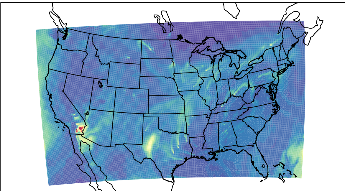
WRF 2023-03-20_18:00:00
