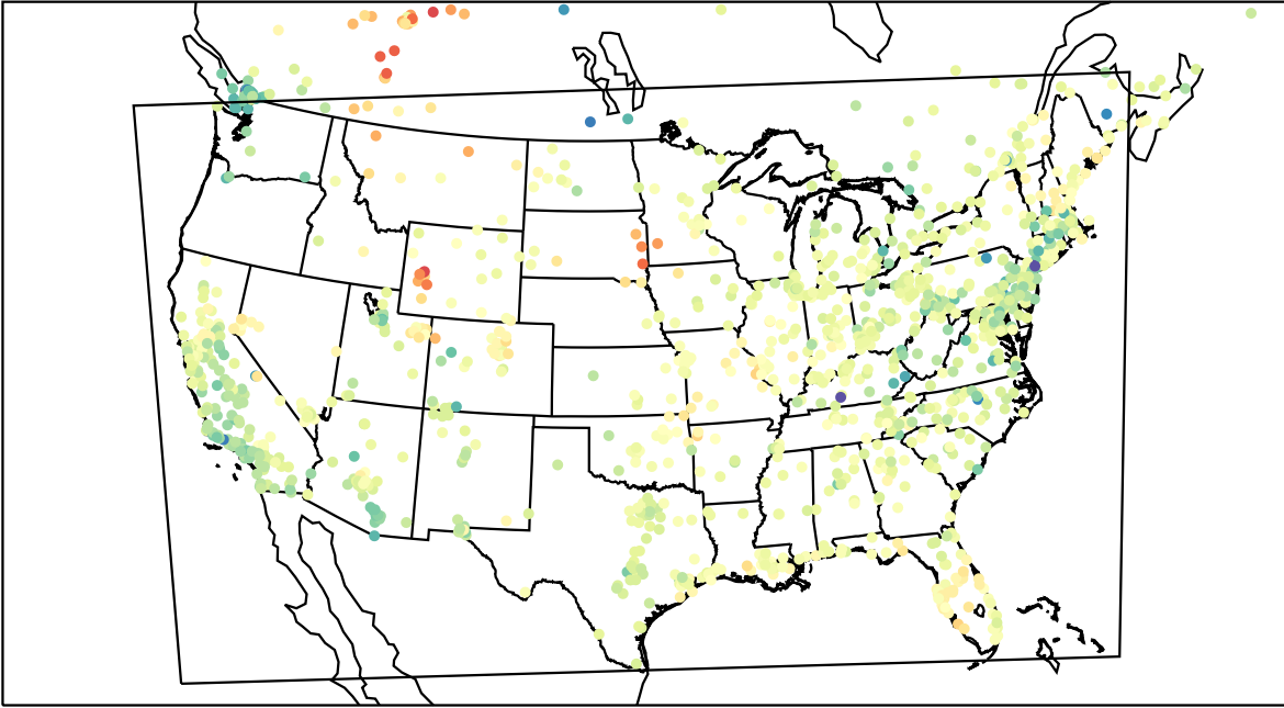
AirNOW (2023-03-20_23:00:00)
