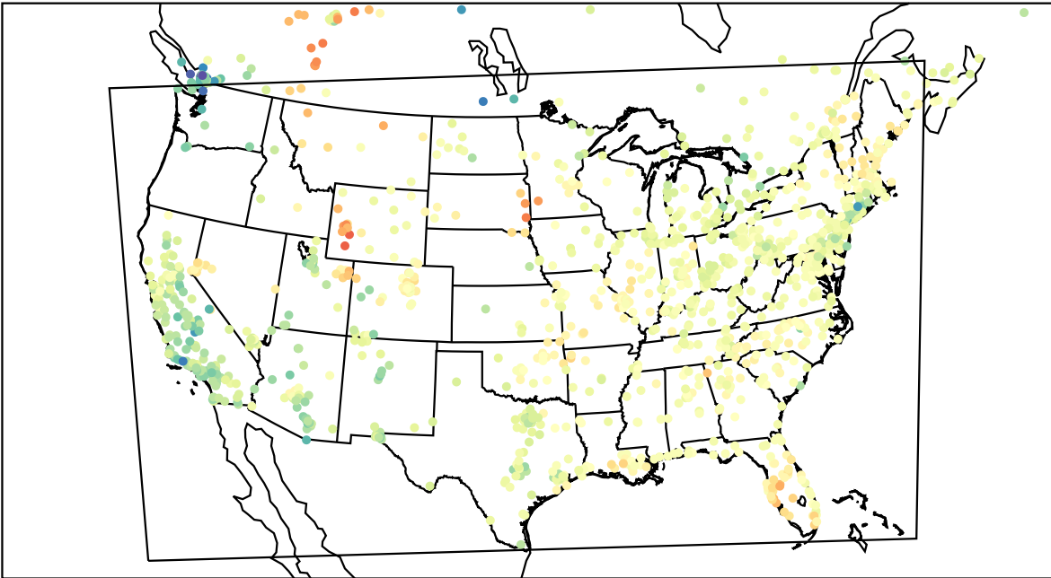
AirNOW (2023-03-20_20:00:00)
