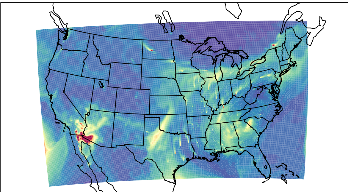
WRF 2023-03-21_16:00:00
