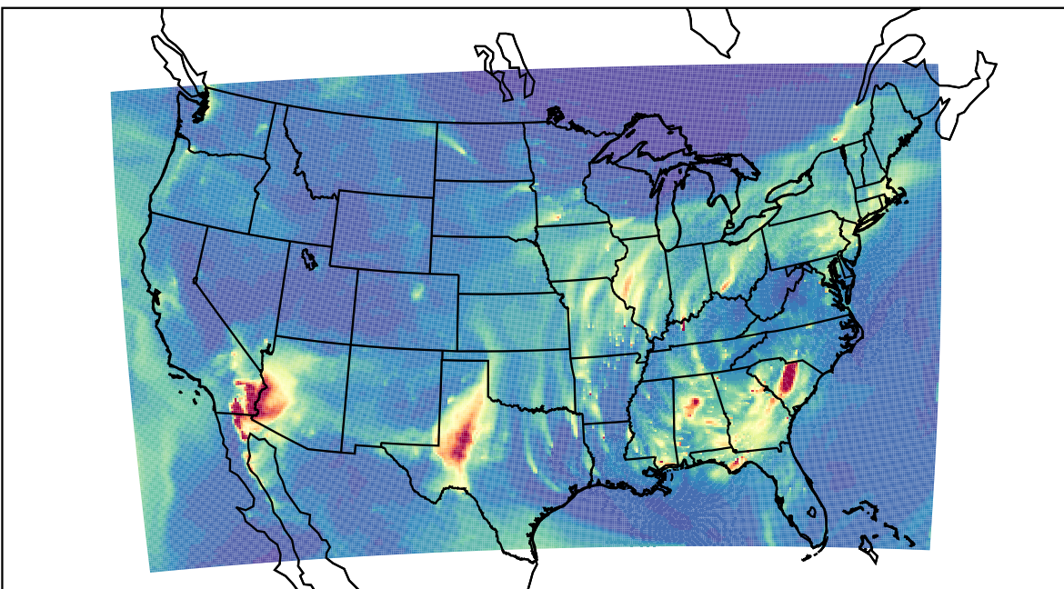
WRF 2023-03-21_08:00:00
