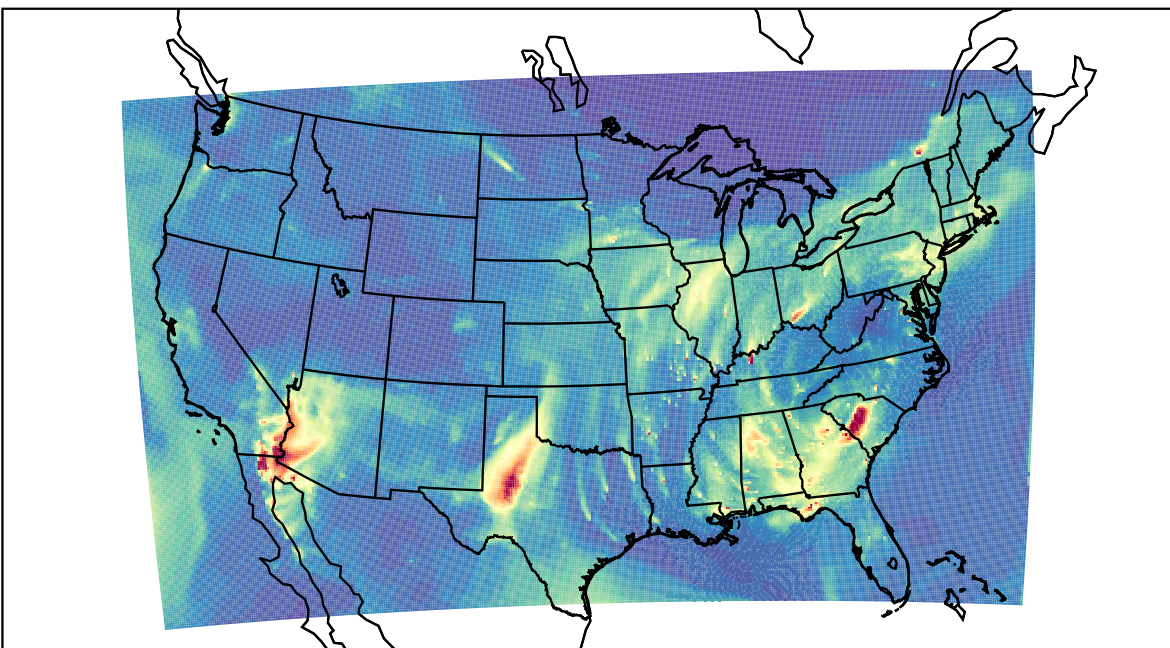
WRF 2023-03-21_11:00:00
