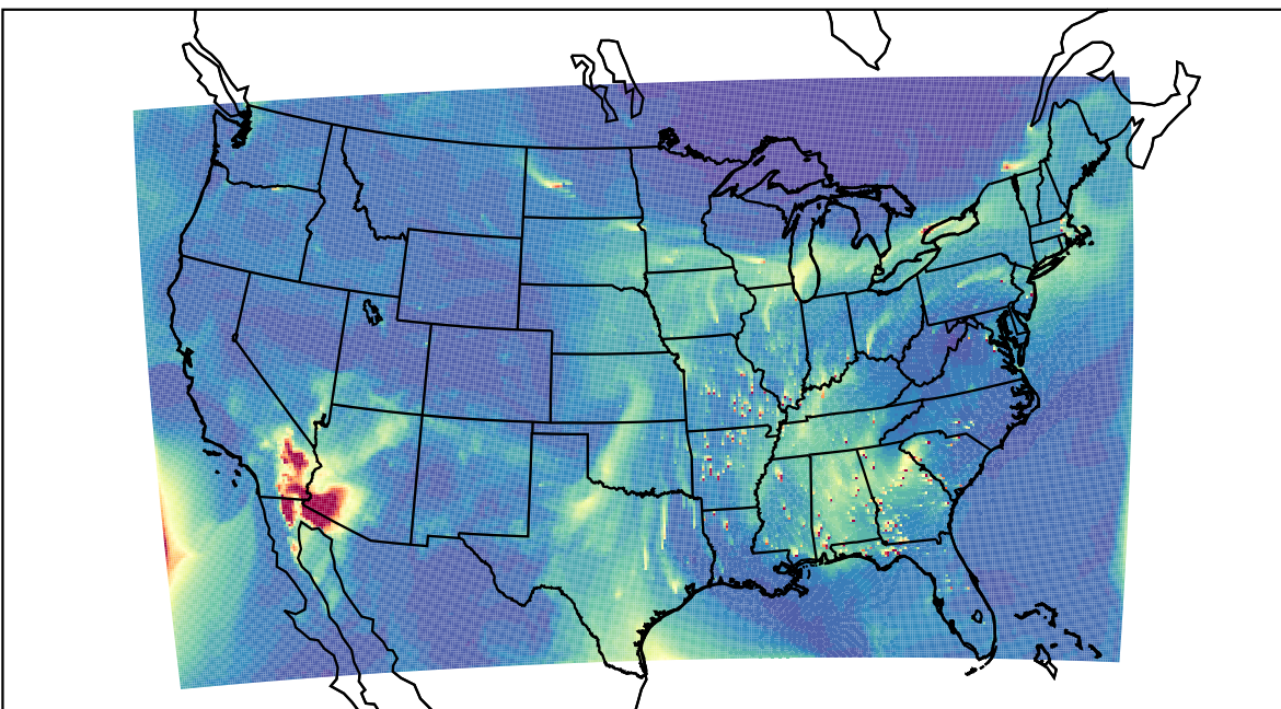
WRF 2023-03-21_18:00:00
