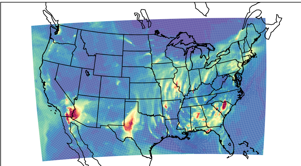
WRF 2023-03-21_06:00:00
