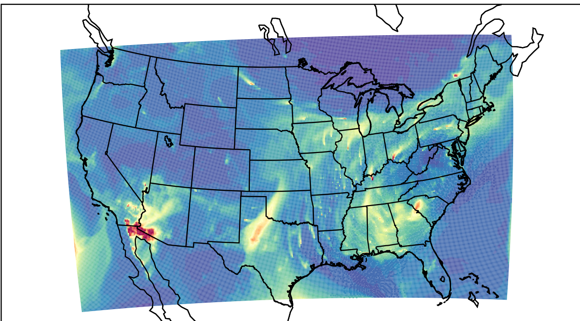
WRF 2023-03-21_15:00:00
