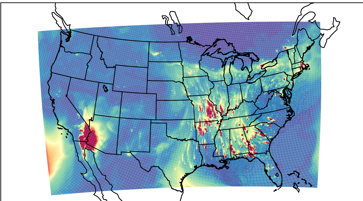
WRF 2023-03-21_23:00:00
