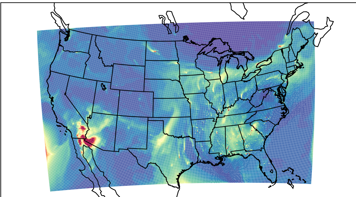
WRF 2023-03-21_17:00:00
