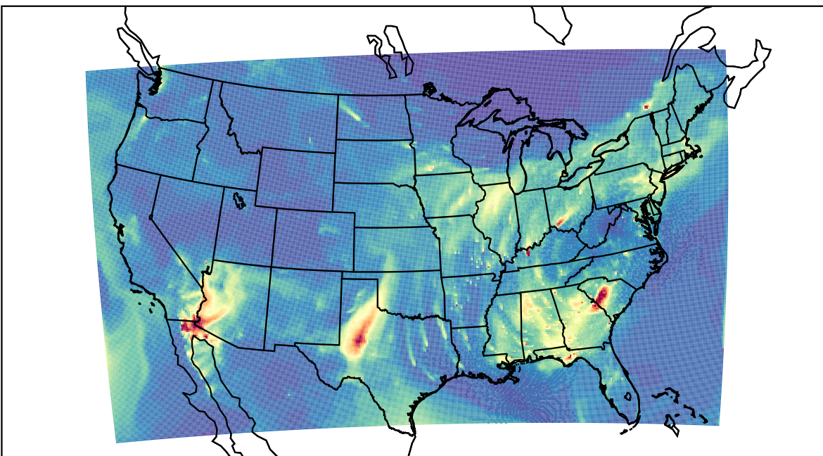
WRF 2023-03-21_12:00:00
