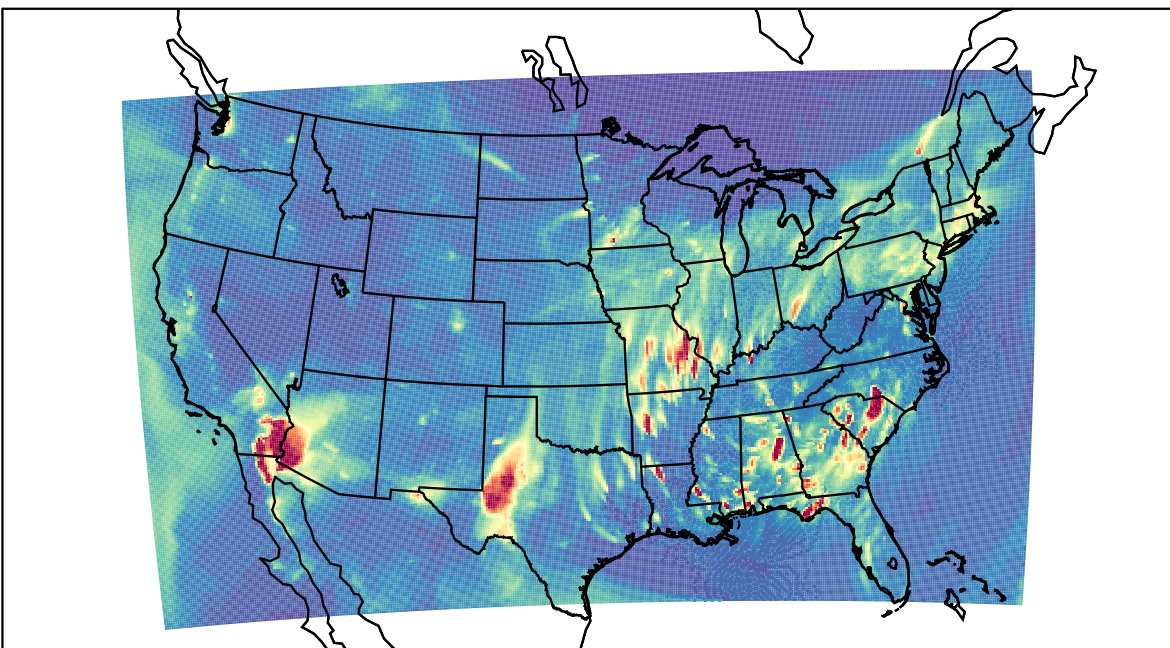
WRF 2023-03-21_04:00:00
