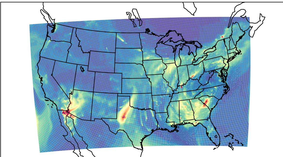
WRF 2023-03-21_13:00:00
