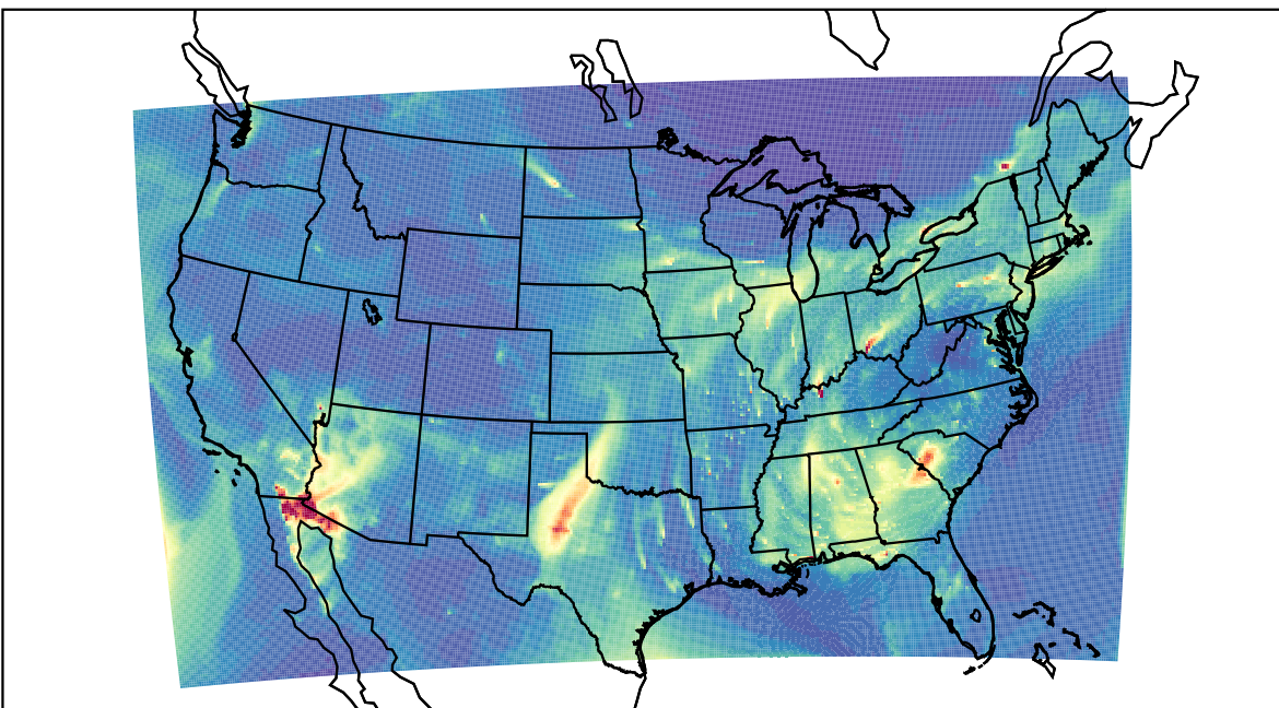
WRF 2023-03-21_14:00:00
