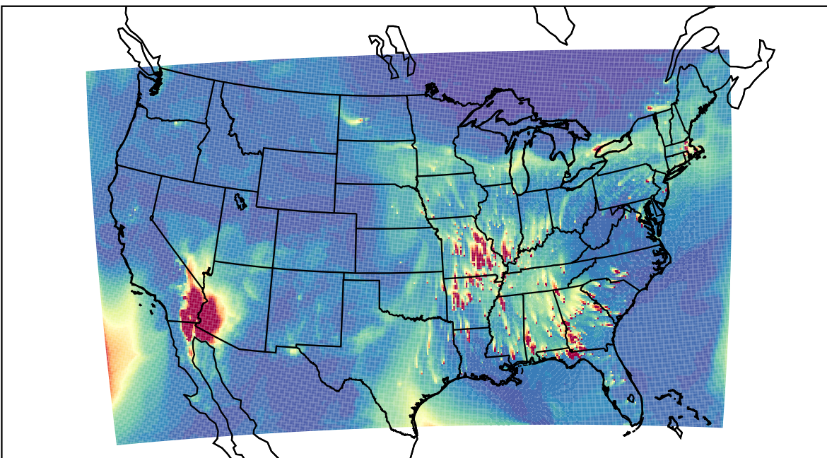
WRF 2023-03-21_22:00:00
