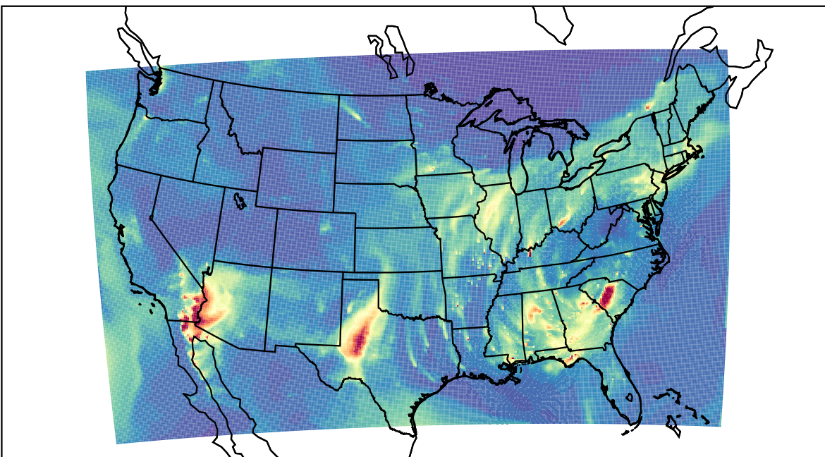
WRF 2023-03-21_10:00:00
