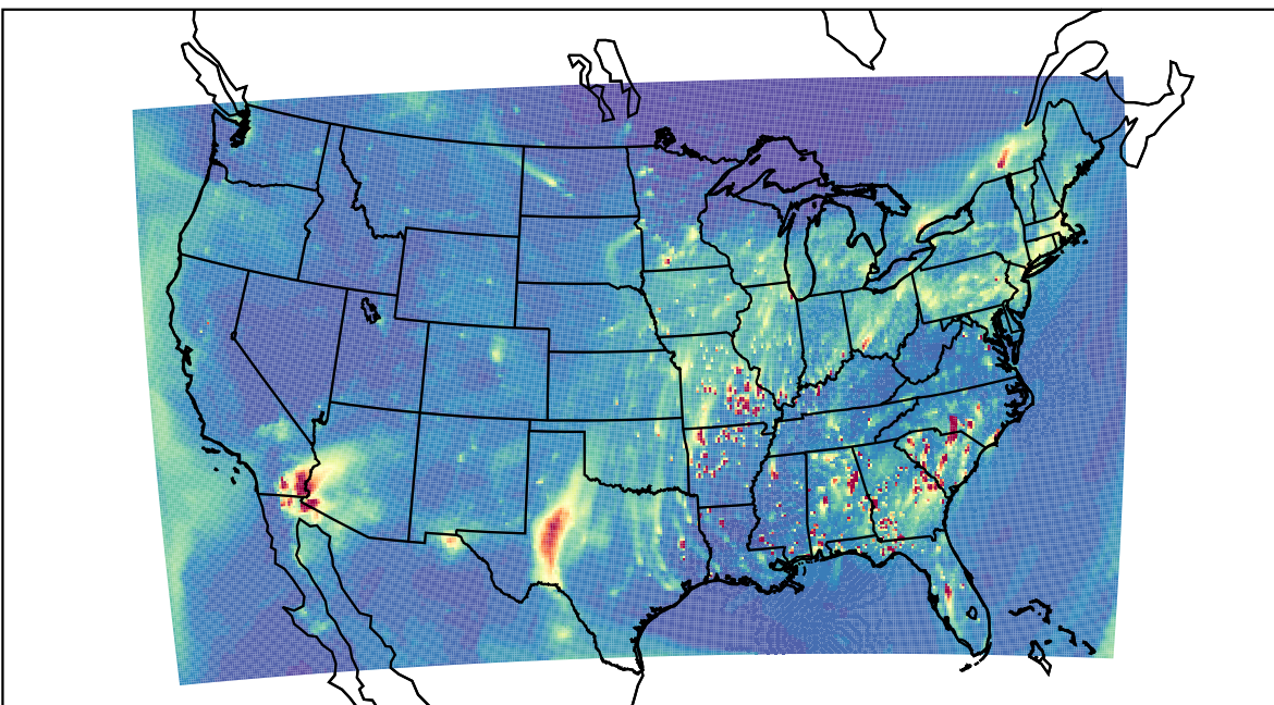
WRF 2023-03-21_01:00:00
