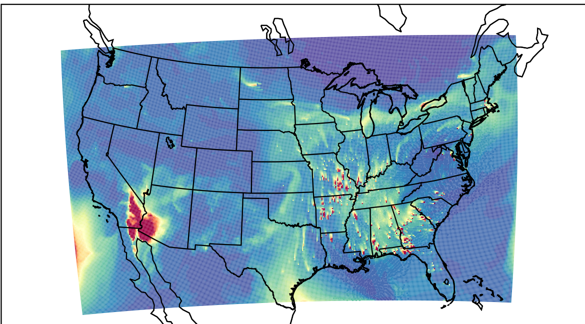
WRF 2023-03-21_20:00:00
