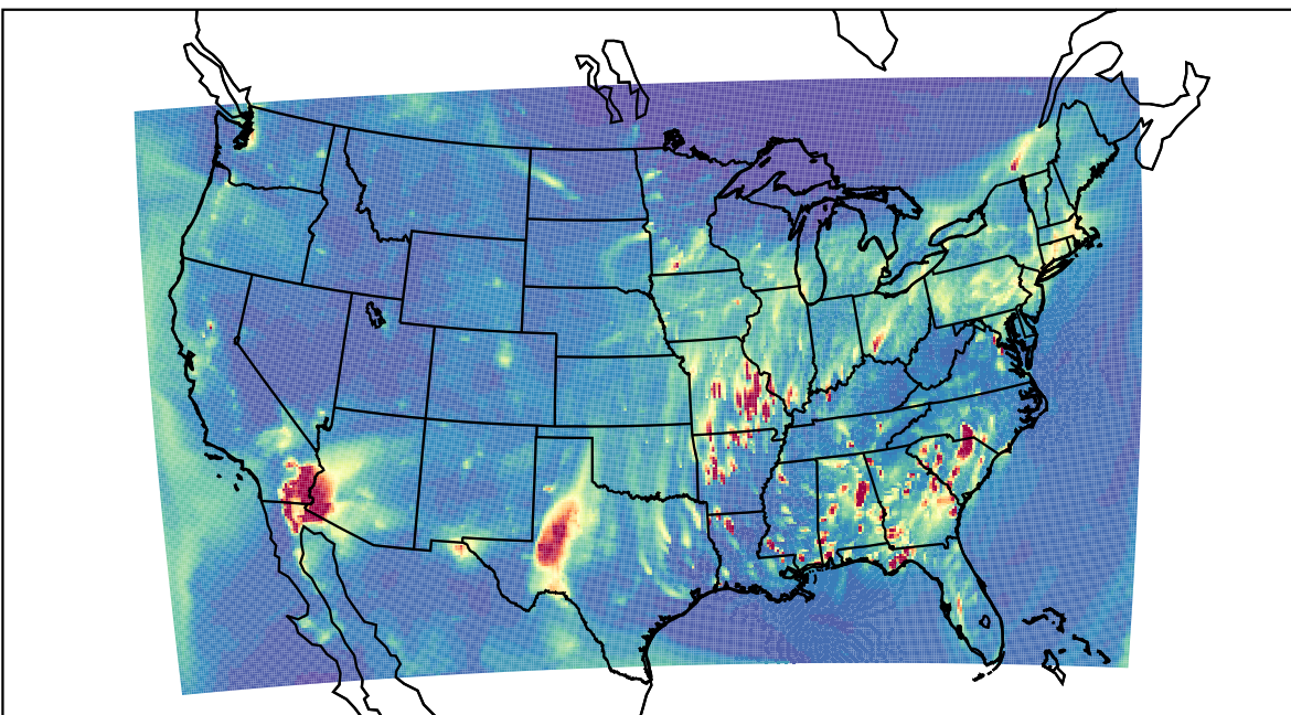
WRF 2023-03-21_03:00:00
