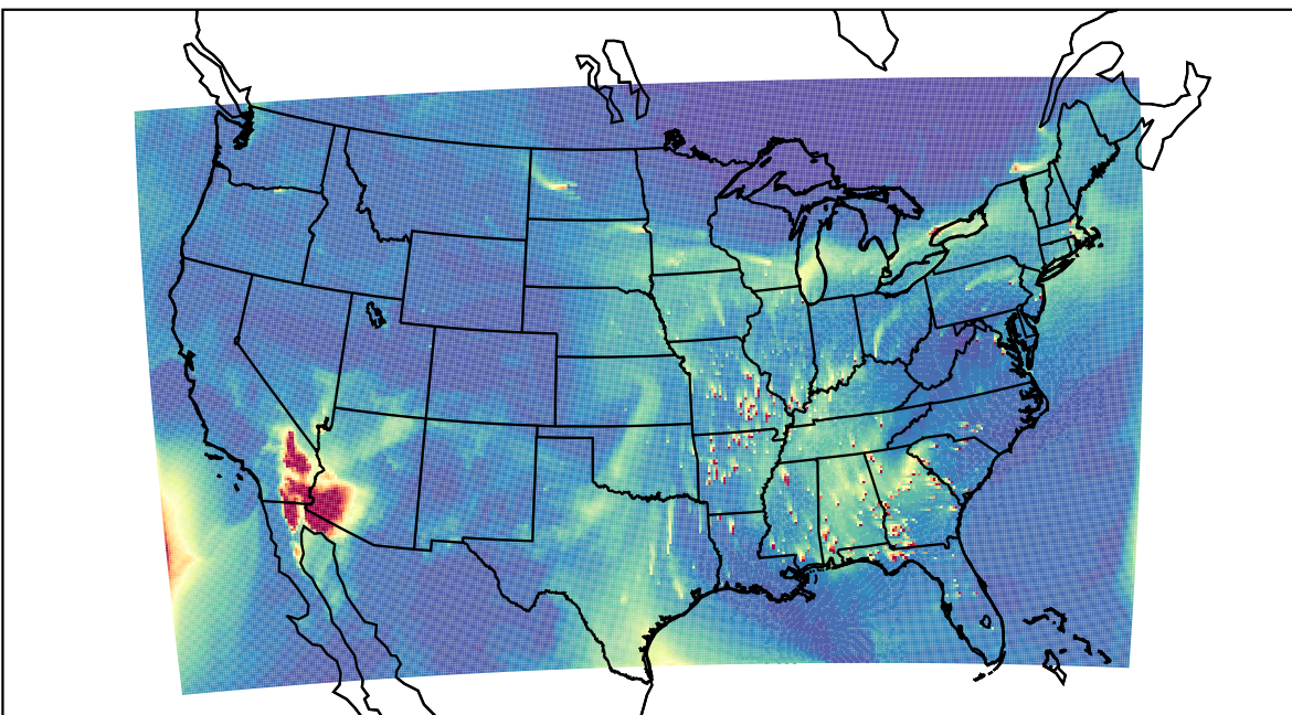
WRF 2023-03-21_19:00:00
