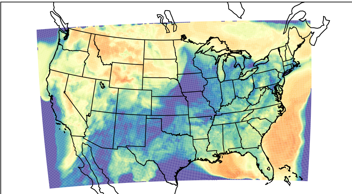
WRF (2023-03-22_10:00:00)
