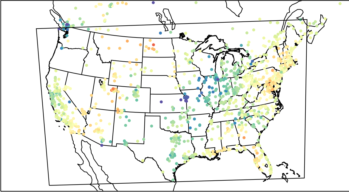
AirNOW (2023-03-22_20:00:00)
