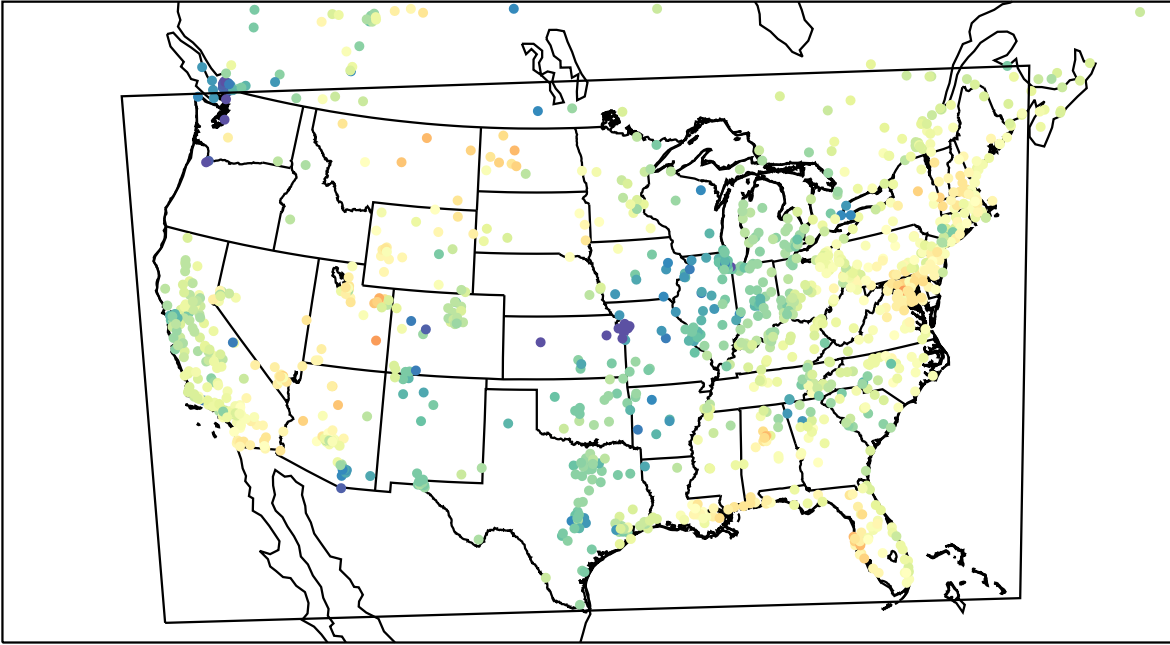
AirNOW (2023-03-22_18:00:00)
