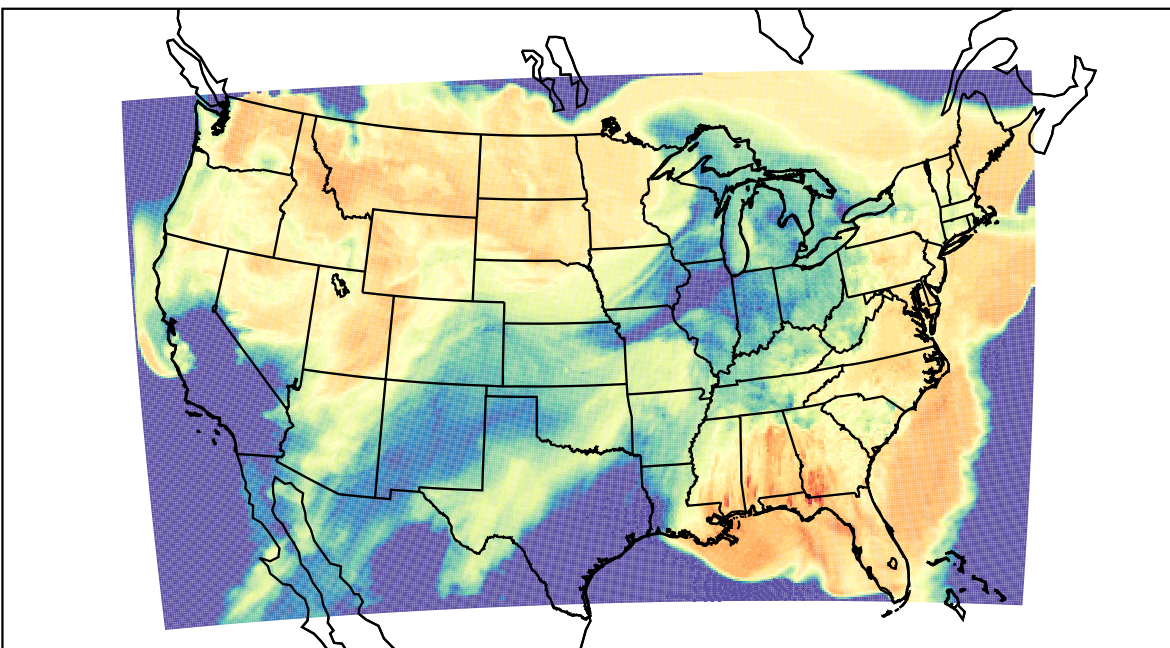
WRF (2023-03-22_20:00:00)
