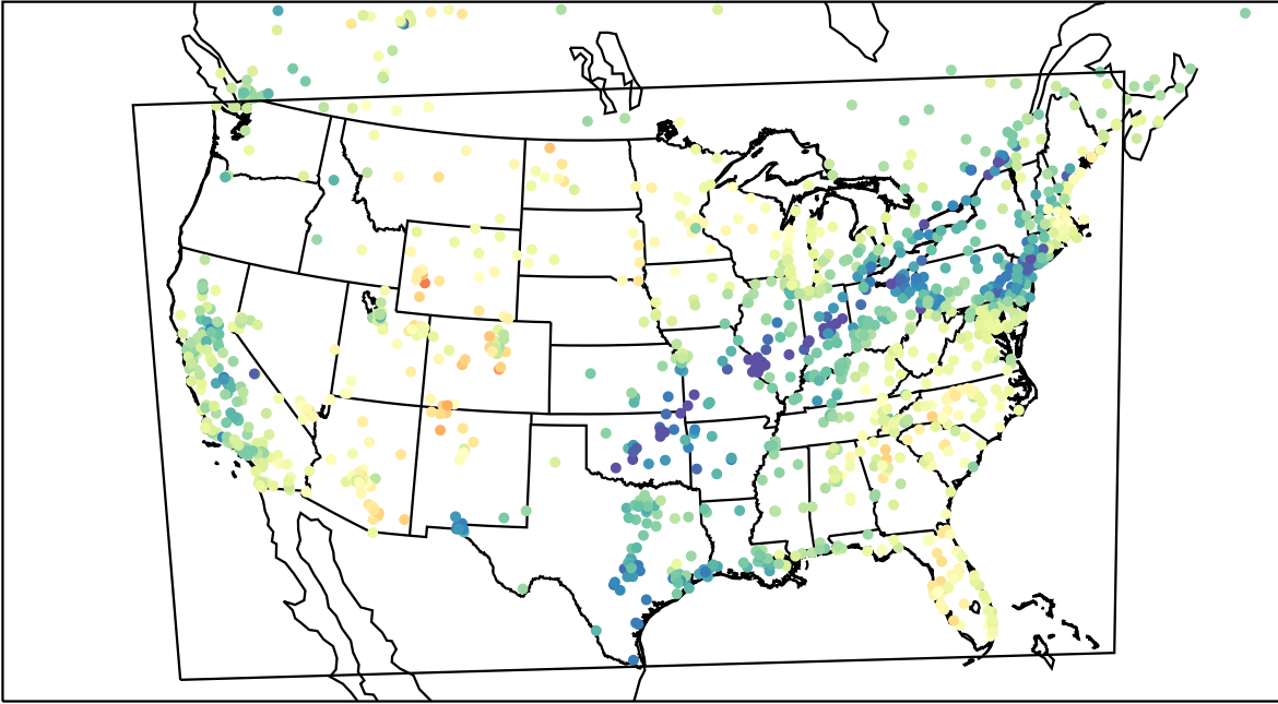
AirNOW (2023-03-23_18:00:00)
