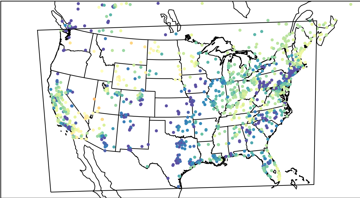
AirNOW (2023-03-22_13:00:00)
