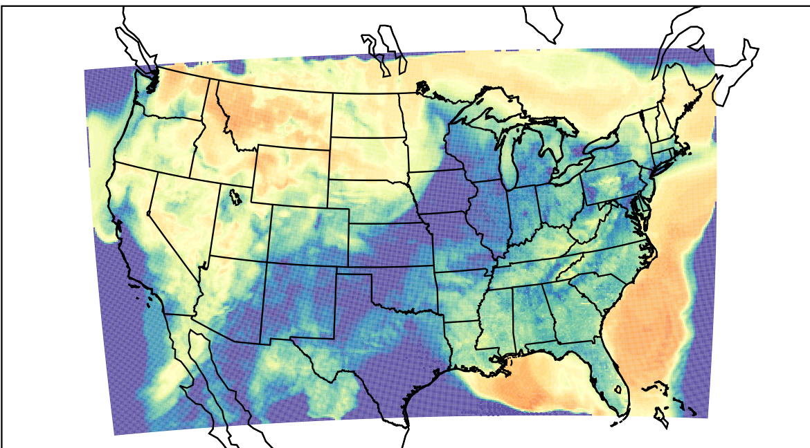
WRF (2023-03-22_13:00:00)
