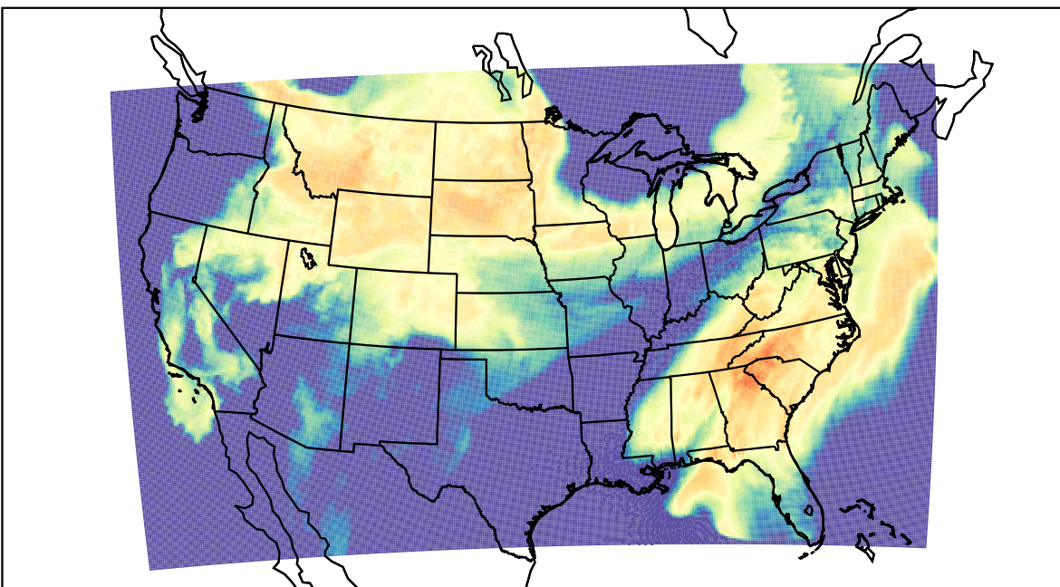
WRF (2023-03-23_18:00:00)
