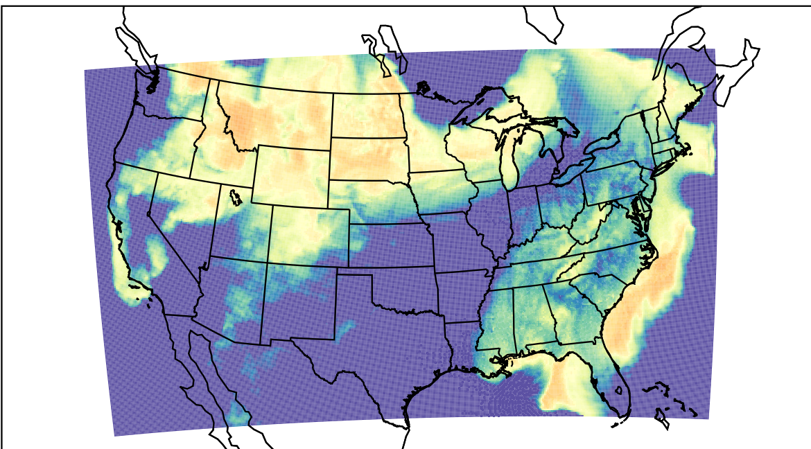
WRF (2023-03-23_10:00:00)
