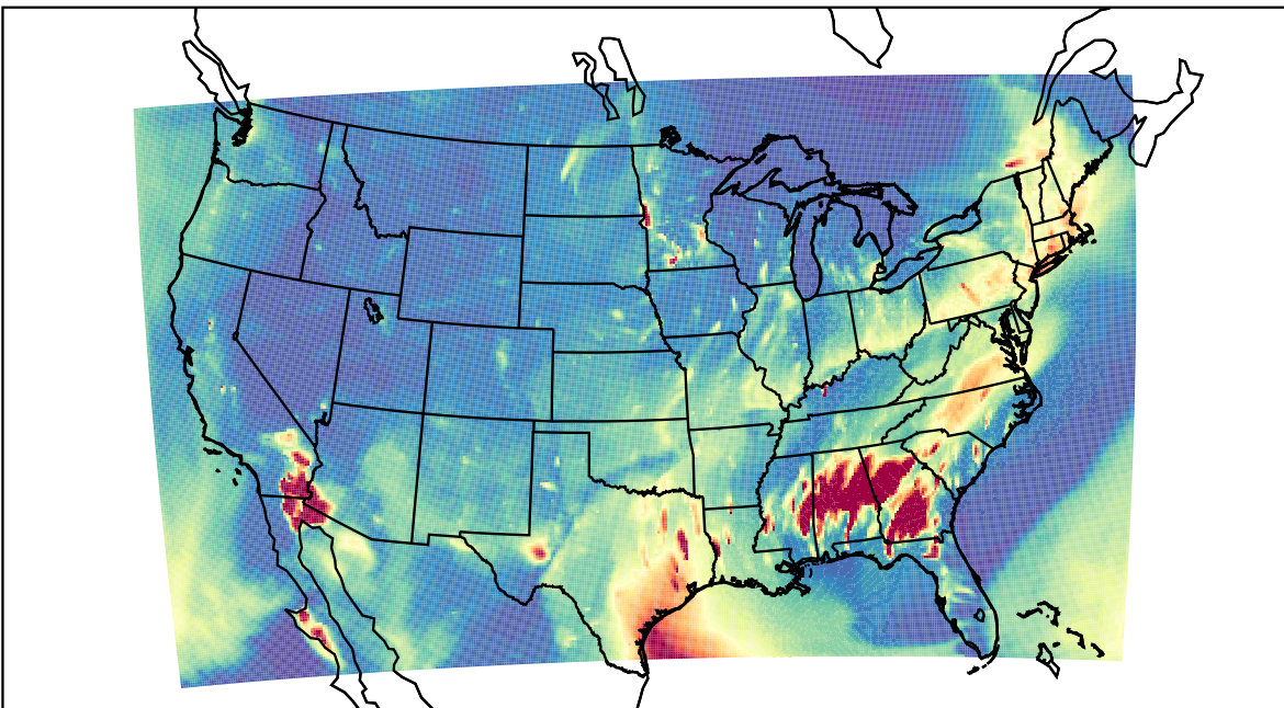
WRF 2023-03-24_03:00:00
