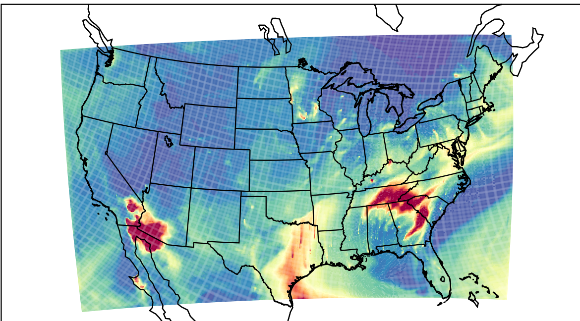
WRF 2023-03-24_10:00:00
