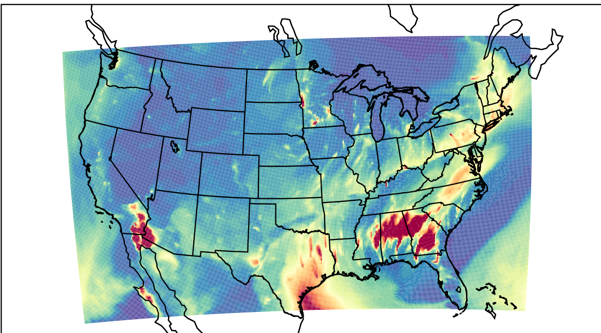
WRF 2023-03-24_04:00:00
