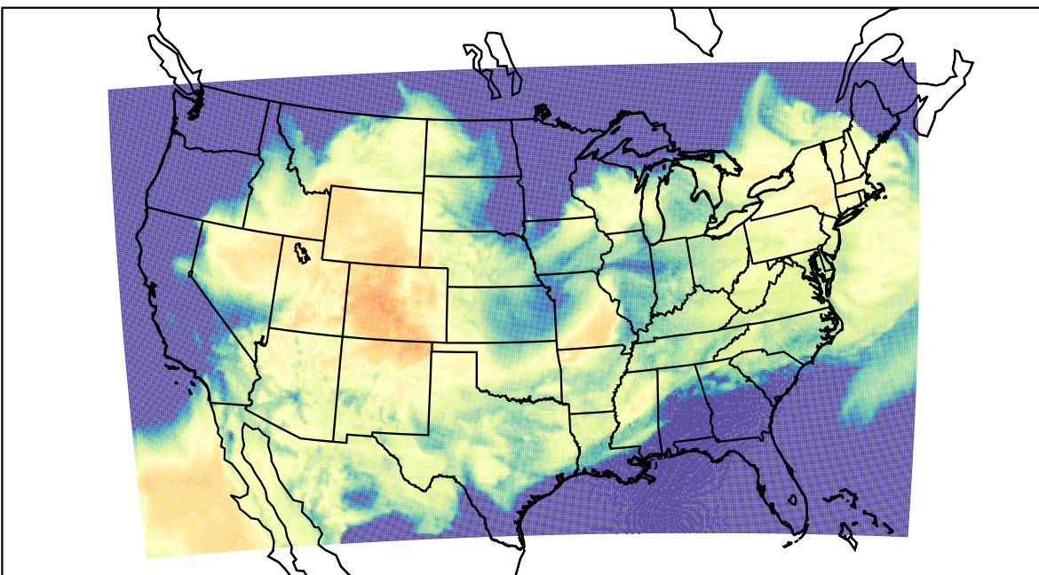
WRF (2023-03-26_16:00:00)
