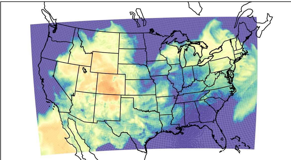
WRF (2023-03-26_13:00:00)
