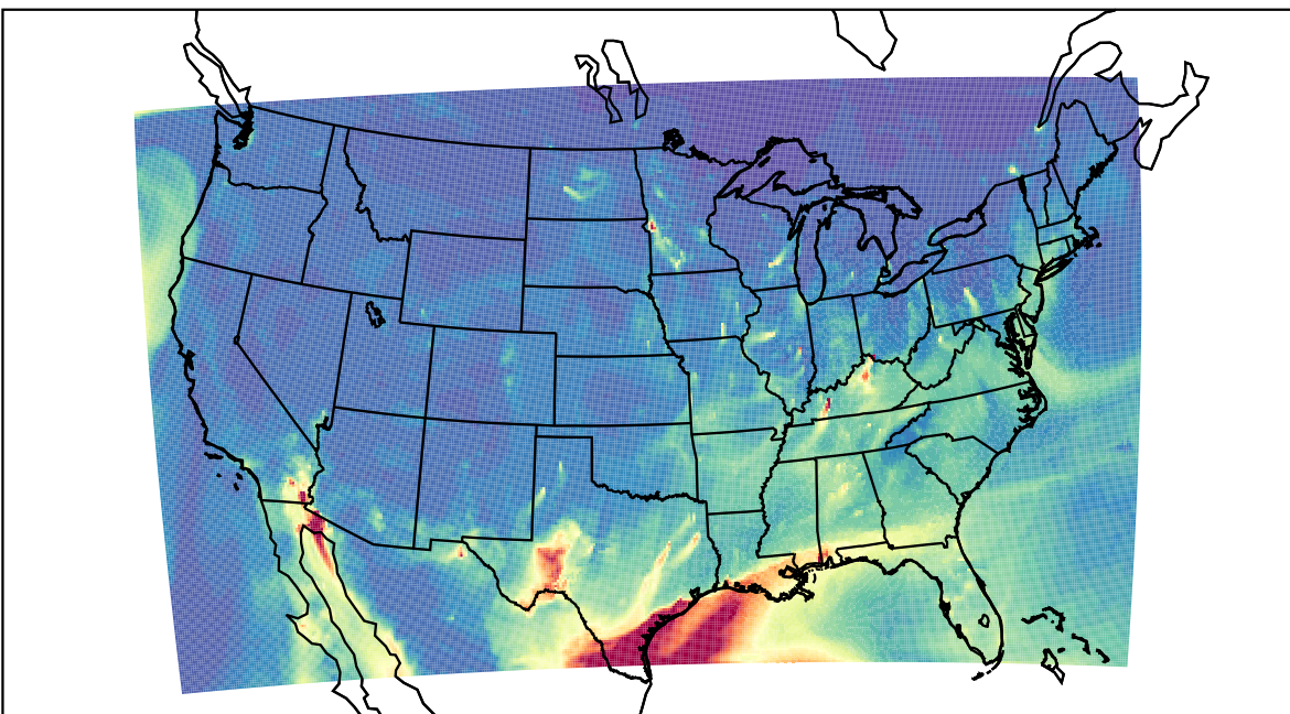
WRF 2023-03-28_13:00:00
