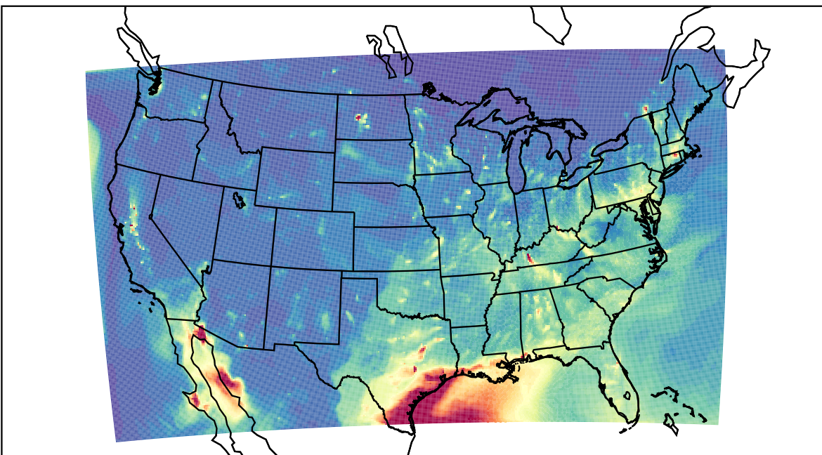
WRF 2023-03-28_03:00:00
