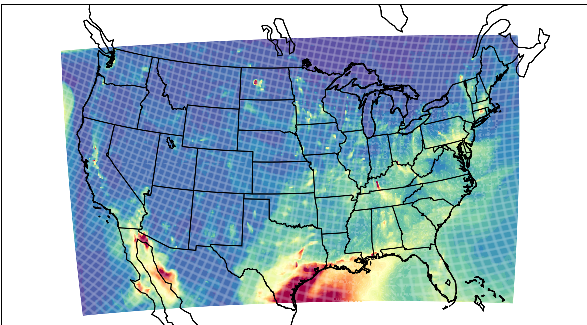
WRF 2023-03-28_04:00:00
