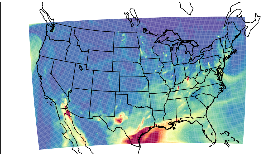
WRF 2023-03-28_10:00:00
