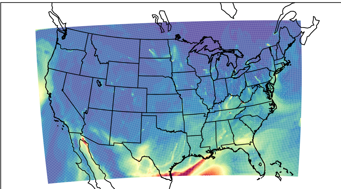
WRF 2023-03-28_19:00:00
