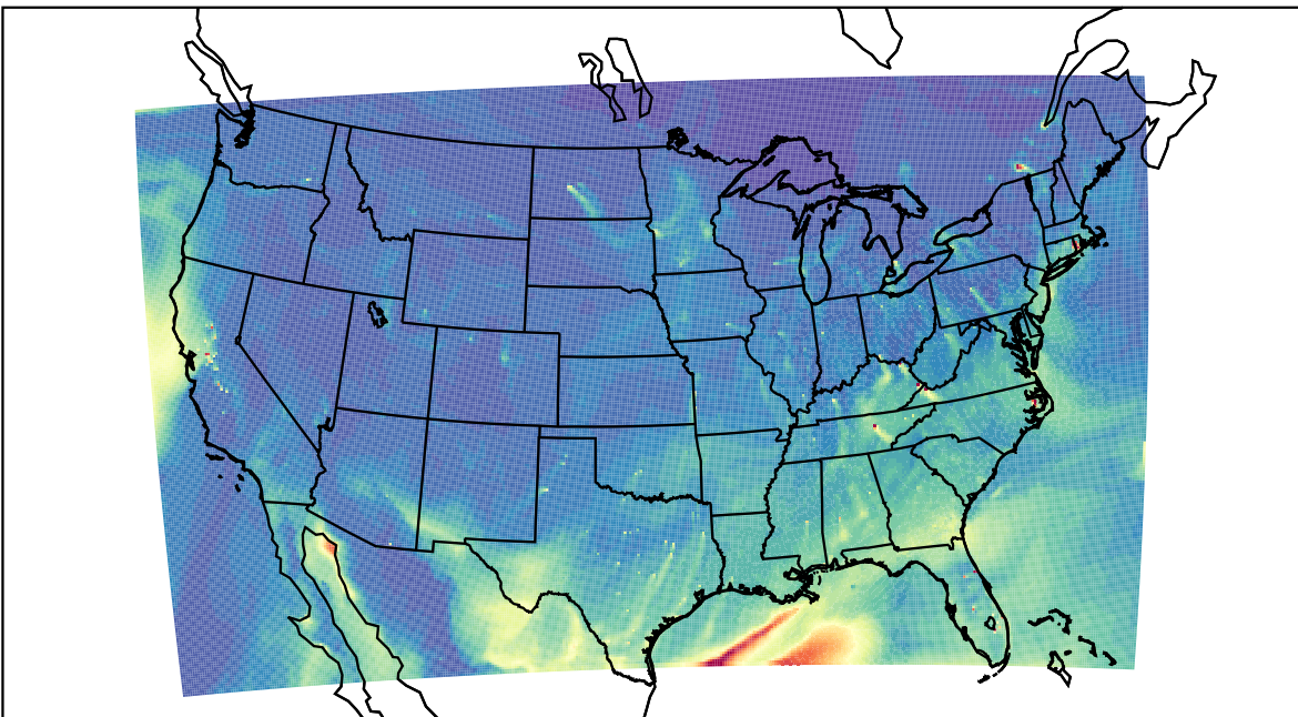
WRF 2023-03-28_22:00:00
