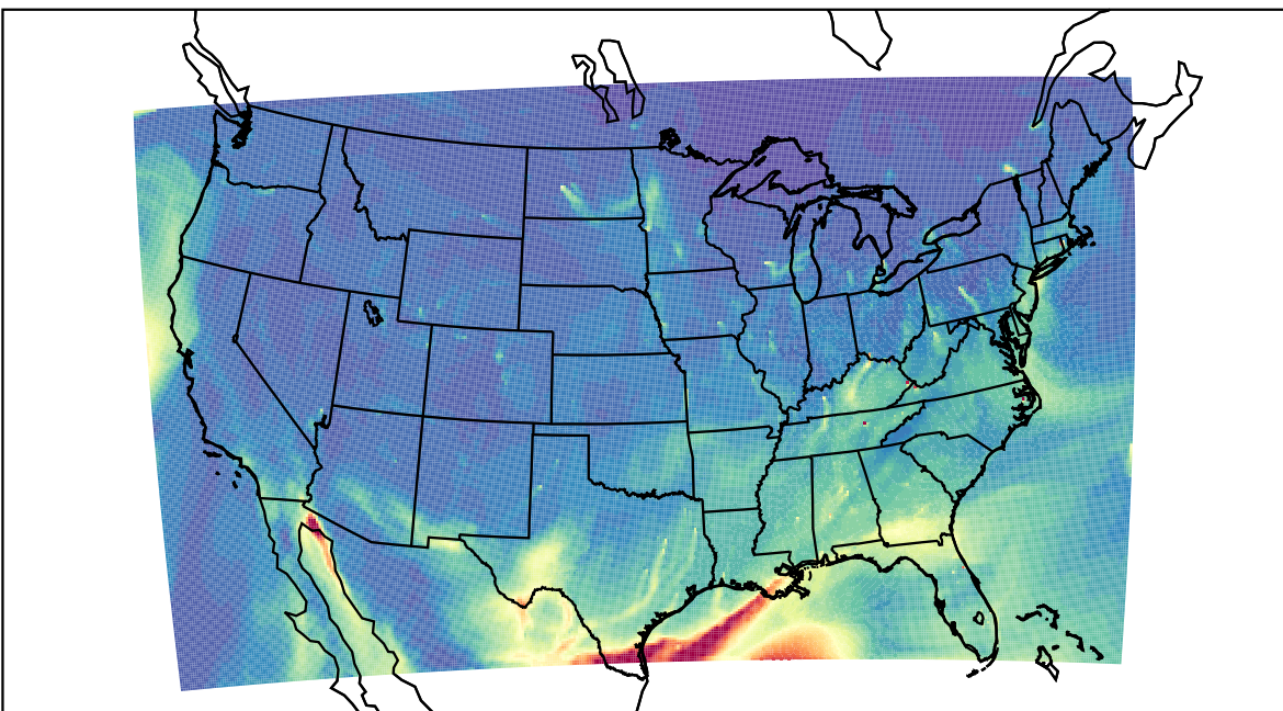
WRF 2023-03-28_18:00:00
