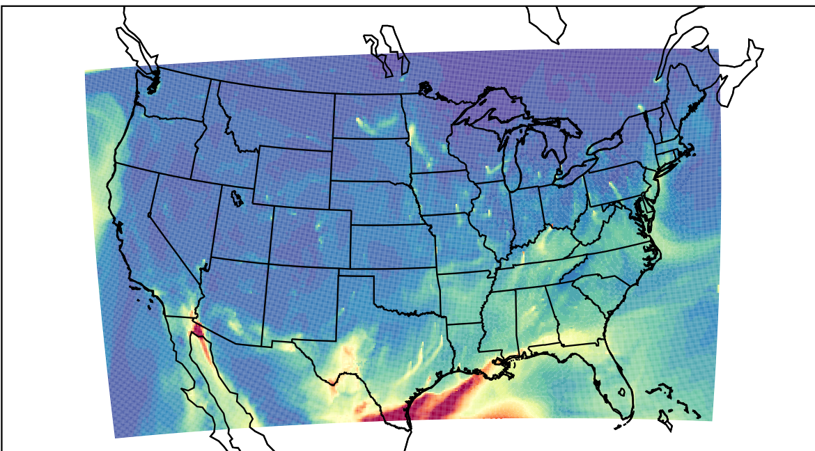
WRF 2023-03-28_16:00:00
