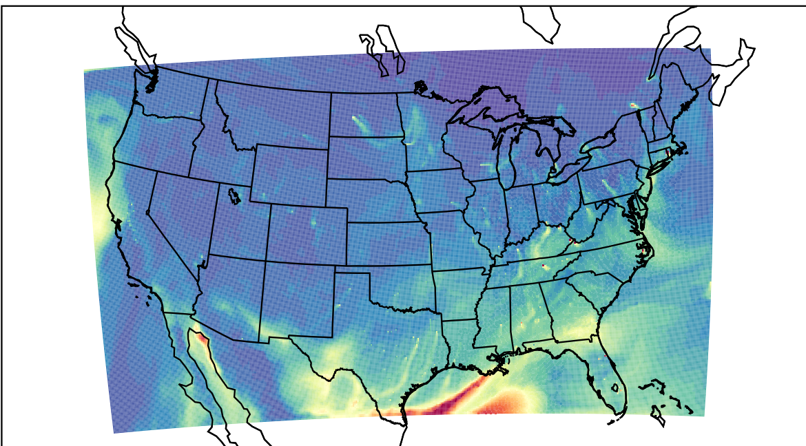
WRF 2023-03-28_20:00:00
