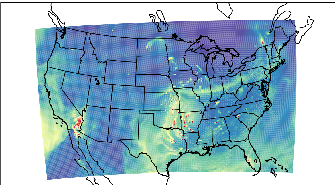
WRF 2023-03-29_23:00:00
