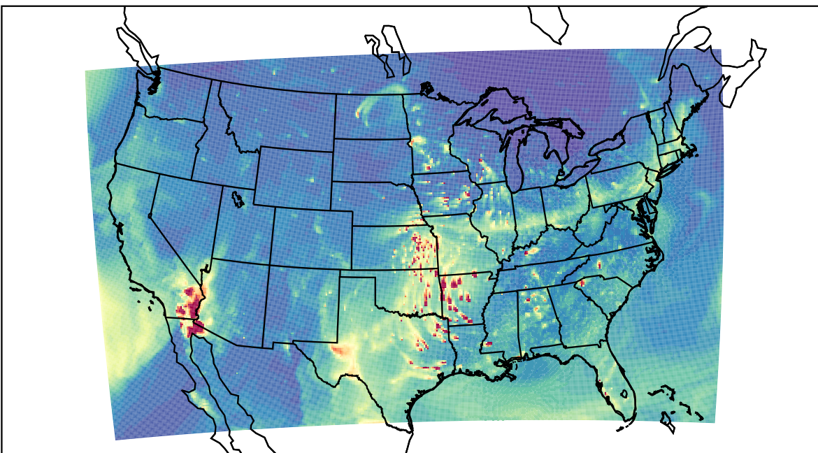
WRF 2023-03-30_01:00:00
