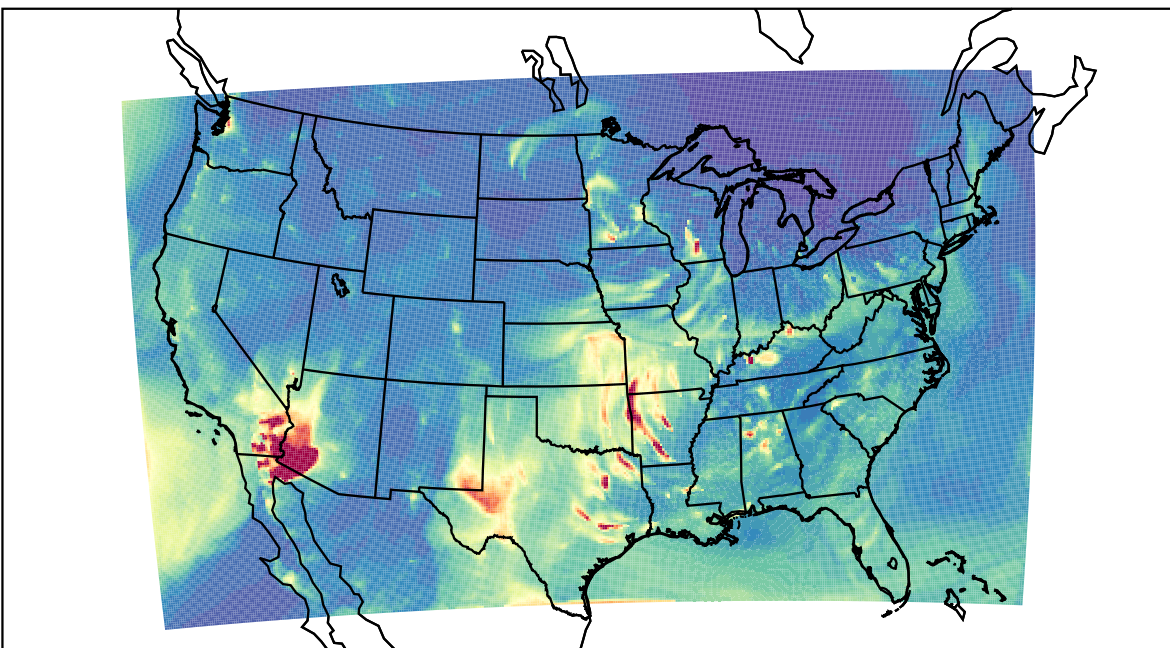
WRF 2023-03-30_05:00:00
