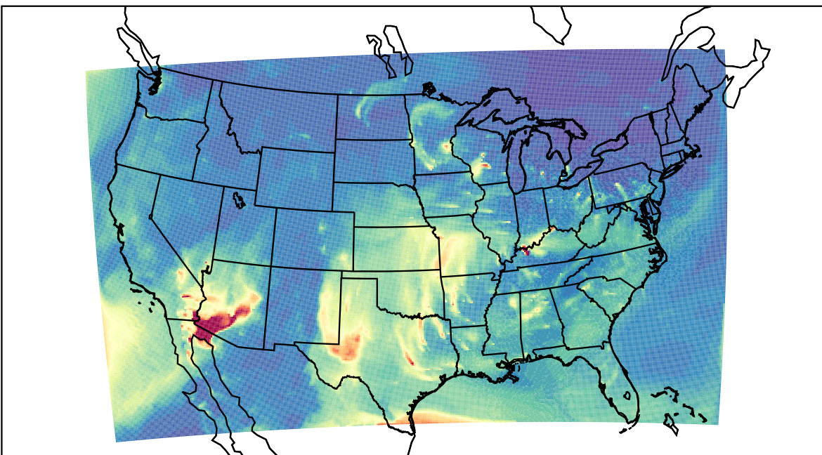
WRF 2023-03-30_11:00:00
