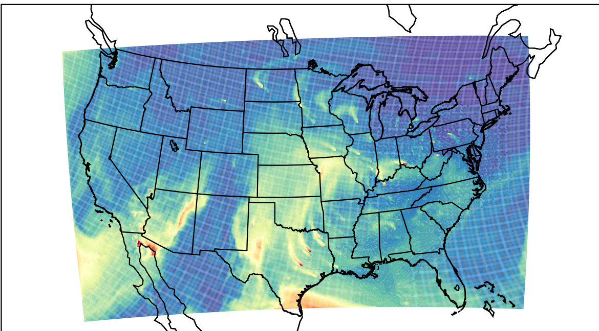
WRF 2023-03-30_16:00:00
