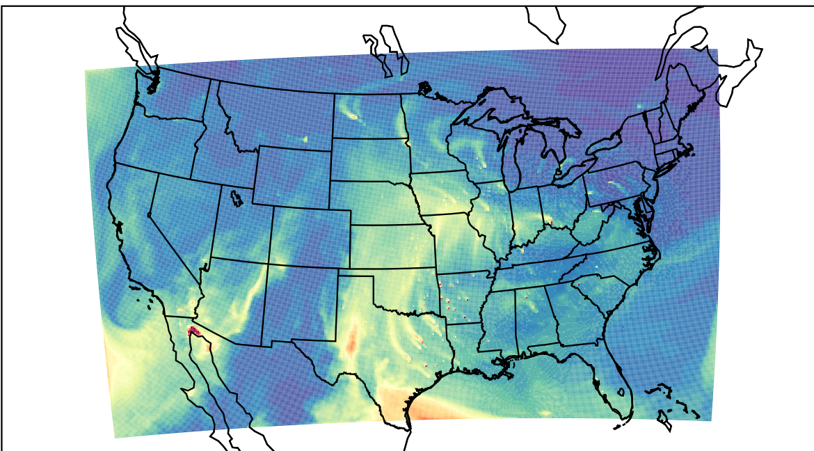
WRF 2023-03-30_18:00:00
