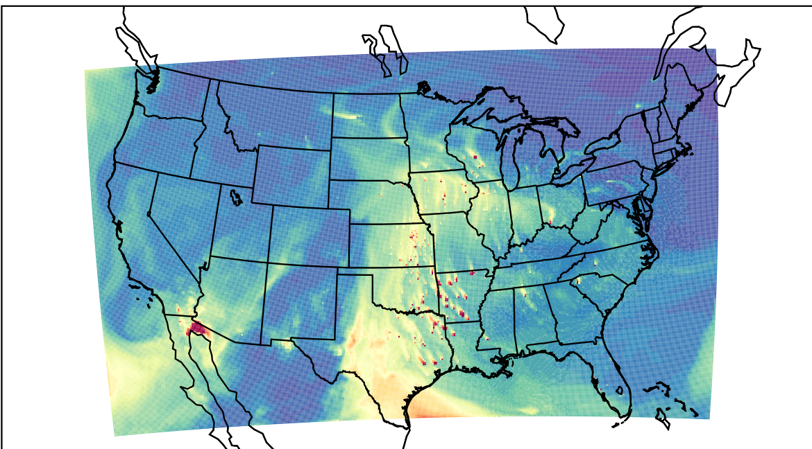
WRF 2023-03-30_22:00:00
