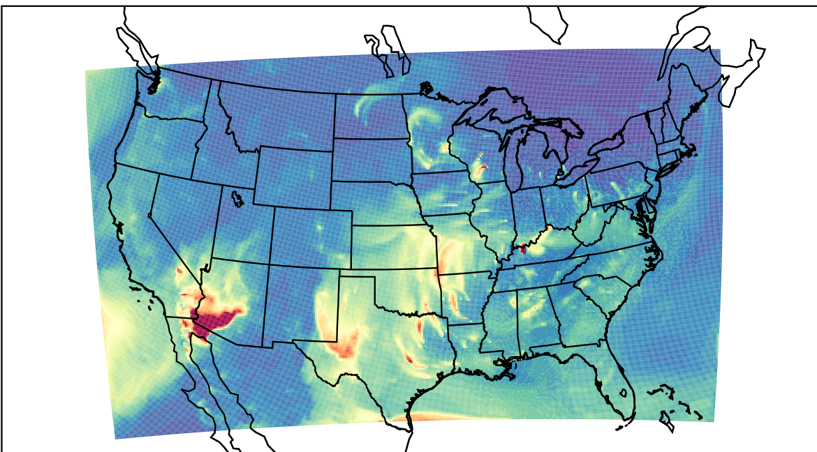
WRF 2023-03-30_09:00:00
