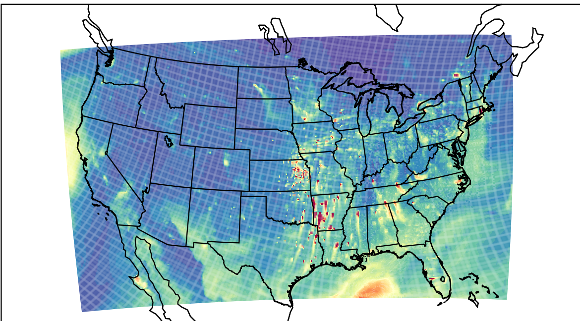
WRF 2023-03-29_01:00:00
