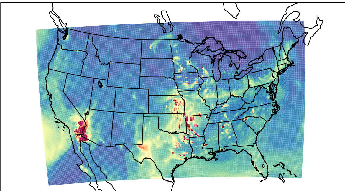
WRF 2023-03-30_02:00:00
