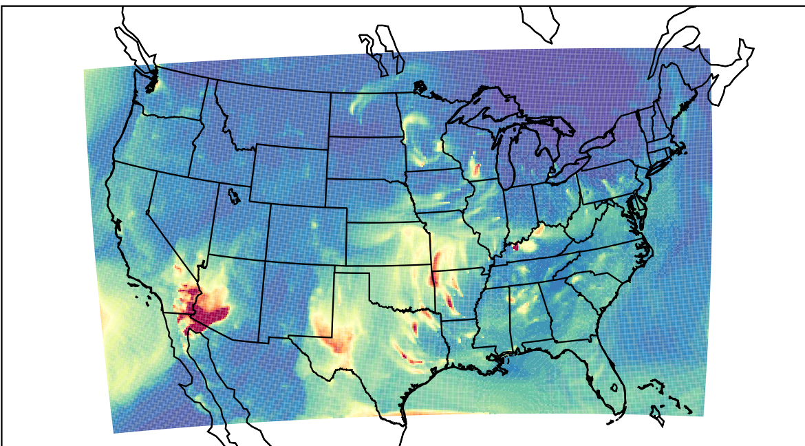
WRF 2023-03-30_07:00:00
