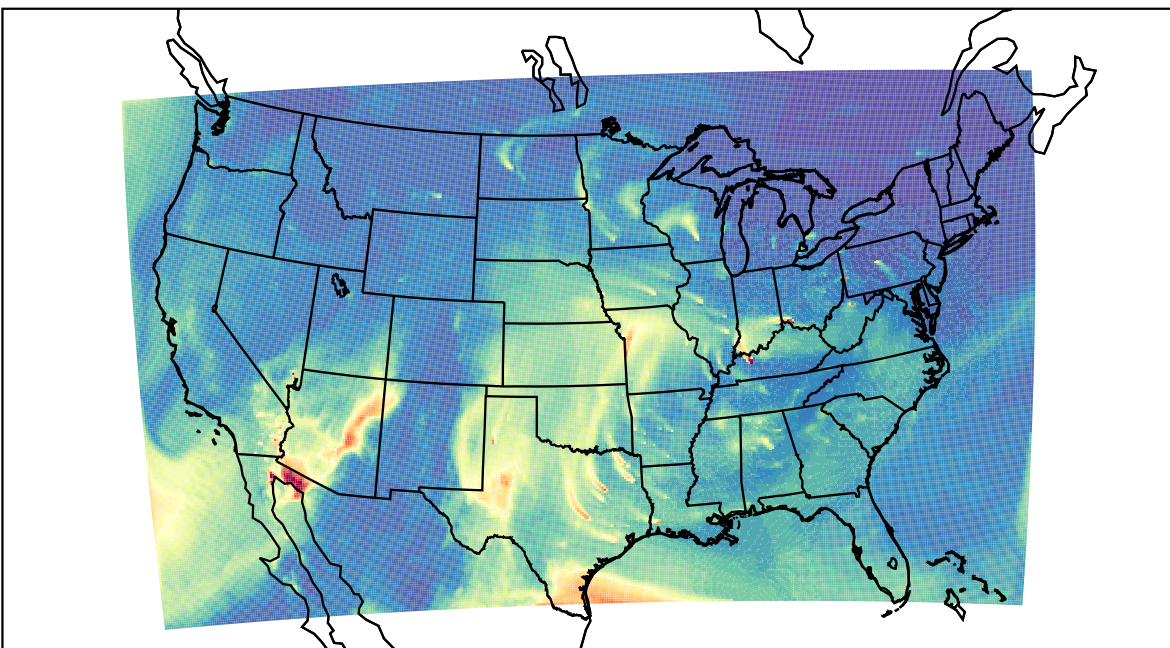
WRF 2023-03-30_15:00:00
