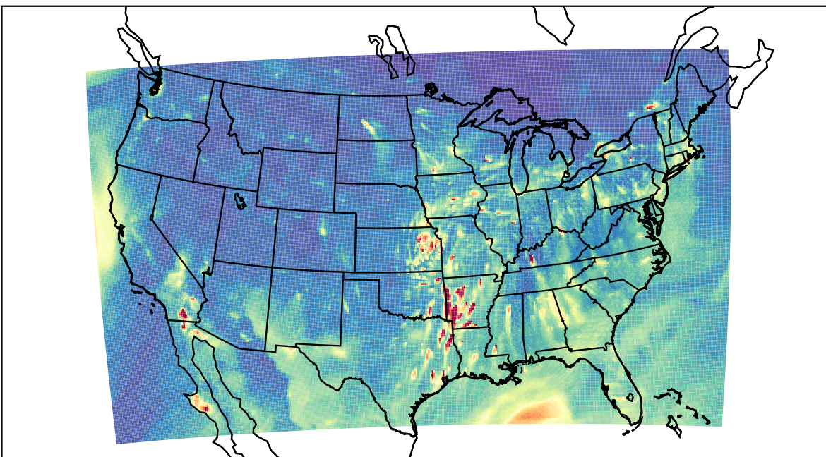
WRF 2023-03-29_03:00:00
