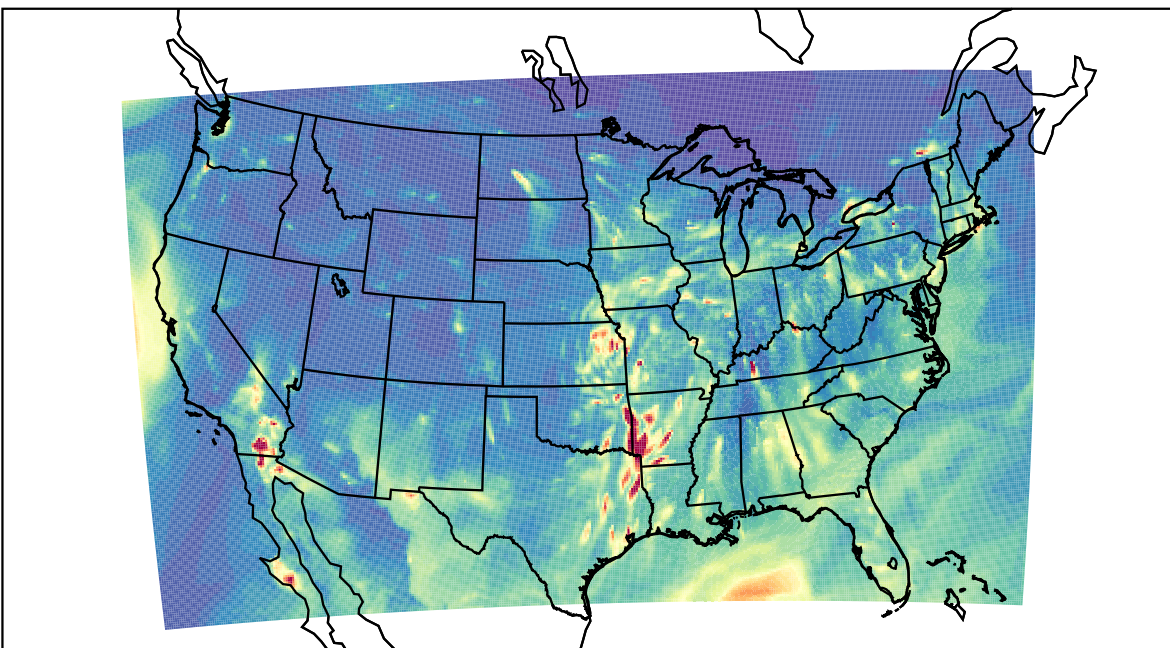
WRF 2023-03-29_04:00:00
