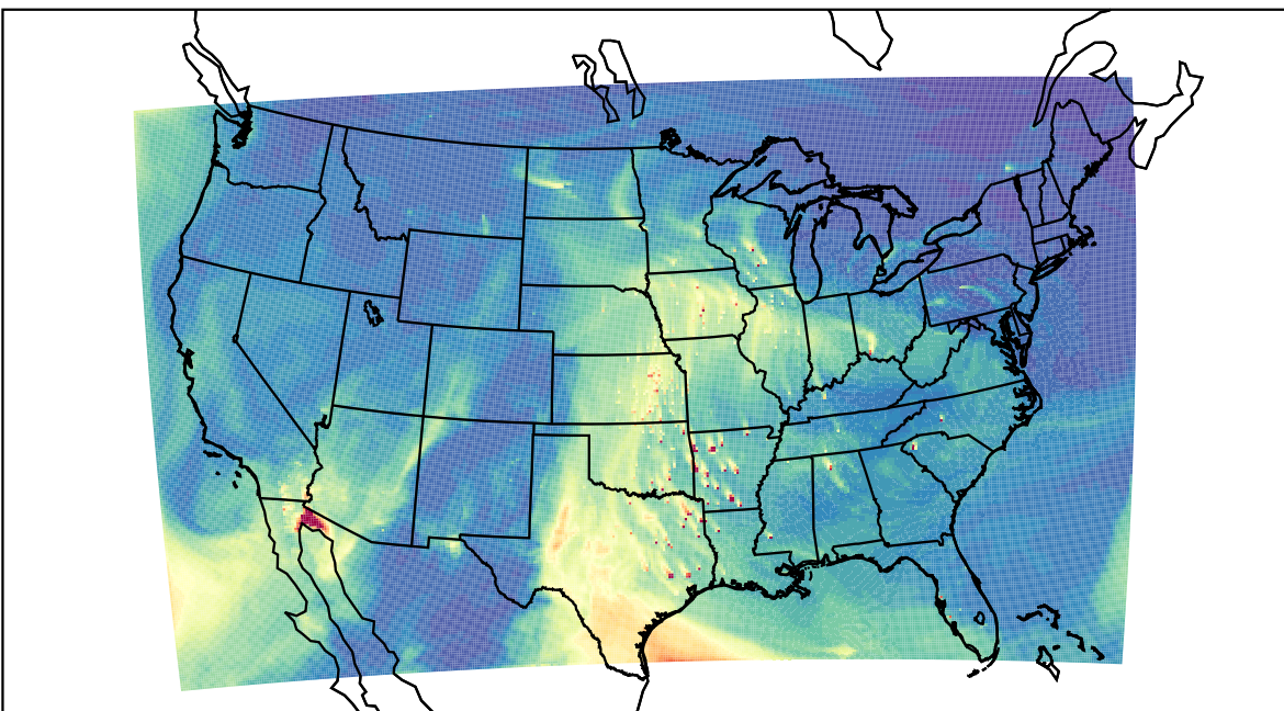
WRF 2023-03-30_21:00:00
