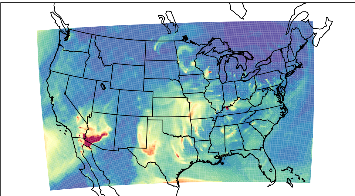
WRF 2023-03-30_10:00:00
