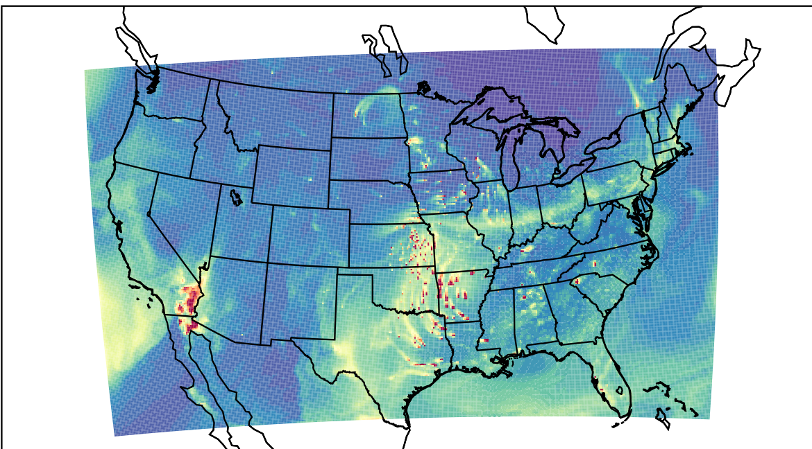
WRF 2023-03-30_00:00:00
