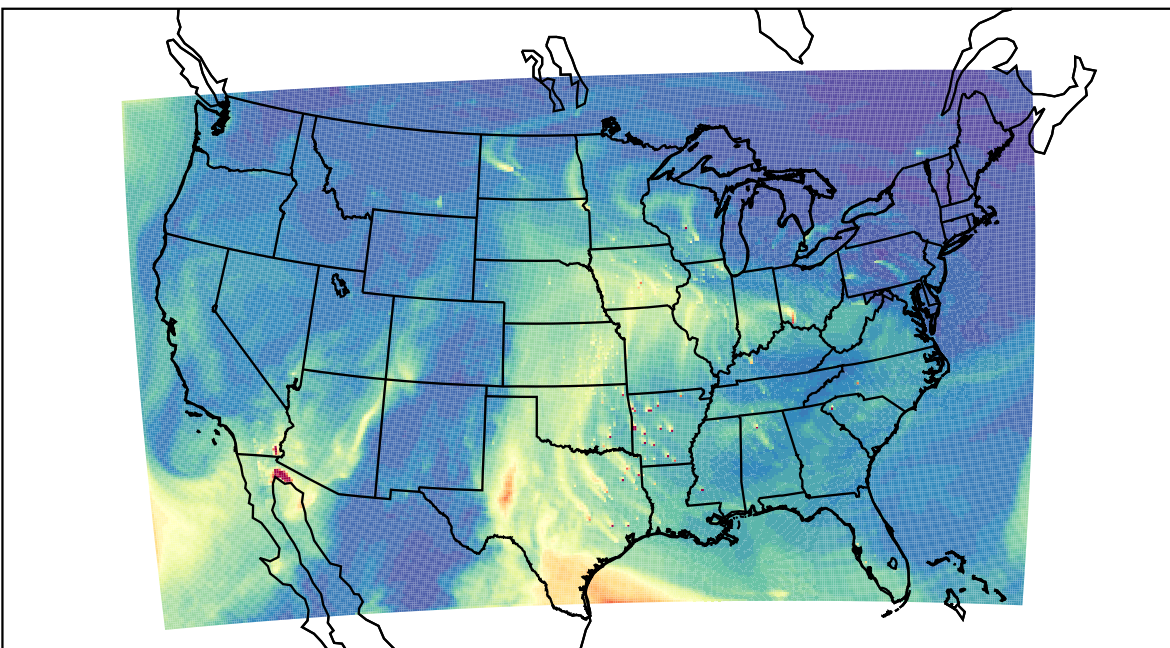
WRF 2023-03-30_19:00:00
