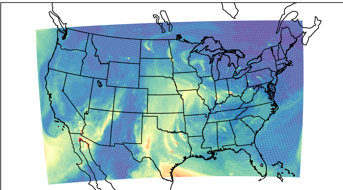
WRF 2023-03-30_17:00:00
