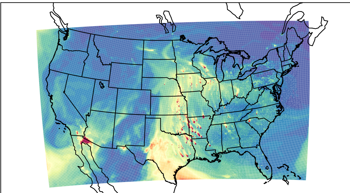
WRF 2023-03-30_23:00:00
