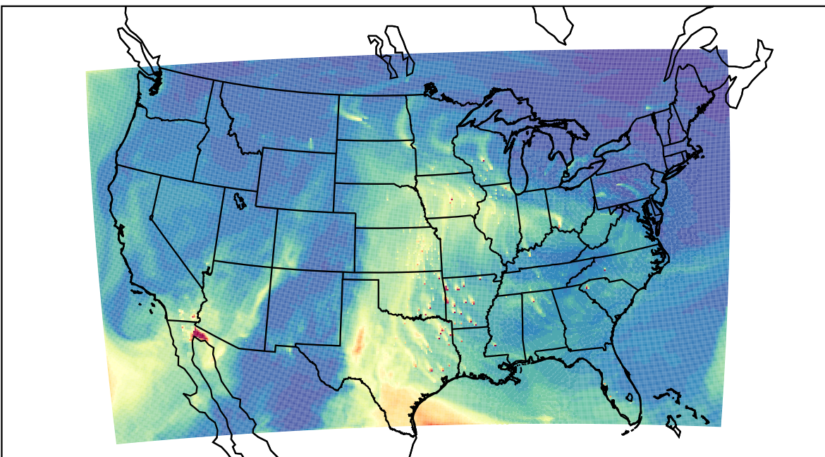
WRF 2023-03-30_20:00:00
