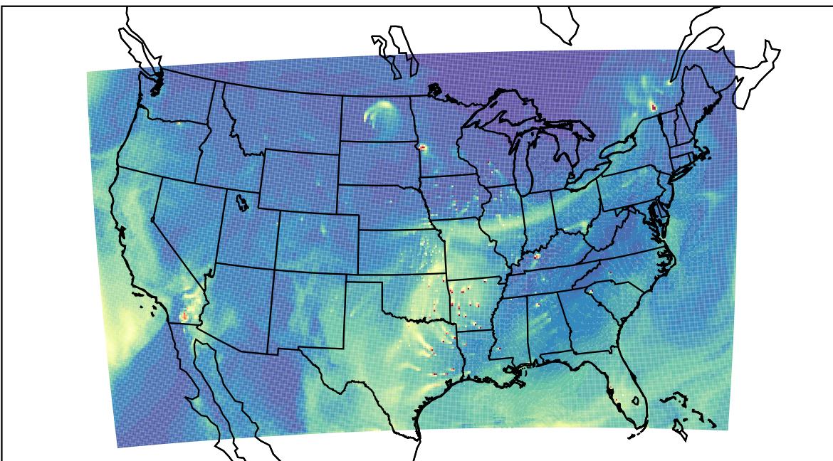
WRF 2023-03-29_20:00:00
