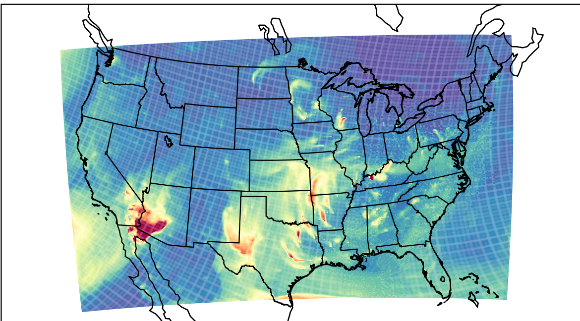
WRF 2023-03-30_08:00:00
