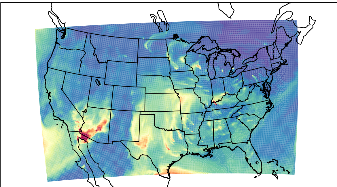
WRF 2023-03-30_13:00:00
