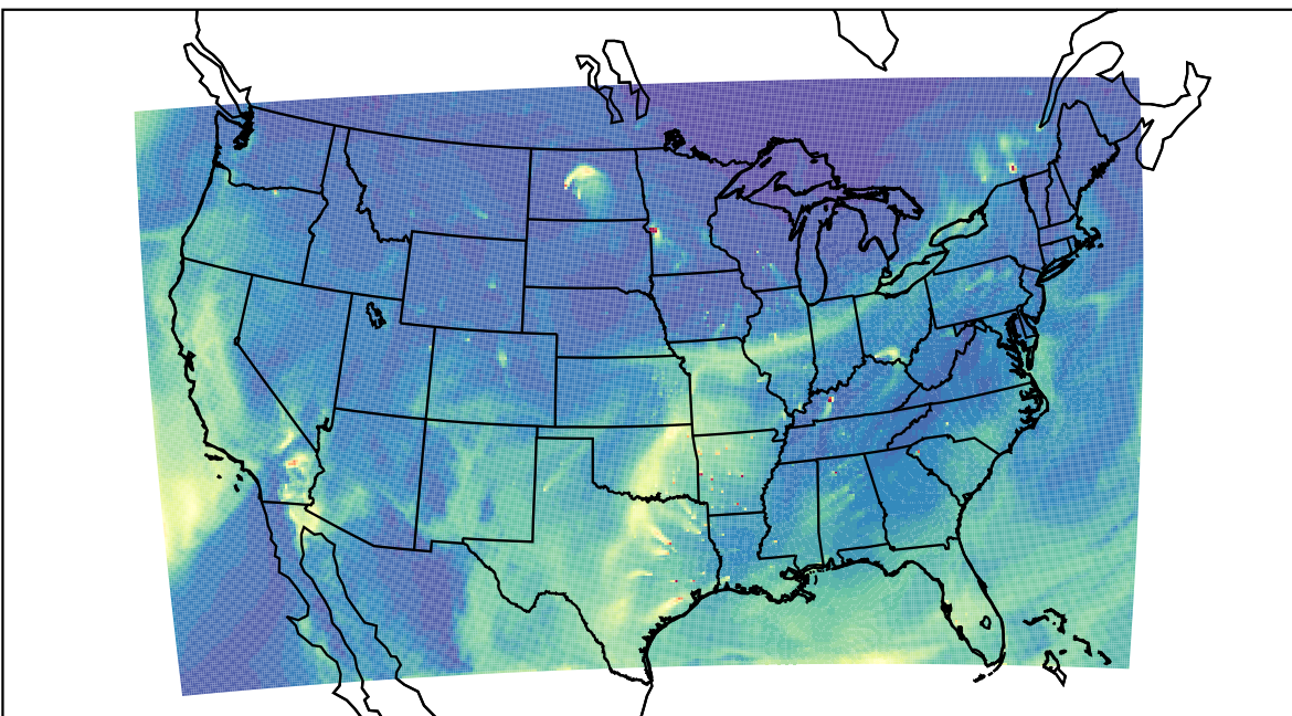
WRF 2023-03-29_18:00:00
