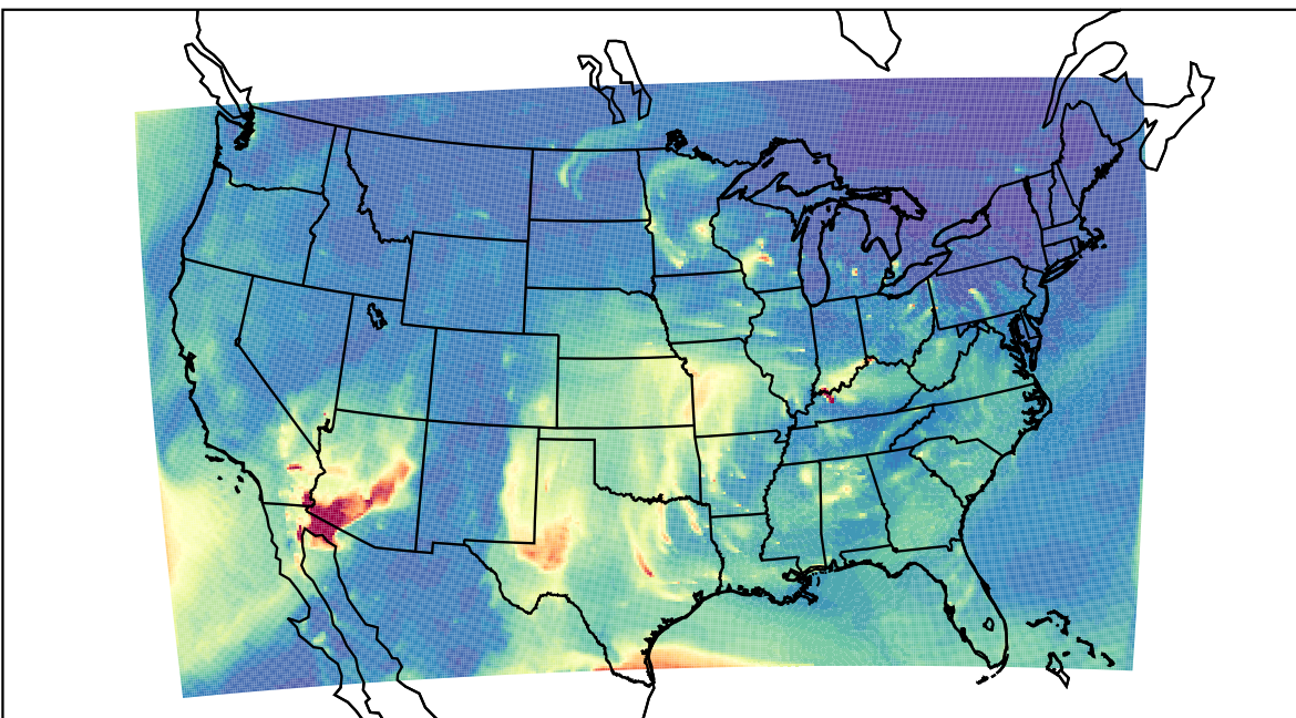
WRF 2023-03-30_12:00:00
