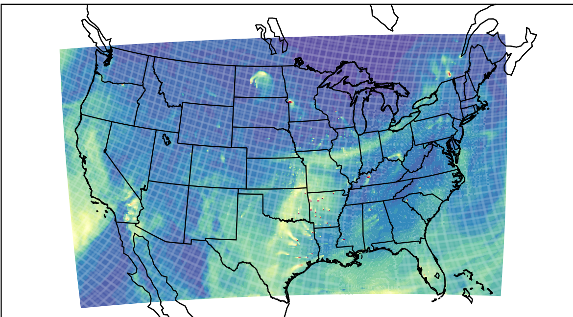
WRF 2023-03-29_19:00:00
