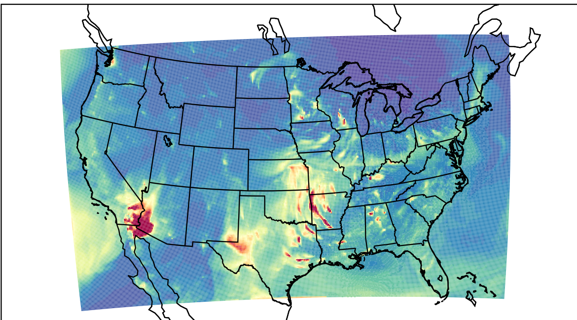
WRF 2023-03-30_04:00:00
