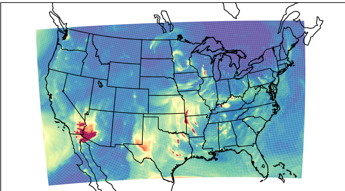
WRF 2023-03-30_06:00:00
