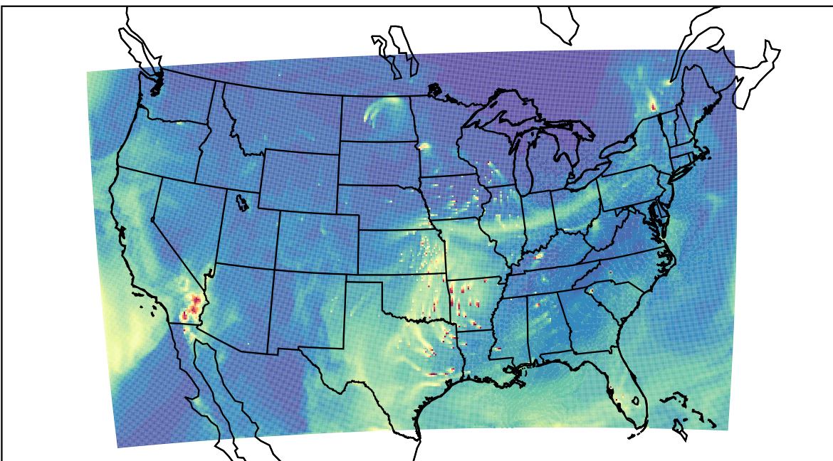
WRF 2023-03-29_22:00:00
