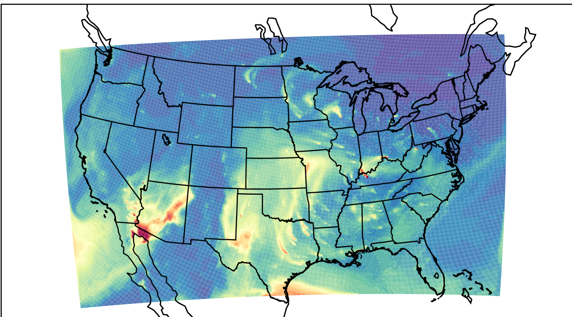
WRF 2023-03-30_14:00:00
