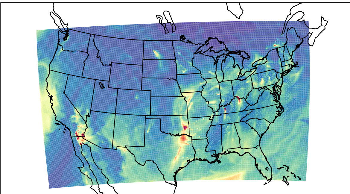
WRF 2023-03-29_10:00:00
