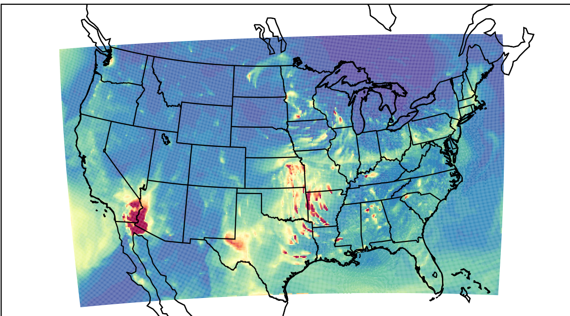
WRF 2023-03-30_03:00:00
