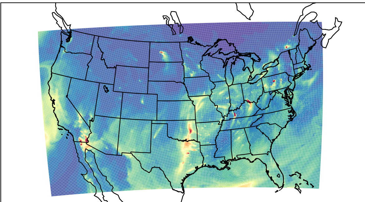
WRF 2023-03-29_13:00:00
