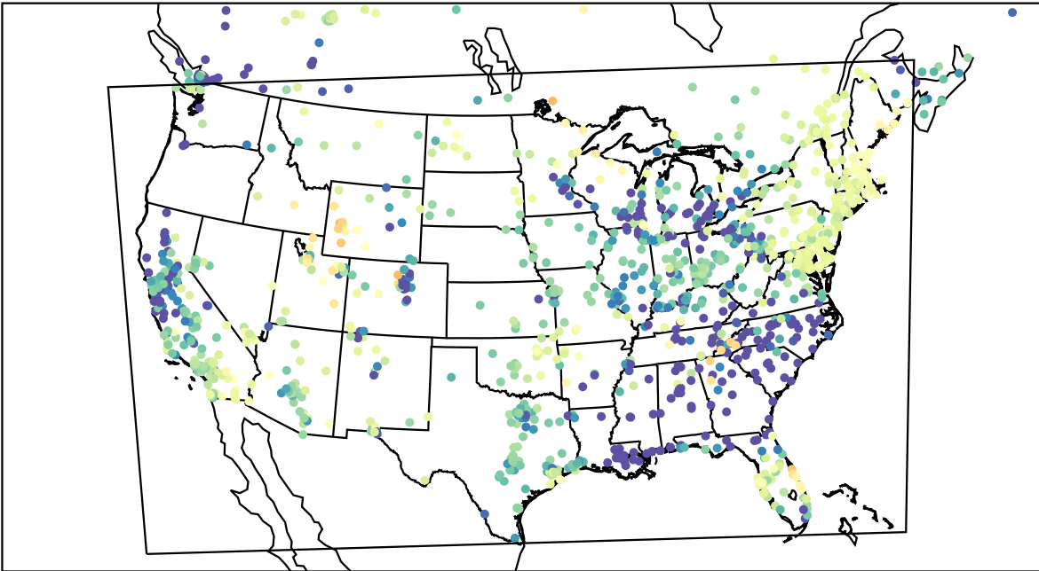
AirNOW (2023-03-30_09:00:00)
