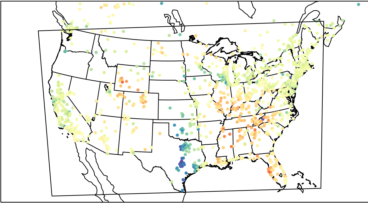
AirNOW (2023-03-30_23:00:00)
