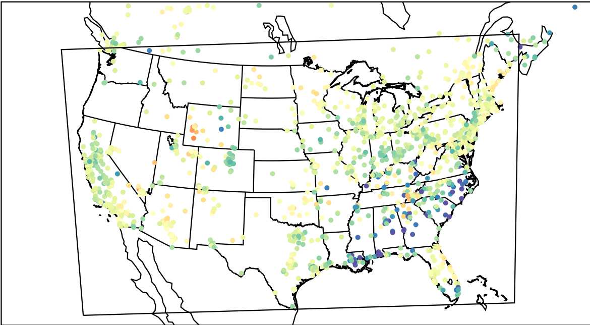
AirNOW (2023-03-30_01:00:00)
