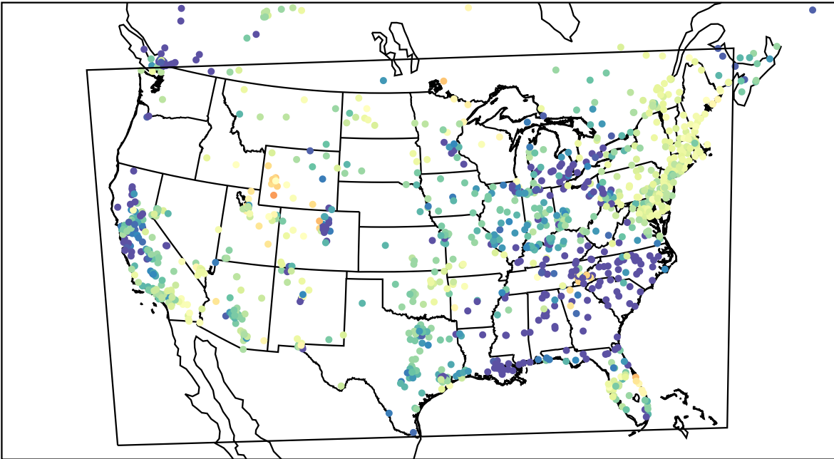
AirNOW (2023-03-30_10:00:00)
