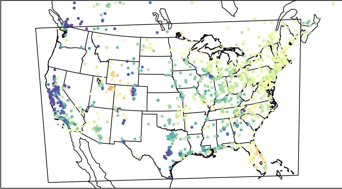
AirNOW (2023-03-30_14:00:00)
