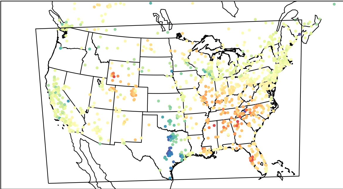
AirNOW (2023-03-30_22:00:00)
