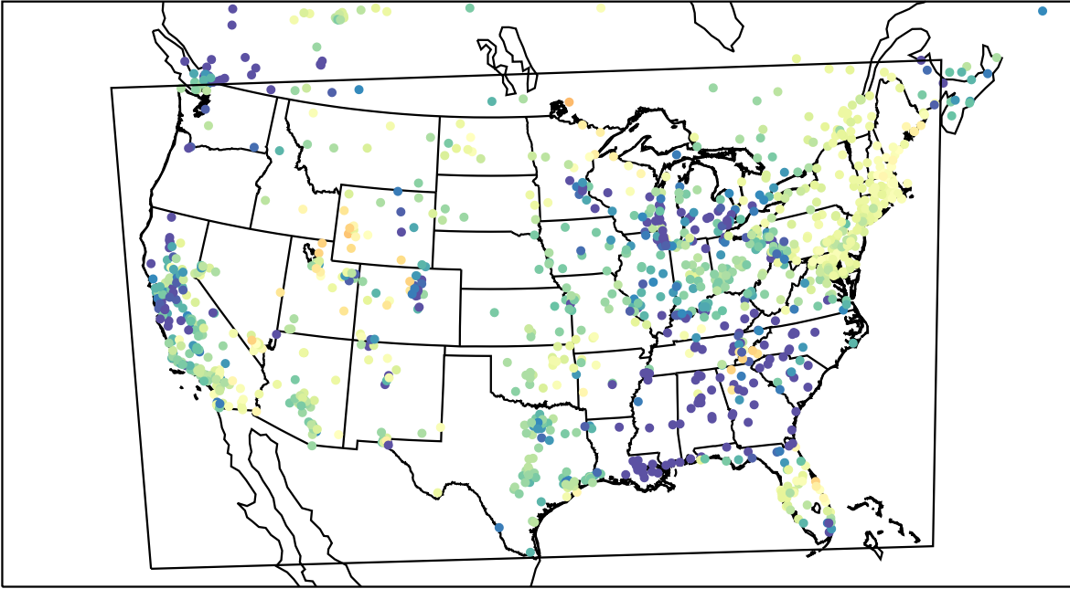
AirNOW (2023-03-30_08:00:00)
