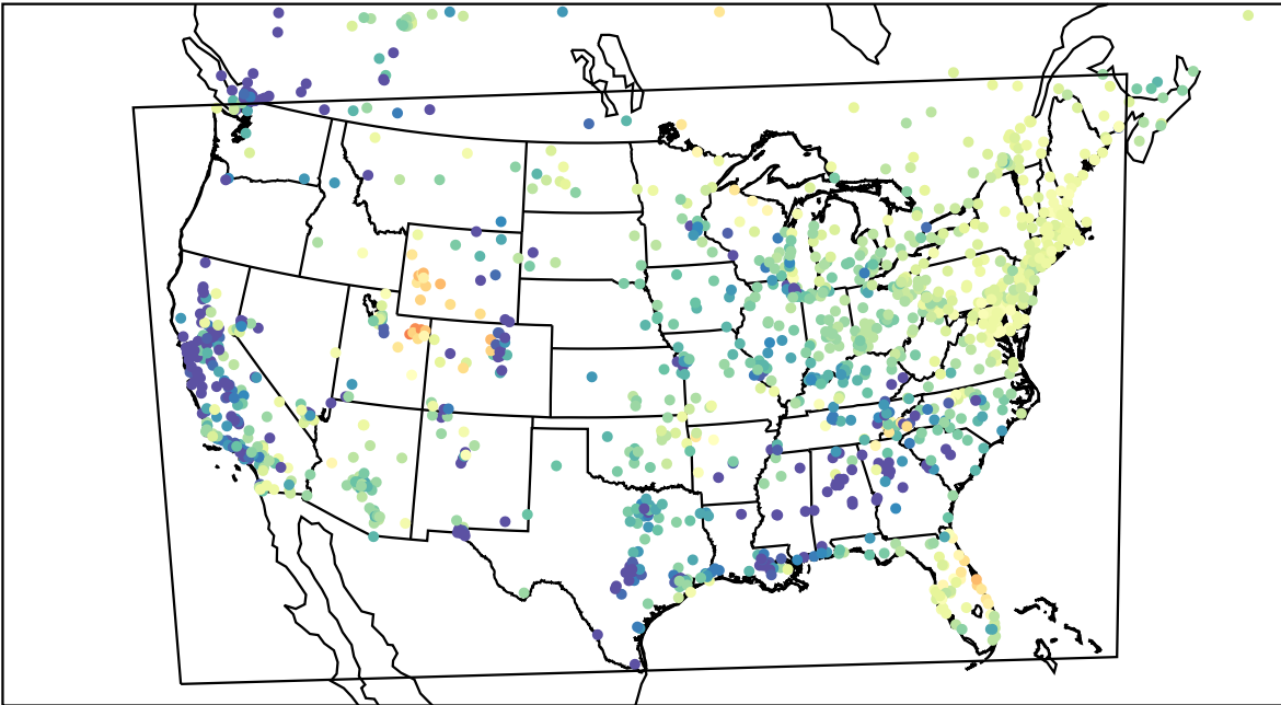
AirNOW (2023-03-30_13:00:00)
