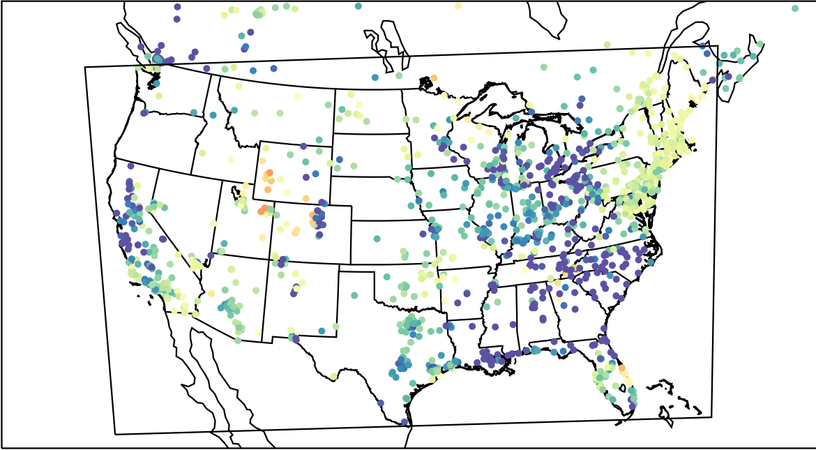
AirNOW (2023-03-30_11:00:00)
