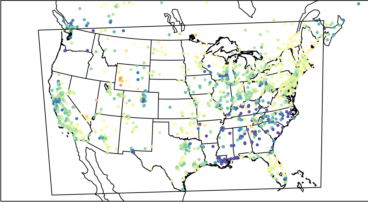
AirNOW (2023-03-30_03:00:00)
