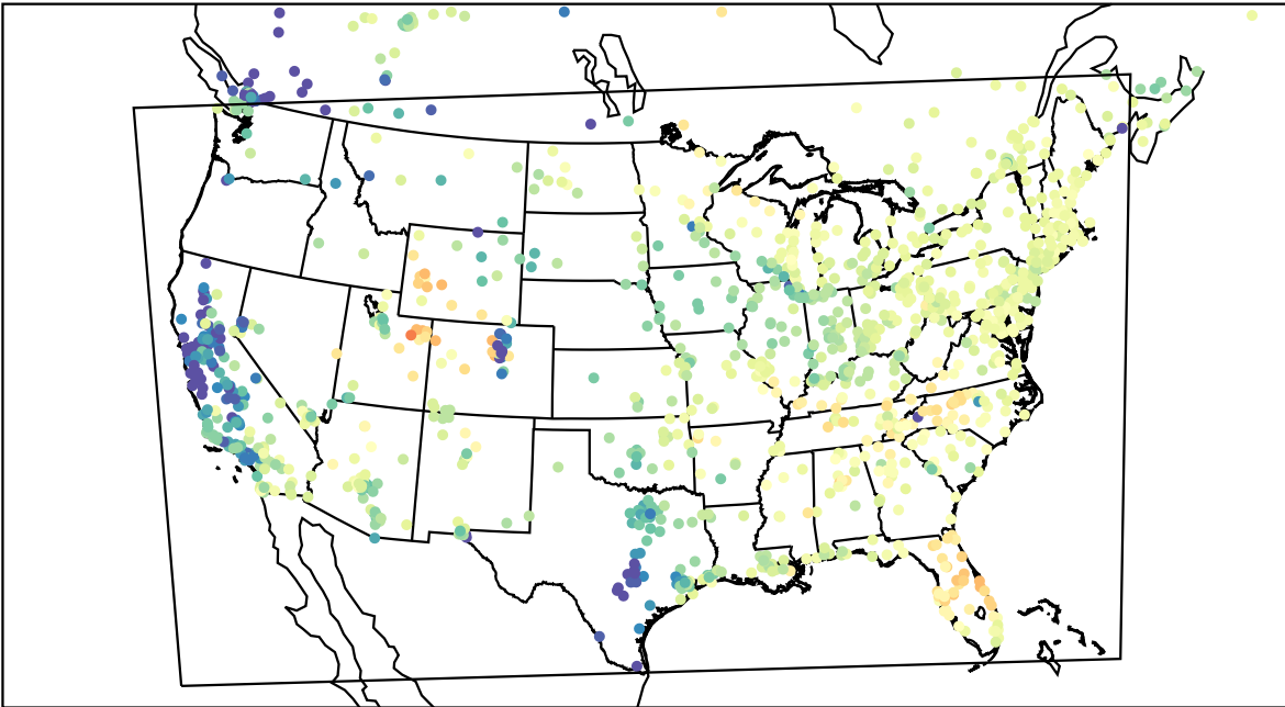
AirNOW (2023-03-30_15:00:00)
