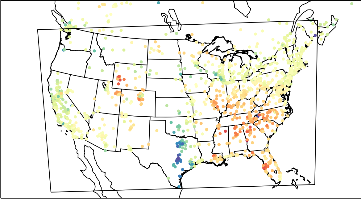
AirNOW (2023-03-30_21:00:00)
