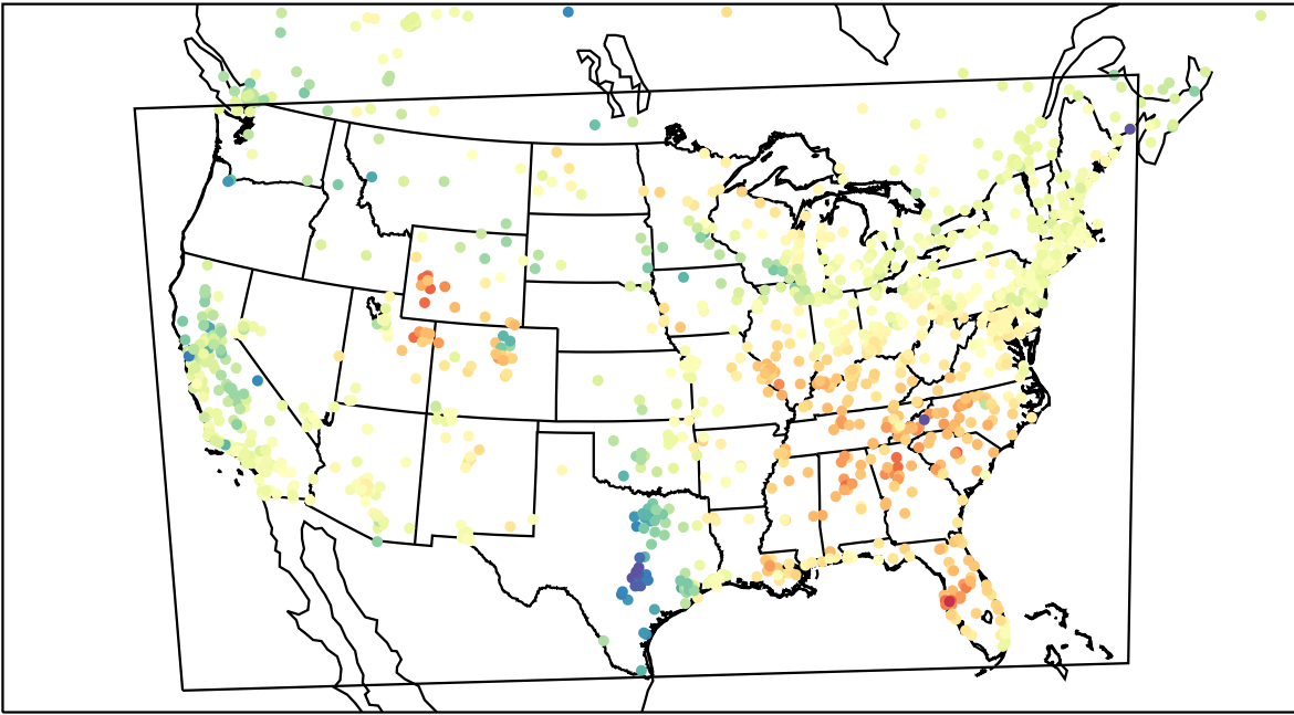
AirNOW (2023-03-30_19:00:00)
