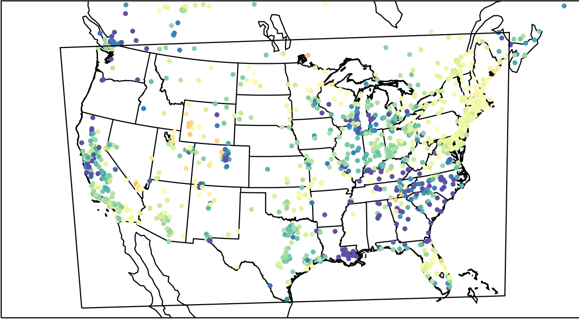
AirNOW (2023-03-30_06:00:00)
