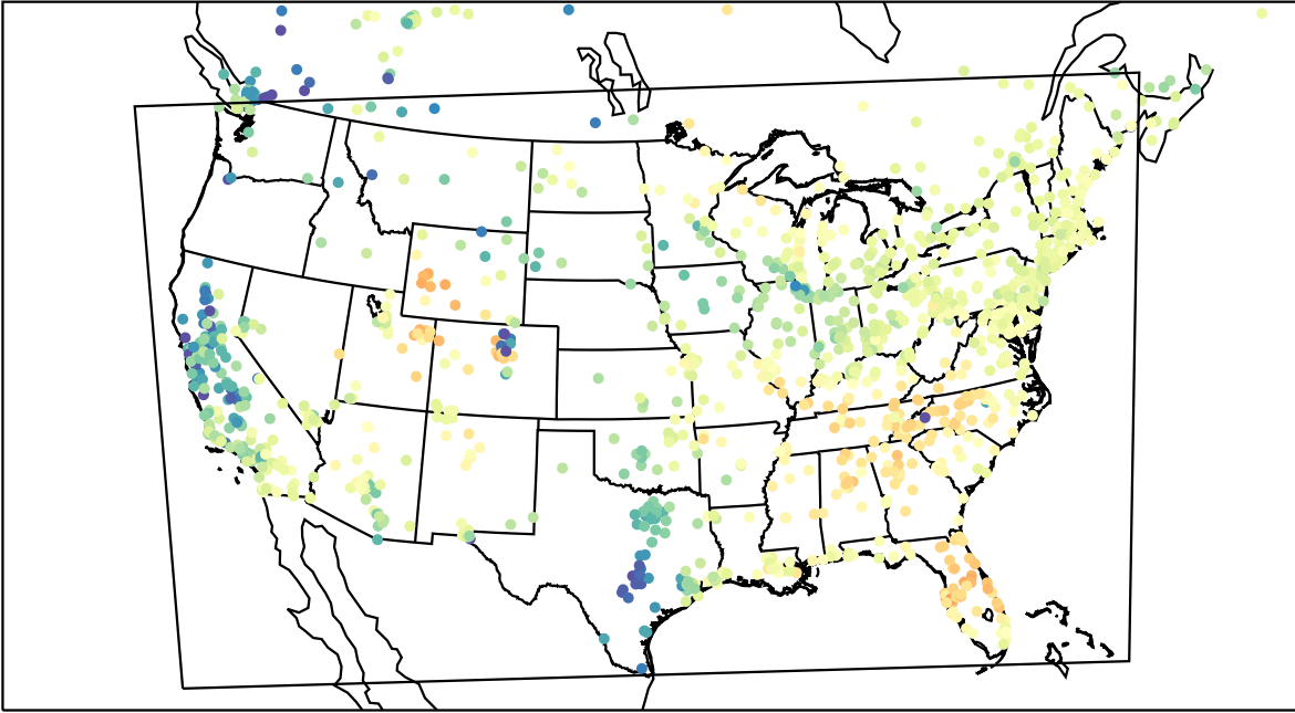
AirNOW (2023-03-30_16:00:00)
