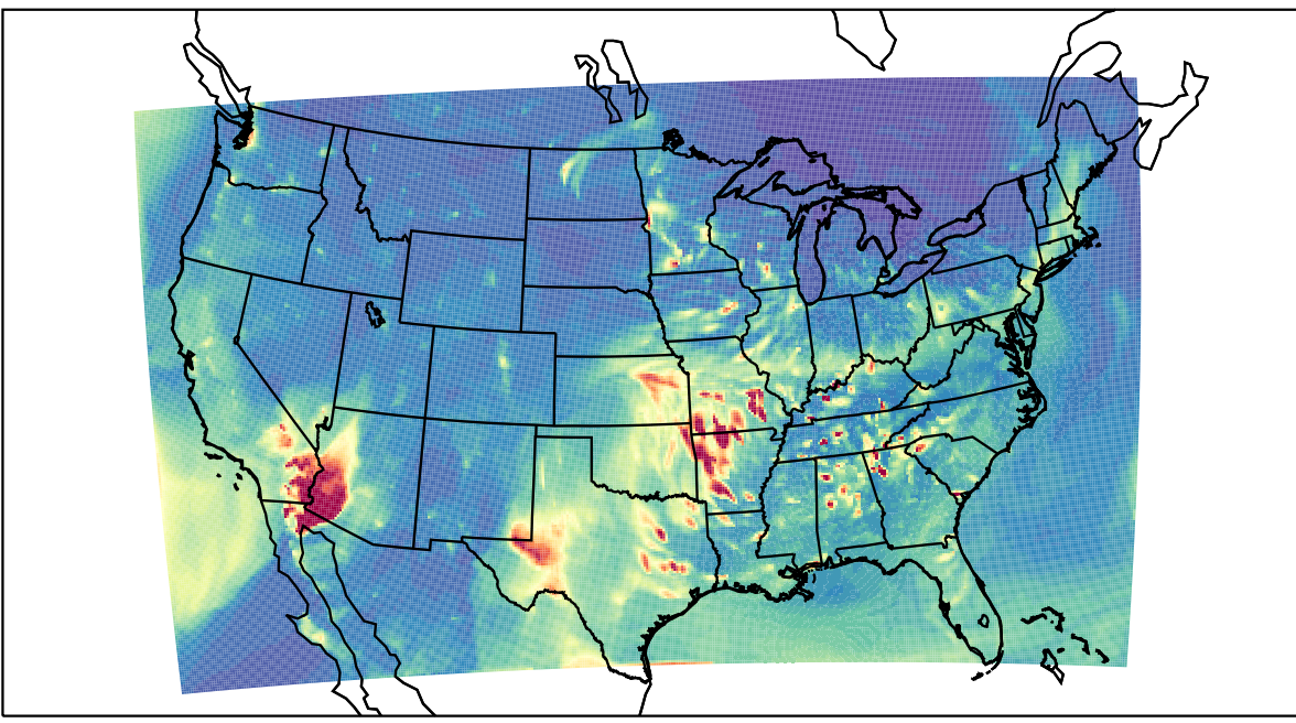
WRF 2023-03-30_04:00:00
