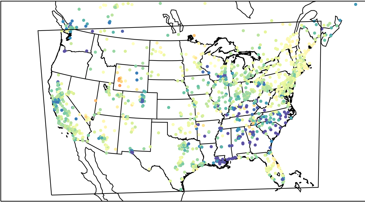
AirNOW (2023-03-30_03:00:00)
