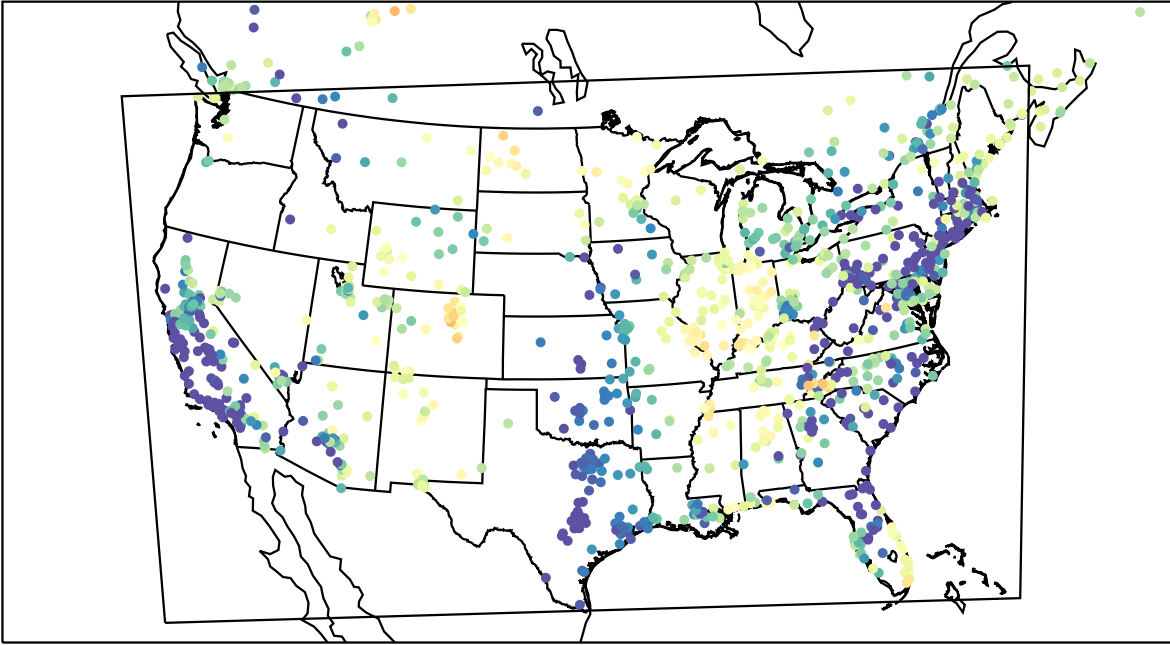
AirNOW (2023-03-31_10:00:00)
