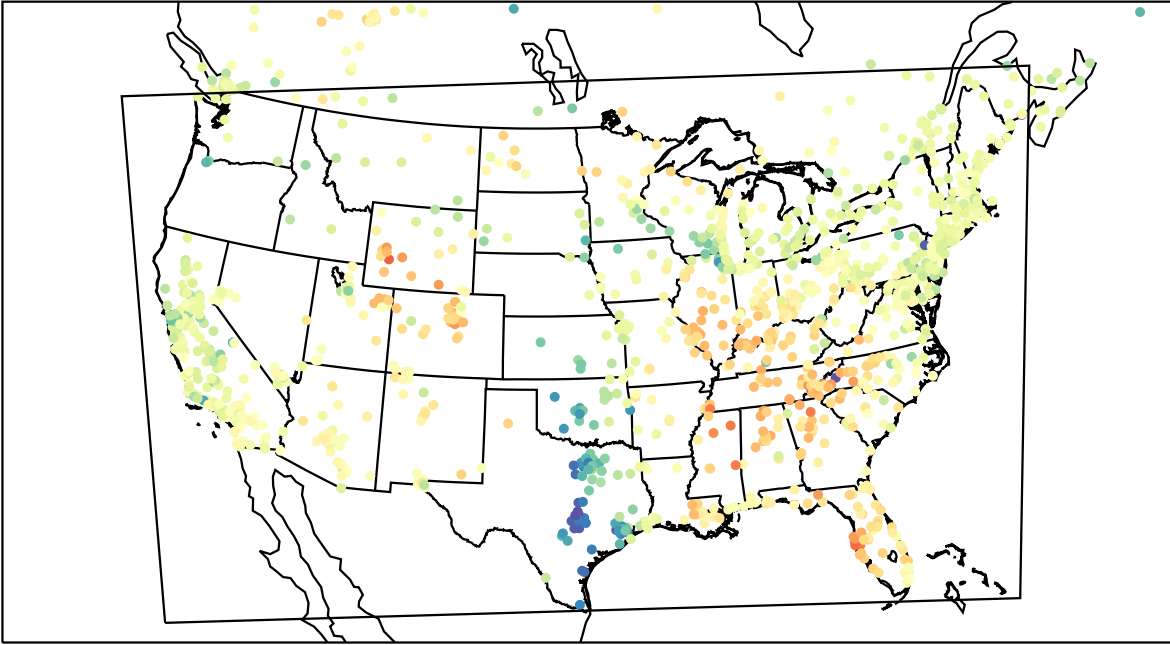
AirNOW (2023-03-30_23:00:00)
