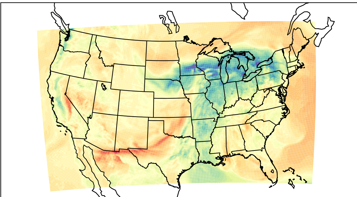
WRF (2023-03-31_18:00:00)
