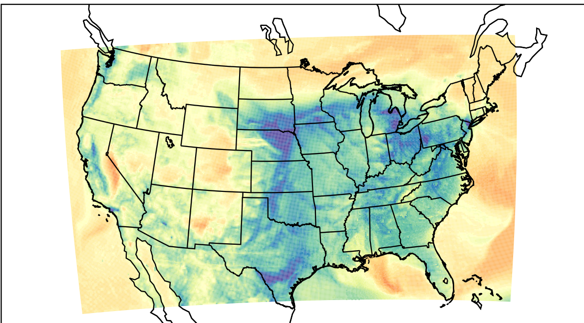
WRF (2023-03-31_10:00:00)
