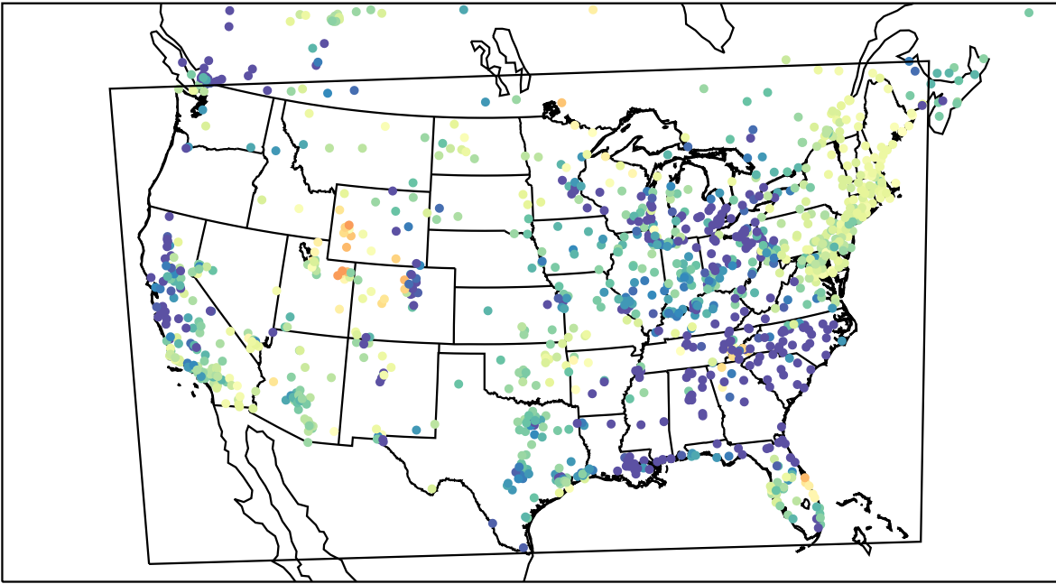
AirNOW (2023-03-30_11:00:00)
