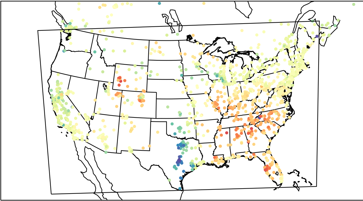
AirNOW (2023-03-30_21:00:00)
