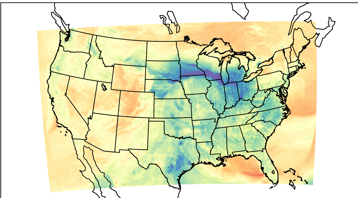
WRF (2023-03-31_01:00:00)
