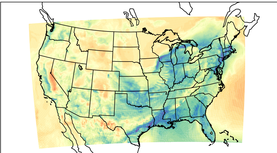
WRF (2023-04-01_10:00:00)
