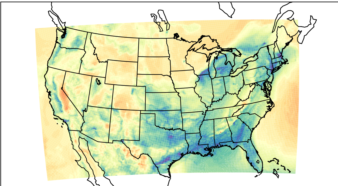
WRF (2023-04-01_13:00:00)
