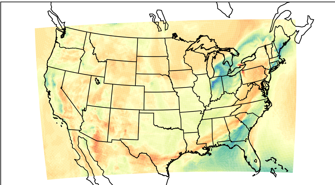
WRF (2023-04-01_18:00:00)
