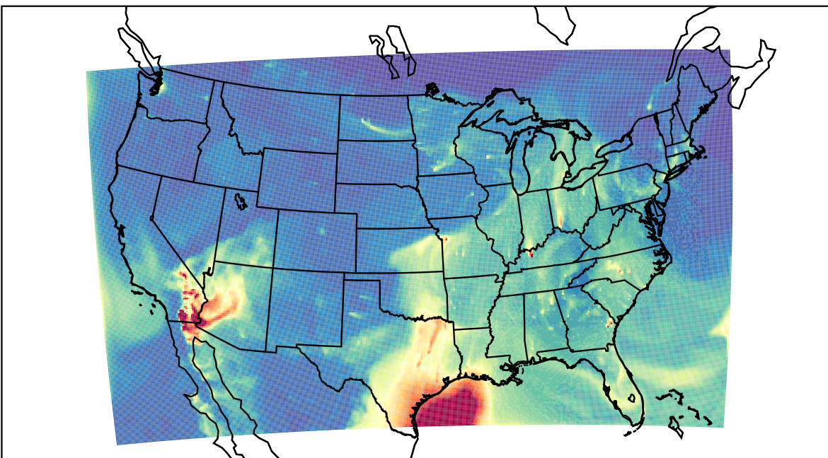
WRF 2023-04-03_10:00:00
