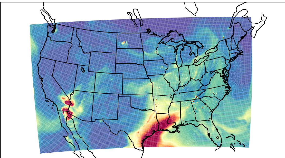
WRF 2023-04-03_18:00:00
