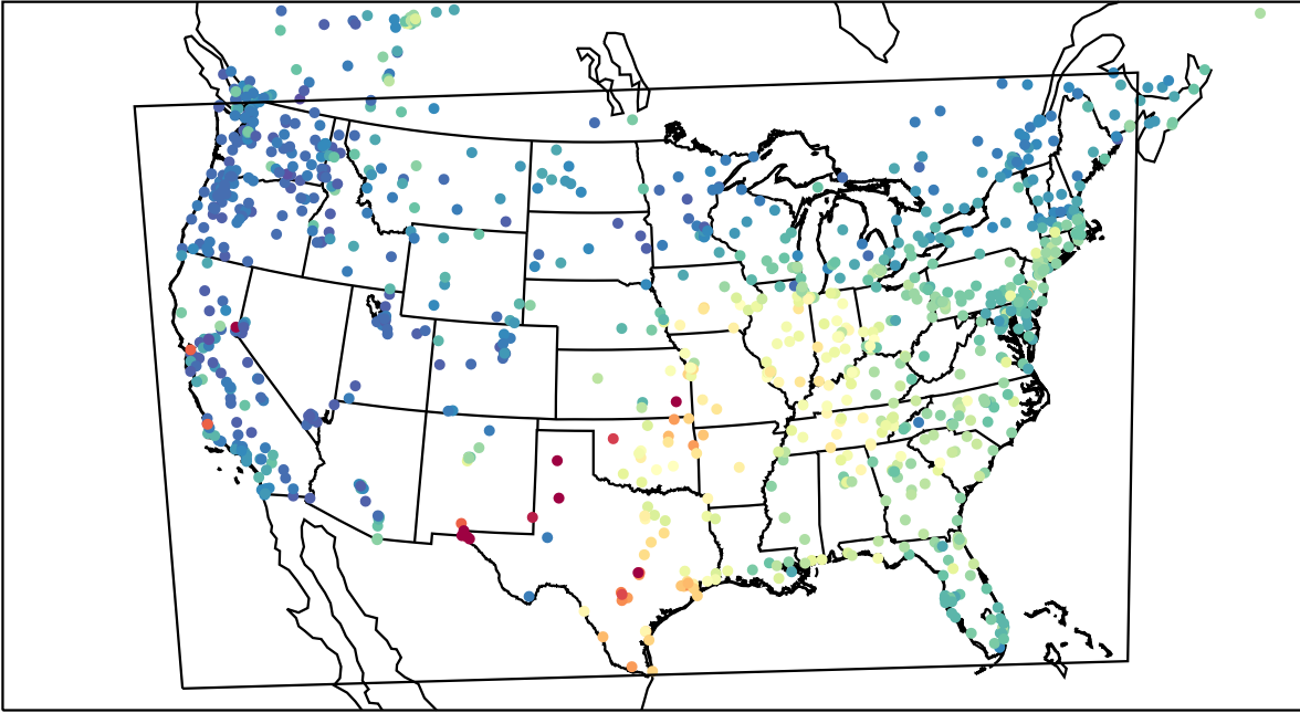
AirNOW
