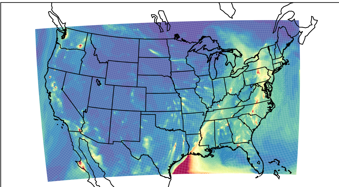
WRF 2023-04-06_04:00:00
