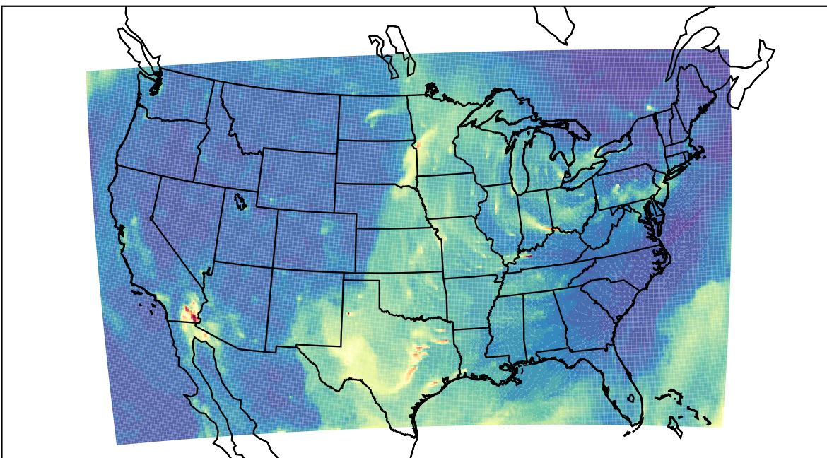
WRF 2023-04-09_14:00:00
