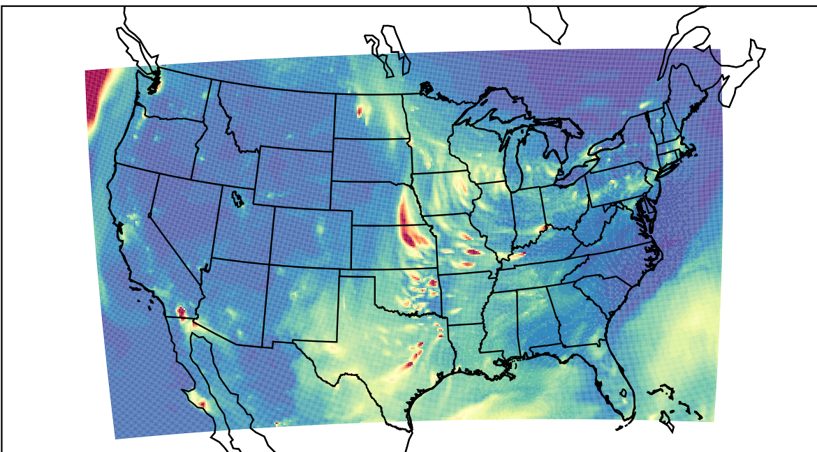
WRF 2023-04-09_04:00:00
