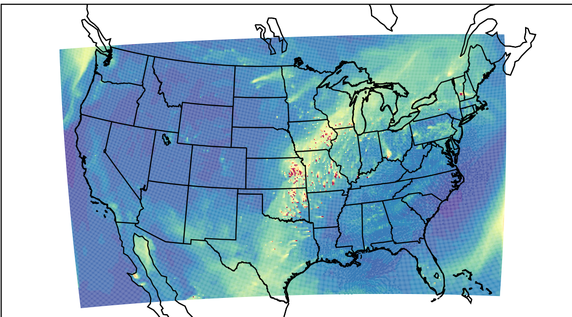
WRF 2023-04-10_23:00:00
