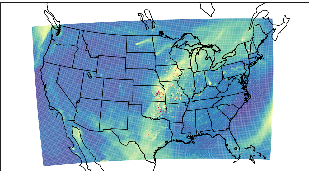
WRF 2023-04-10_22:00:00
