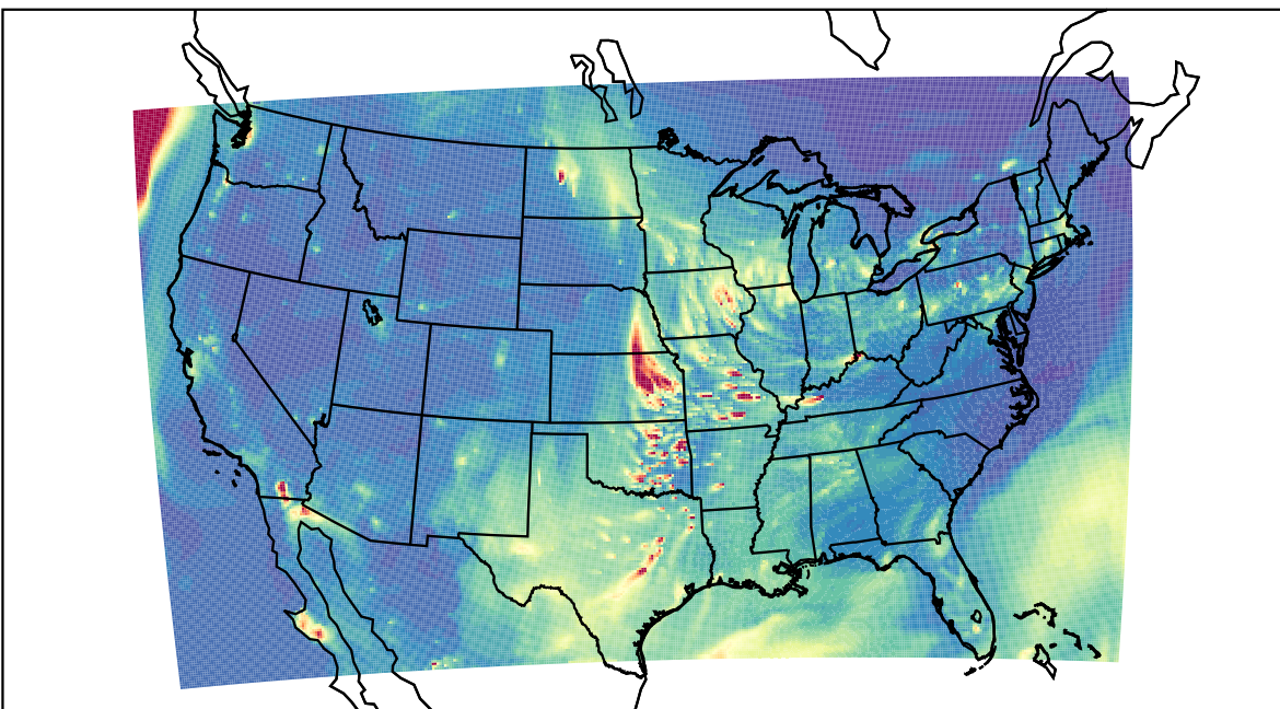
WRF 2023-04-09_03:00:00
