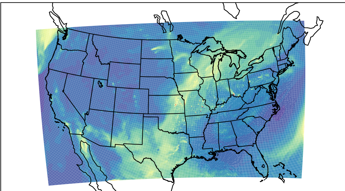
WRF 2023-04-10_18:00:00
