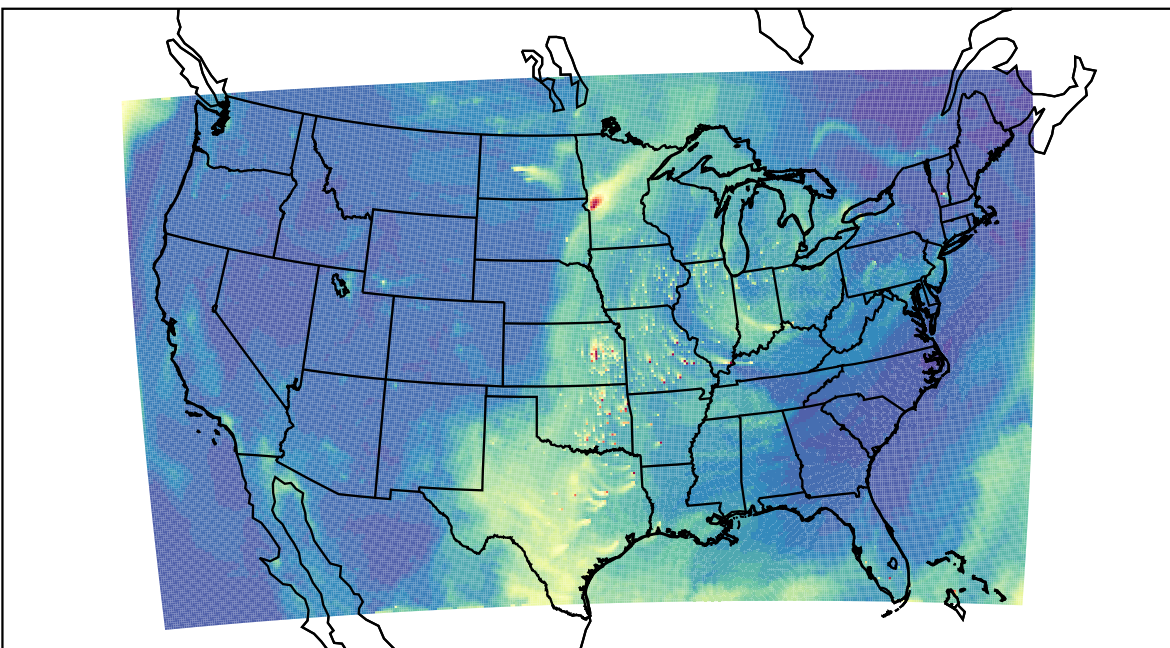
WRF 2023-04-09_20:00:00
