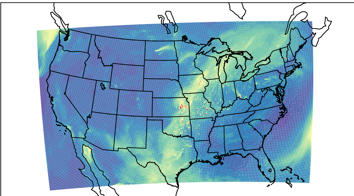
WRF 2023-04-10_20:00:00
