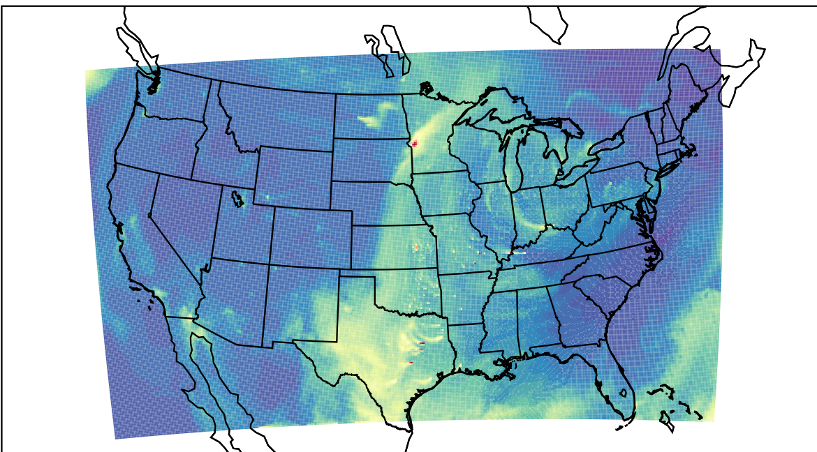
WRF 2023-04-09_18:00:00
