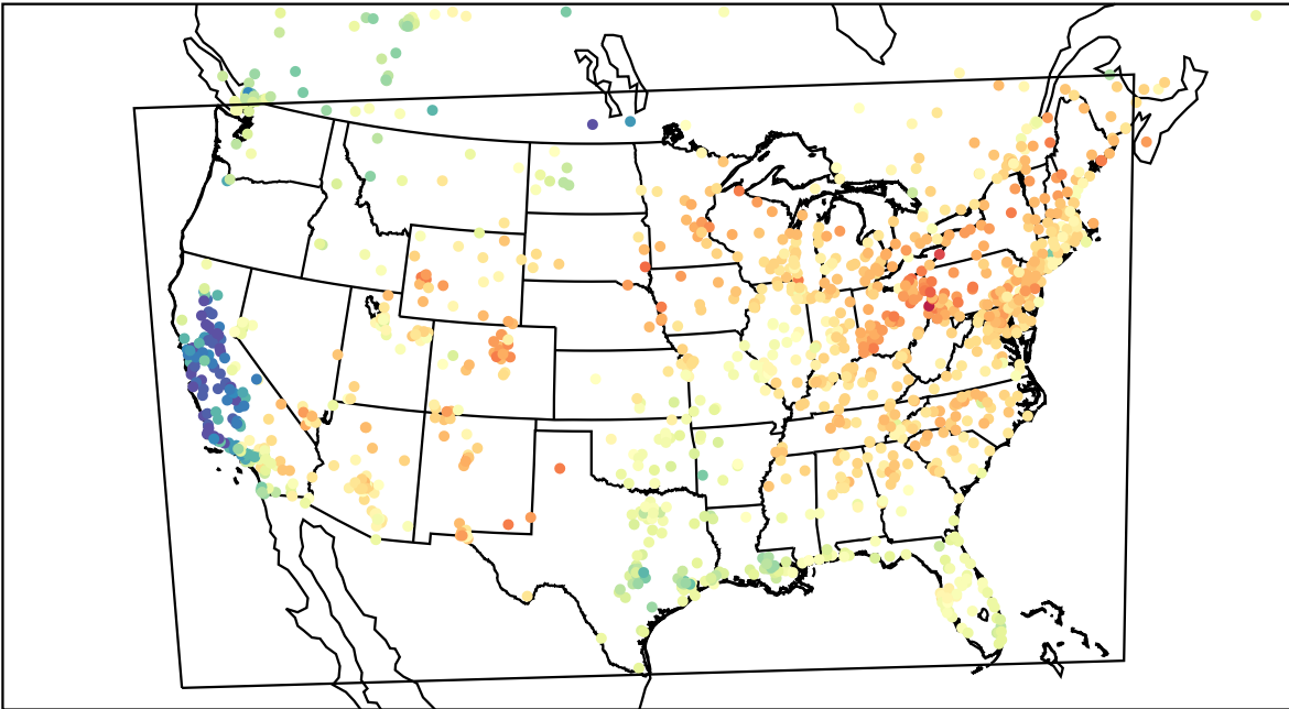
AirNOW (2023-04-11_18:00:00)
