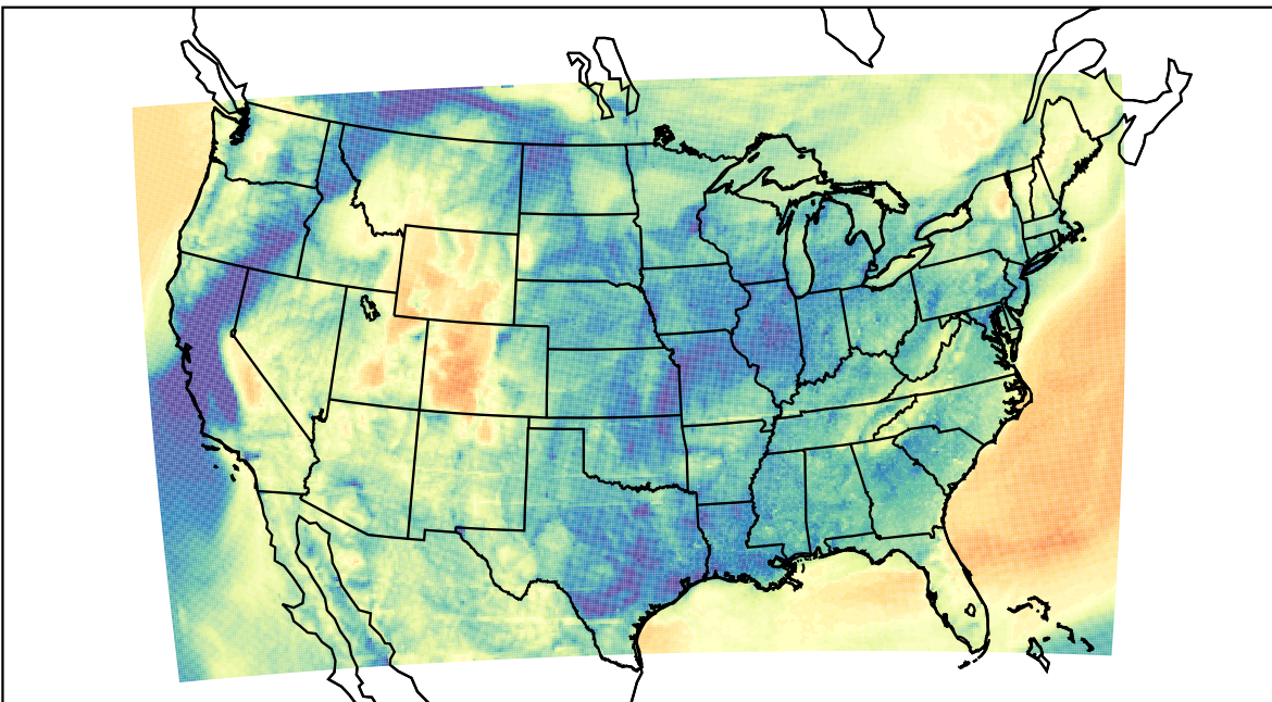
WRF (2023-04-11_13:00:00)
