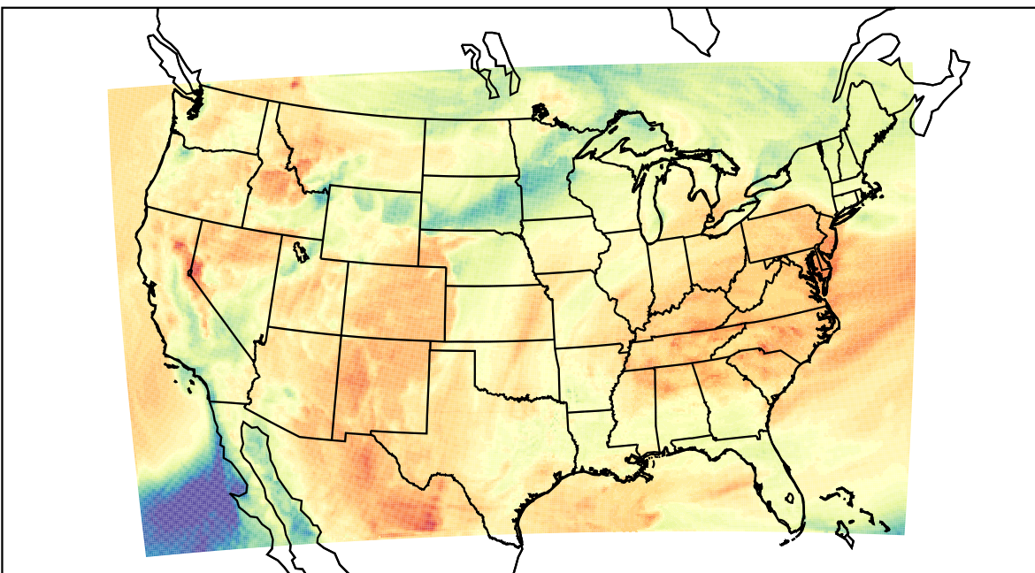
WRF (2023-04-12_18:00:00)
