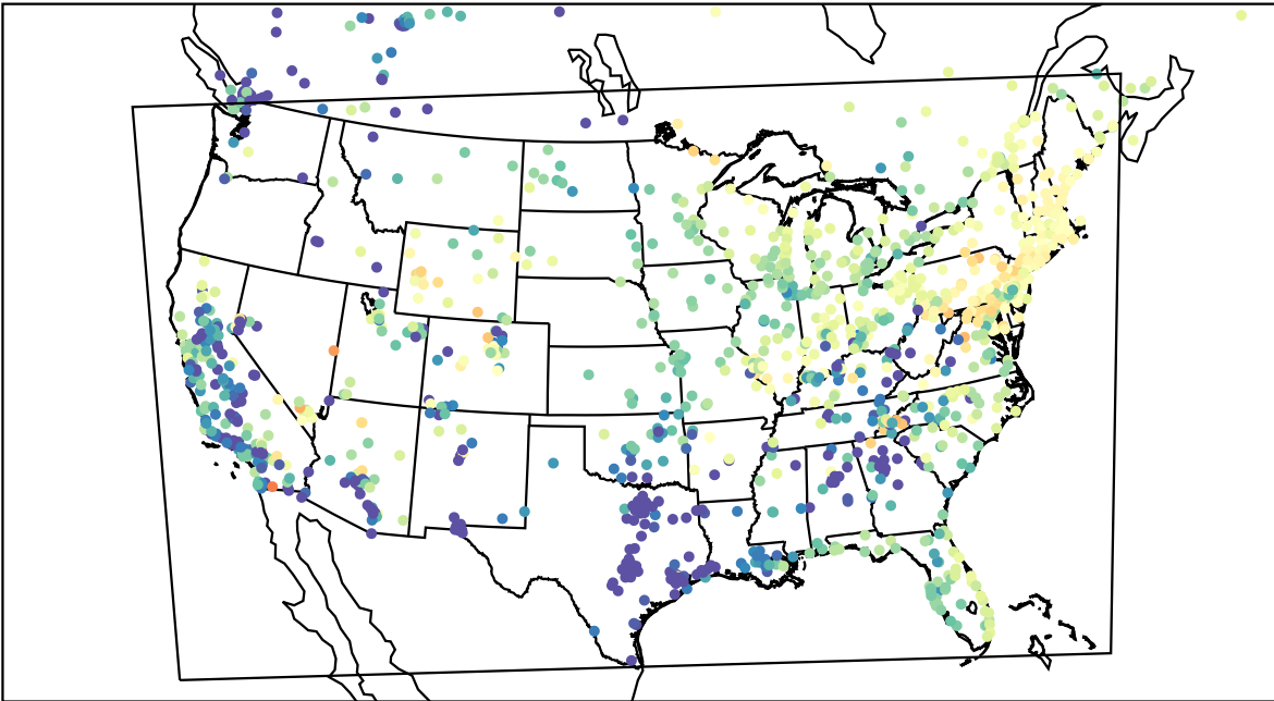
AirNOW (2023-04-12_13:00:00)
