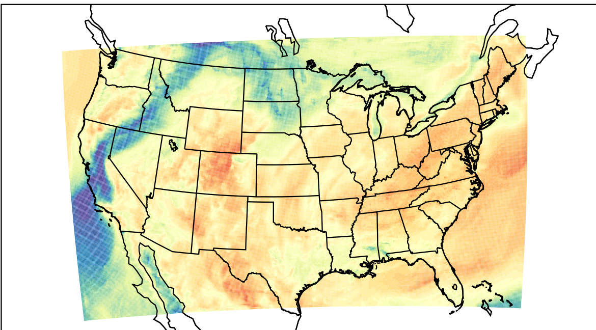
WRF (2023-04-11_18:00:00)
