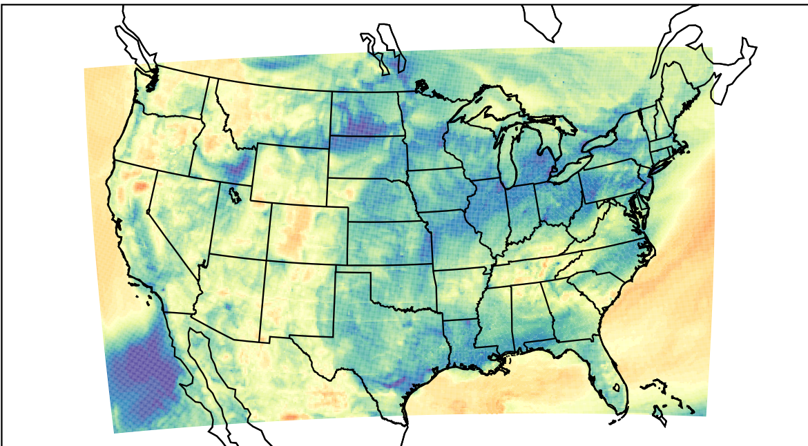
WRF (2023-04-12_10:00:00)
