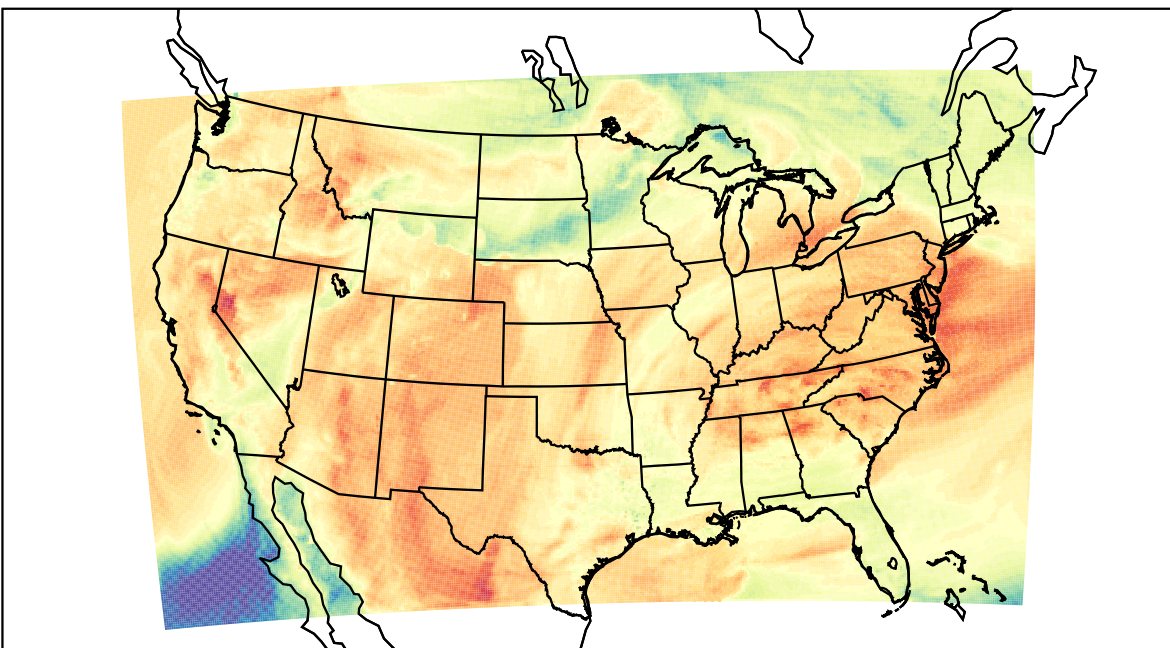
WRF (2023-04-12_20:00:00)
