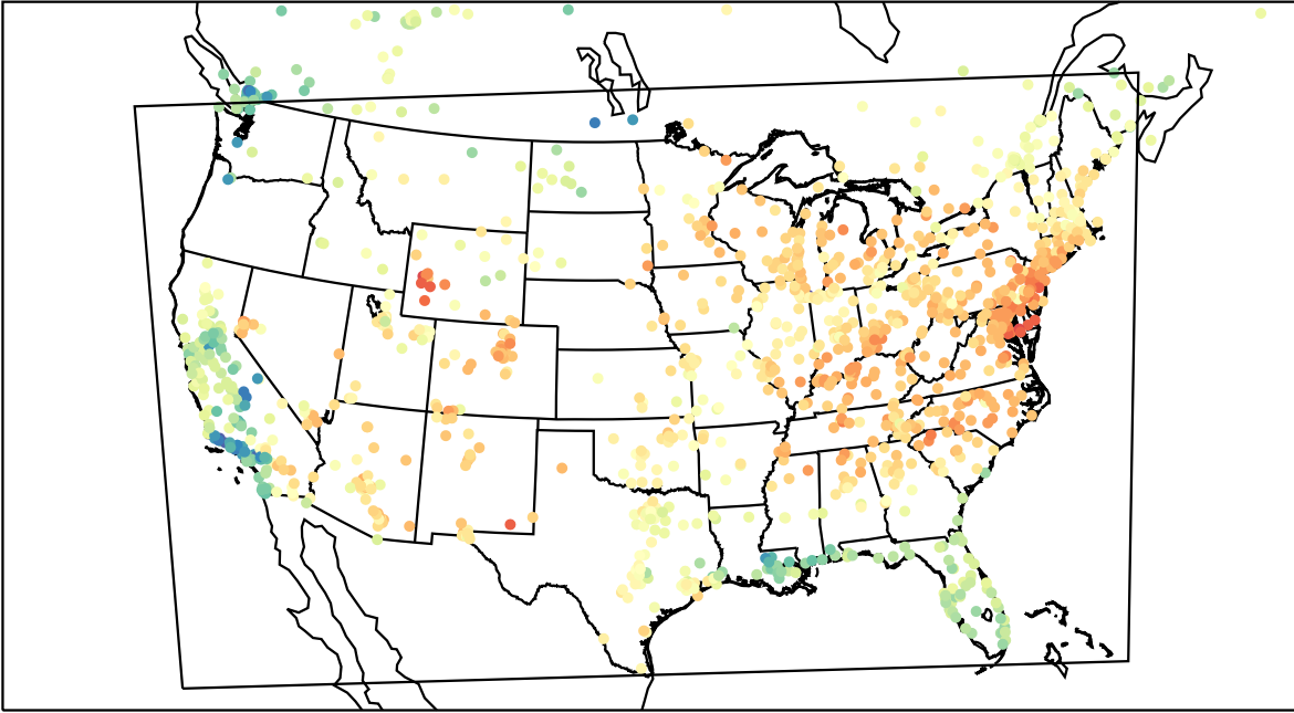
AirNOW (2023-04-12_18:00:00)
