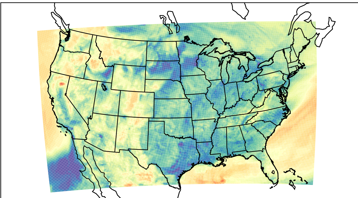
WRF (2023-04-12_13:00:00)
