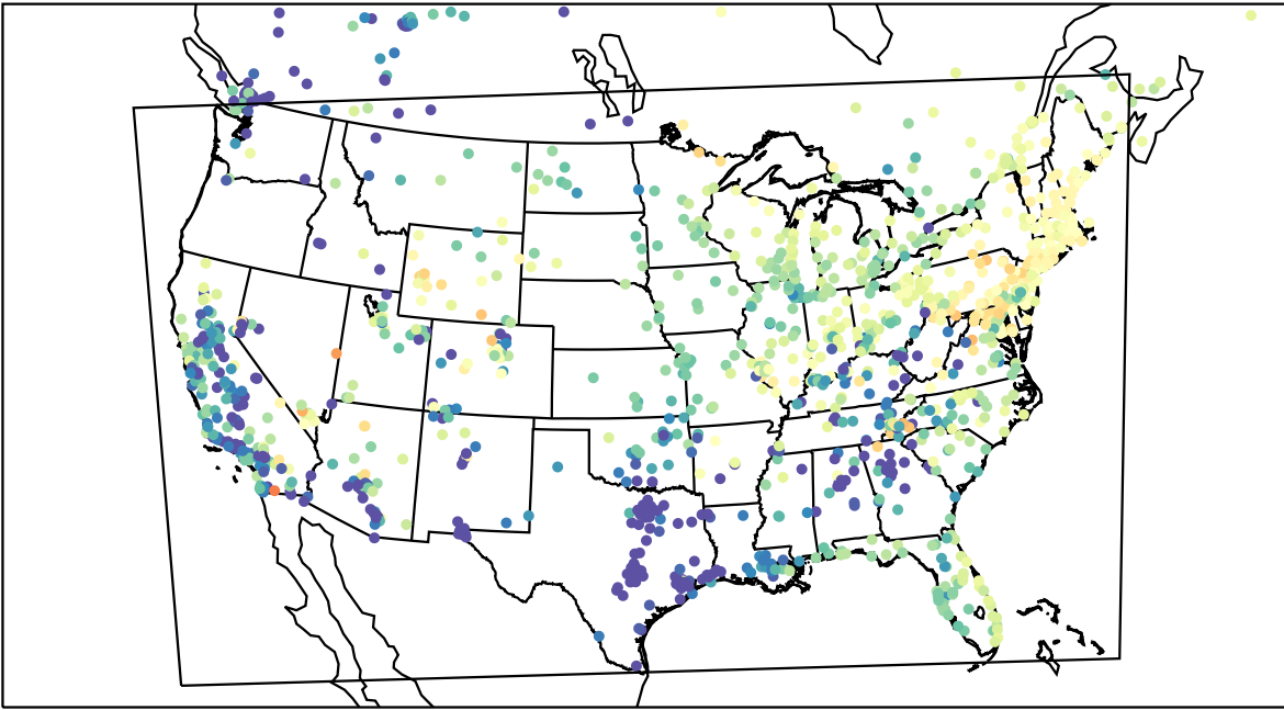
AirNOW (2023-04-12_13:00:00)
