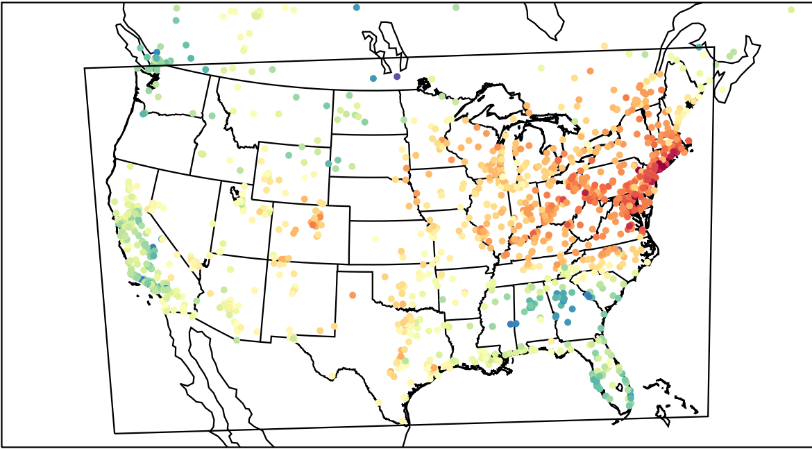
AirNOW (2023-04-13_18:00:00)
