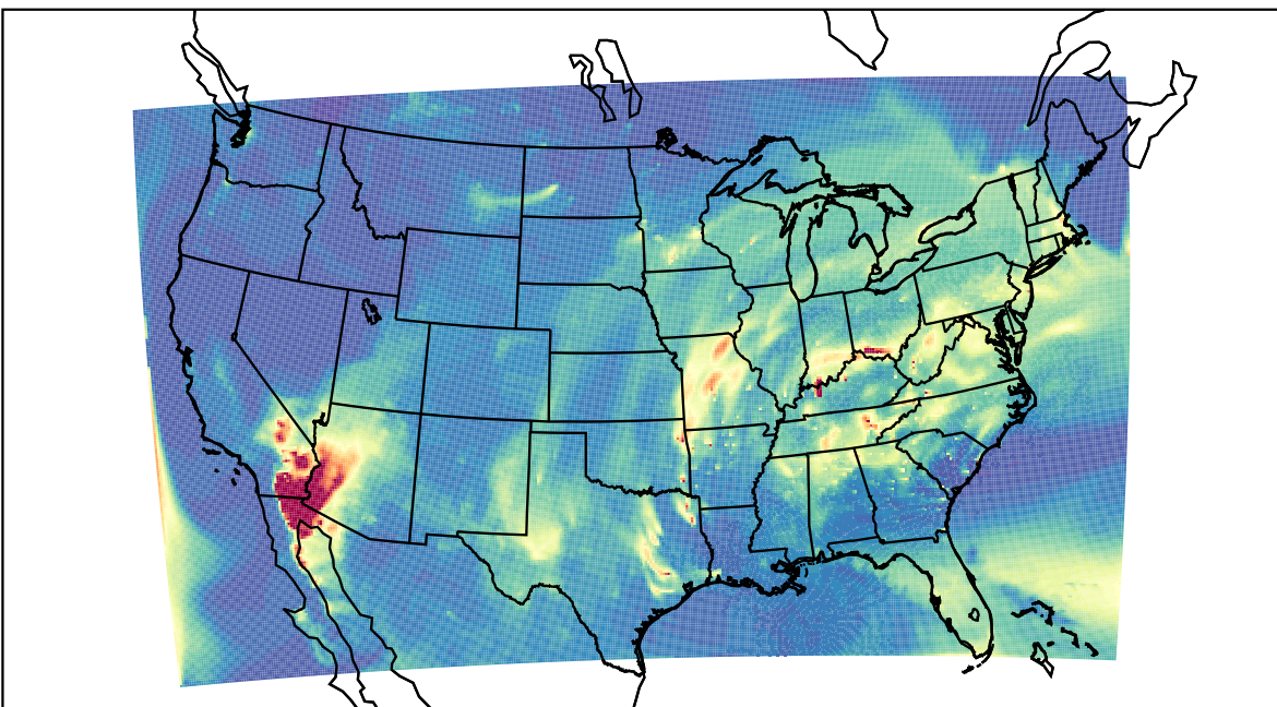
WRF 2023-04-13_10:00:00
