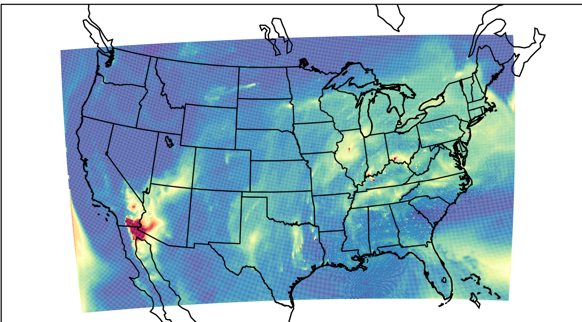
WRF 2023-04-13_16:00:00
