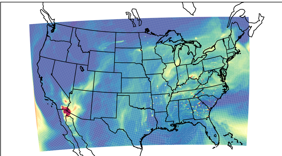
WRF 2023-04-13_18:00:00
