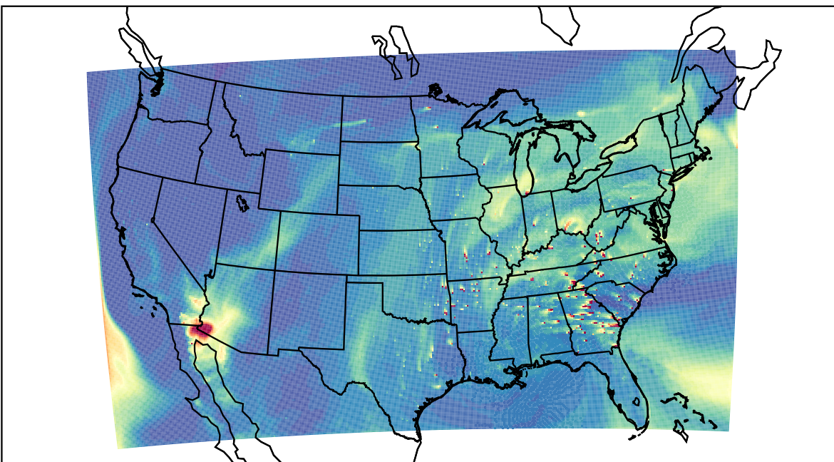
WRF 2023-04-13_20:00:00
