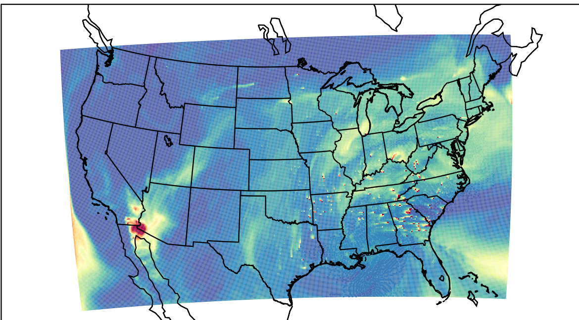
WRF 2023-04-13_19:00:00
