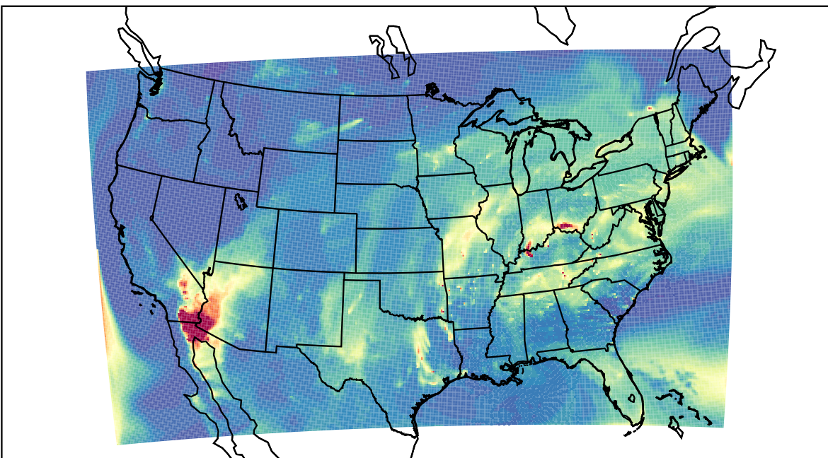
WRF 2023-04-13_13:00:00
