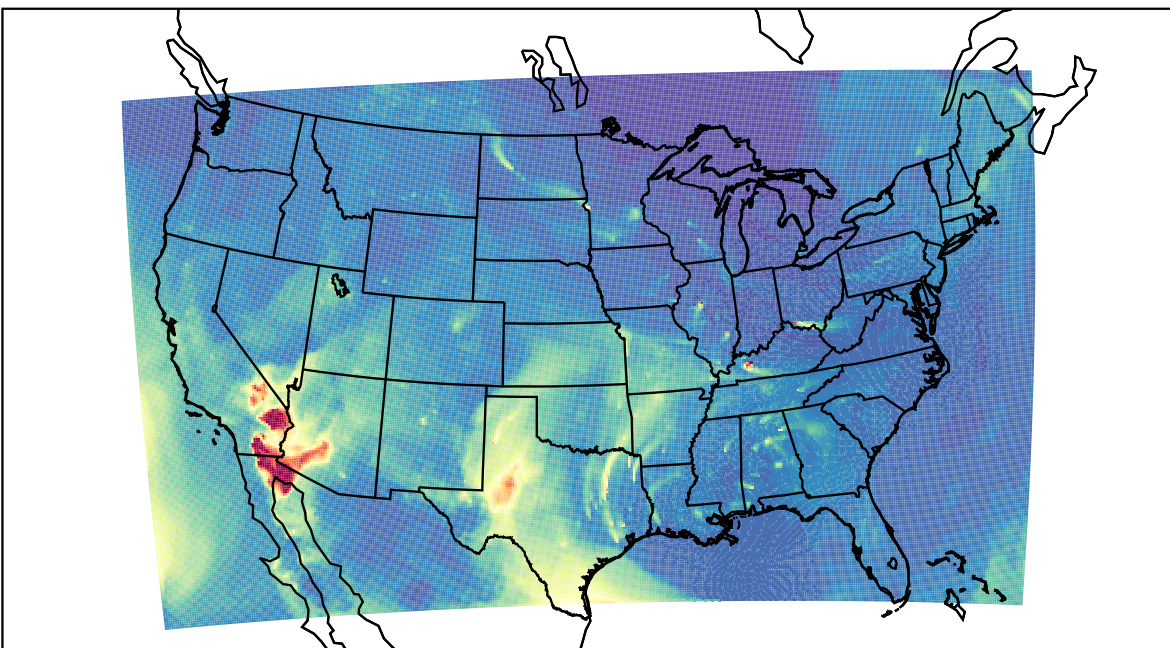
WRF 2023-04-18_14:00:00
