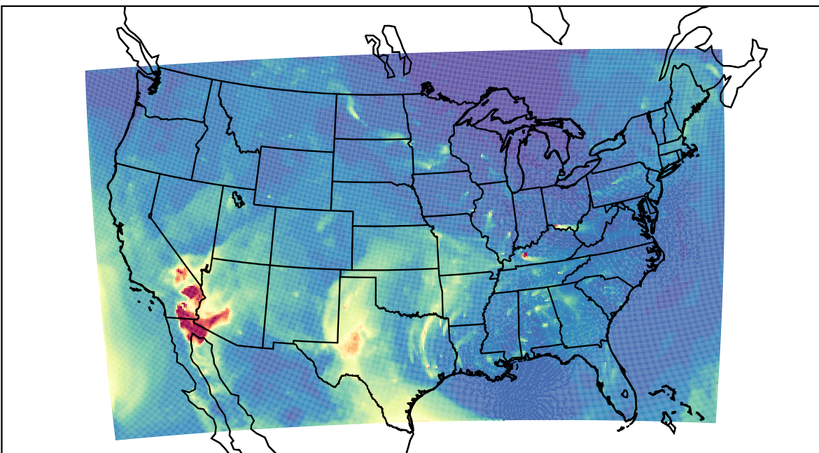
WRF 2023-04-18_13:00:00
