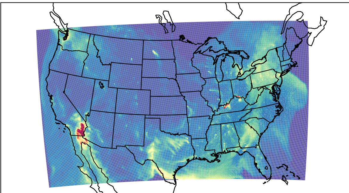
WRF 2023-04-22_13:00:00
