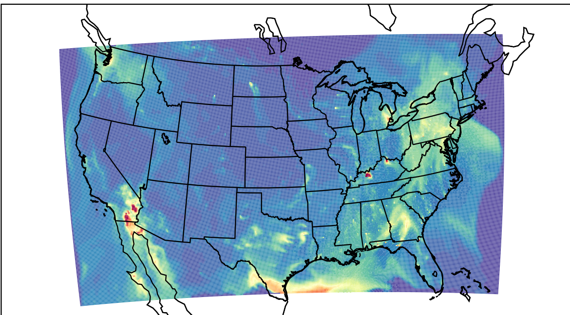
WRF 2023-04-22_10:00:00
