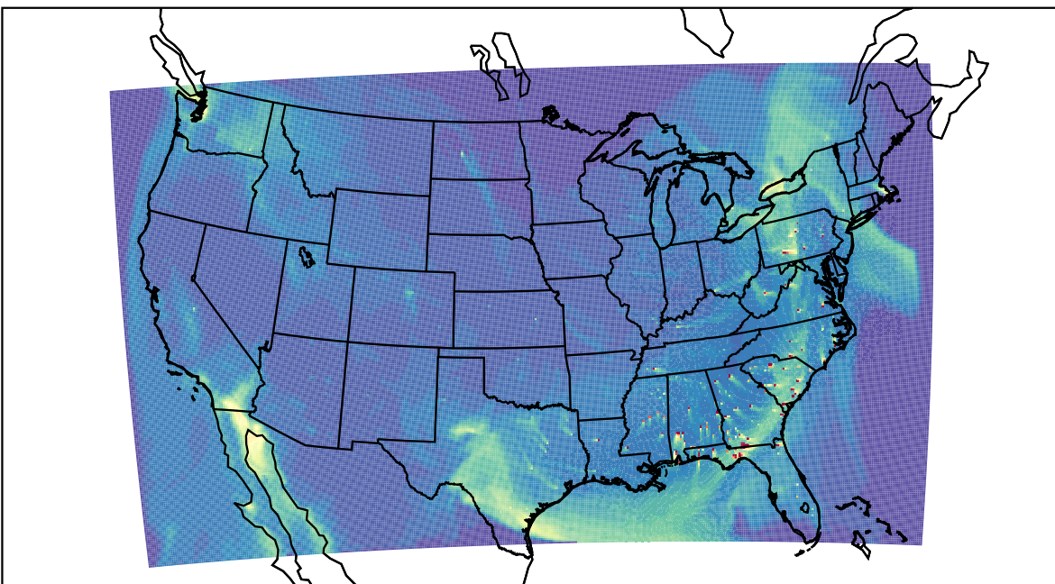
WRF 2023-04-22_20:00:00
