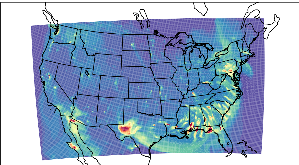
WRF 2023-04-23_03:00:00
