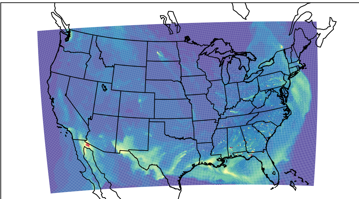
WRF 2023-04-23_18:00:00
