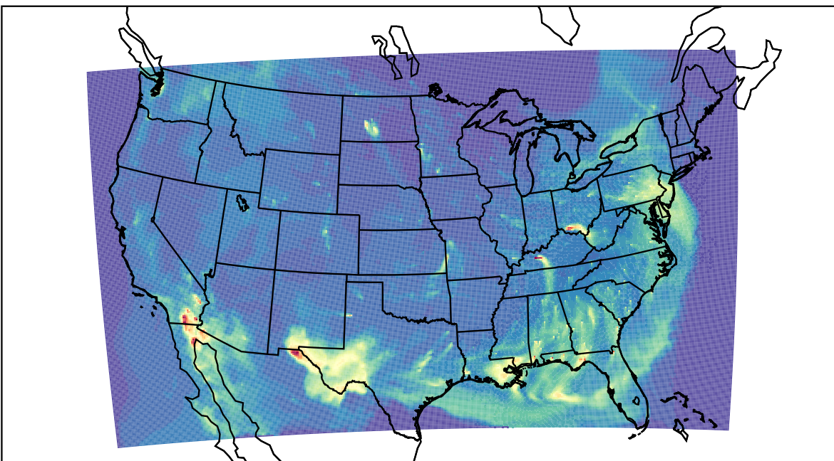
WRF 2023-04-23_10:00:00
