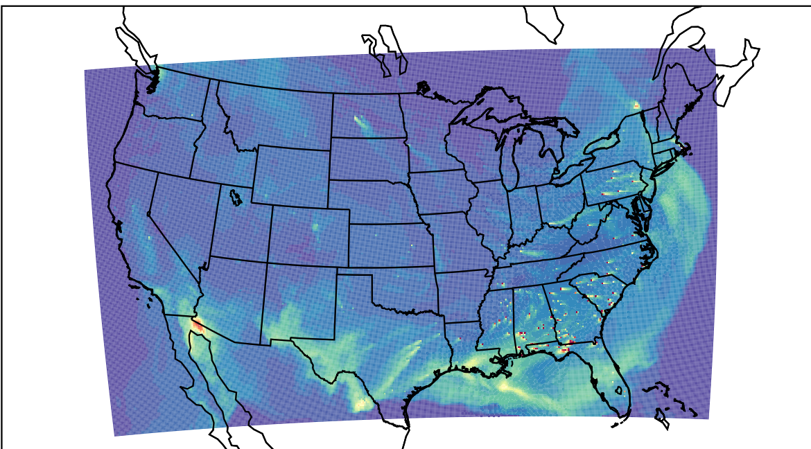
WRF 2023-04-23_20:00:00
