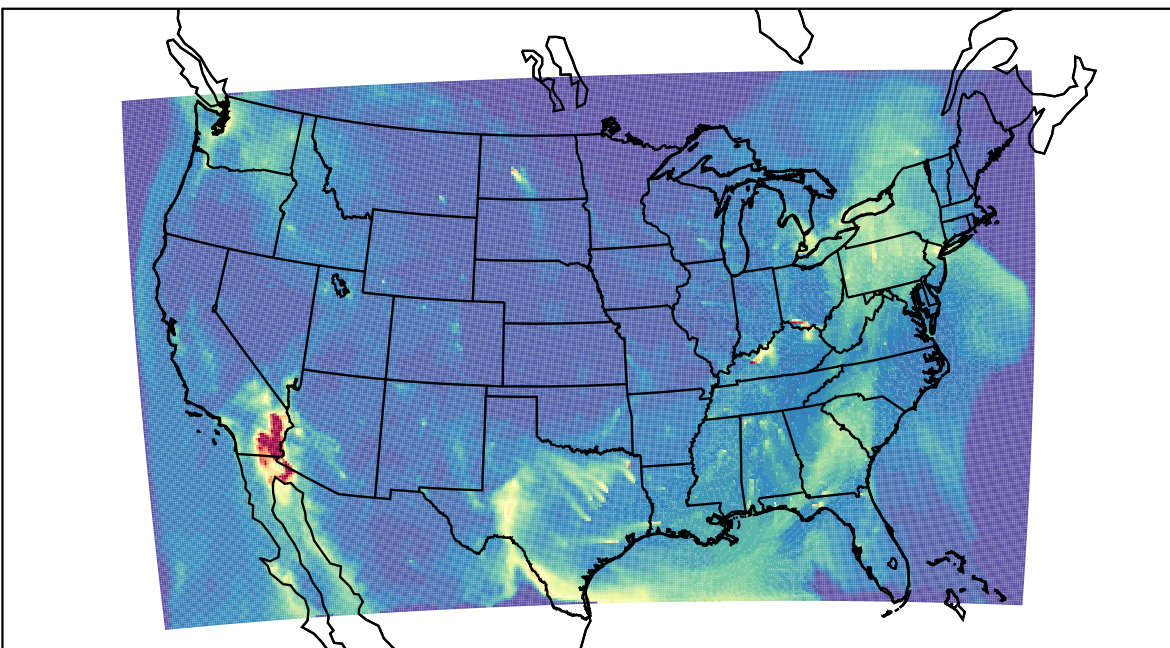
WRF 2023-04-22_14:00:00
