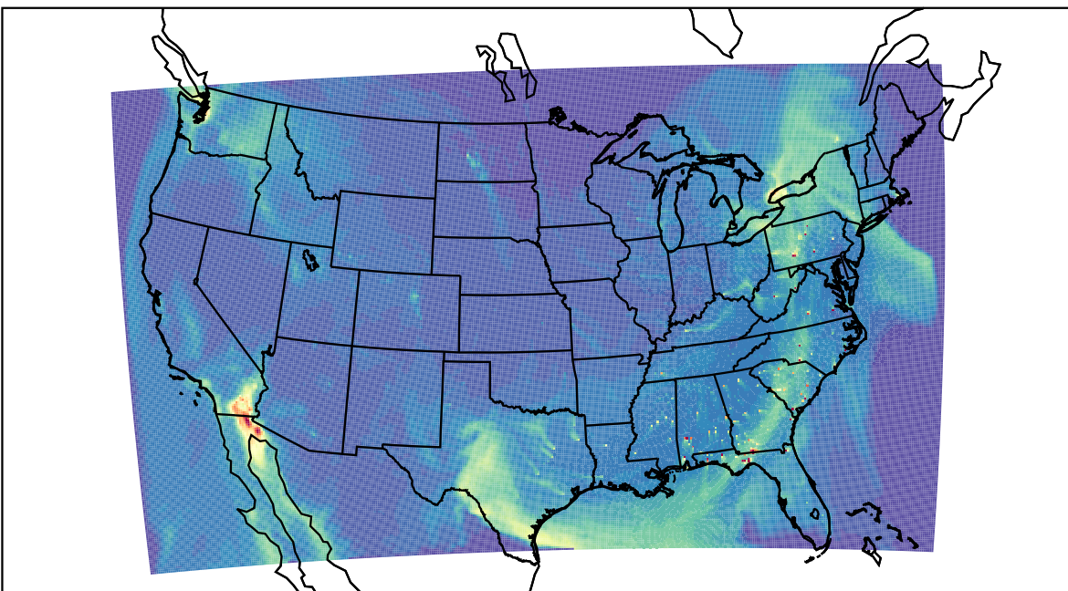
WRF 2023-04-22_18:00:00
