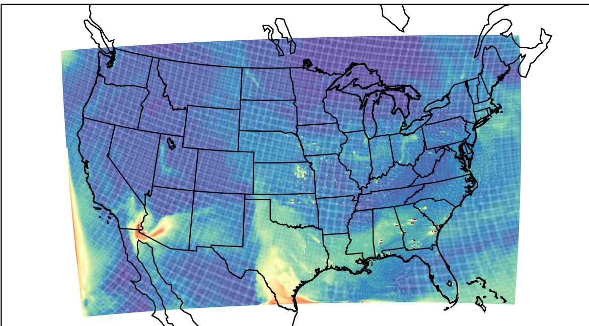
WRF 2023-04-25_20:00:00
