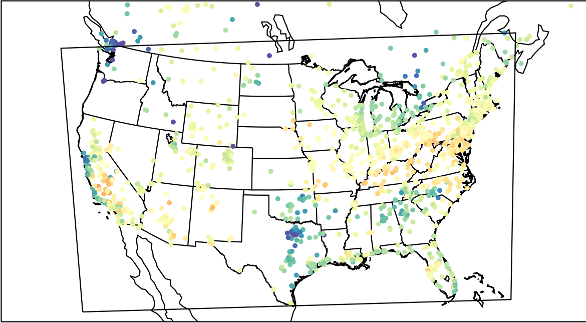
AirNOW (2023-04-26_18:00:00)
