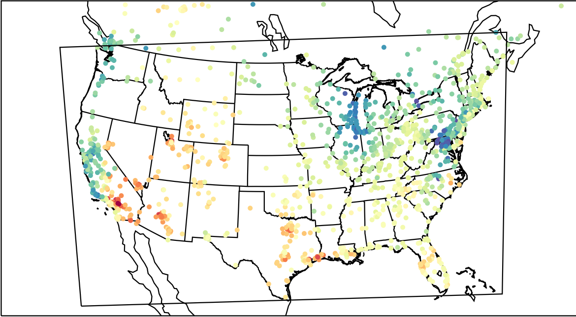
AirNOW (2023-04-30_20:00:00)
