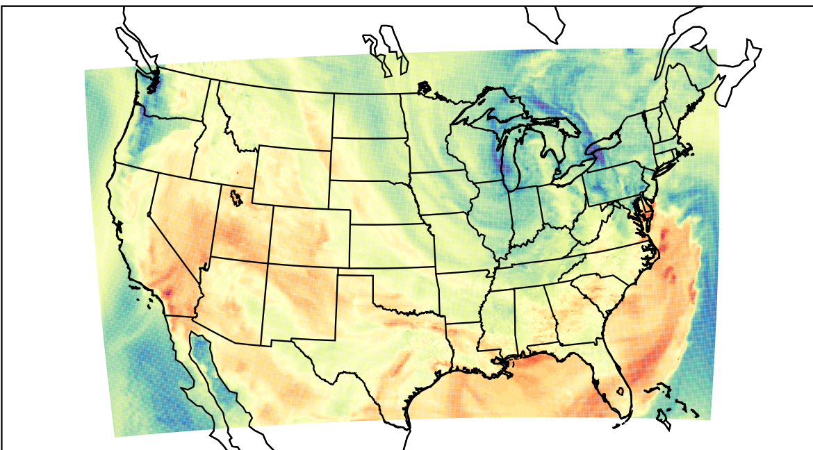
WRF (2023-04-30_23:00:00)
