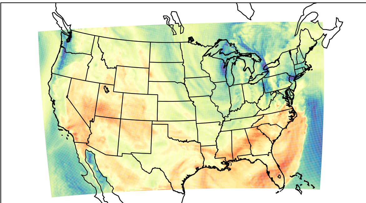
WRF (2023-04-30_20:00:00)
