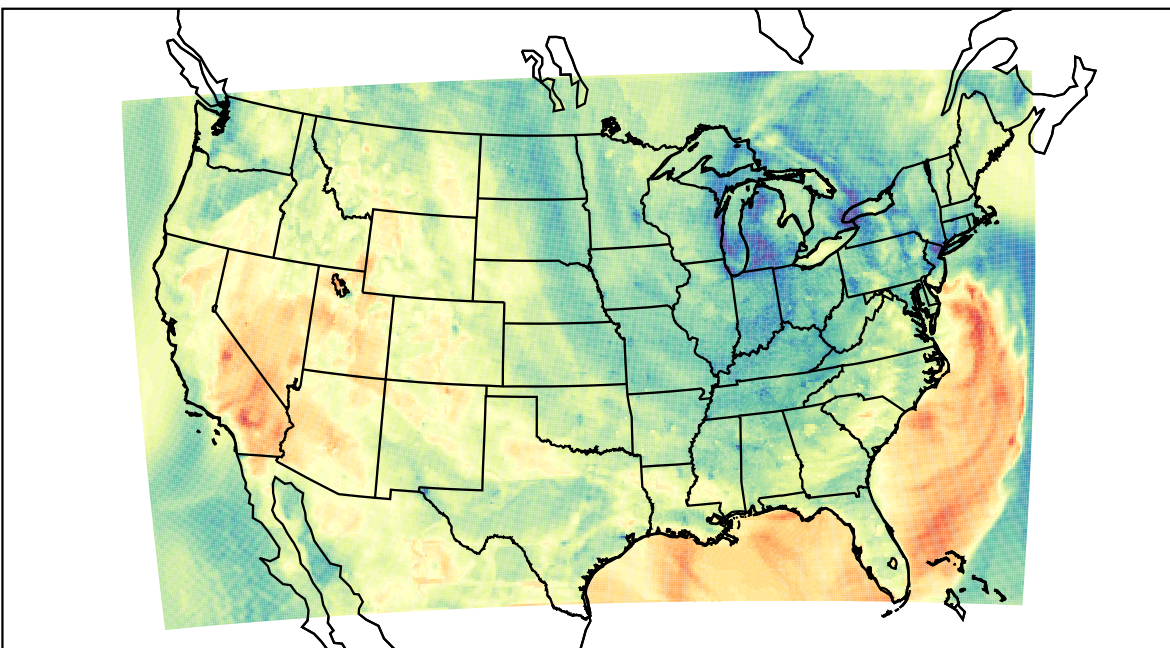
WRF (2023-05-01_01:00:00)
