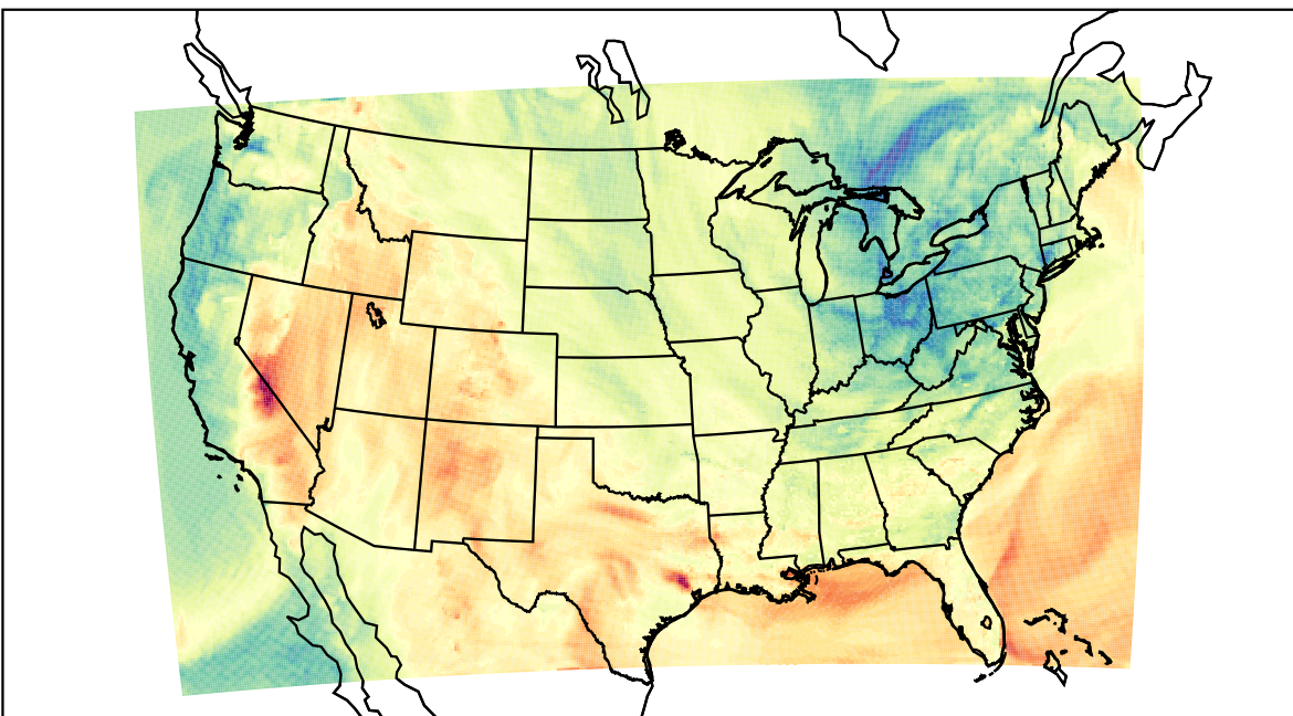
WRF (2023-05-01_23:00:00)
