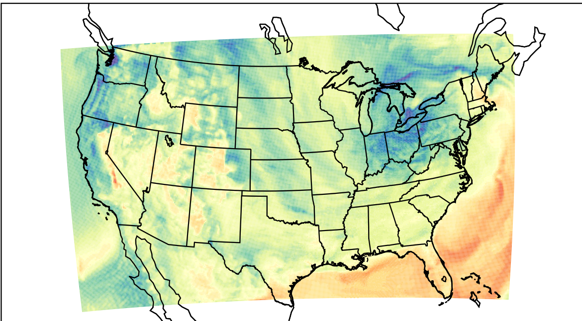
WRF (2023-05-01_16:00:00)
