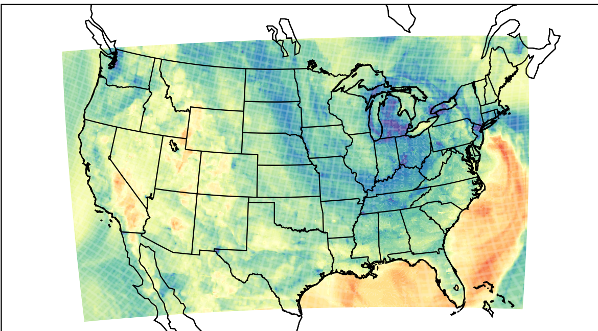
WRF (2023-05-01_03:00:00)
