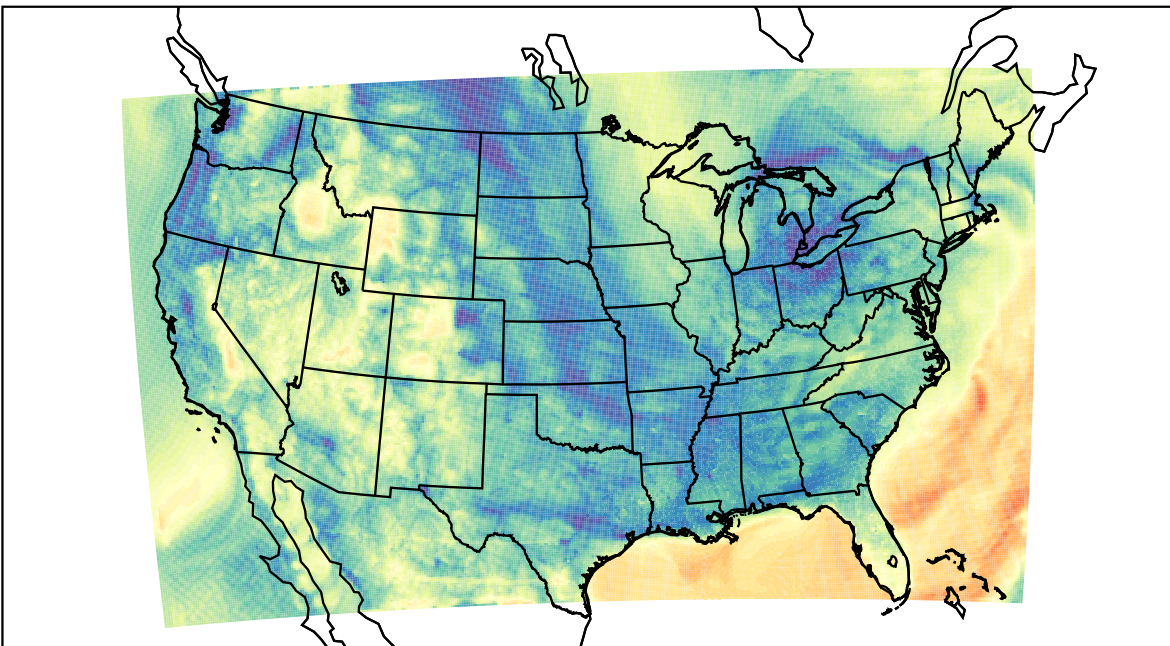
WRF (2023-05-01_13:00:00)
