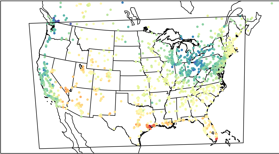
AirNOW (2023-05-01_18:00:00)
