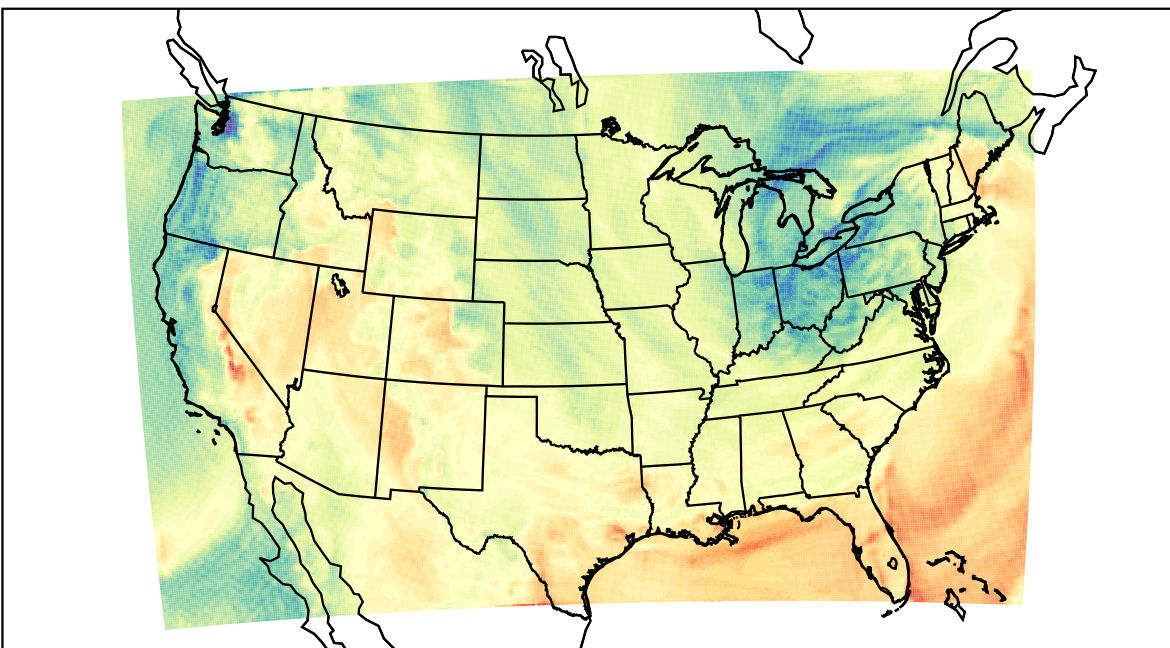
WRF (2023-05-01_18:00:00)
