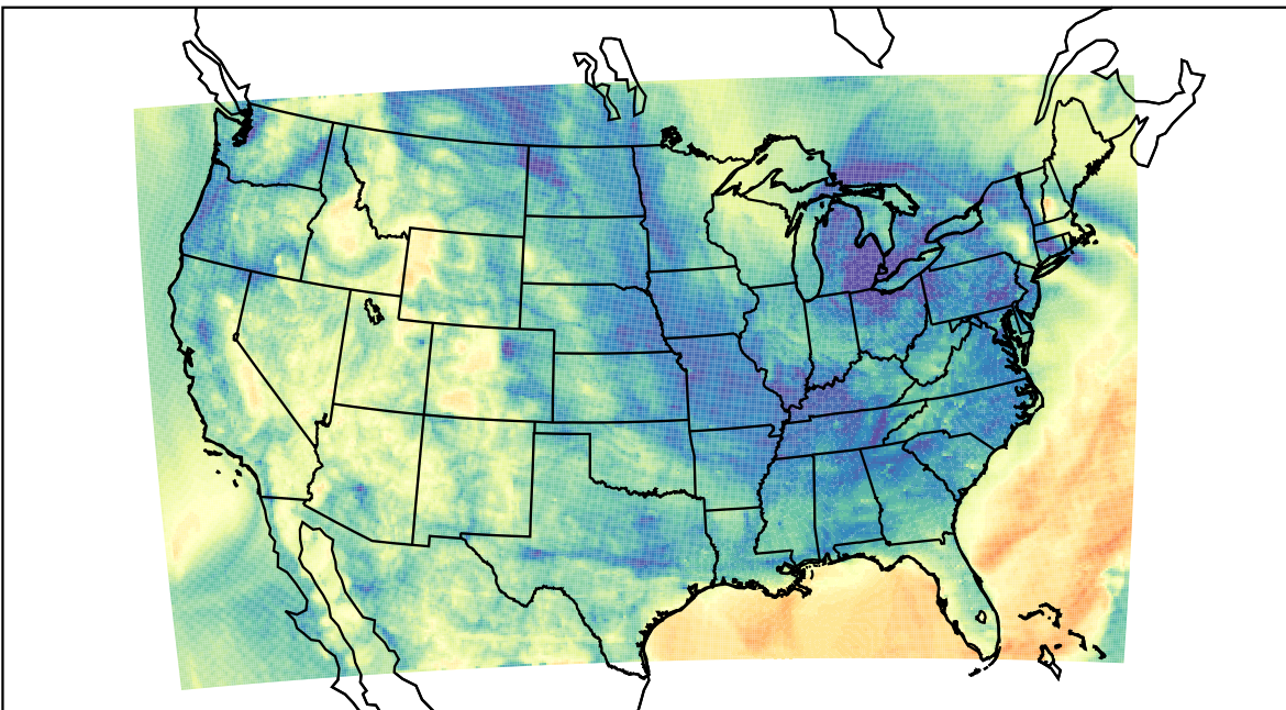
WRF (2023-05-01_10:00:00)
