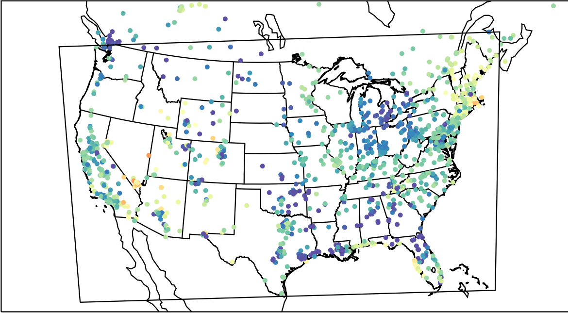
AirNOW (2023-05-01_10:00:00)
