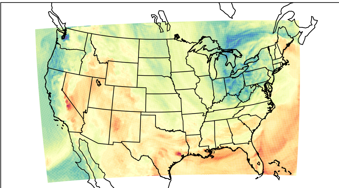
WRF (2023-05-01_20:00:00)
