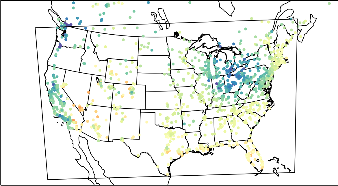
AirNOW (2023-05-01_16:00:00)
