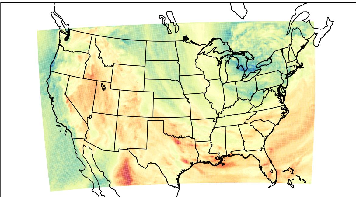
WRF (2023-05-02_20:00:00)
