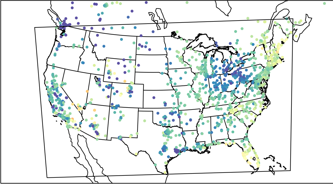
AirNOW (2023-05-01_13:00:00)
