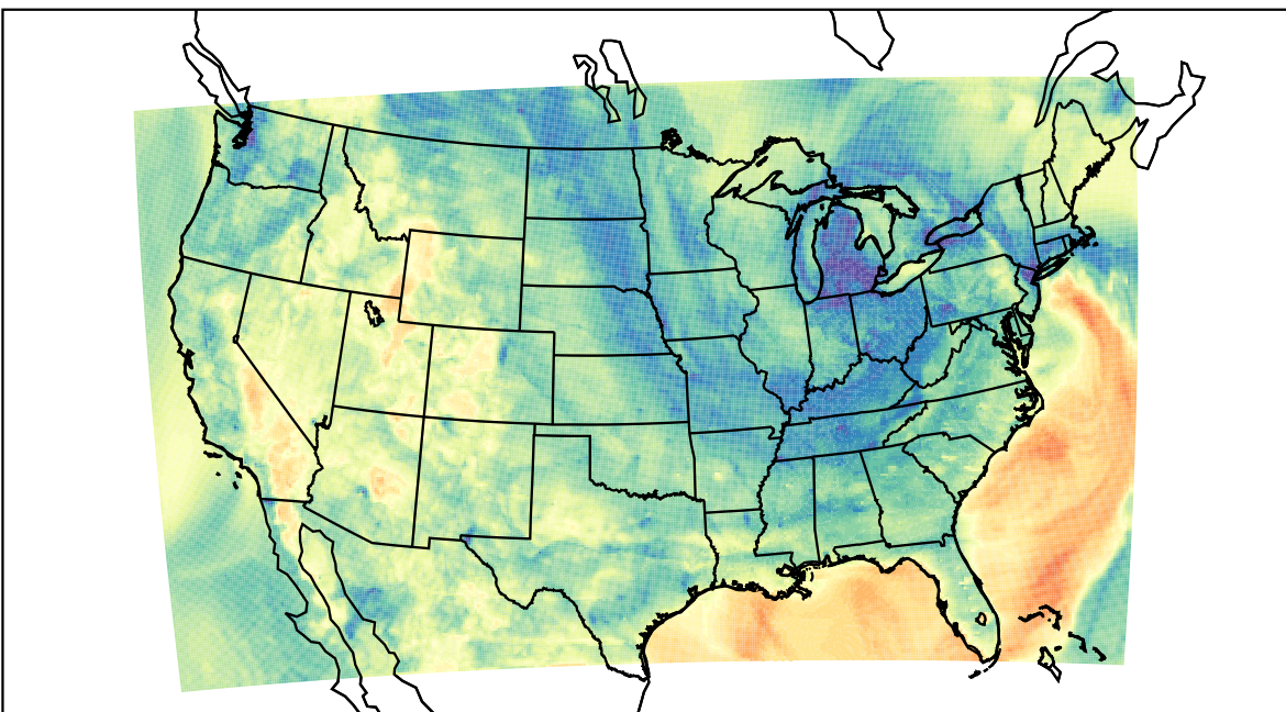
WRF (2023-05-01_04:00:00)
