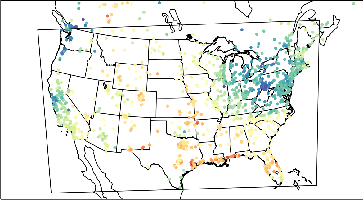
AirNOW (2023-05-03_18:00:00)
