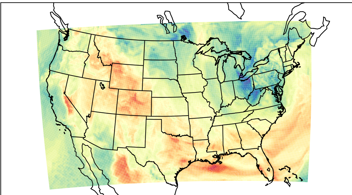
WRF (2023-05-03_18:00:00)
