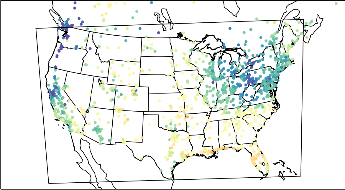
AirNOW (2023-05-03_16:00:00)
