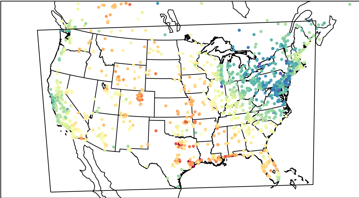
AirNOW (2023-05-03_23:00:00)
