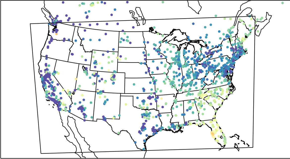
AirNOW (2023-05-03_13:00:00)
