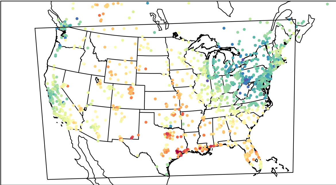
AirNOW (2023-05-03_20:00:00)
