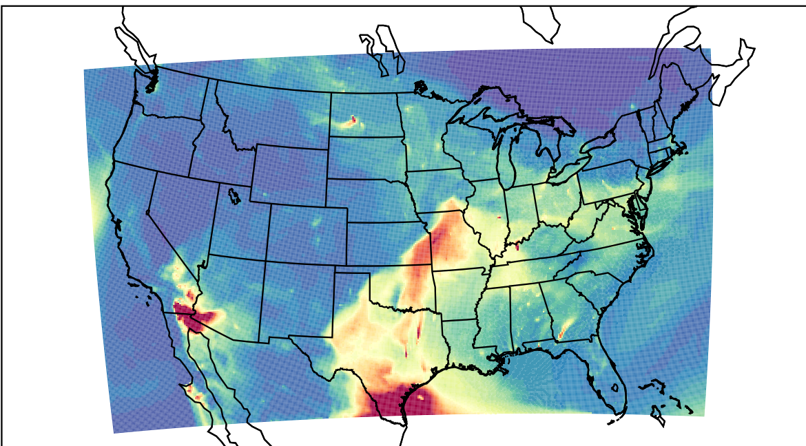
WRF 2023-05-08_11:00:00
