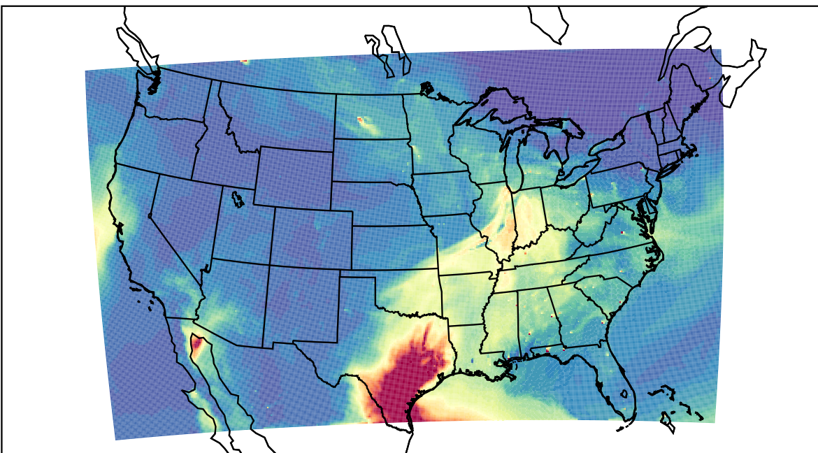
WRF 2023-05-08_20:00:00
