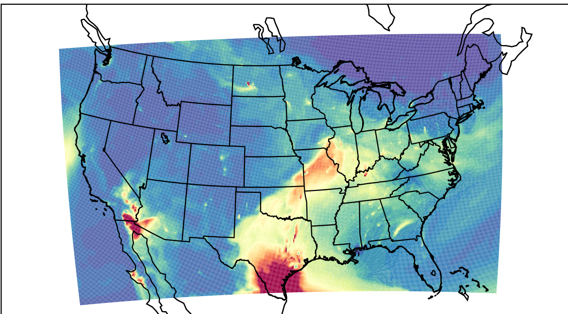
WRF 2023-05-08_14:00:00
