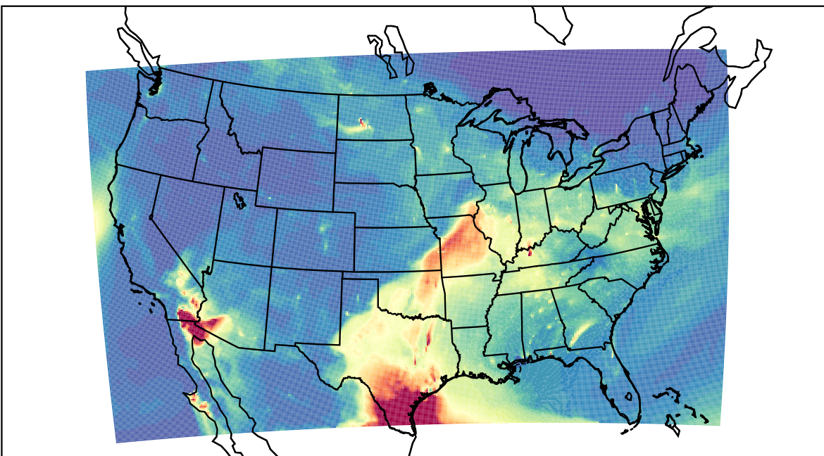
WRF 2023-05-08_13:00:00
