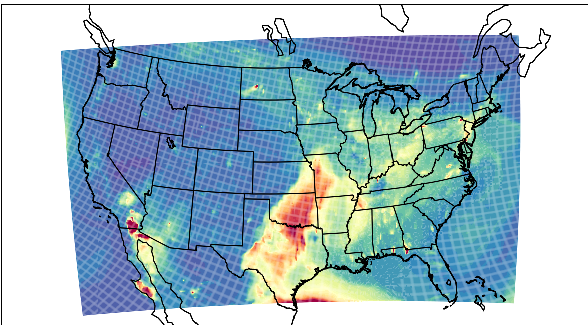
WRF 2023-05-08_03:00:00
