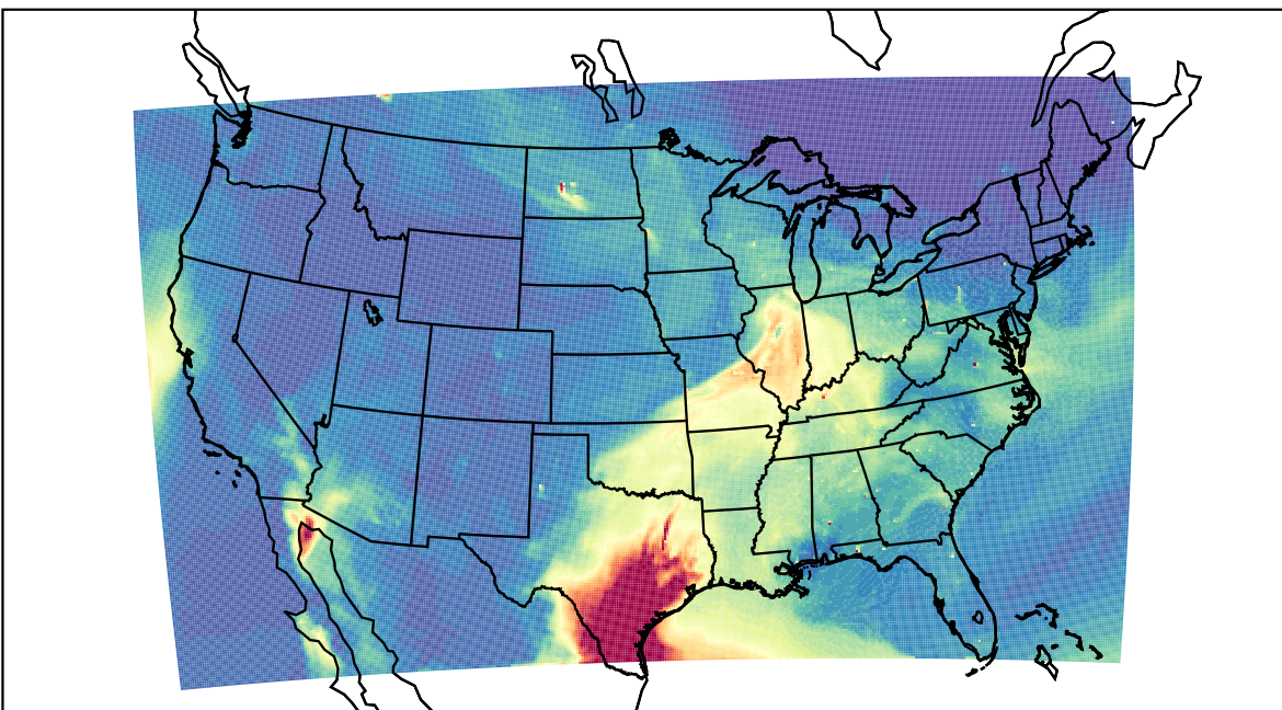
WRF 2023-05-08_18:00:00
