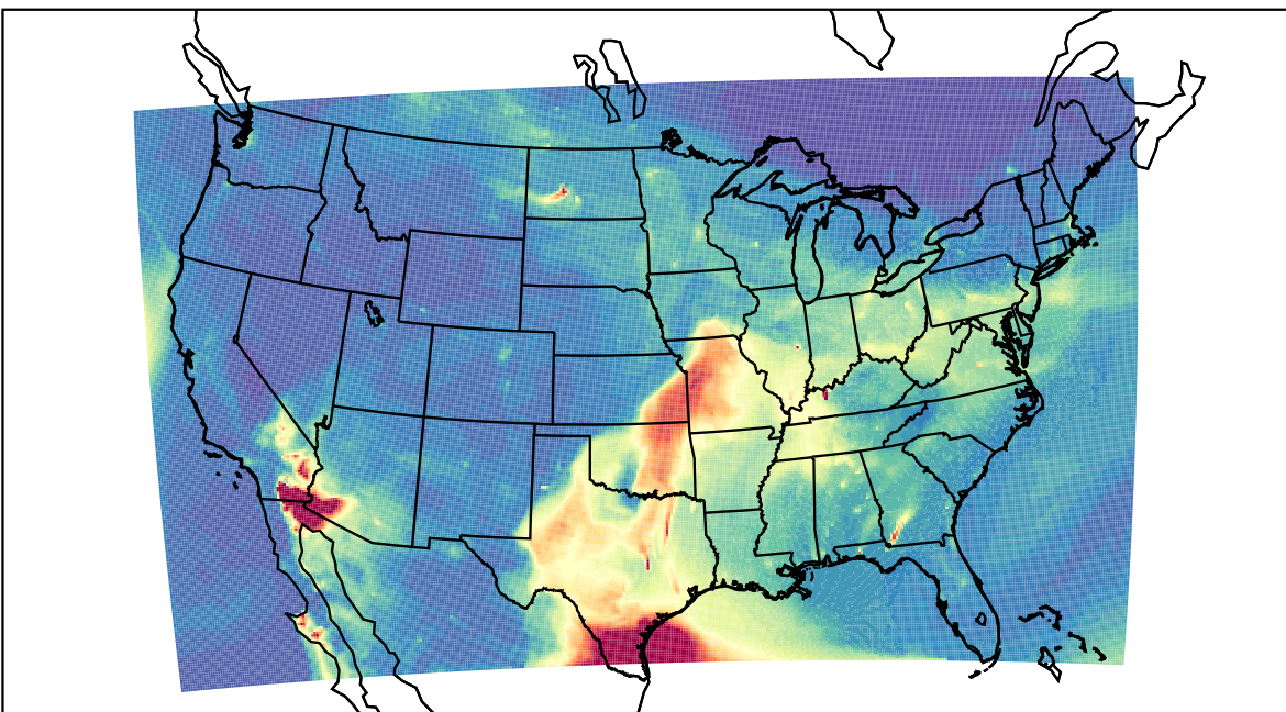
WRF 2023-05-08_10:00:00
