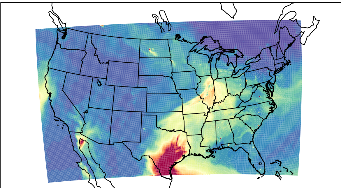
WRF 2023-05-08_19:00:00
