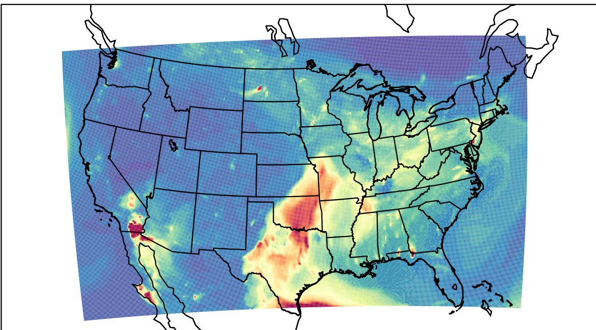
WRF 2023-05-08_04:00:00
