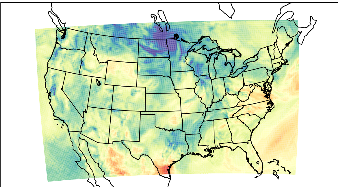
WRF (2023-05-08_16:00:00)
