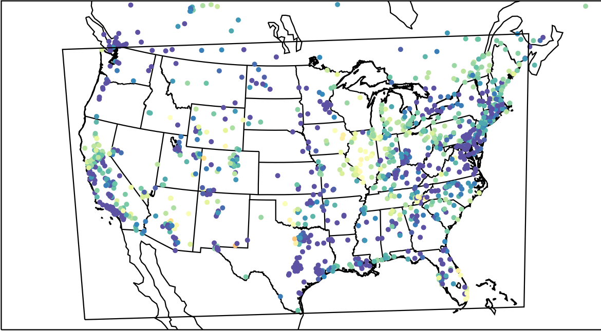
AirNOW (2023-05-08_10:00:00)
