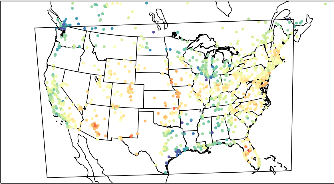
AirNOW (2023-05-08_20:00:00)
