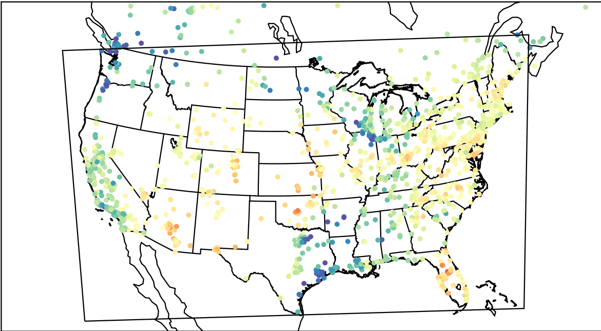
AirNOW (2023-05-08_18:00:00)
