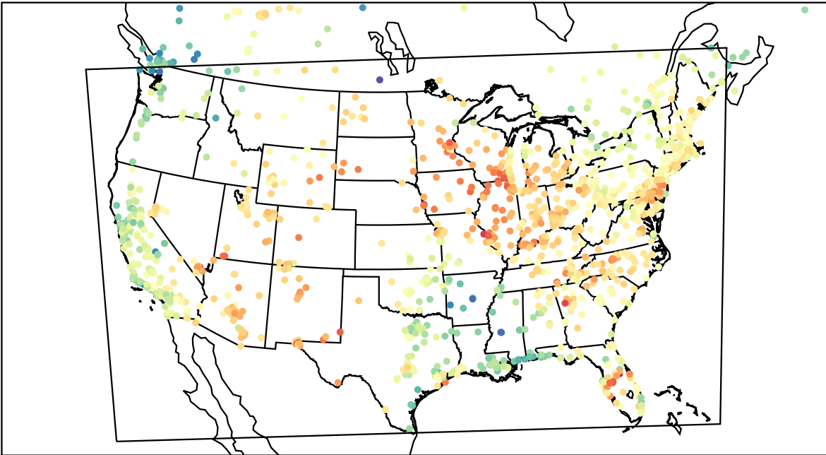
AirNOW (2023-05-10_20:00:00)
