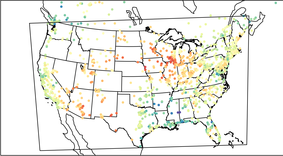
AirNOW (2023-05-10_23:00:00)
