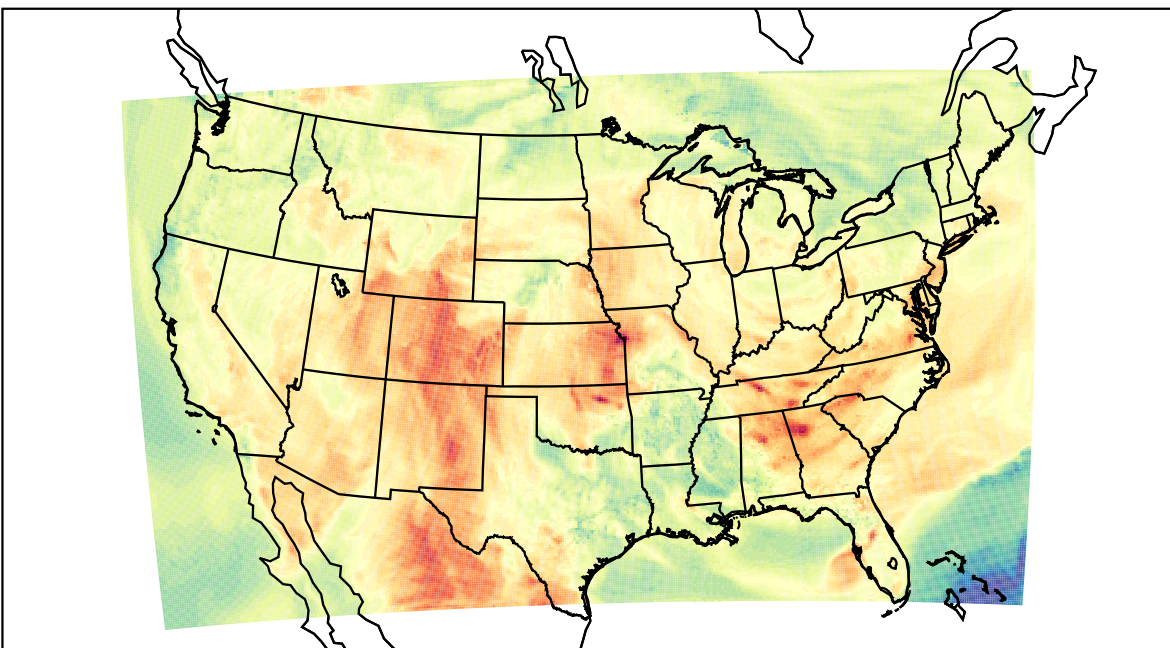
WRF (2023-05-10_20:00:00)
