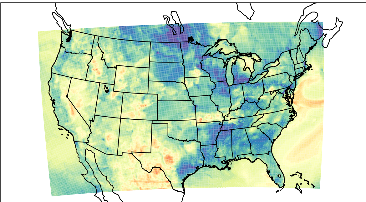
WRF (2023-05-09_04:00:00)
