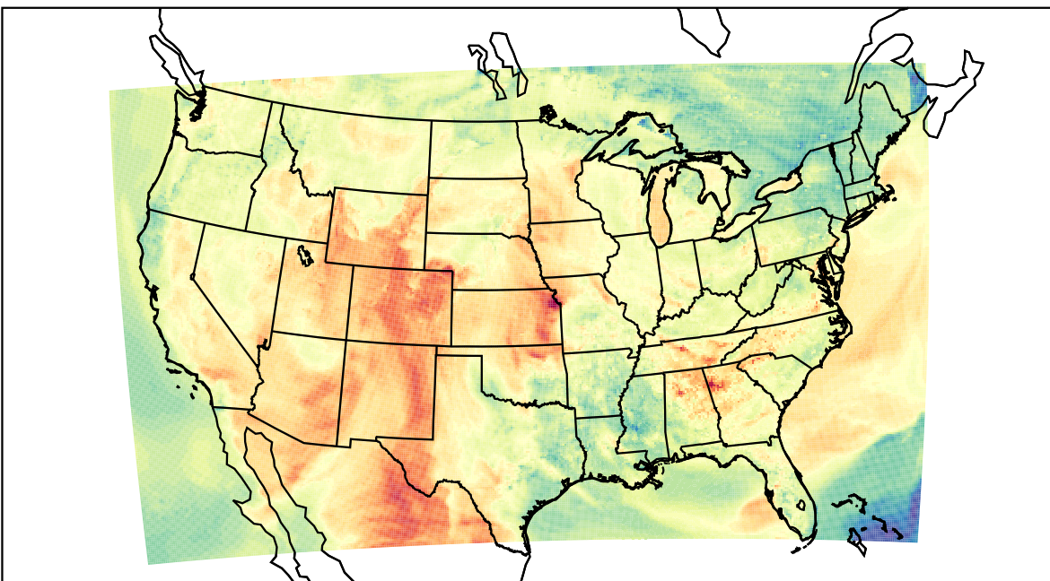
WRF (2023-05-10_23:00:00)
