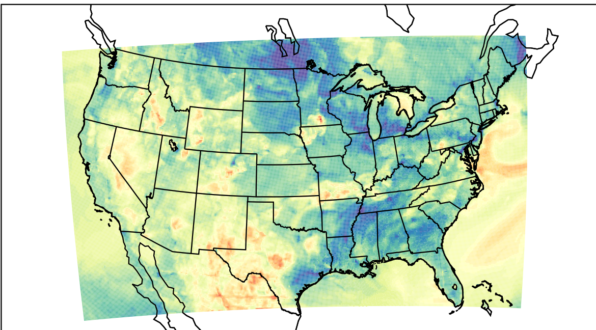
WRF (2023-05-09_03:00:00)
