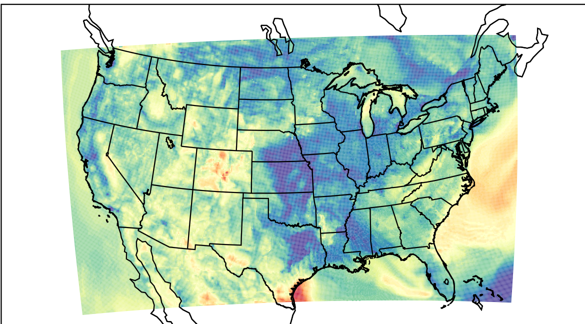
WRF (2023-05-11_13:00:00)
