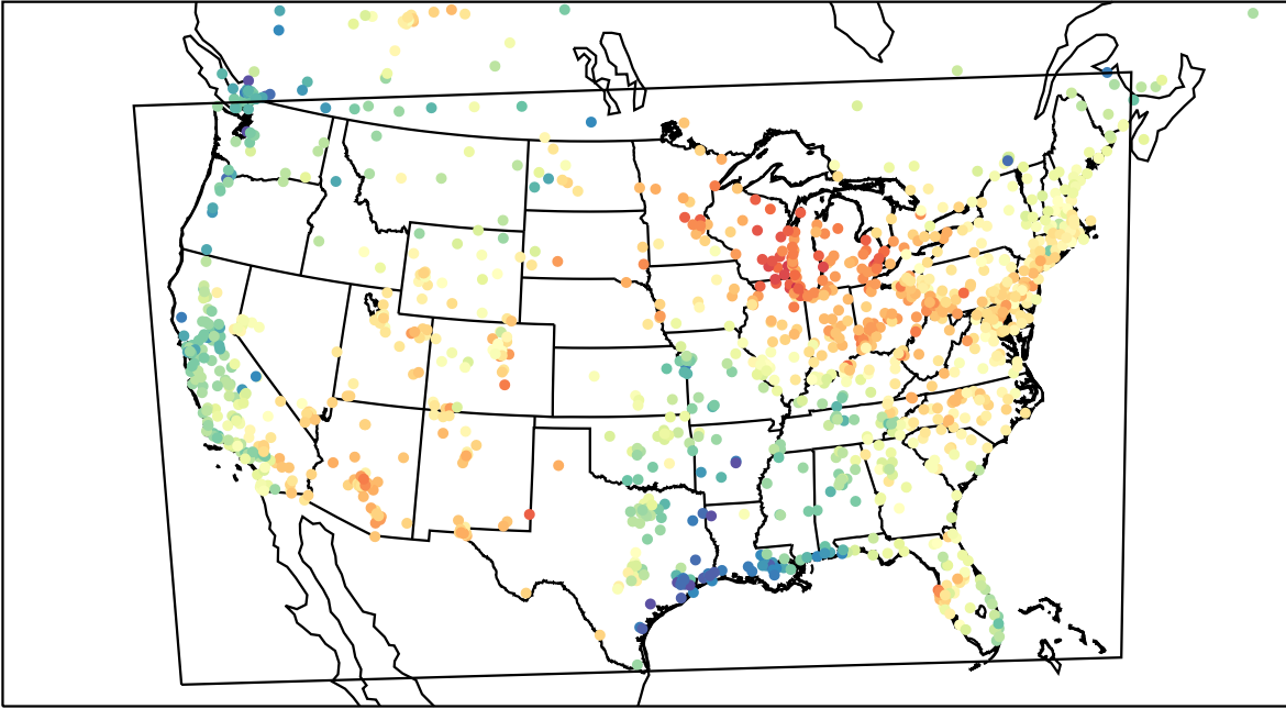
AirNOW (2023-05-11_18:00:00)
