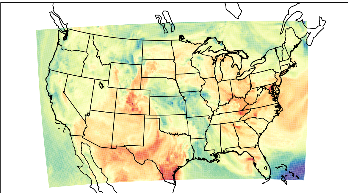
WRF (2023-05-11_18:00:00)
