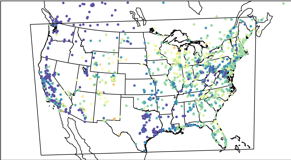
AirNOW (2023-05-11_13:00:00)
