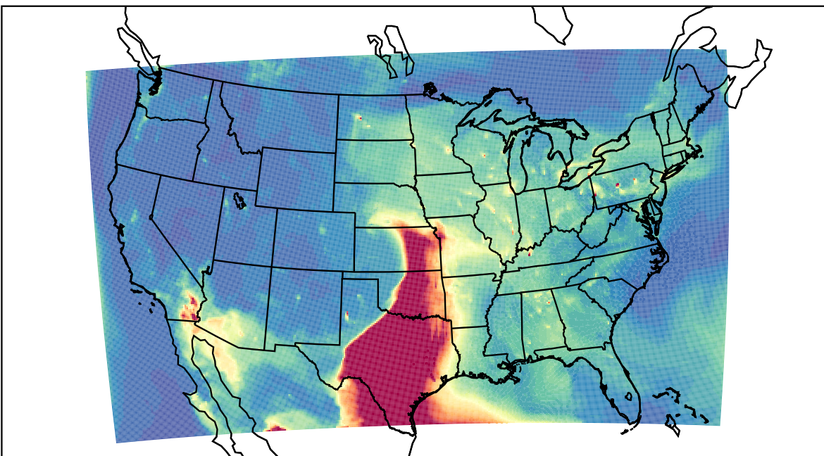
WRF 2023-05-12_14:00:00
