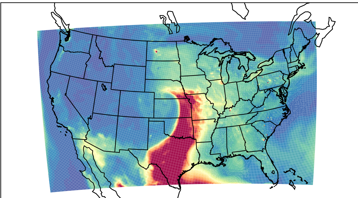
WRF 2023-05-12_18:00:00
