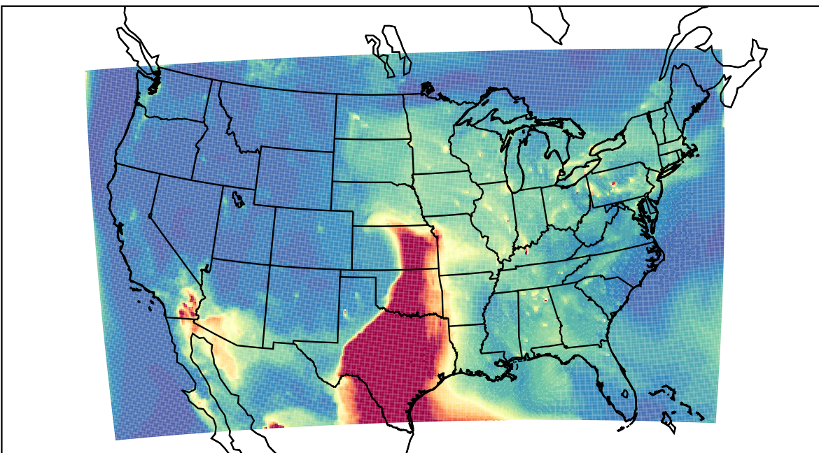
WRF 2023-05-12_13:00:00
