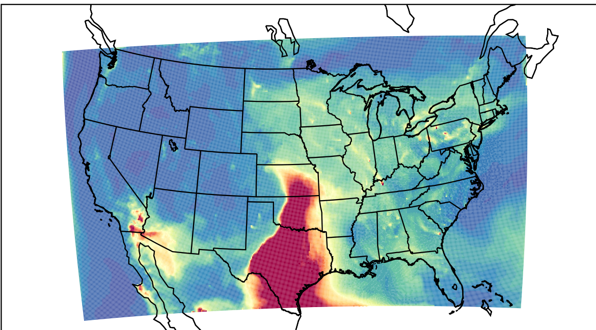
WRF 2023-05-12_10:00:00
