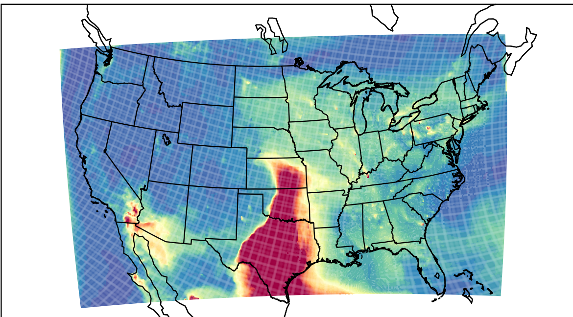
WRF 2023-05-12_11:00:00
