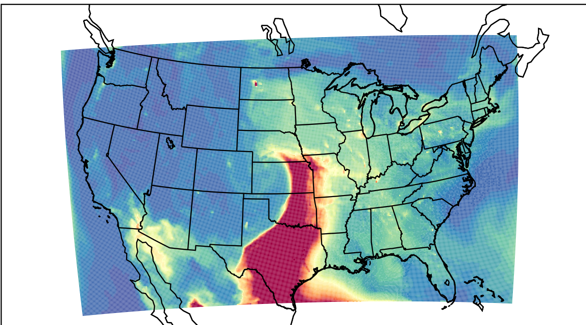
WRF 2023-05-12_16:00:00
