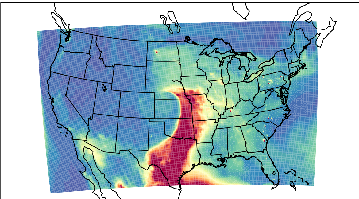
WRF 2023-05-12_19:00:00
