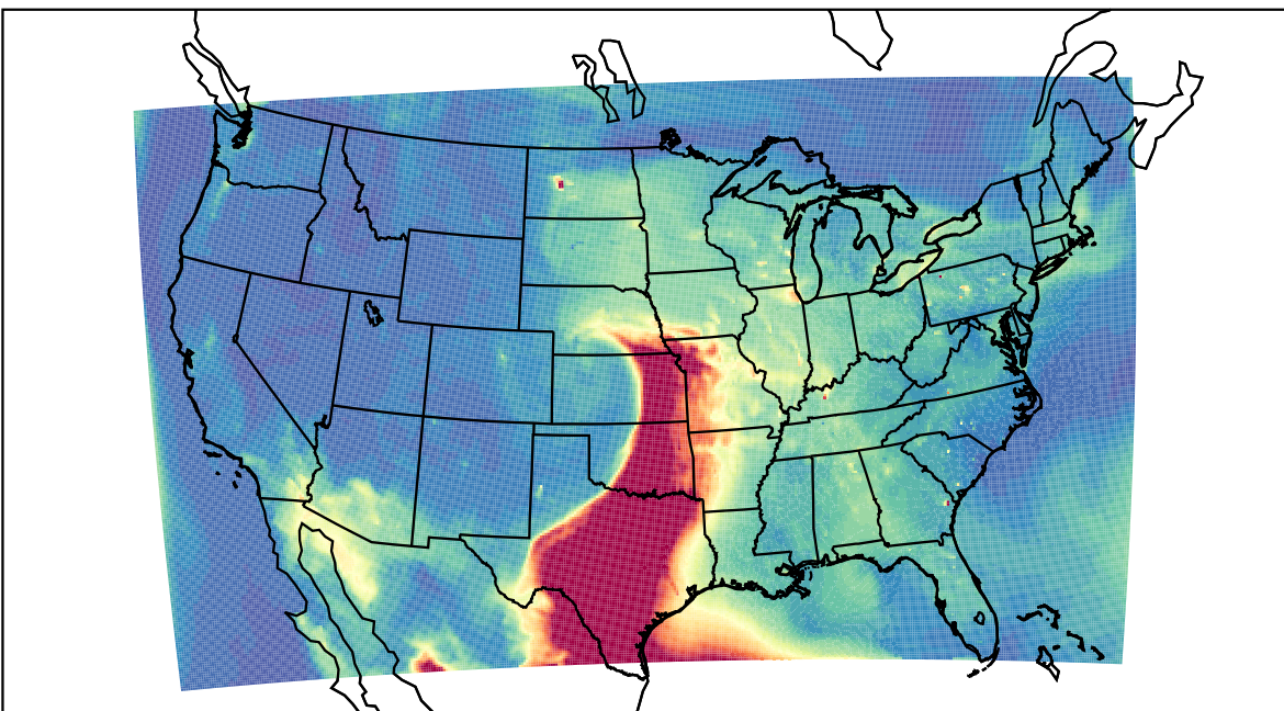
WRF 2023-05-12_17:00:00
