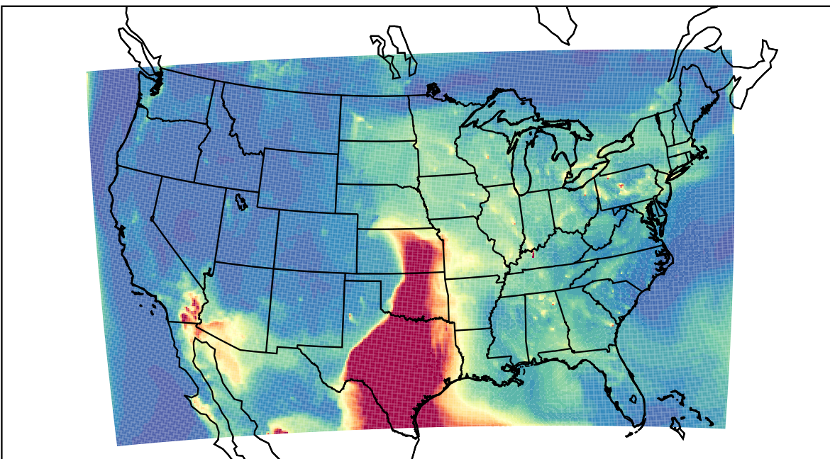
WRF 2023-05-12_12:00:00
