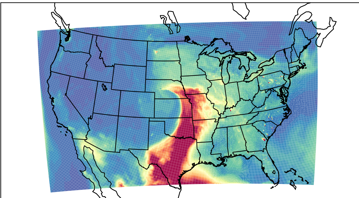
WRF 2023-05-12_20:00:00
