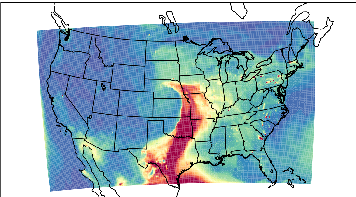
WRF 2023-05-12_23:00:00
