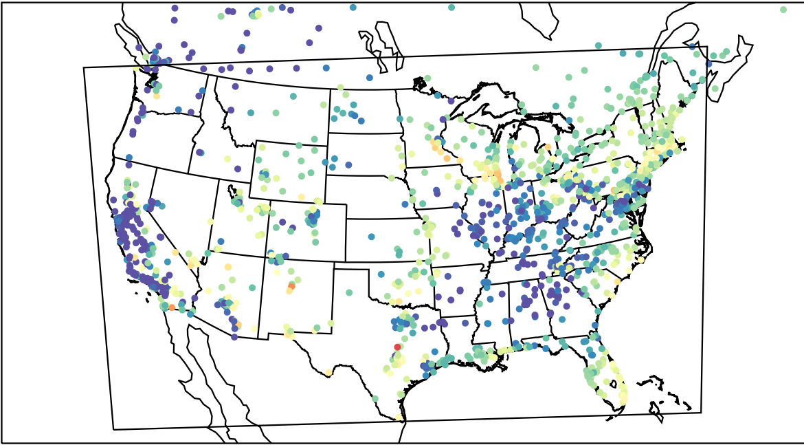
AirNOW (2023-05-13_13:00:00)
