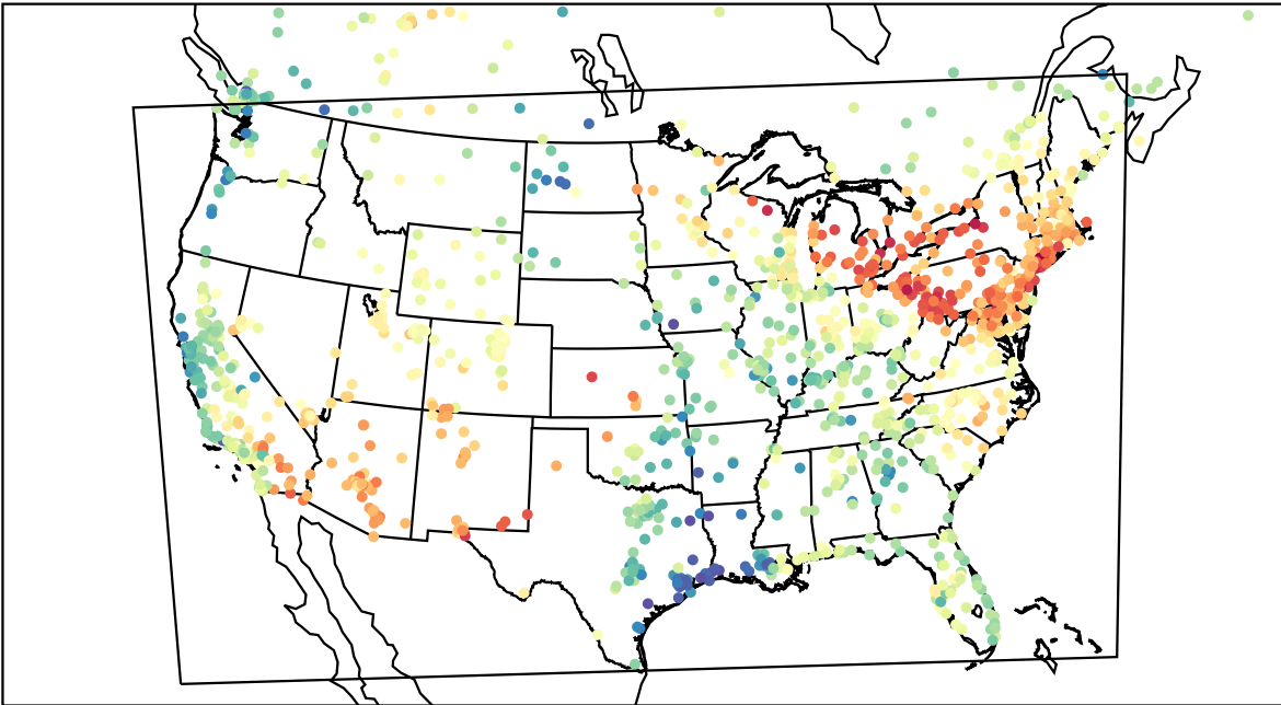
AirNOW (2023-05-12_18:00:00)
