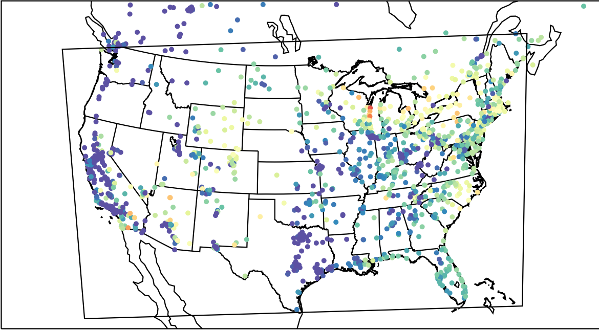
AirNOW (2023-05-12_13:00:00)
