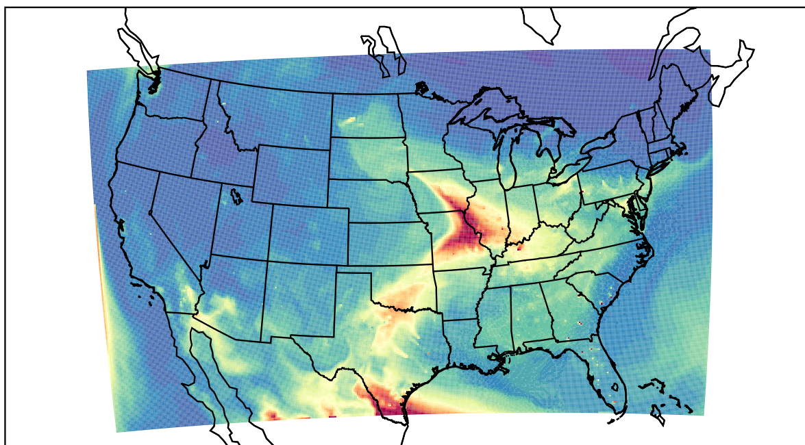
WRF 2023-05-13_19:00:00
