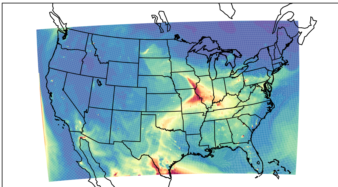
WRF 2023-05-13_22:00:00
