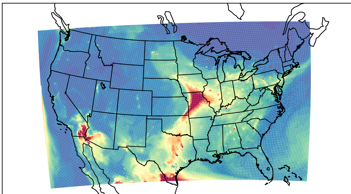
WRF 2023-05-13_14:00:00
