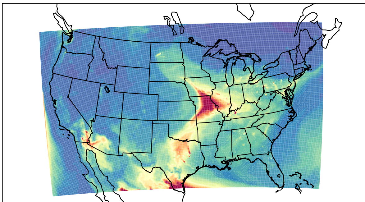
WRF 2023-05-13_16:00:00
