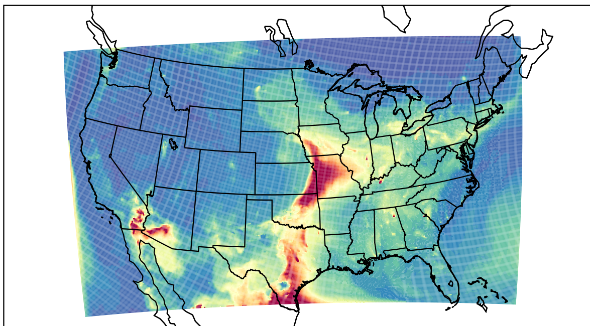
WRF 2023-05-13_10:00:00
