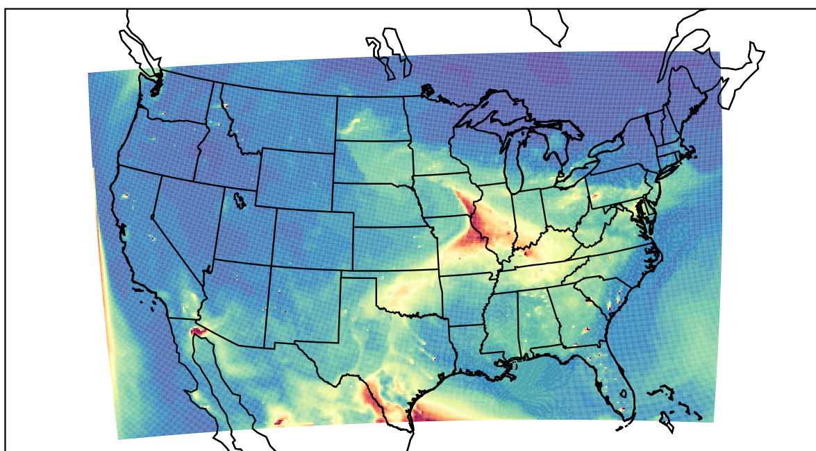
WRF 2023-05-13_23:00:00
