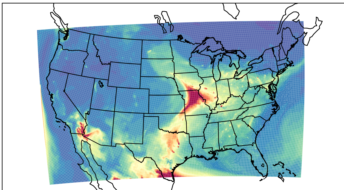
WRF 2023-05-13_15:00:00
