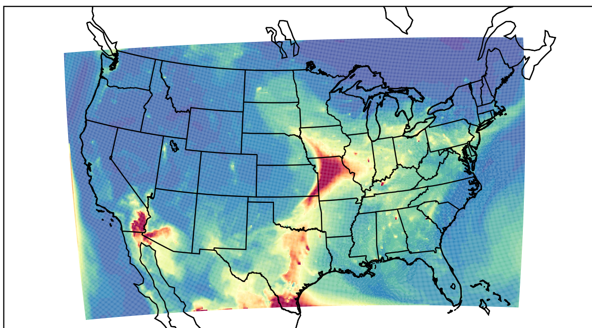
WRF 2023-05-13_13:00:00
