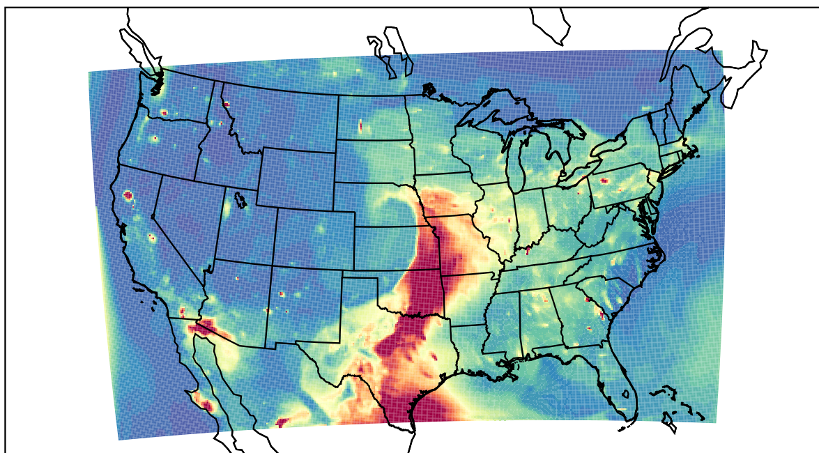
WRF 2023-05-13_03:00:00
