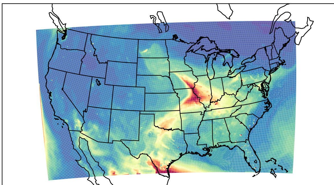
WRF 2023-05-13_20:00:00
