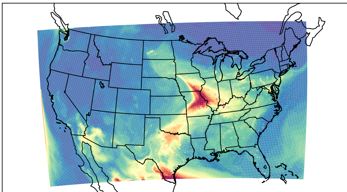
WRF 2023-05-13_18:00:00
