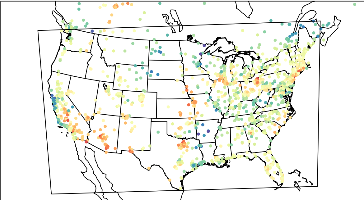
AirNOW (2023-05-13_18:00:00)
