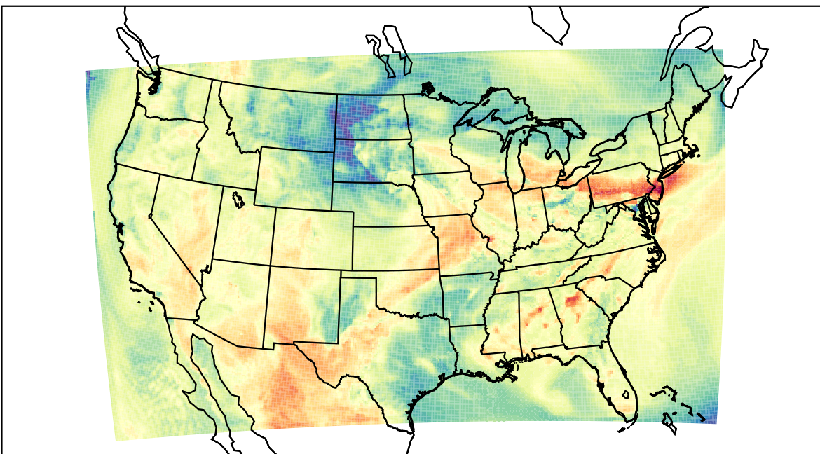
WRF (2023-05-13_18:00:00)
