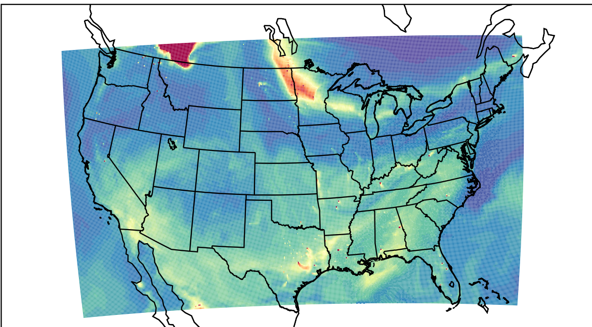
WRF 2023-05-16_20:00:00
