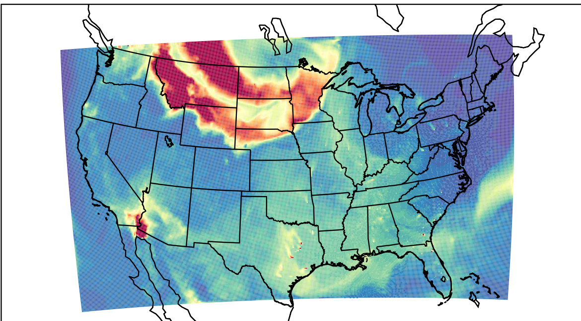
WRF 2023-05-18_18:00:00
