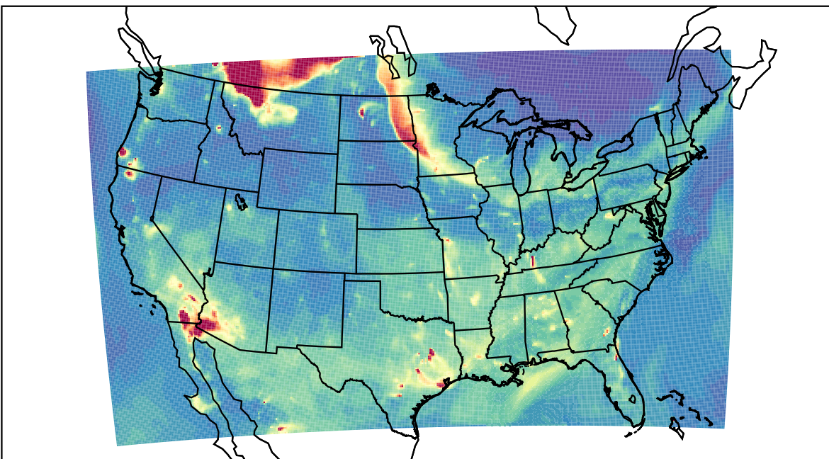
WRF 2023-05-17_04:00:00
