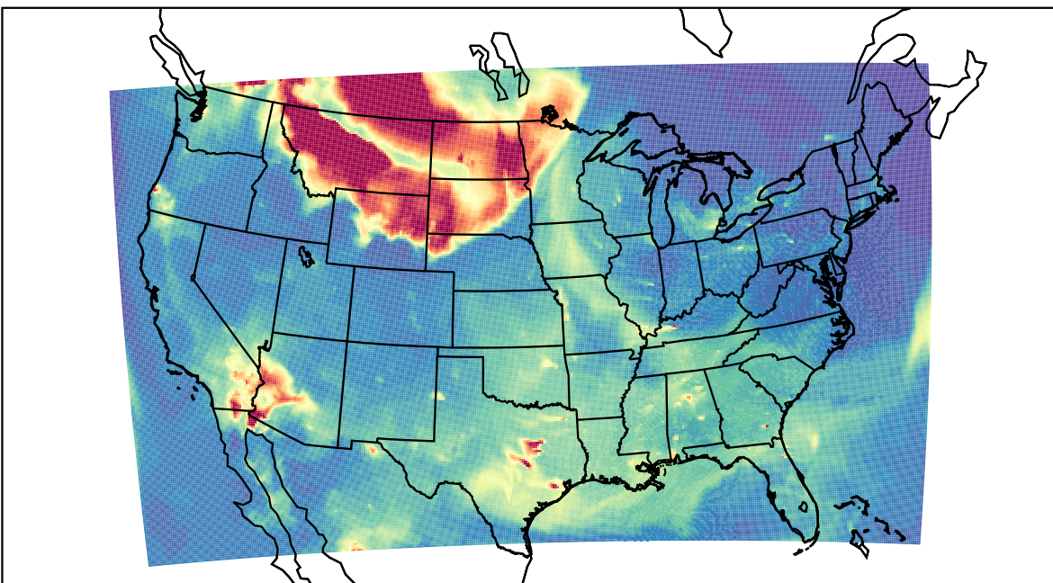
WRF 2023-05-18_10:00:00
