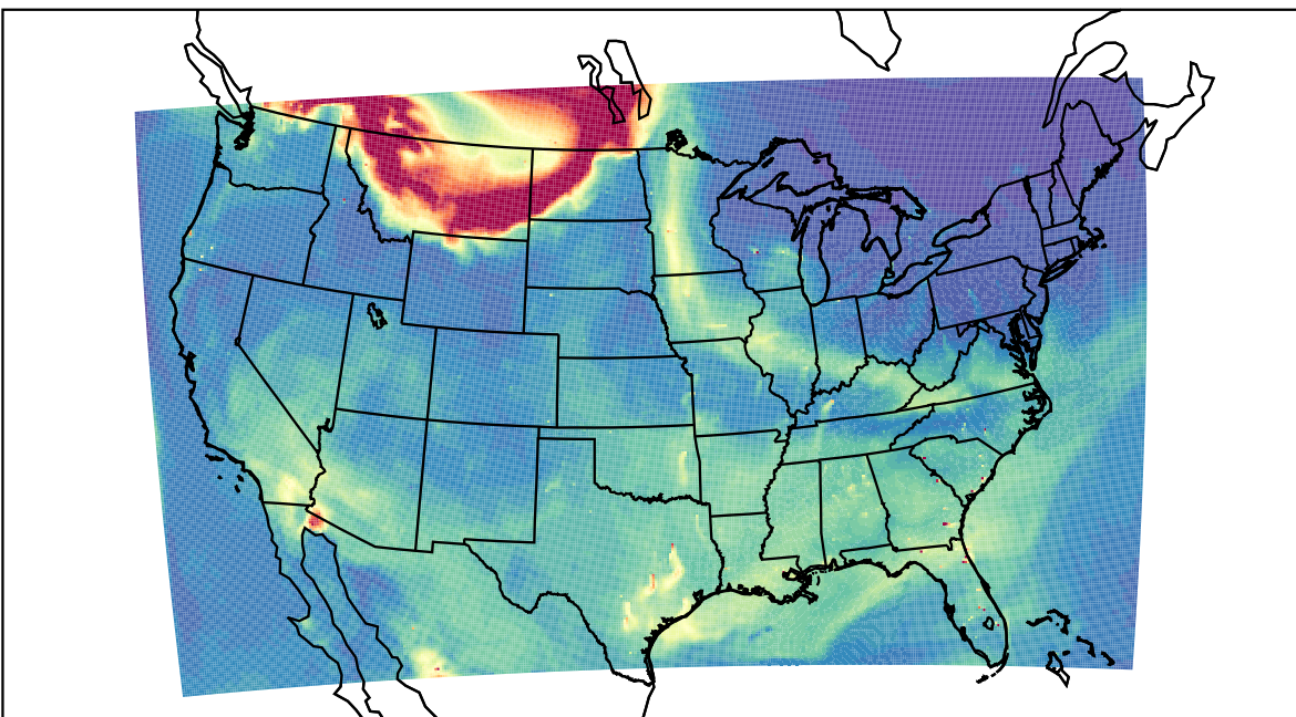
WRF 2023-05-17_20:00:00
