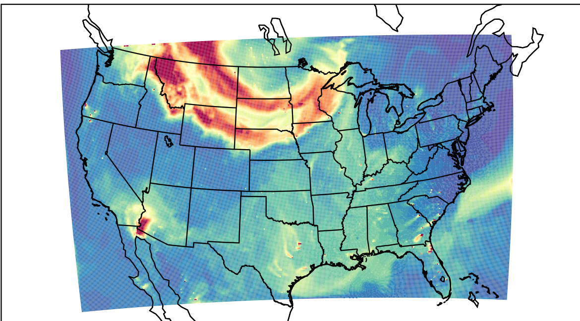
WRF 2023-05-18_23:00:00
