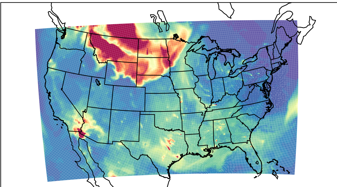
WRF 2023-05-18_13:00:00
