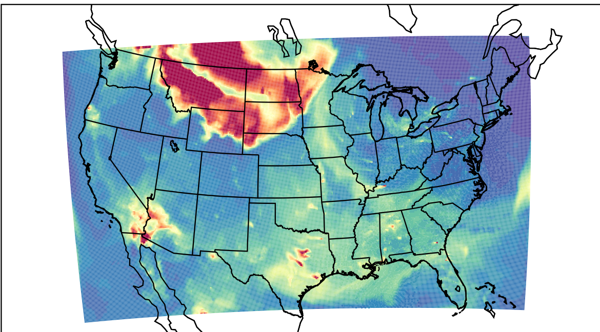
WRF 2023-05-18_11:00:00
