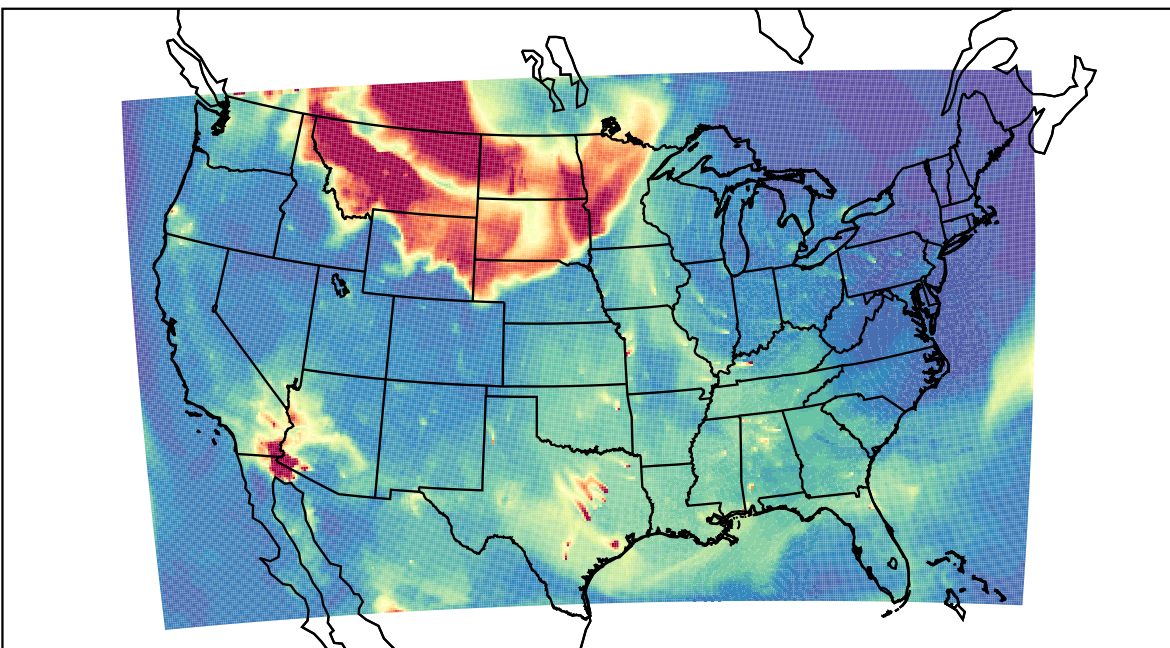
WRF 2023-05-18_14:00:00
