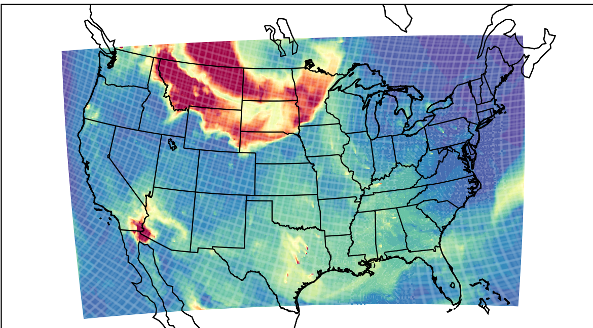
WRF 2023-05-18_16:00:00
