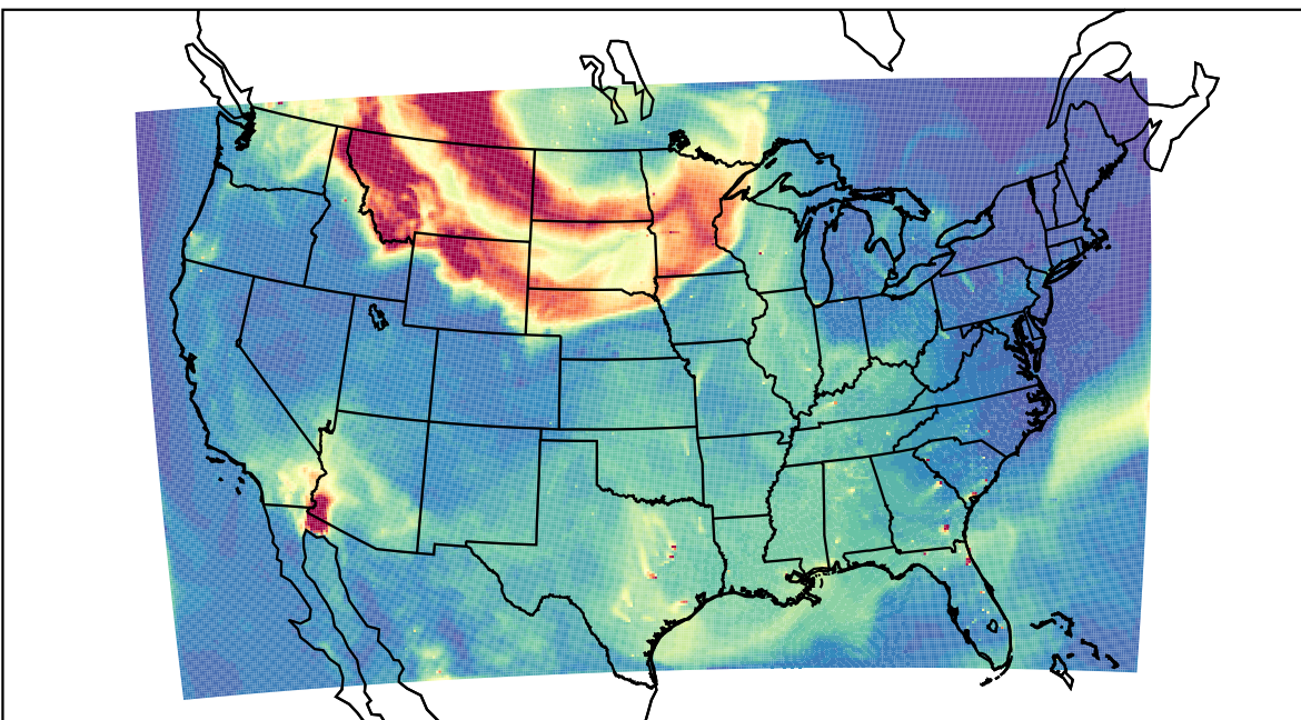
WRF 2023-05-18_20:00:00
