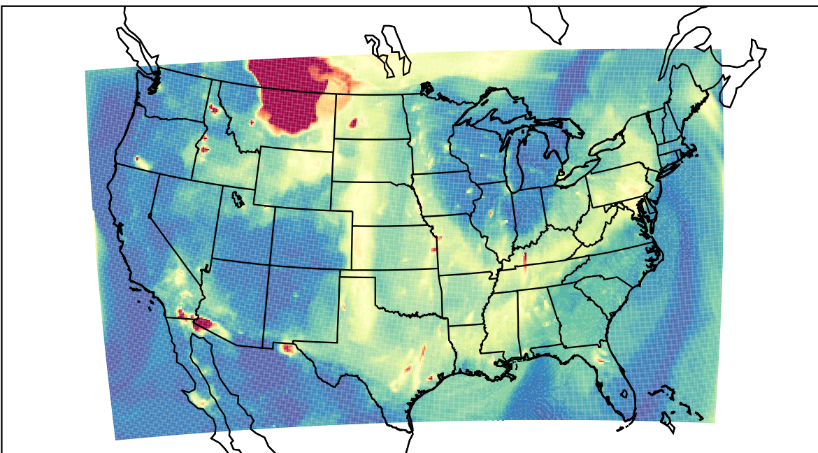
WRF 2023-05-21_04:00:00
