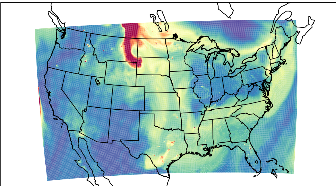
WRF 2023-05-21_22:00:00
