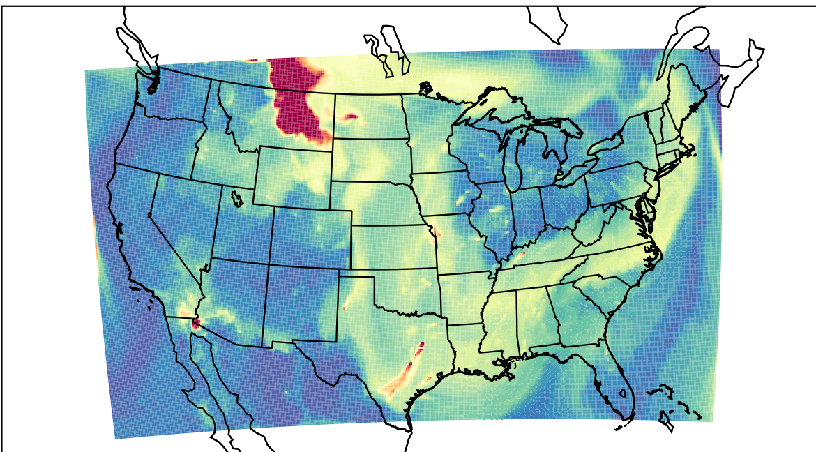
WRF 2023-05-21_14:00:00
