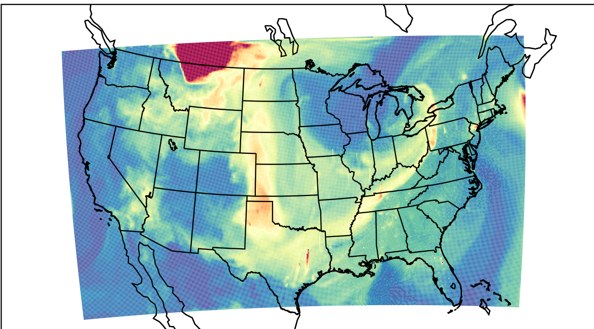
WRF 2023-05-20_18:00:00
