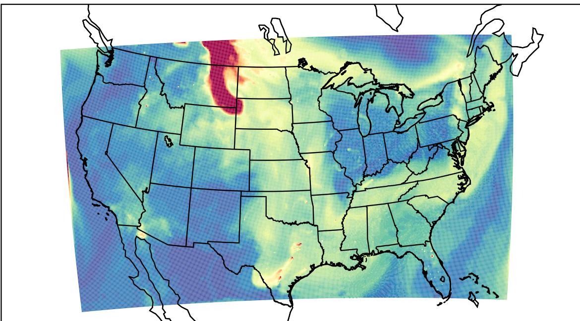
WRF 2023-05-21_19:00:00
