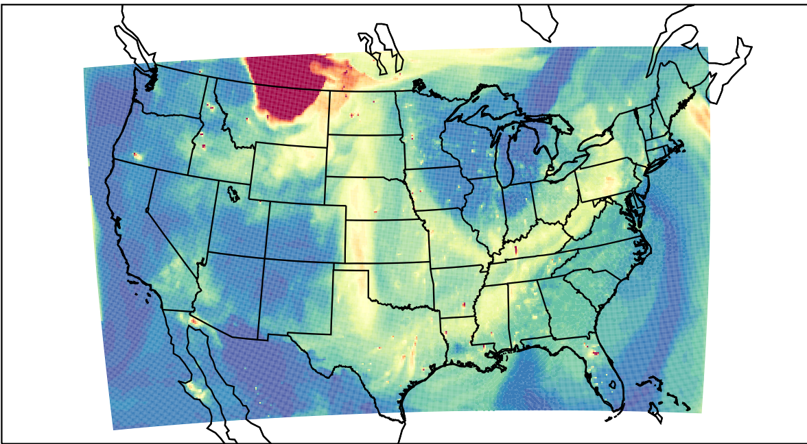
WRF 2023-05-21_01:00:00
