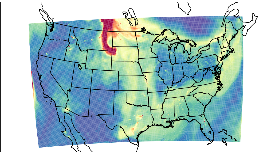
WRF 2023-05-21_23:00:00
