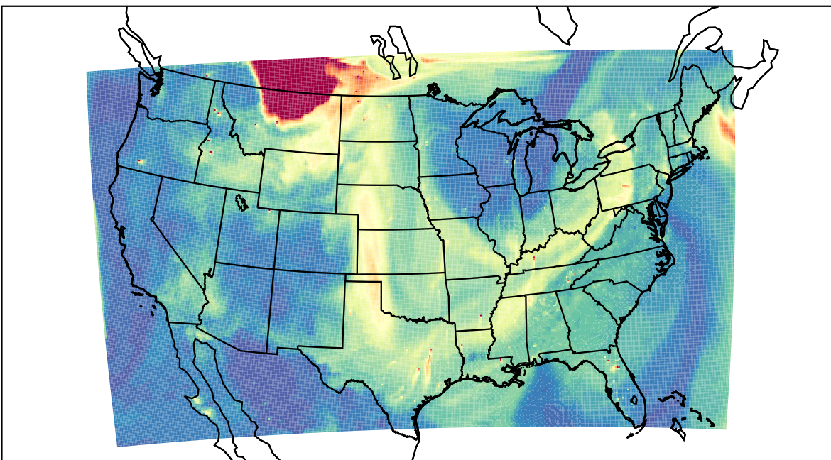
WRF 2023-05-20_23:00:00
