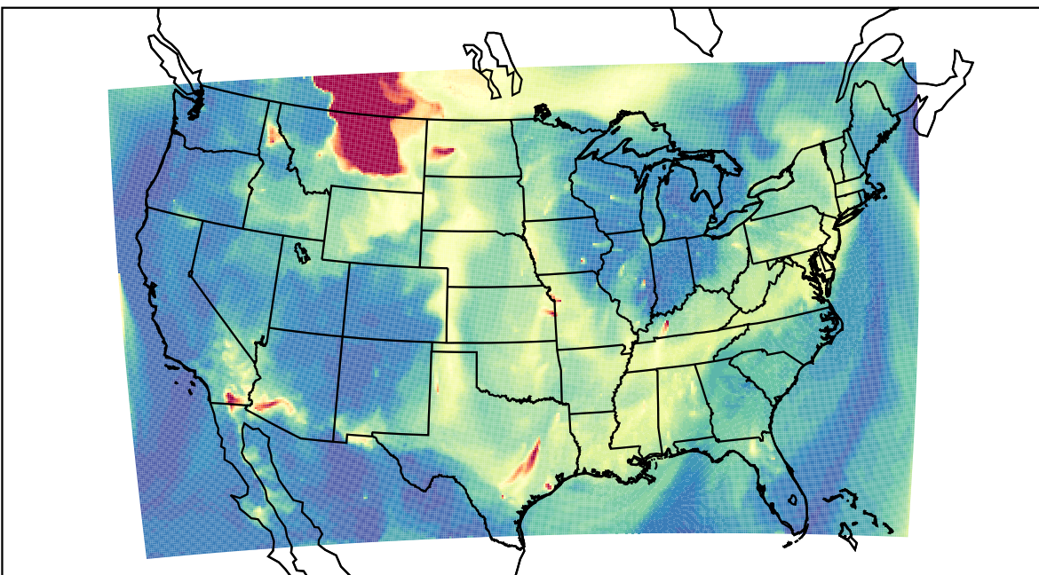
WRF 2023-05-21_08:00:00
