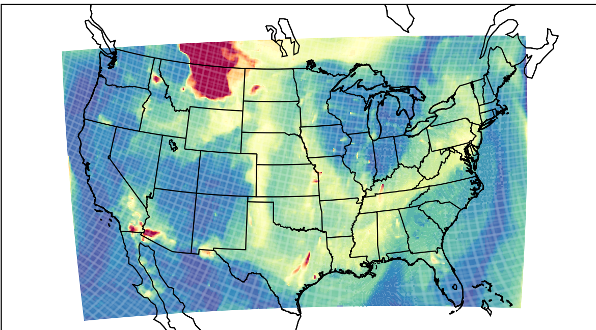
WRF 2023-05-21_06:00:00
