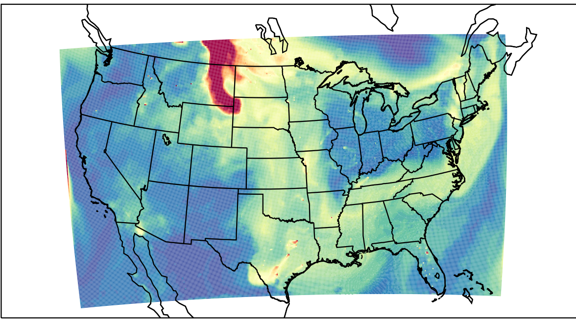
WRF 2023-05-21_20:00:00
