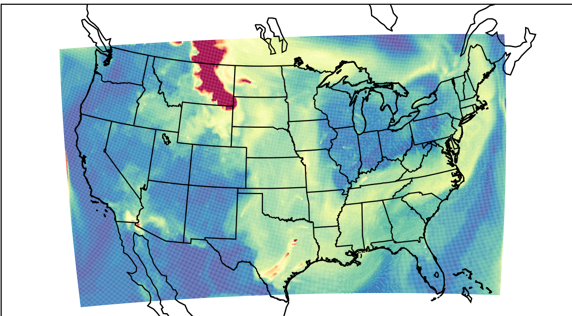
WRF 2023-05-21_16:00:00
