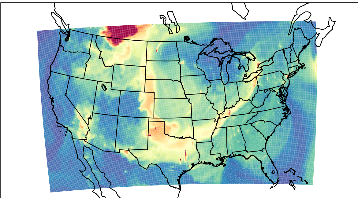
WRF 2023-05-20_14:00:00
