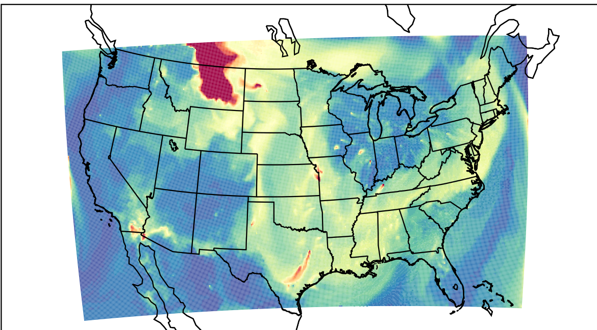
WRF 2023-05-21_12:00:00
