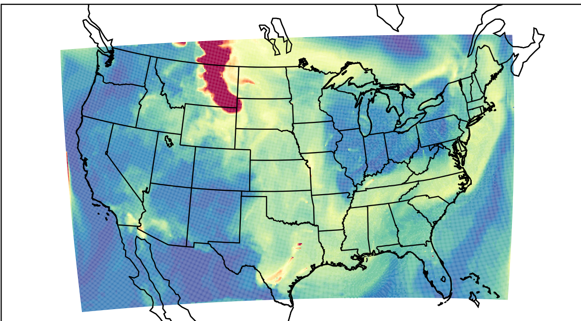
WRF 2023-05-21_17:00:00
