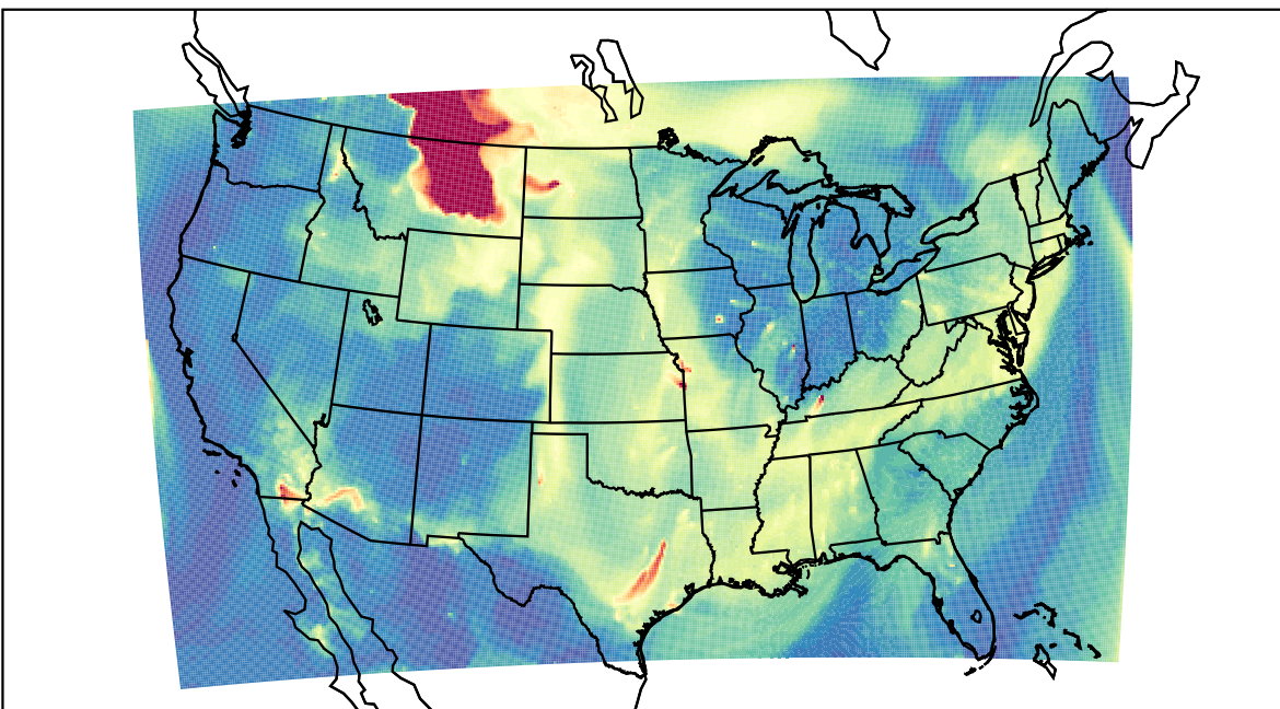
WRF 2023-05-21_10:00:00
