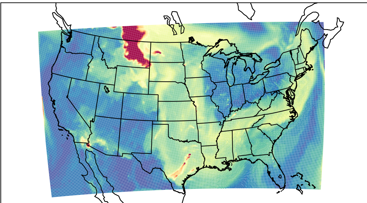
WRF 2023-05-21_15:00:00
