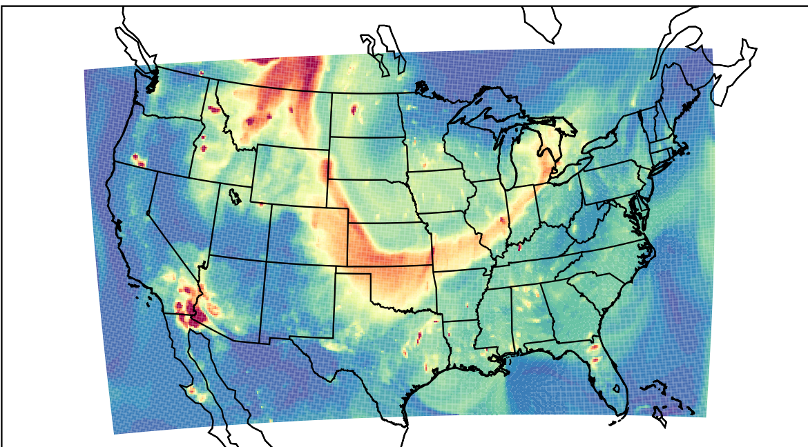
WRF 2023-05-20_03:00:00
