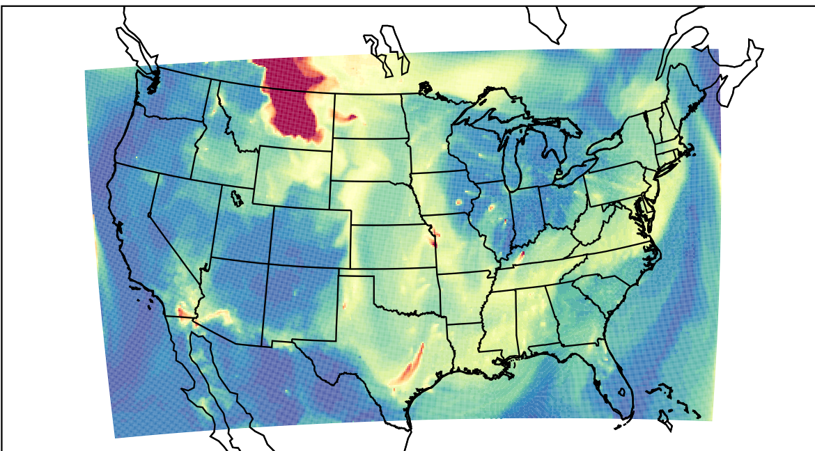
WRF 2023-05-21_11:00:00
