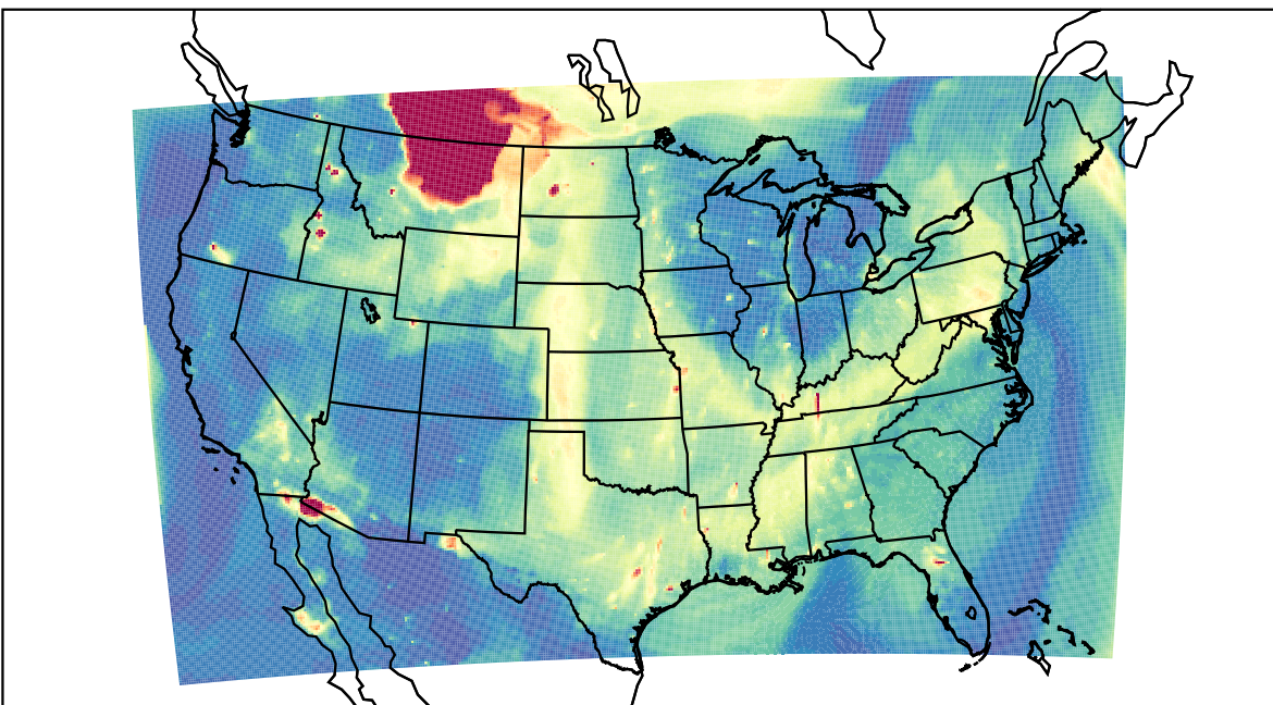
WRF 2023-05-21_03:00:00
