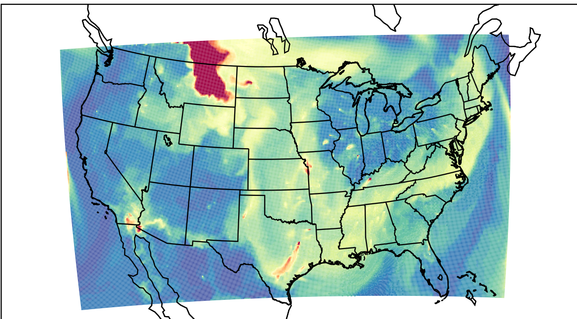
WRF 2023-05-21_13:00:00
