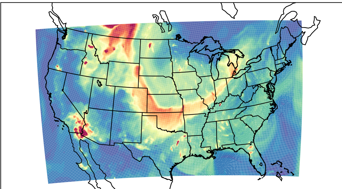
WRF 2023-05-20_04:00:00
