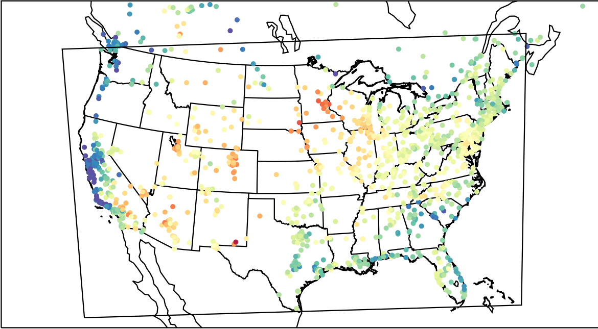
AirNOW (2023-05-21_17:00:00)
