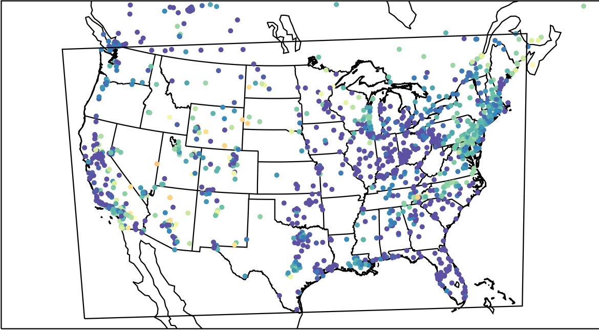
AirNOW (2023-05-21_11:00:00)
