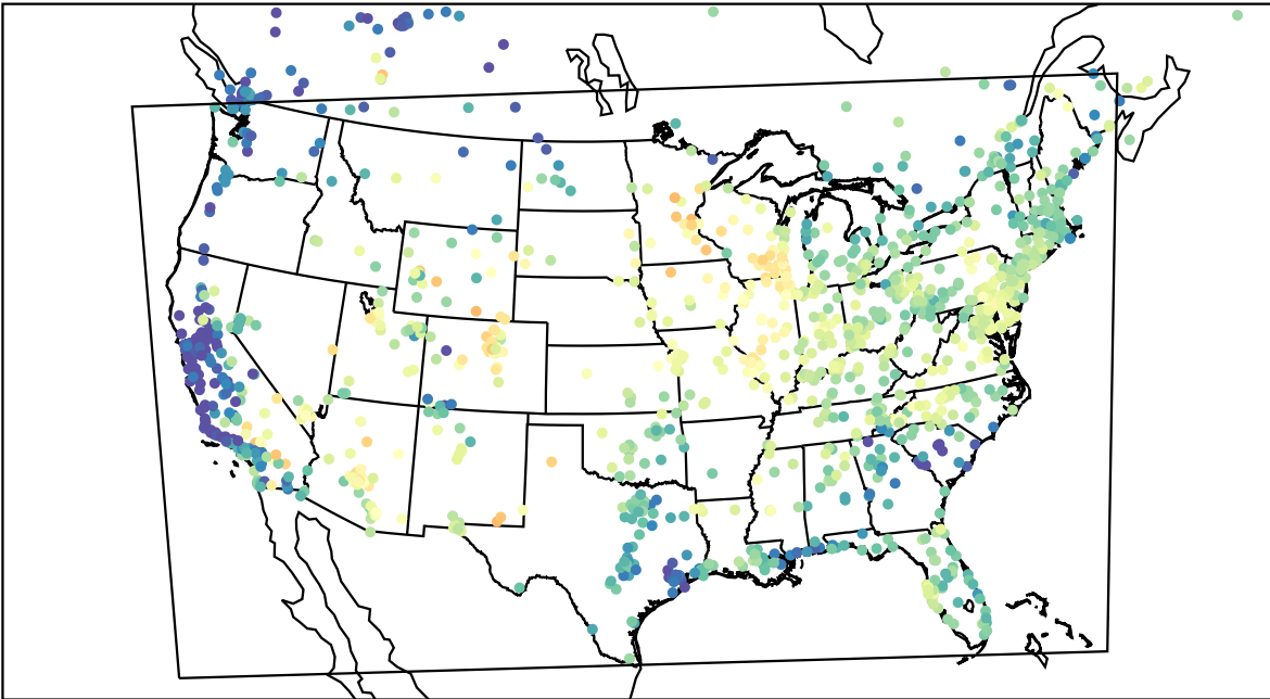
AirNOW (2023-05-21_15:00:00)
