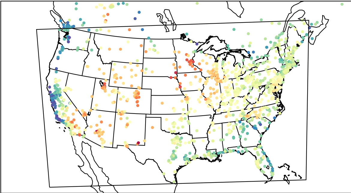
AirNOW (2023-05-21_18:00:00)
