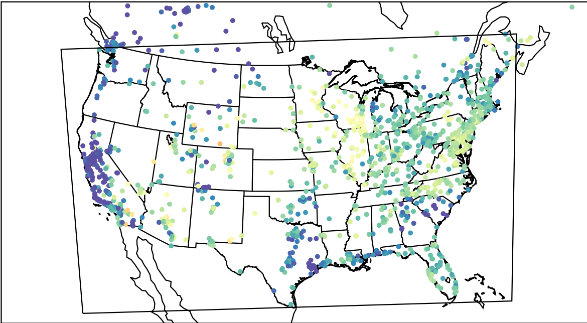
AirNOW (2023-05-21_14:00:00)
