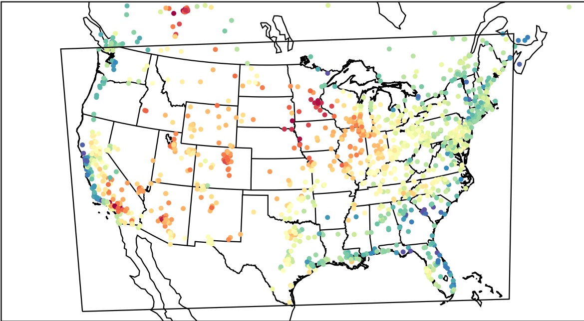
AirNOW (2023-05-21_23:00:00)
