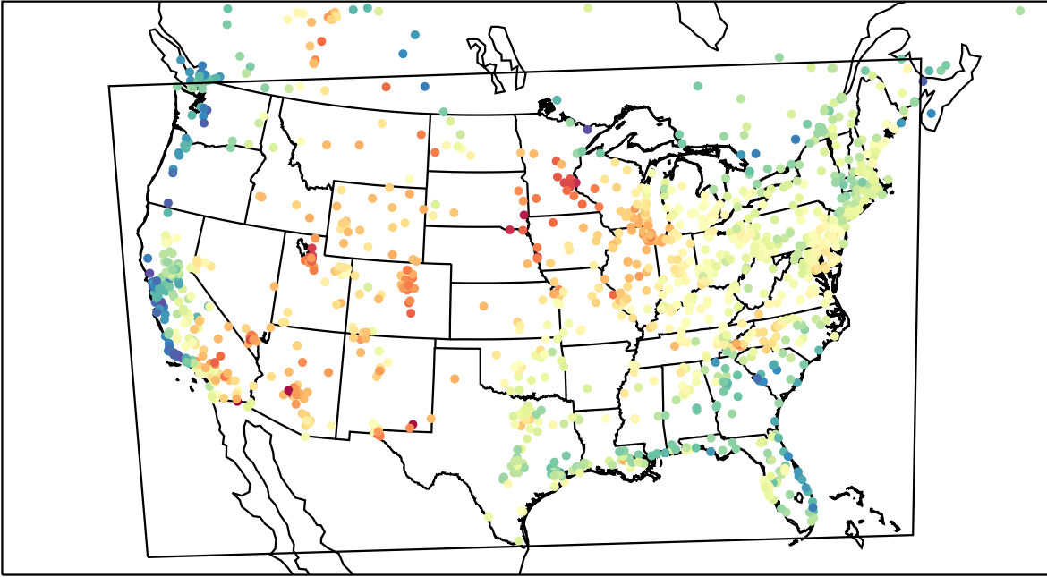
AirNOW (2023-05-21_19:00:00)
