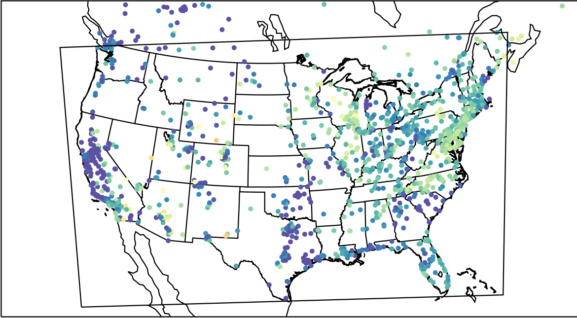
AirNOW (2023-05-21_13:00:00)
