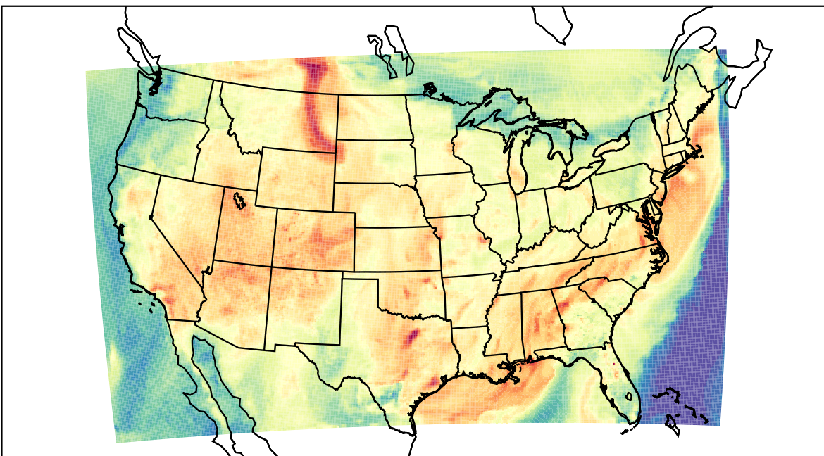
WRF (2023-05-21_20:00:00)
