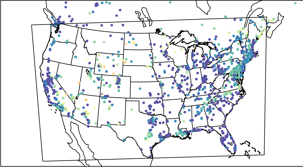
AirNOW (2023-05-21_10:00:00)
