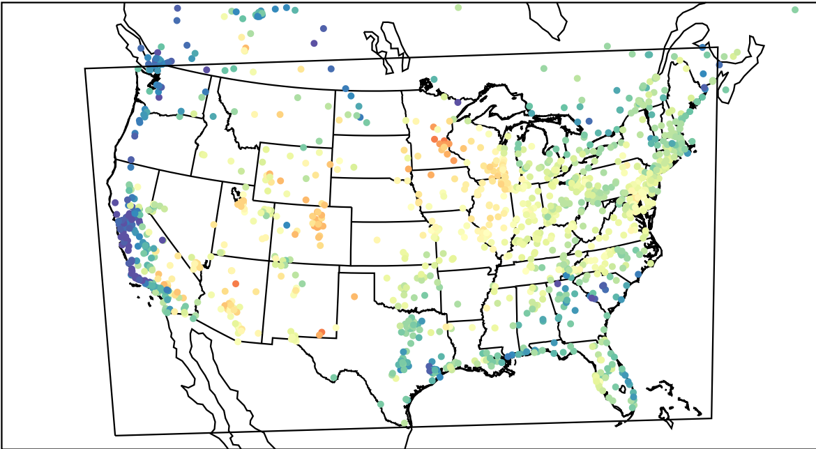
AirNOW (2023-05-21_16:00:00)
