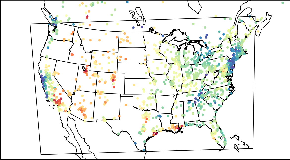
AirNOW (2023-05-20_20:00:00)
