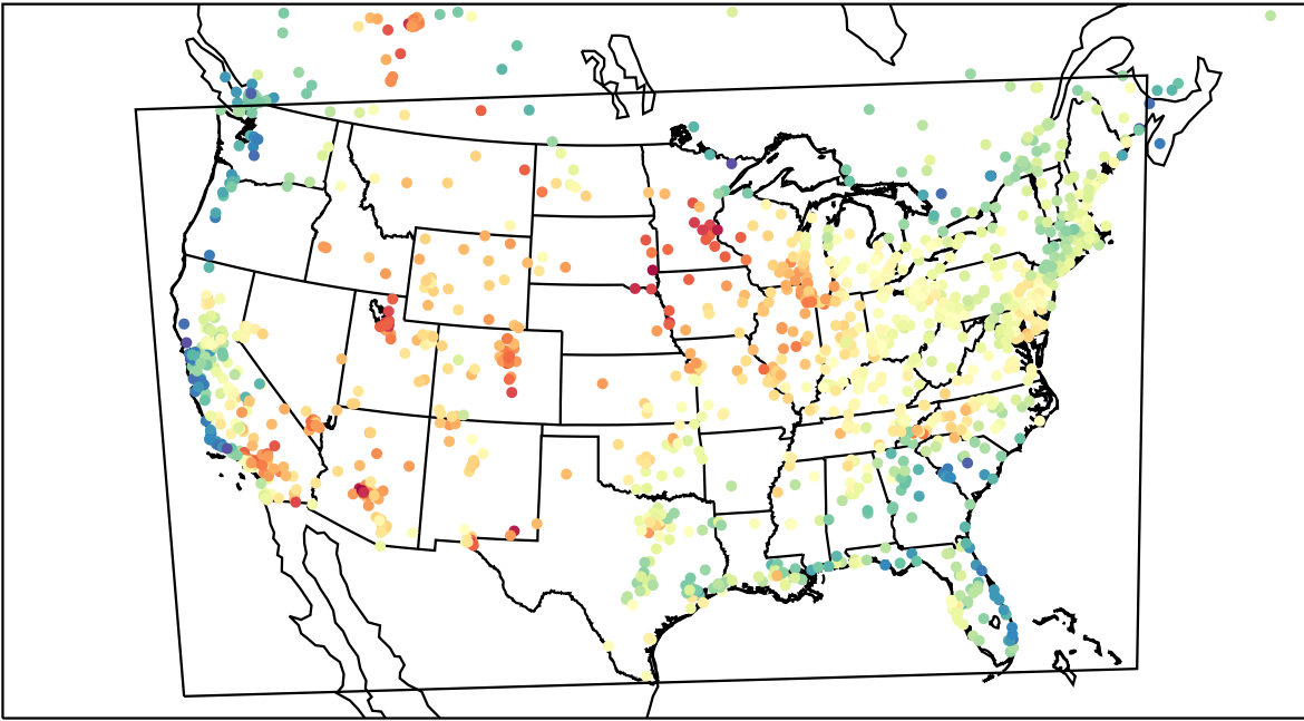
AirNOW (2023-05-21_20:00:00)
