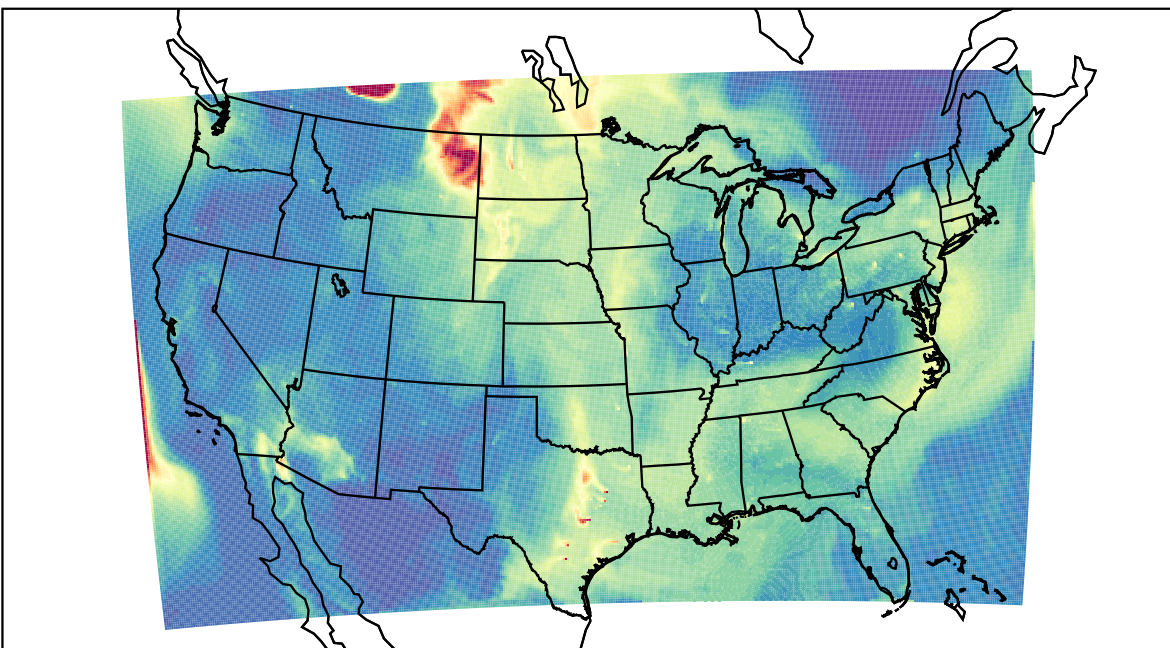
WRF 2023-05-22_17:00:00
