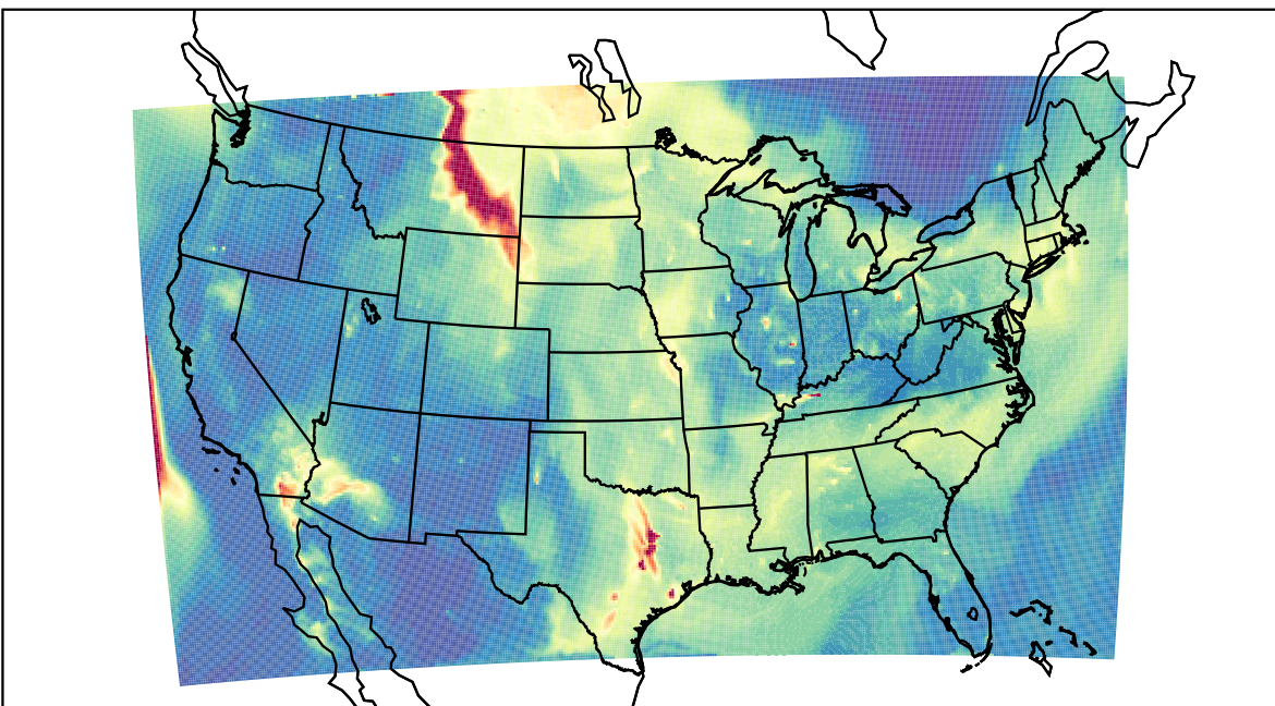
WRF 2023-05-22_10:00:00
