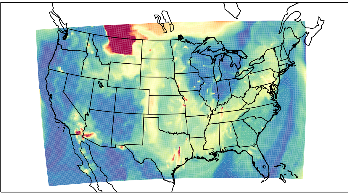
WRF 2023-05-21_06:00:00
