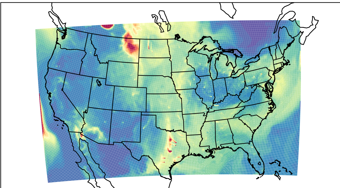
WRF 2023-05-22_15:00:00
