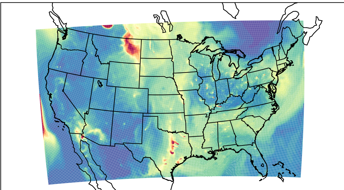
WRF 2023-05-22_14:00:00
