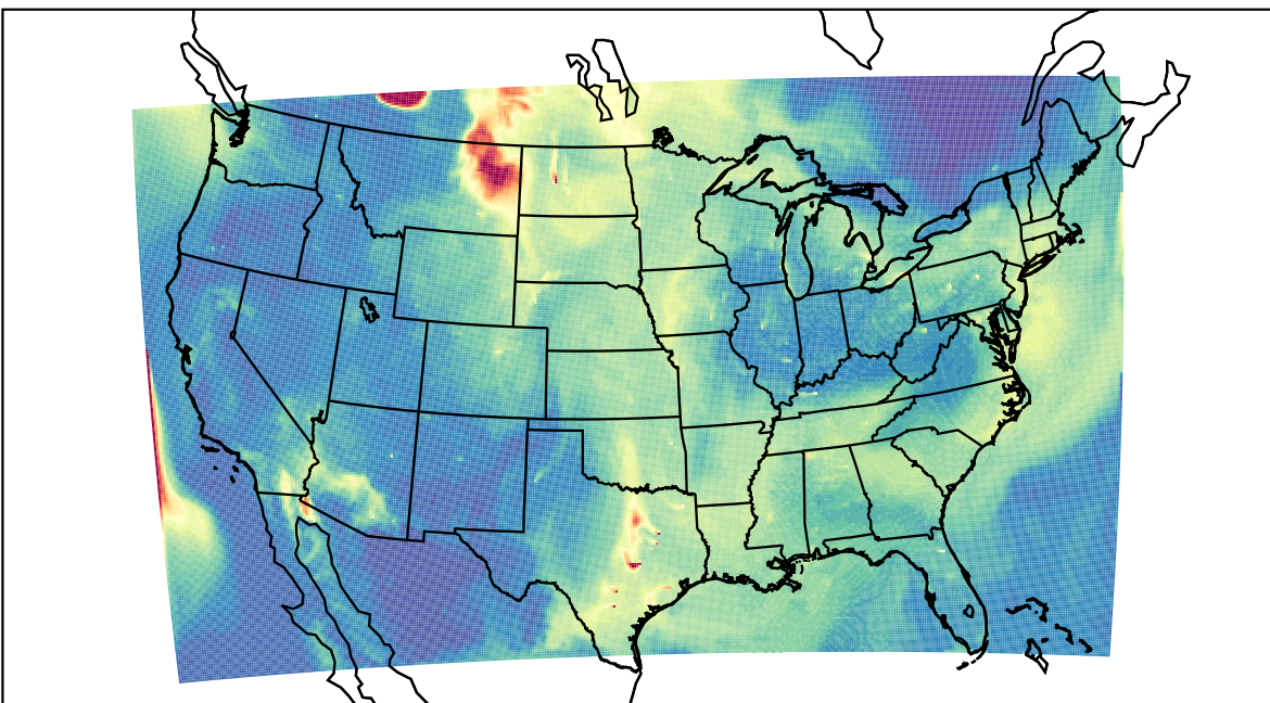
WRF 2023-05-22_16:00:00
