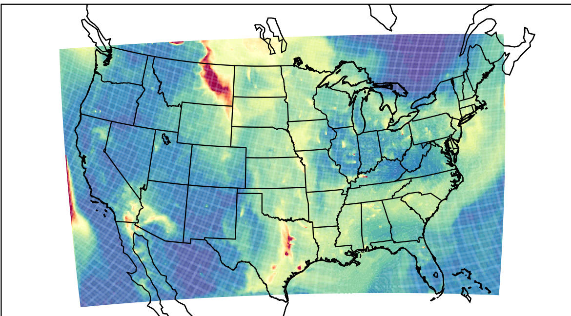
WRF 2023-05-22_12:00:00
