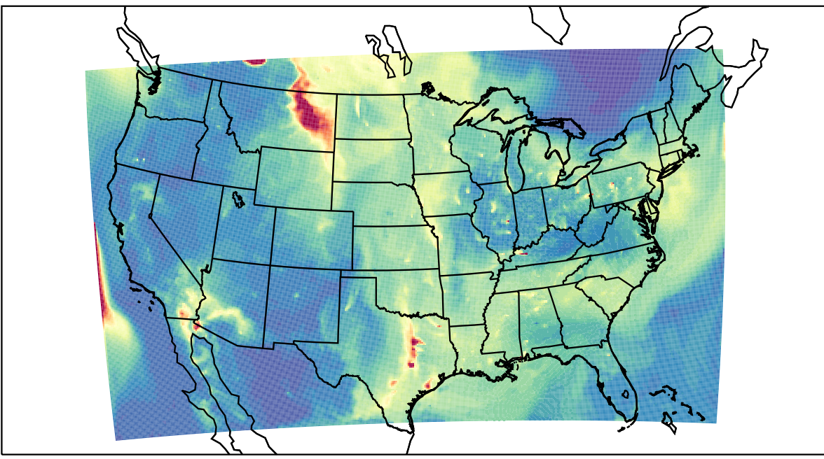
WRF 2023-05-22_13:00:00
