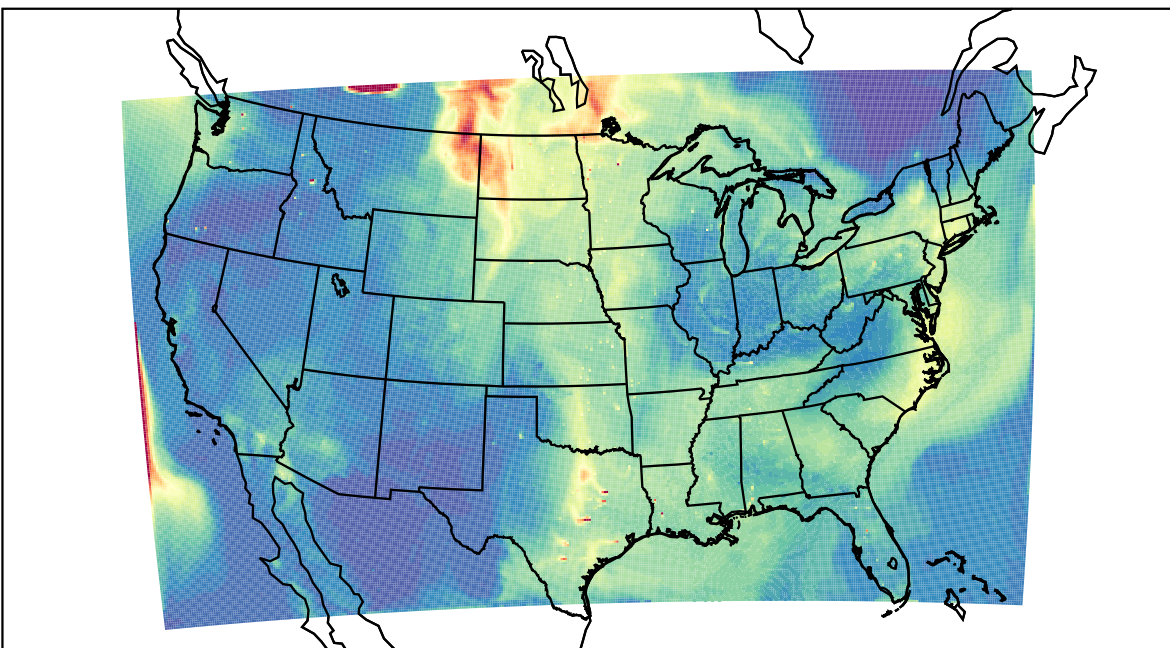
WRF 2023-05-22_20:00:00
