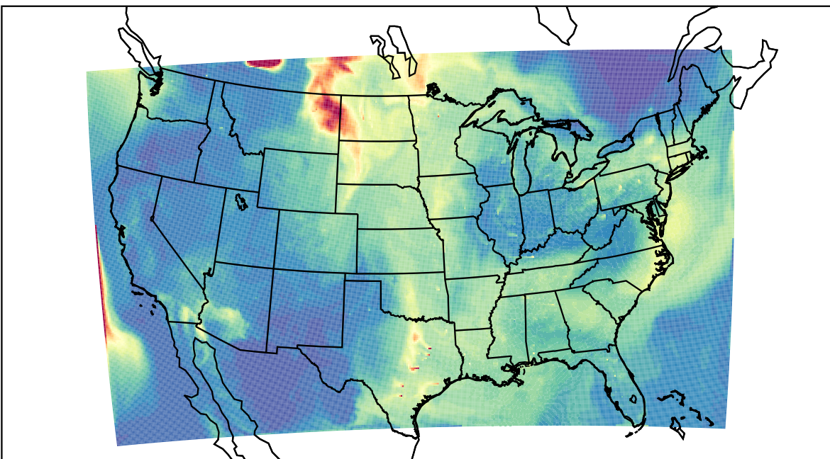
WRF 2023-05-22_18:00:00
