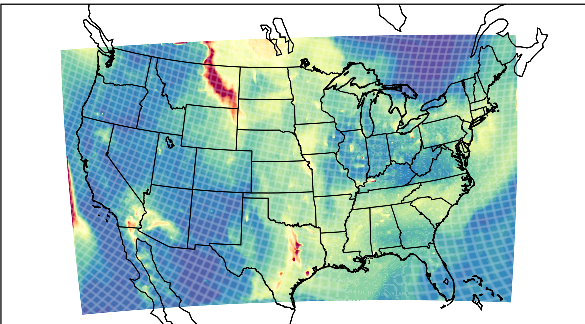
WRF 2023-05-22_11:00:00
