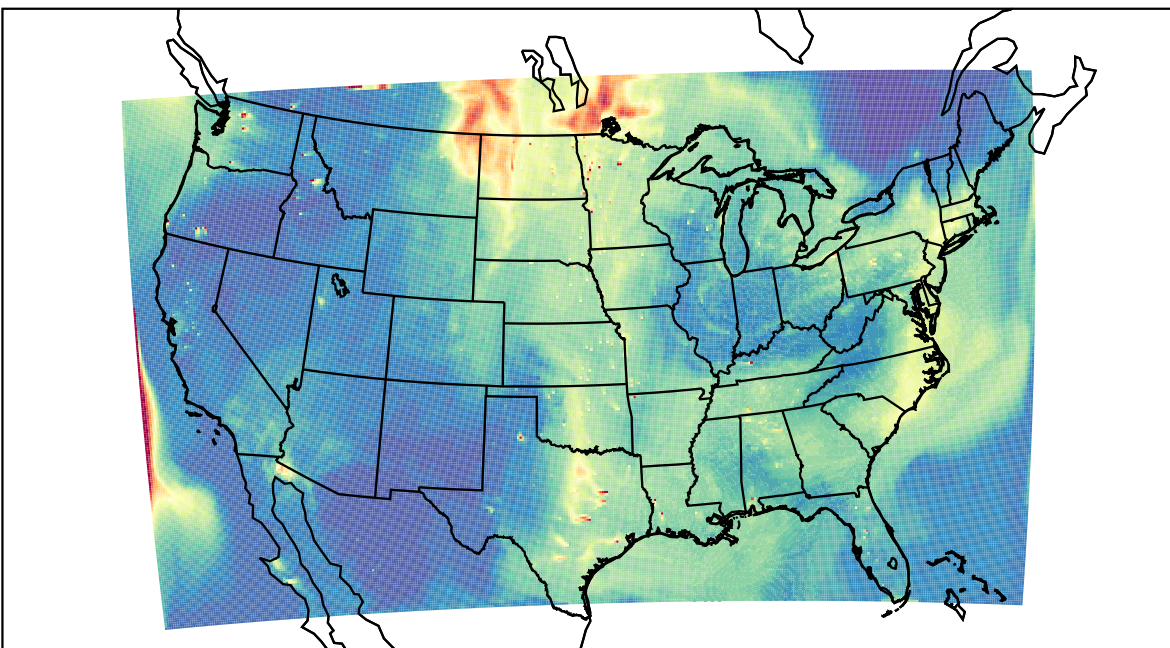
WRF 2023-05-22_23:00:00
