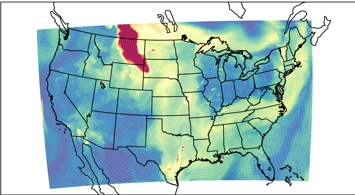
WRF 2023-05-21_18:00:00
